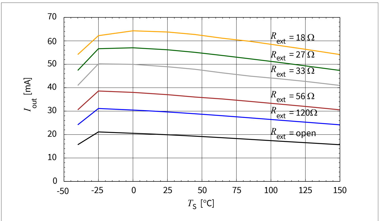
图 3-9 输出电流与 T_S 的关系 I_{out} = f(T_S) , V_S = 10\text{ V} , V_S - V_{out} = 1.4\text{ V} , R_{ext} = \text{Parameter}
