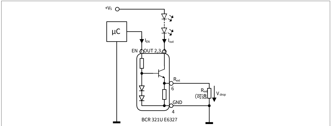
图 4-1 应用电路：通过微控制器启用/PWM
