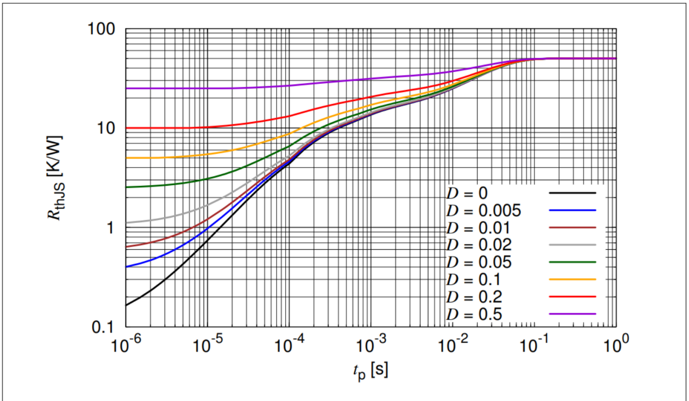
图 3-2 允许脉冲负载 R_{thJS} = f(t_p)
