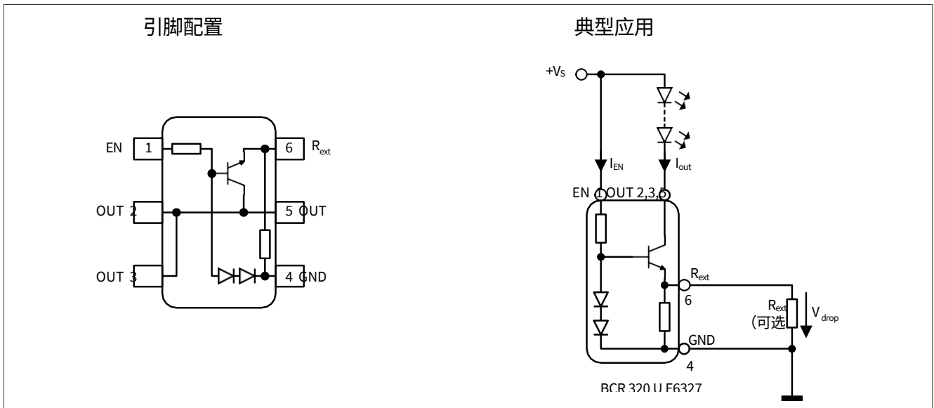
图1-1 引脚配置及典型应用
