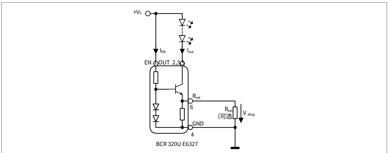
图 4-2 应用电路：通过连接到 V_s 启用
