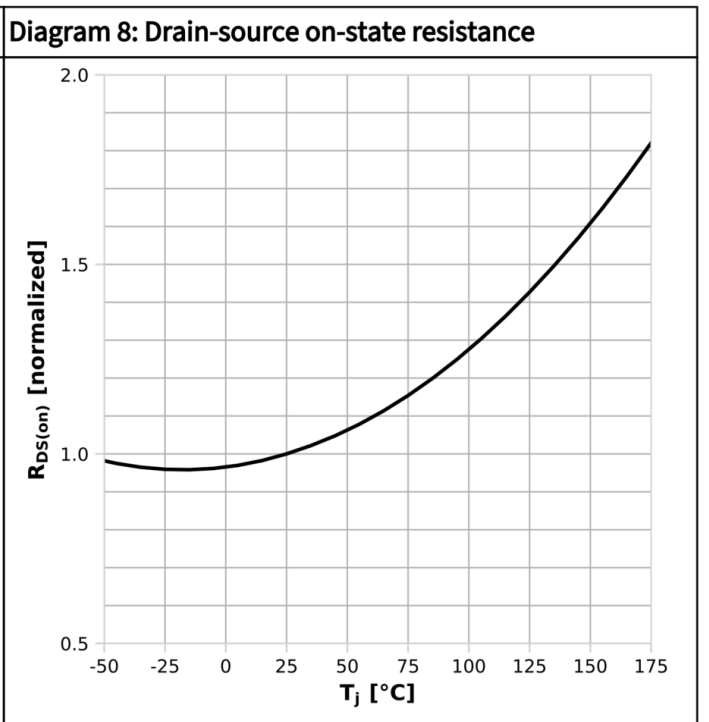
R_{DS(on)}=f(T_J); I_D=17.2 \text{ A}; V_{GS}=18 \text{ V}
