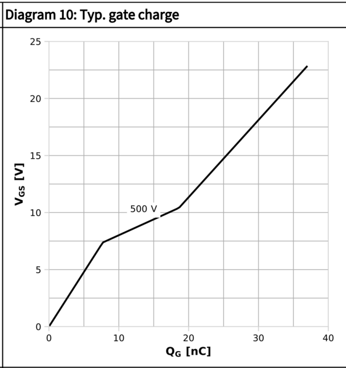
V_{GS}=f(Q_G); I_D=21.7\text{ A pulsed}; \text{parameter: } V_{DD}
