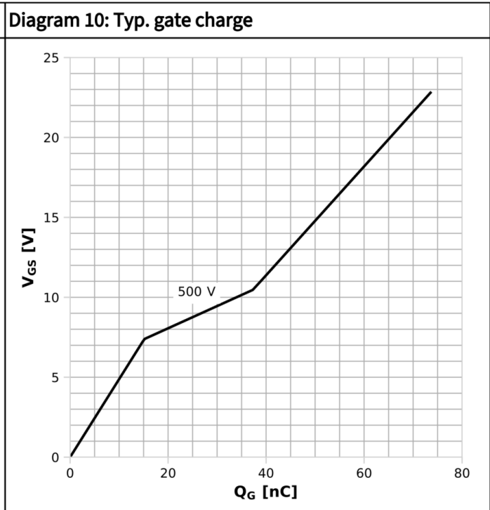
V_{GS}=f(Q_G); I_D=44.7\text{ A pulsed}; \text{parameter: } V_{DD}
