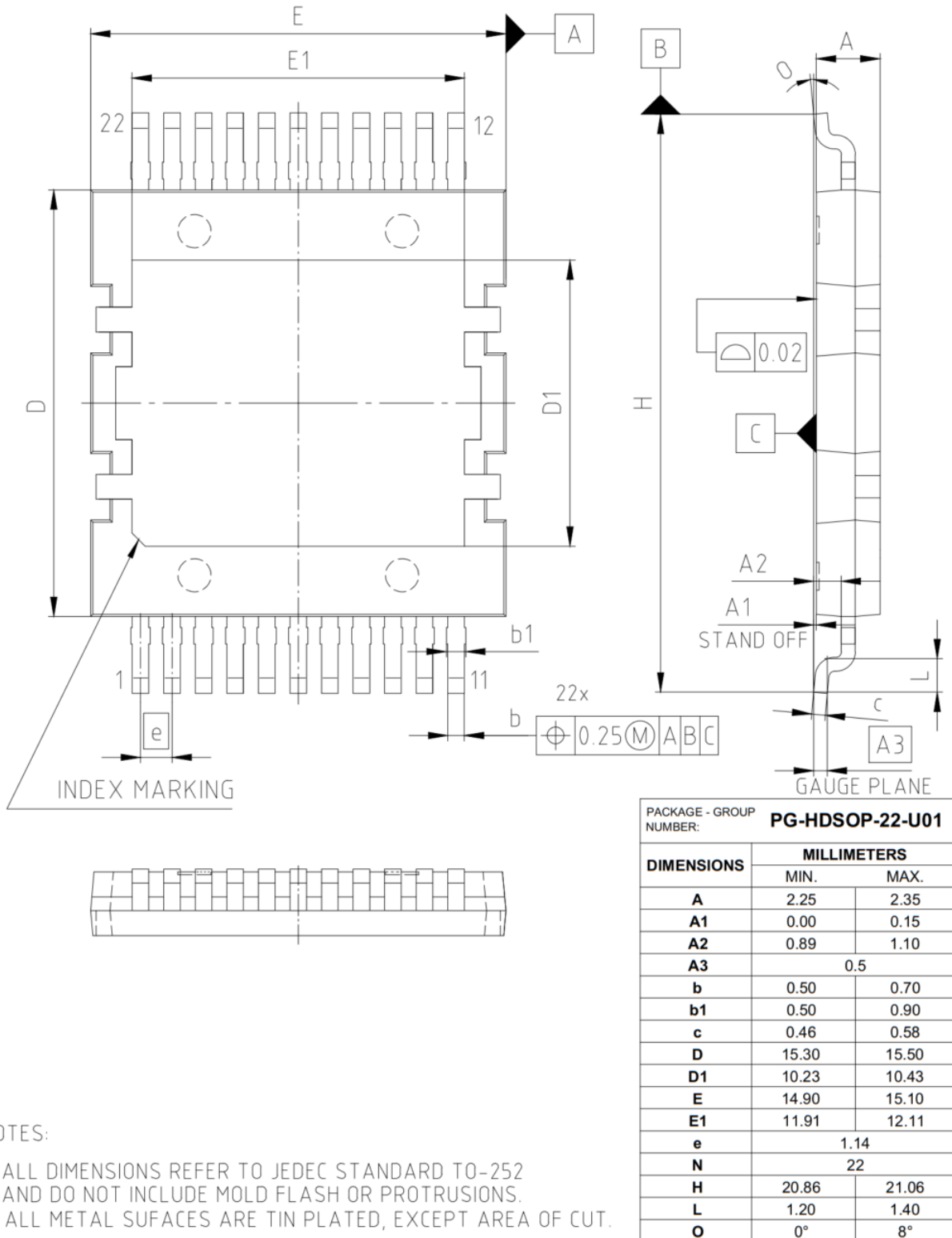
图 1 PG-HDSOP-22 外形图，尺寸单位为毫米
