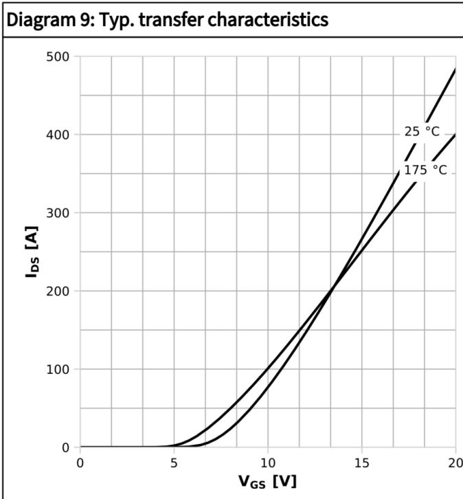
I_{DS}=f(V_{GS}); V_{DS}=20\text{ V}; \text{parameter: } T_j
