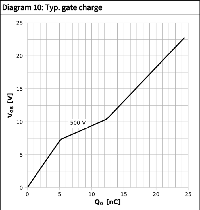
V_{GS}=f(Q_G); I_D=13.8\text{ A pulsed}; \text{parameter: } V_{DD}
