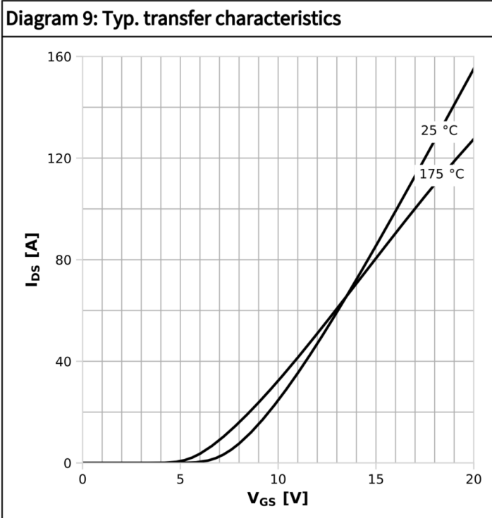
I_{DS}=f(V_{GS}); V_{DS}=20\text{ V}; \text{parameter: } T_j
