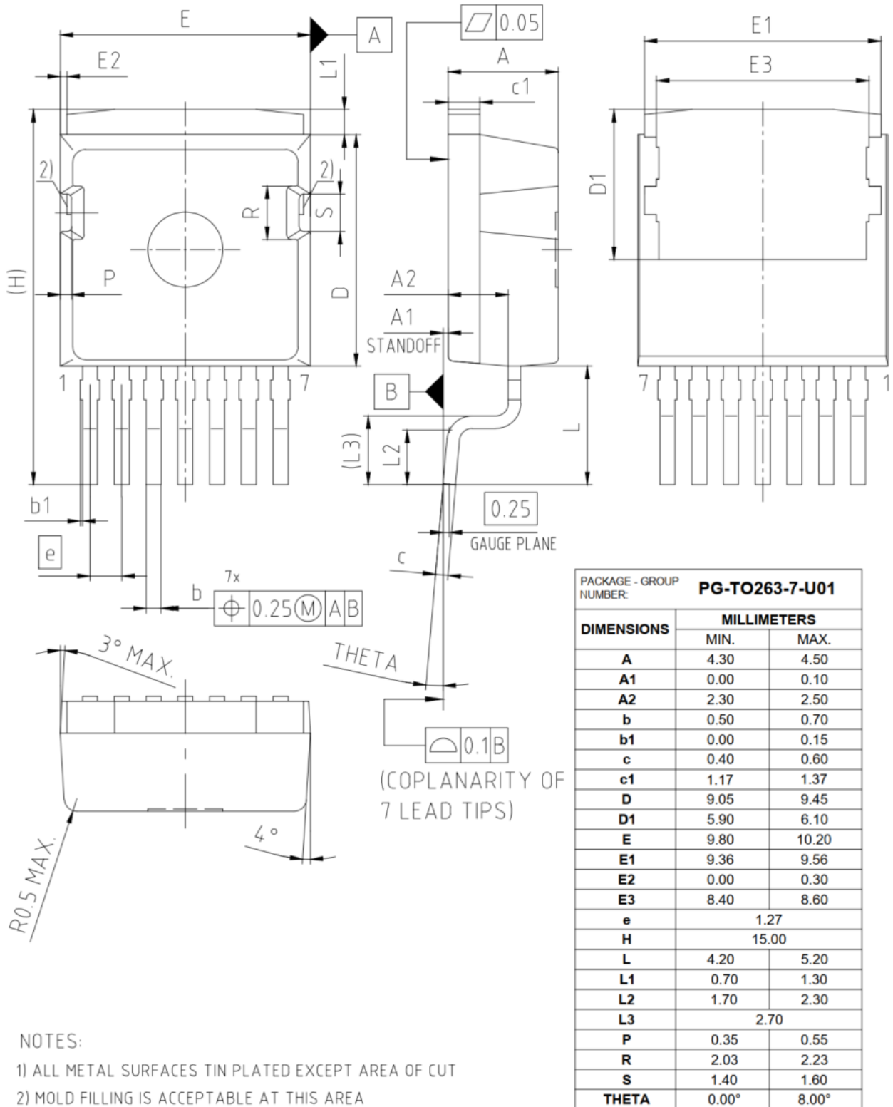
图 1 PG-TO263-7 外形图，尺寸单位为毫米
