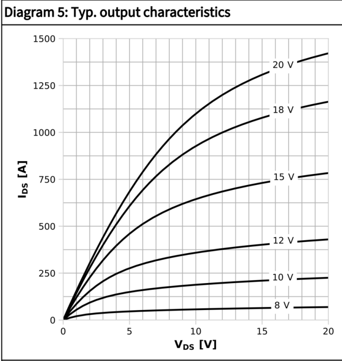
I_{DS}=f(V_{DS}); T_j=25^{\circ}\text{C}; \text{parameter: } V_{GS}
