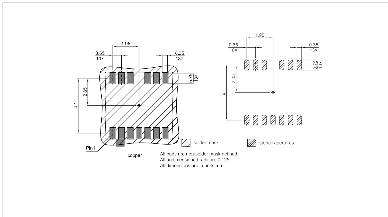
图22 PG-TFLGA-13-4 焊盘
