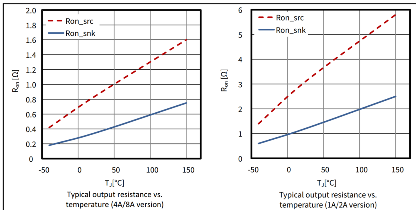
图9 输出电阻
