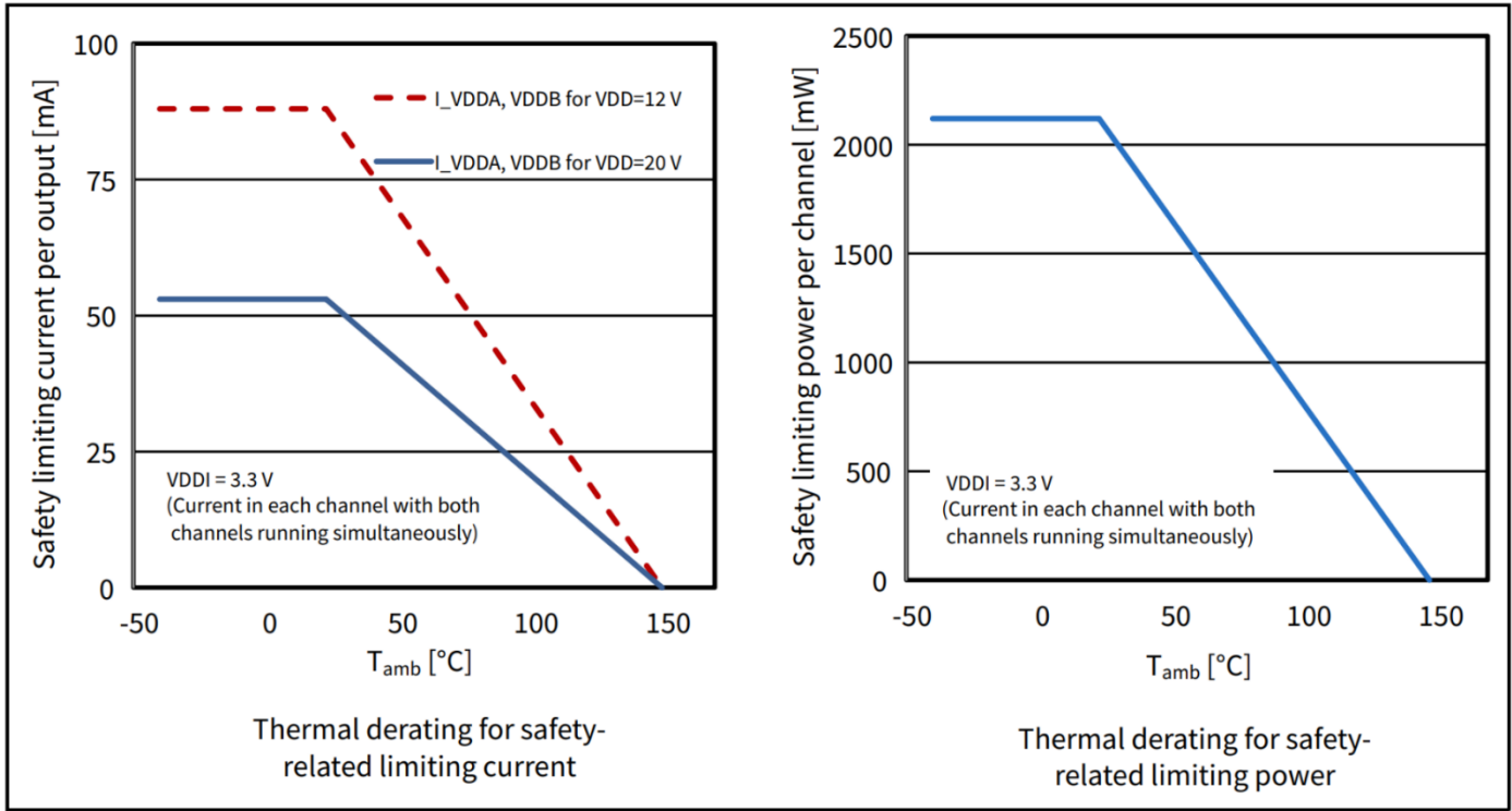
图14 热降额曲线
