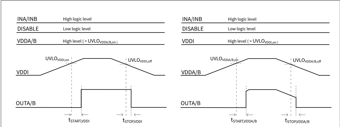
图5 UVLO 行为、启动和停用时间（空载输出）
