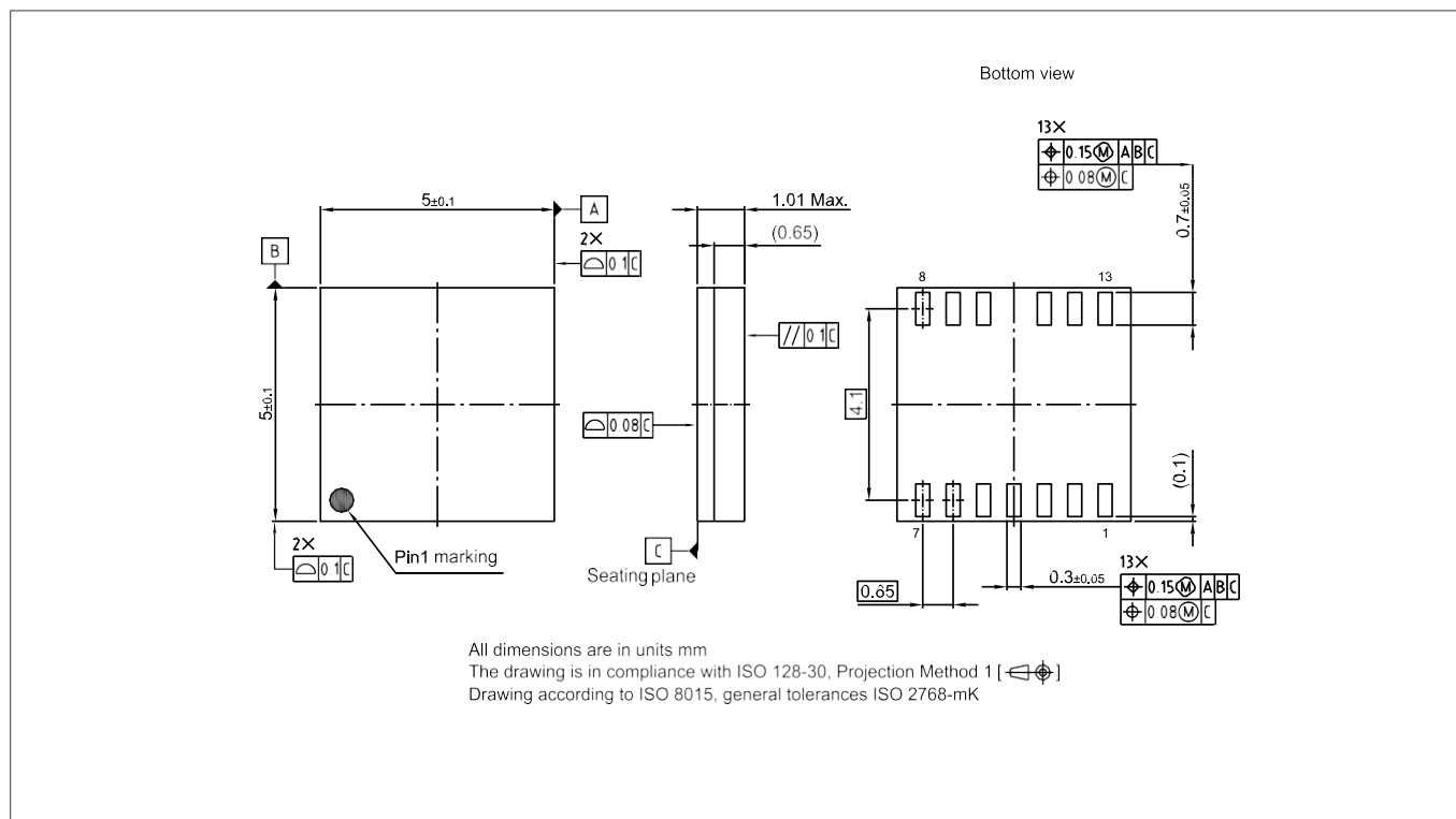
图21 PG-TFLGA-13-4 外形图
