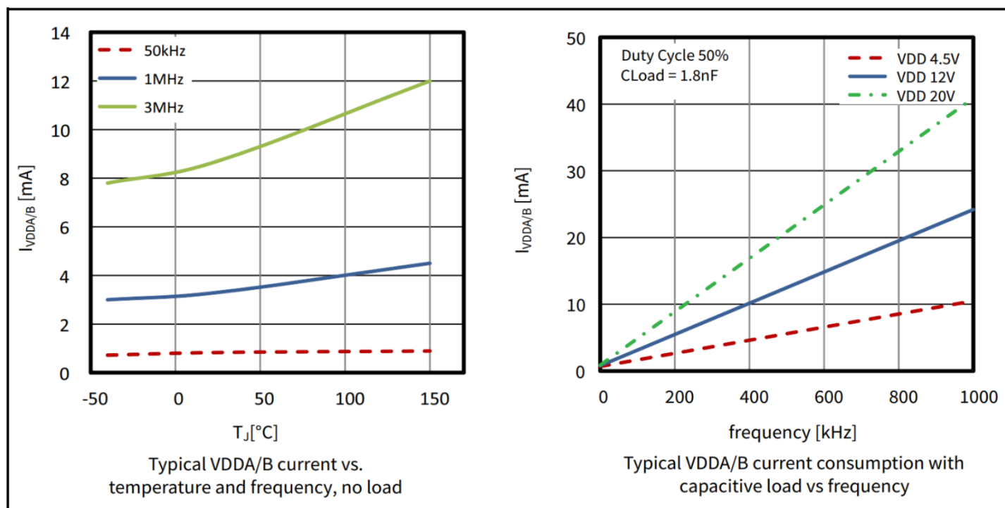
图8 电源电流 VDDA、VDDB (有/无负载)
