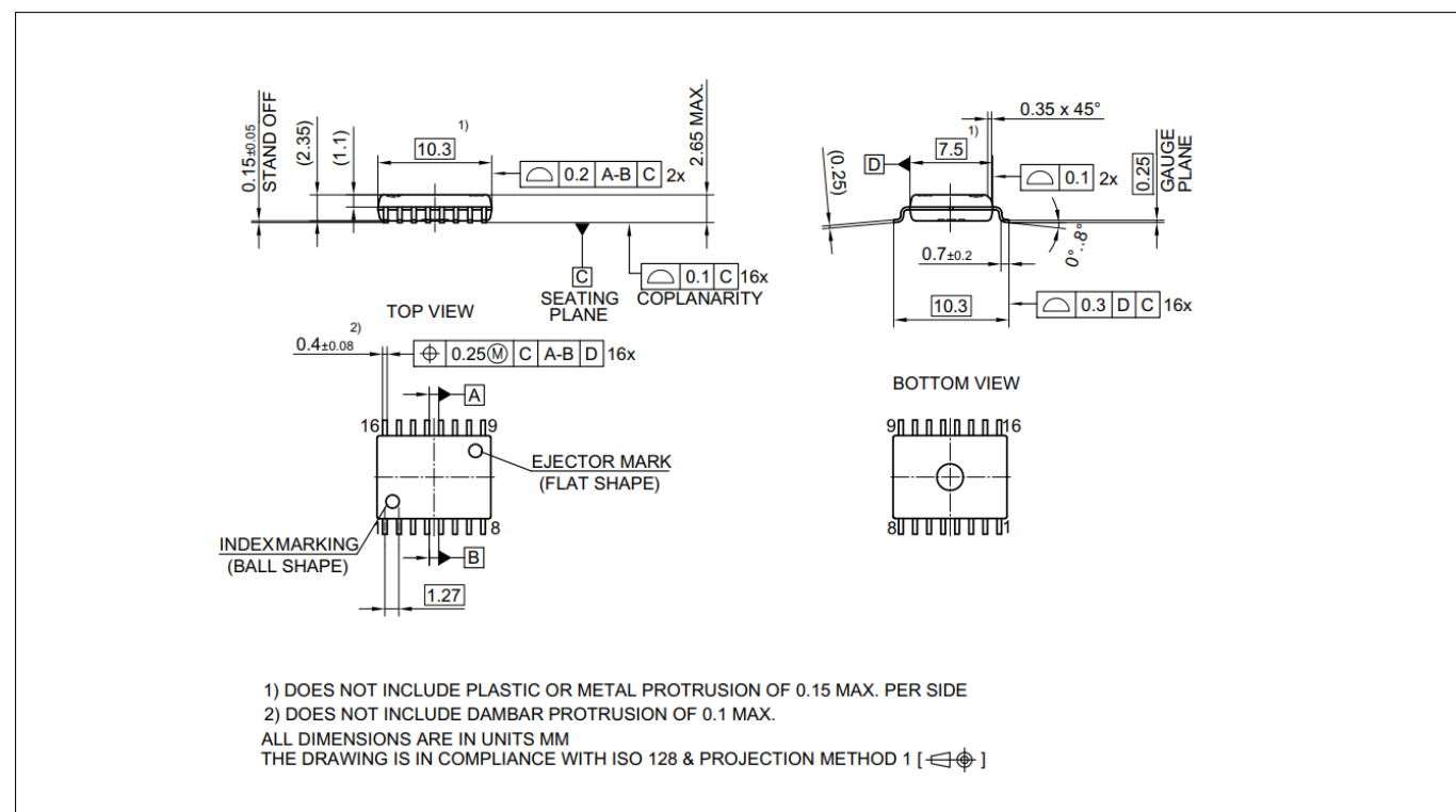
图18 PG-DSO-16-30外形图
