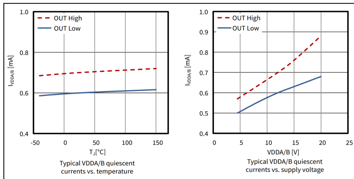
图7 电源电流 VDDA、VDDB
