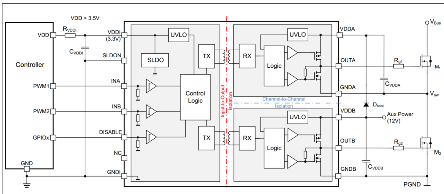
图 1 具有 5 V 控制器和自举高侧 VDDA 的典型应用
