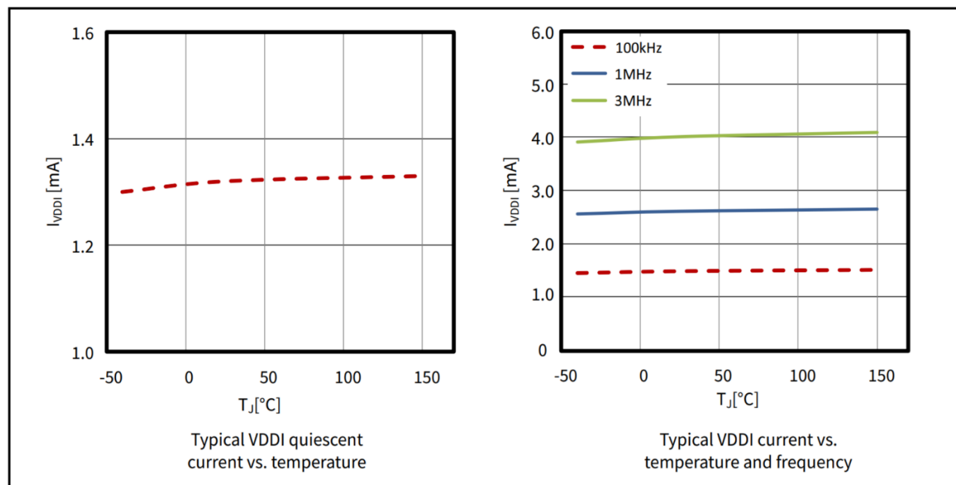
图6 电源电流 VDDI
