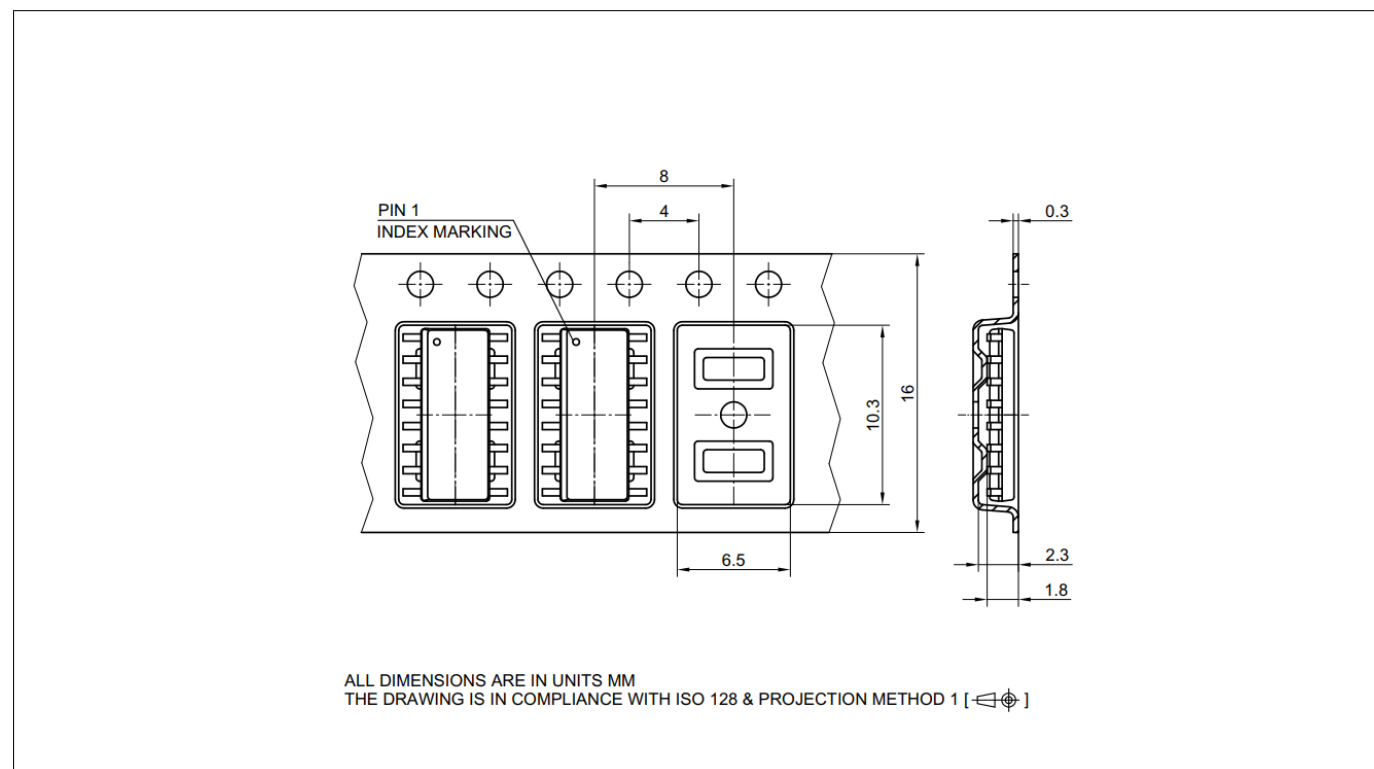
图 17 PG-DSO-16-11封装
