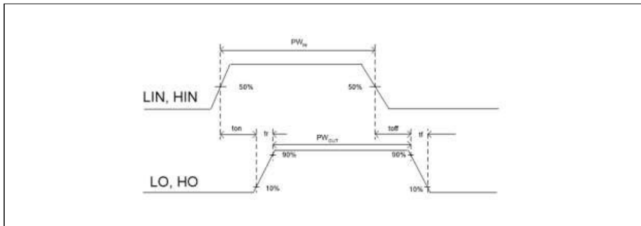
图 6 开关时序图
