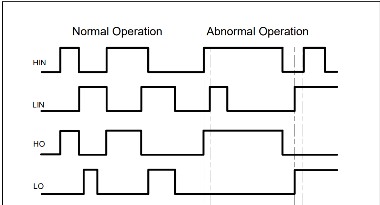
图7 输入/输出时序图
