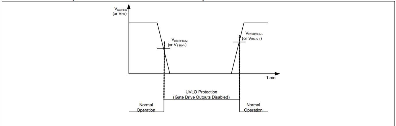
图 11 UVLO 保护
