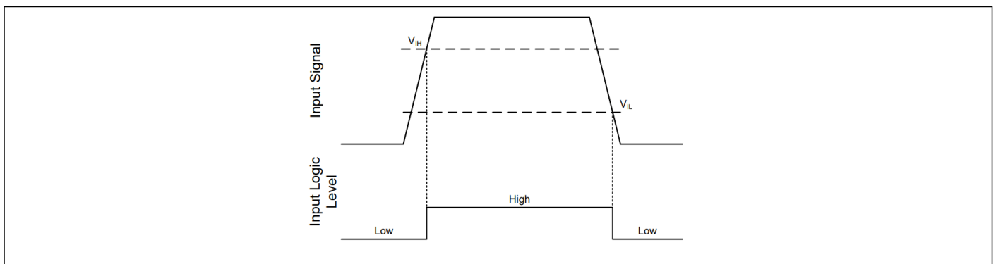
图 10 HIN &amp; LIN 输入阈值
