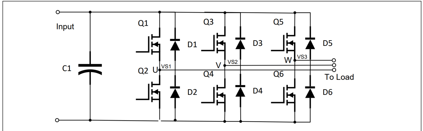
图 15 半桥逆变器
