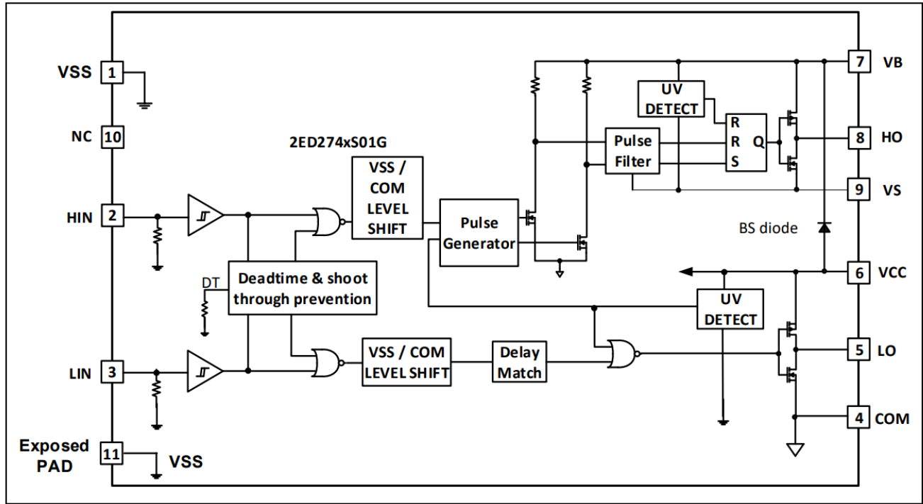
图 2 功能框图
