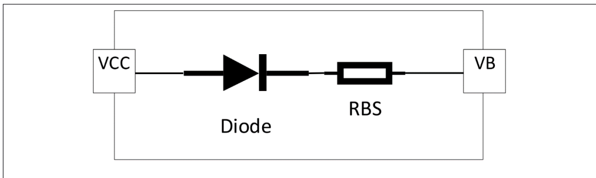
图 13 带集成器件的 2ED2772S01G
