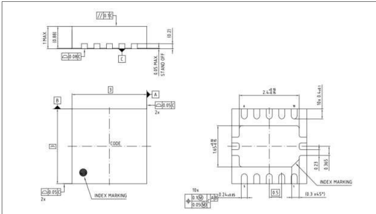
图 21 目标封装尺寸：PG-VSON-10-5 (2ED2772S01G)
