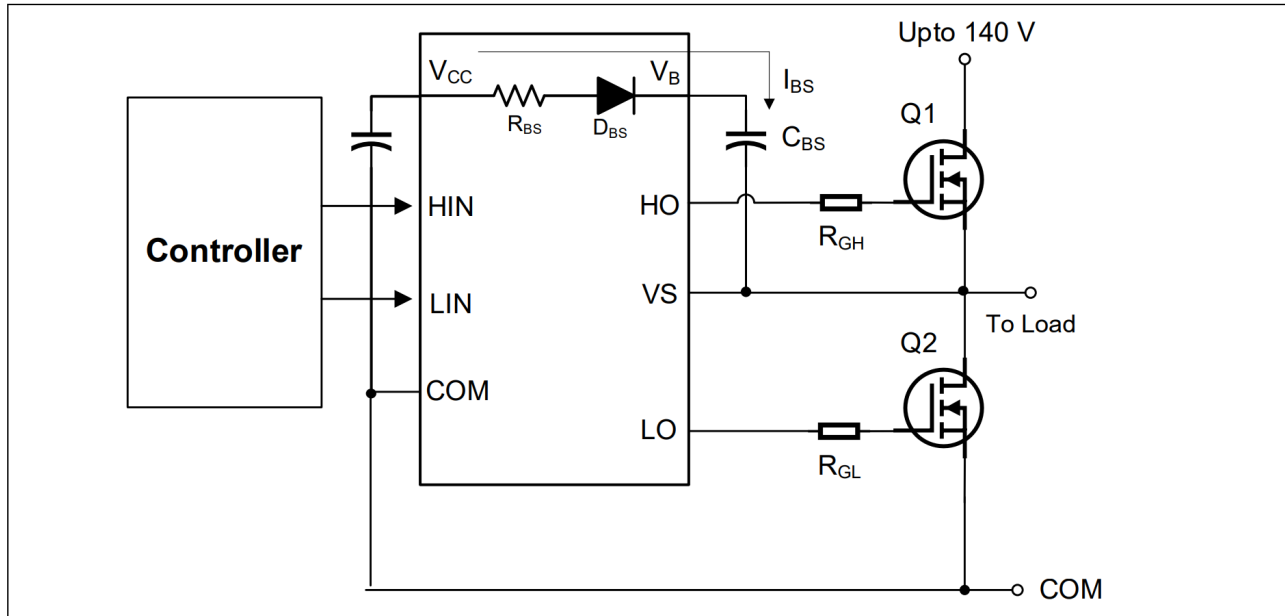
图 14 2ED2772S01G 中的半桥桥自举电路
