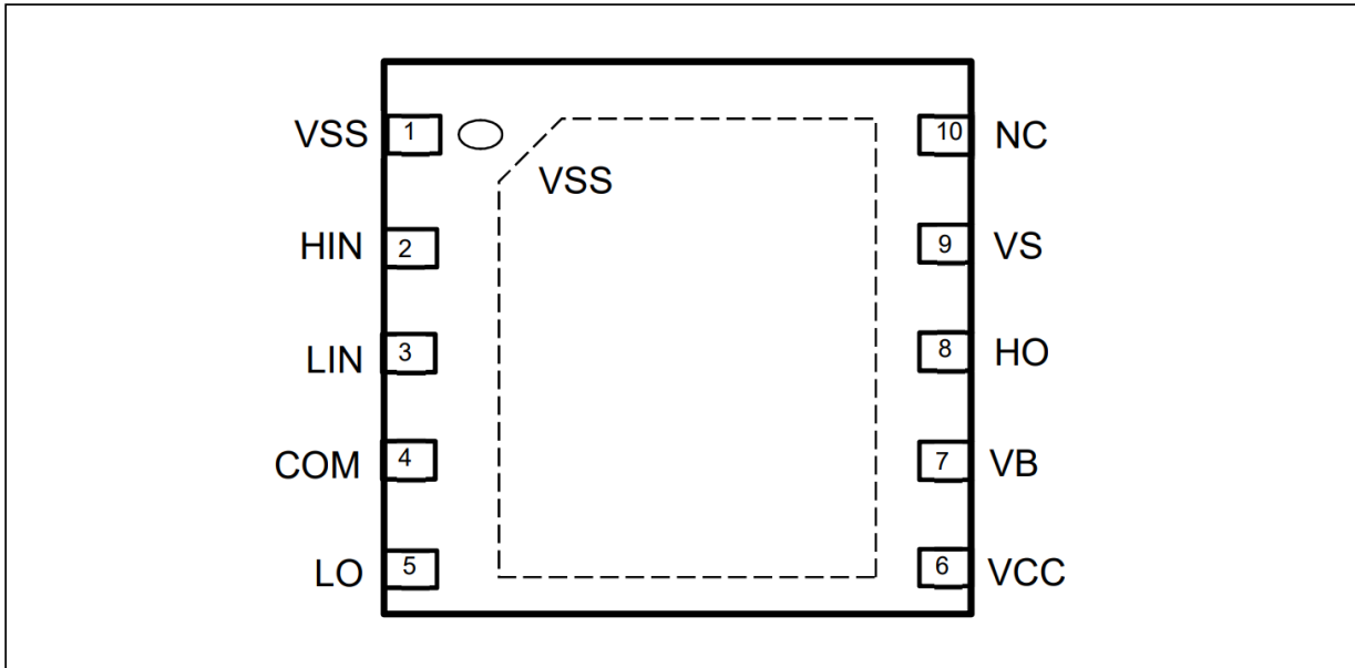
图 3 2ED2748S01G引脚分配（俯视图） 引脚功能
