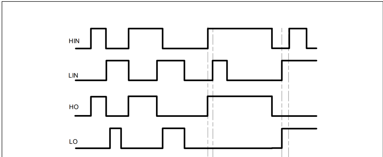
图7 输入/输出时序图
