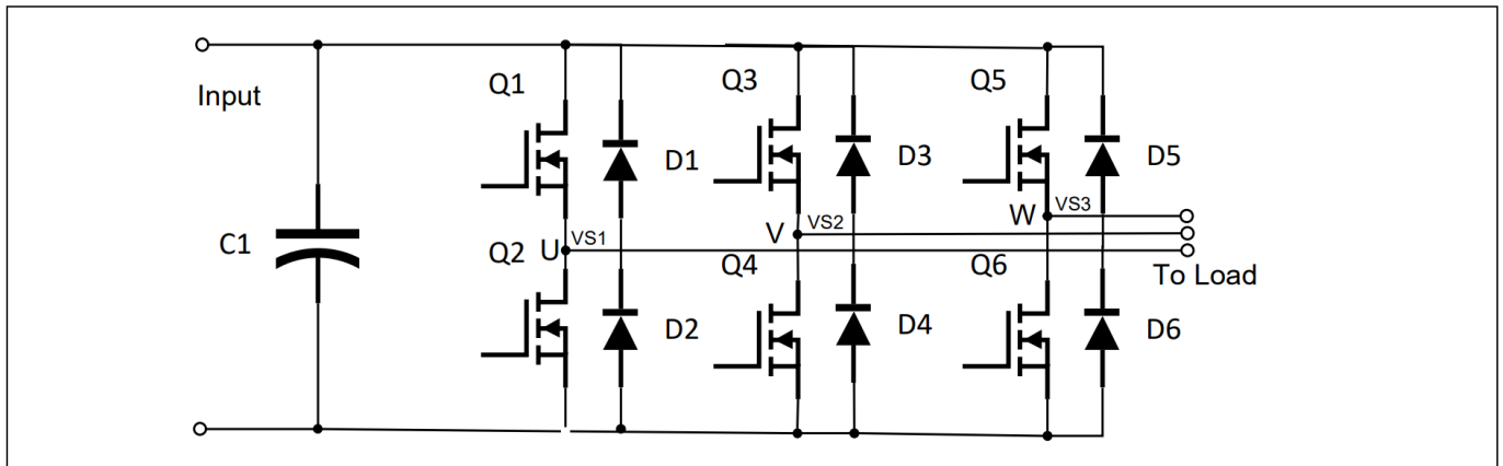
图 15 半桥逆变器
