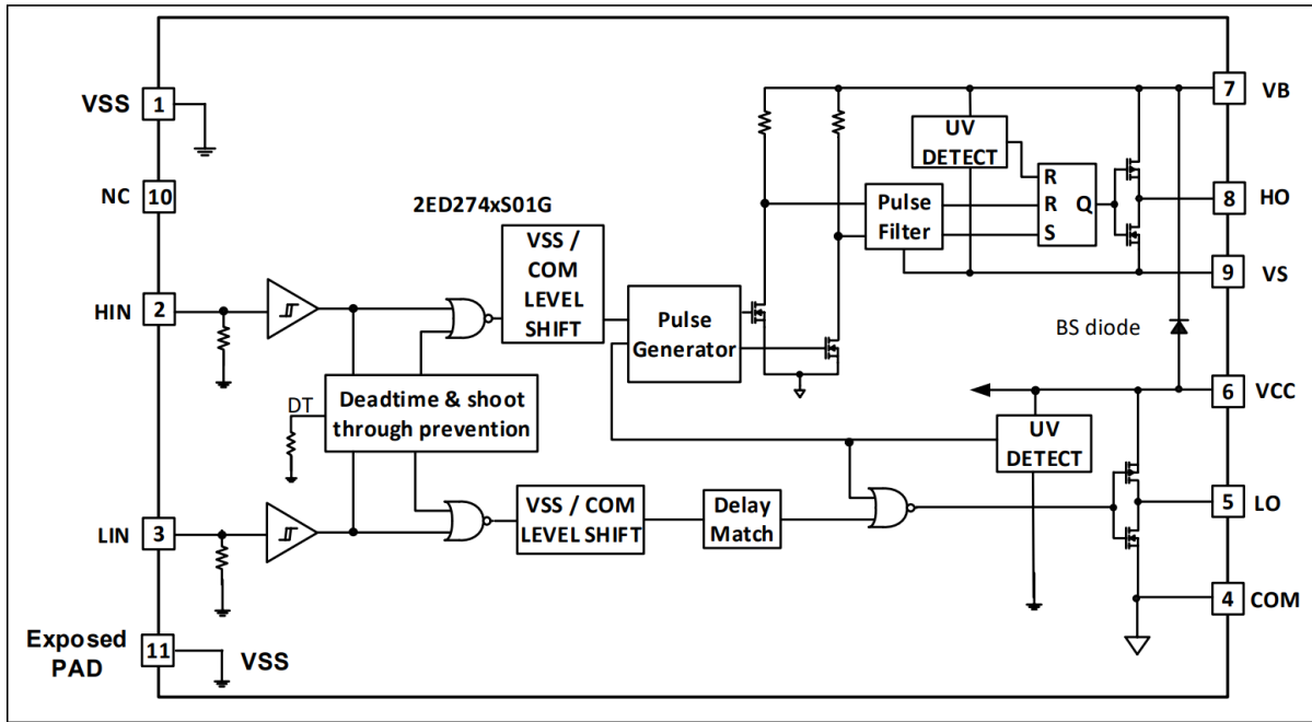
图 2 功能框图
