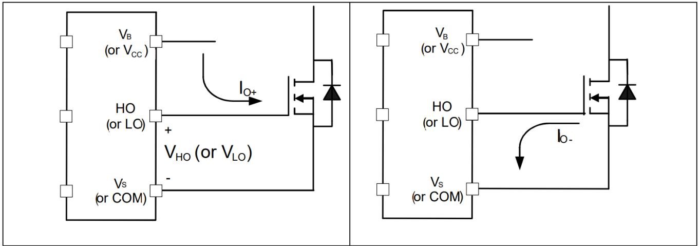
图 4 HVIC 拉电流
