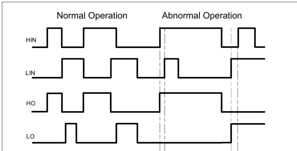
图 12 直通保护电路示意图
