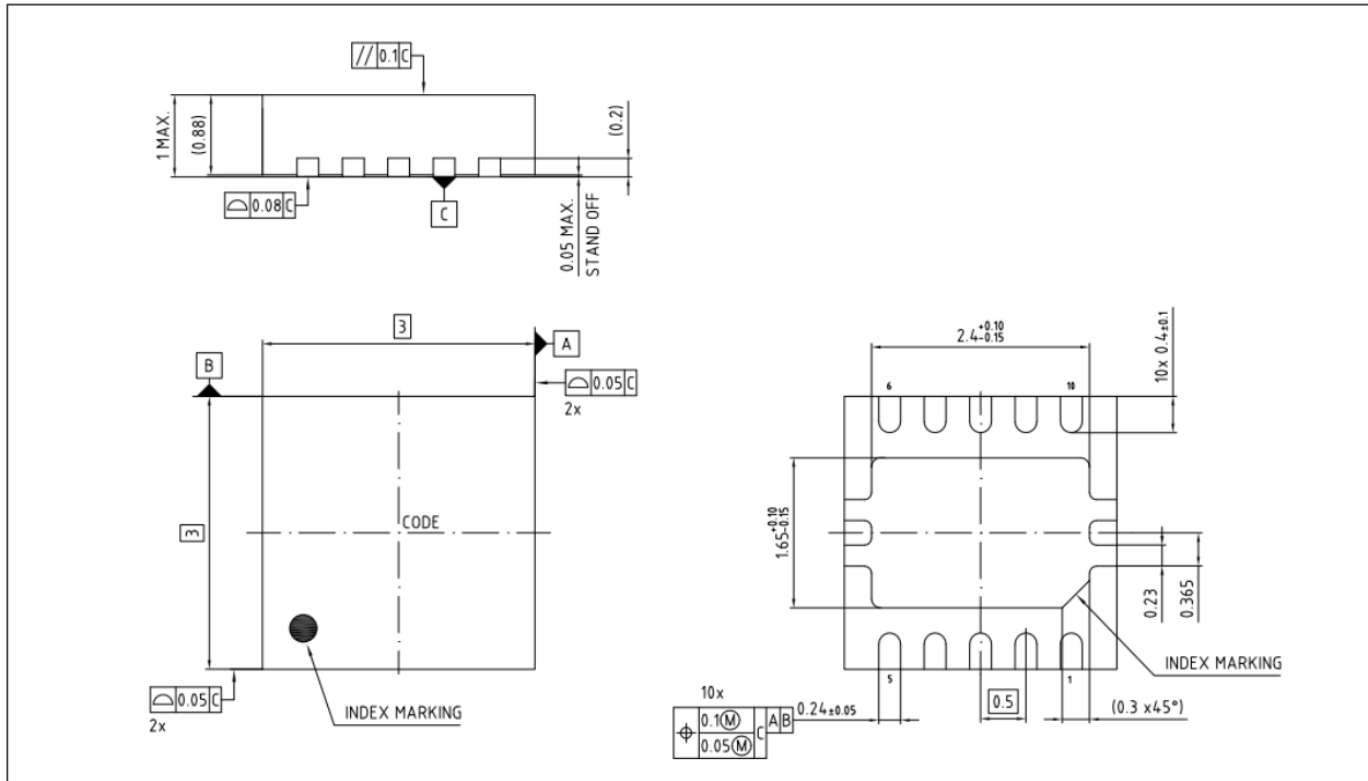
图 21 目标封装尺寸：PG-VSON-10-5 (2ED2748S01G)
