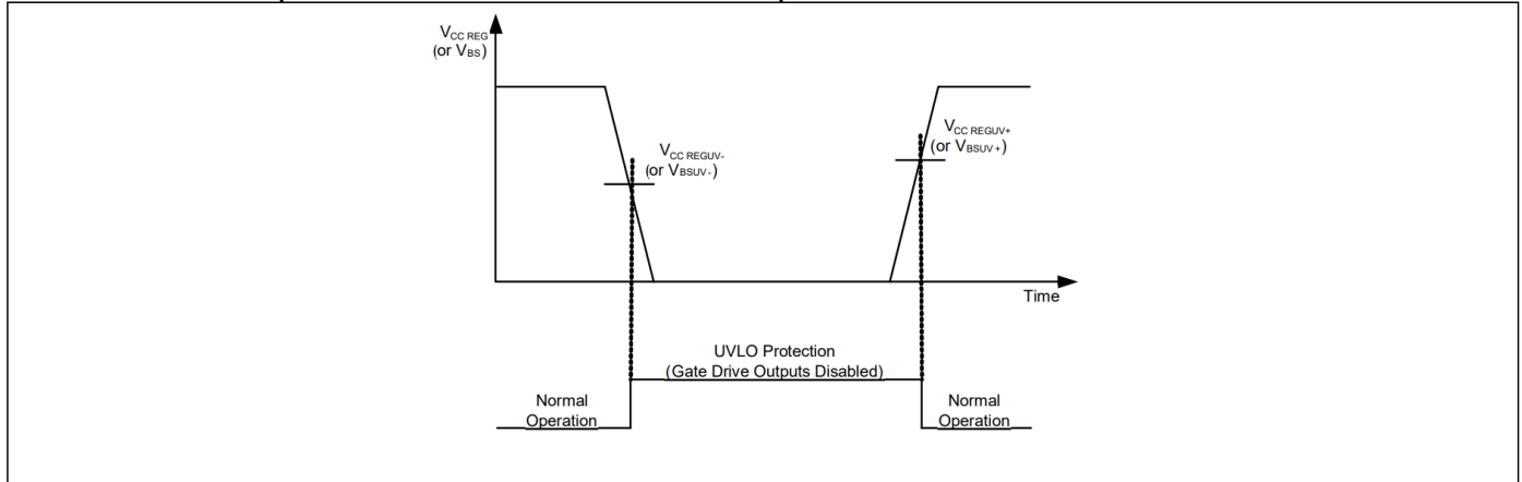
图 11 UVLO 保护
