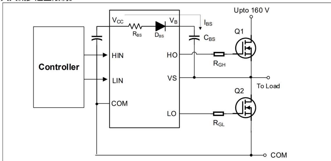
图 14 2ED2748S01G 中的半桥桥自举电路
