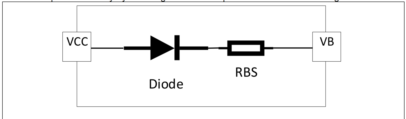
图 13 带集成器件的 2ED2748S01G
