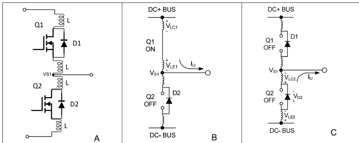
图 17 图 A 显示了寄生元件。图 B 显示了 V_S 正极的产生。图 C 显示了 V_S 负极的产生
