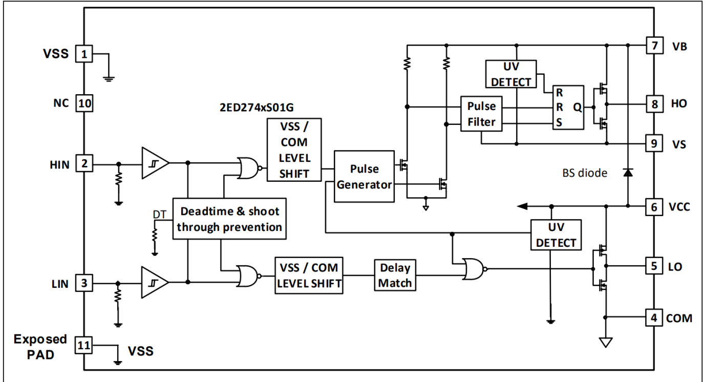
图 2 功能框图
