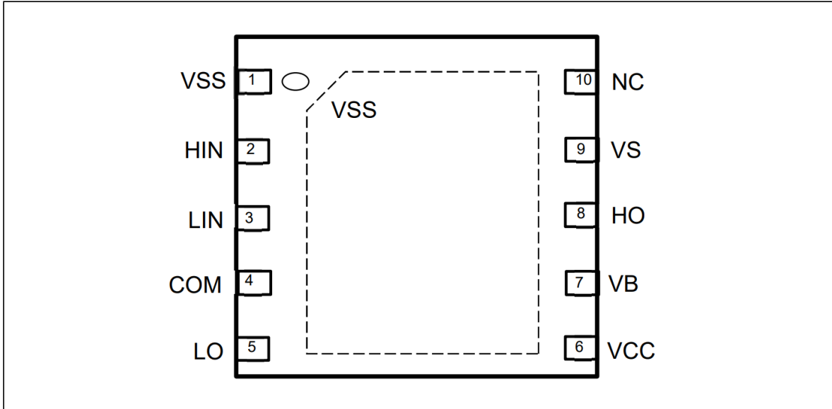
图 3 2ED2742S01G引脚分配（俯视图） 引脚功能
