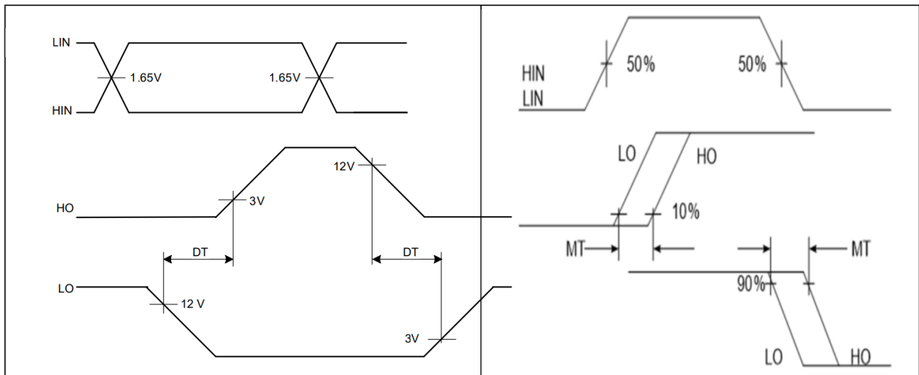
图 8 死区时间定义
