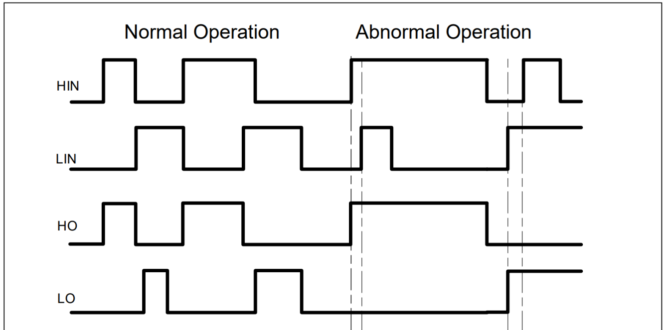
图 12 直通保护电路示意图
