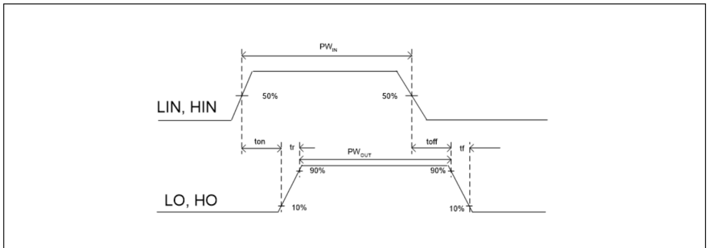
图 6 开关时序图
