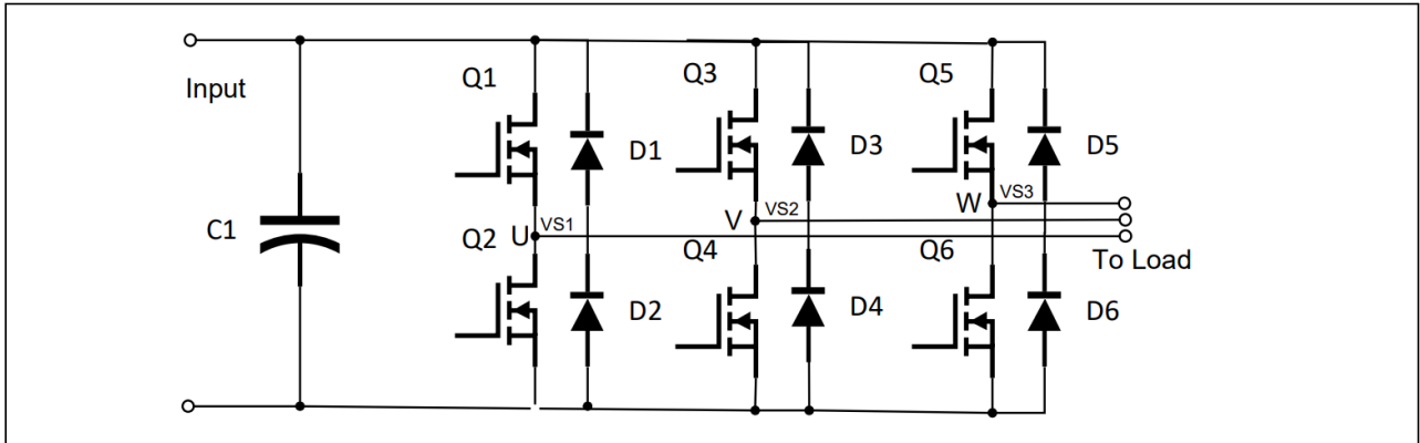
图 15 半桥逆变器
