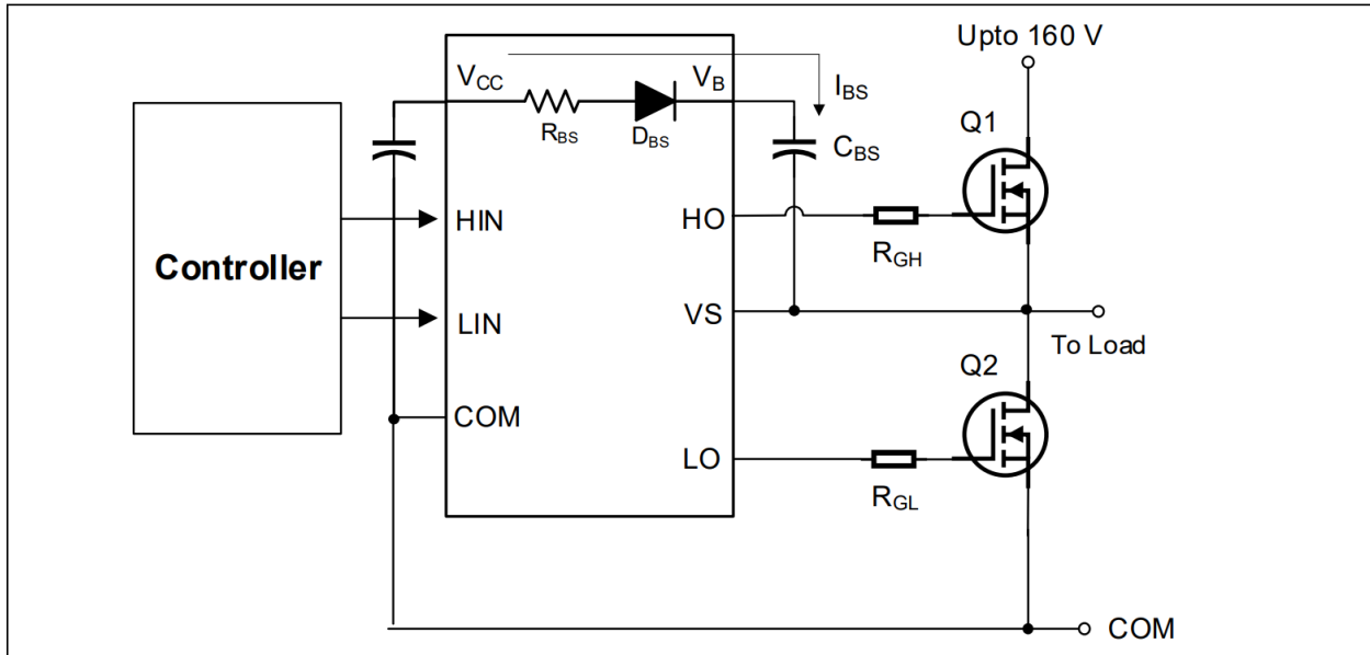
图 14 2ED2742S01G中的半桥桥自举电路
