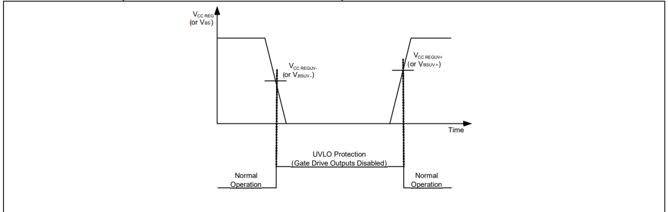
图 11 UVLO 保护
