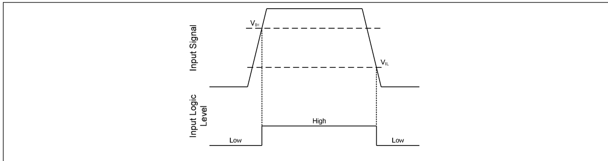
图 10 HIN & LIN 输入阈值
