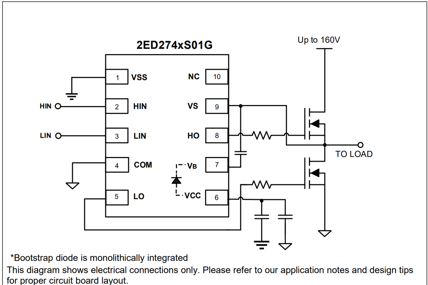
图 1 典型应用框图
