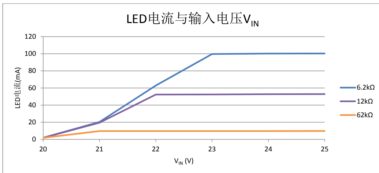
图13 LED 电流与输入电压（室温条件下）
