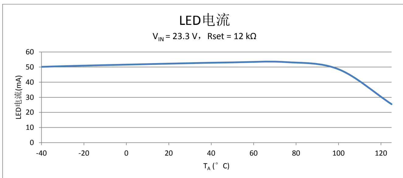
图8 LED 电流与 T_A
