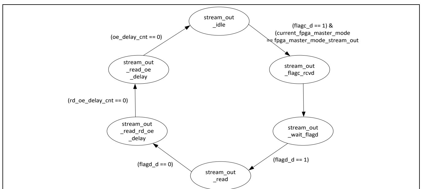
Figure 26 串流 OUT 传输的状态机
