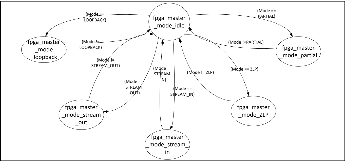
Figure 22 用于选择模式的 FPGA 状态机
