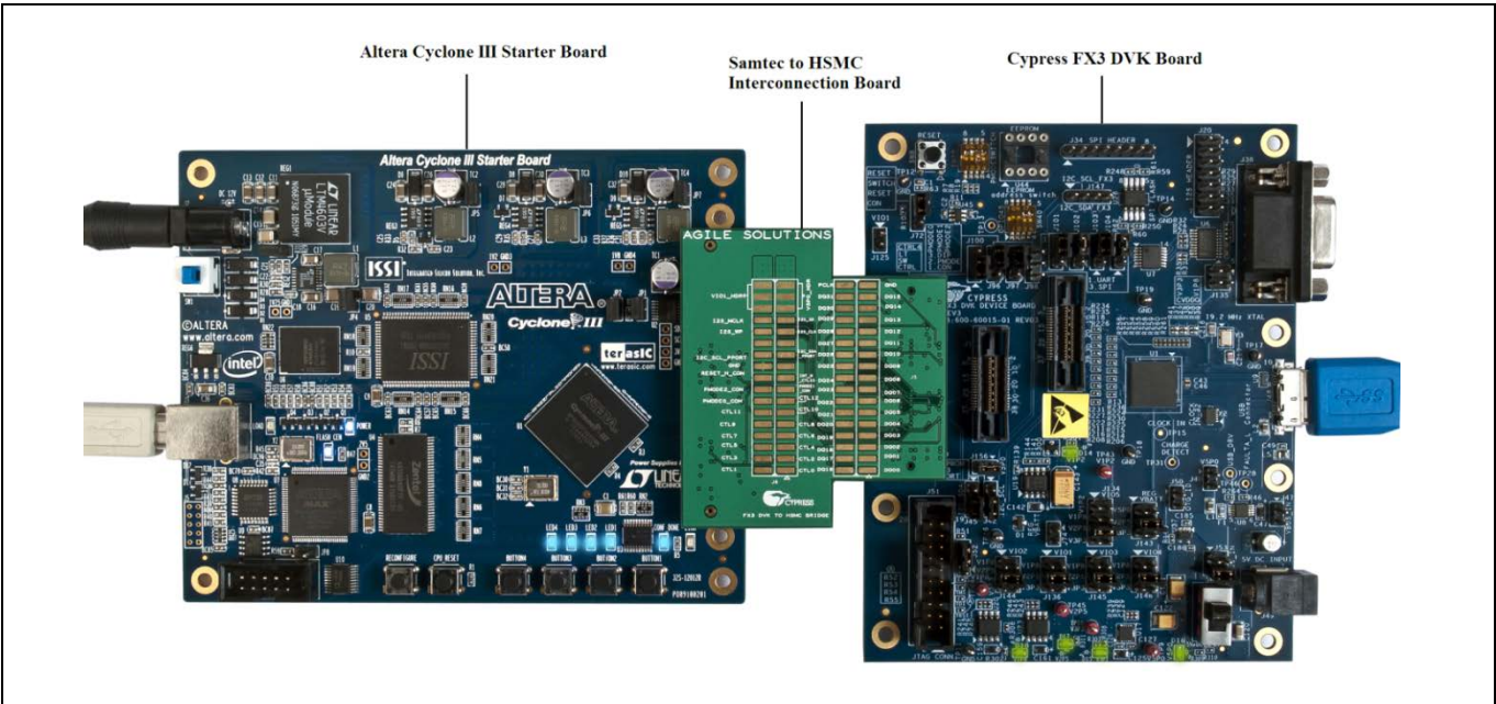
Figure 60 英飞凌 EZ-USB™ FX3 开发套件通过 HSMC 互联电路板与 Altera Cyclone III 电路板相连
