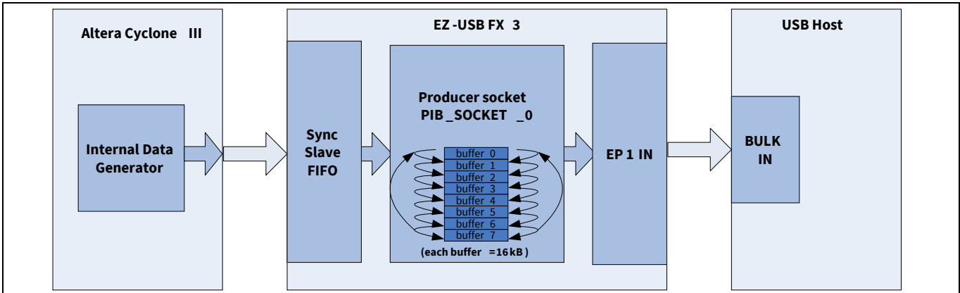
Figure 42 串流 IN 传输设置 – 优化缓冲区数量和大小，以得到更好的性能
