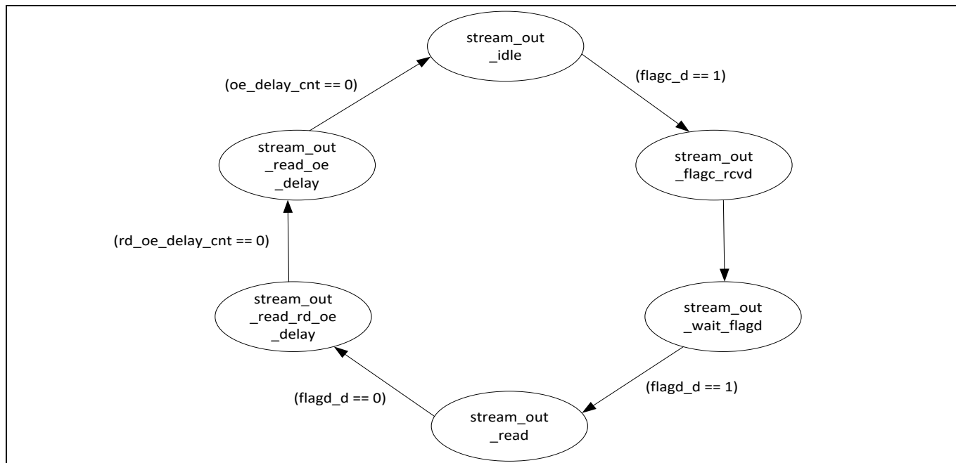
Figure 48 串流 OUT 传输的状态机
