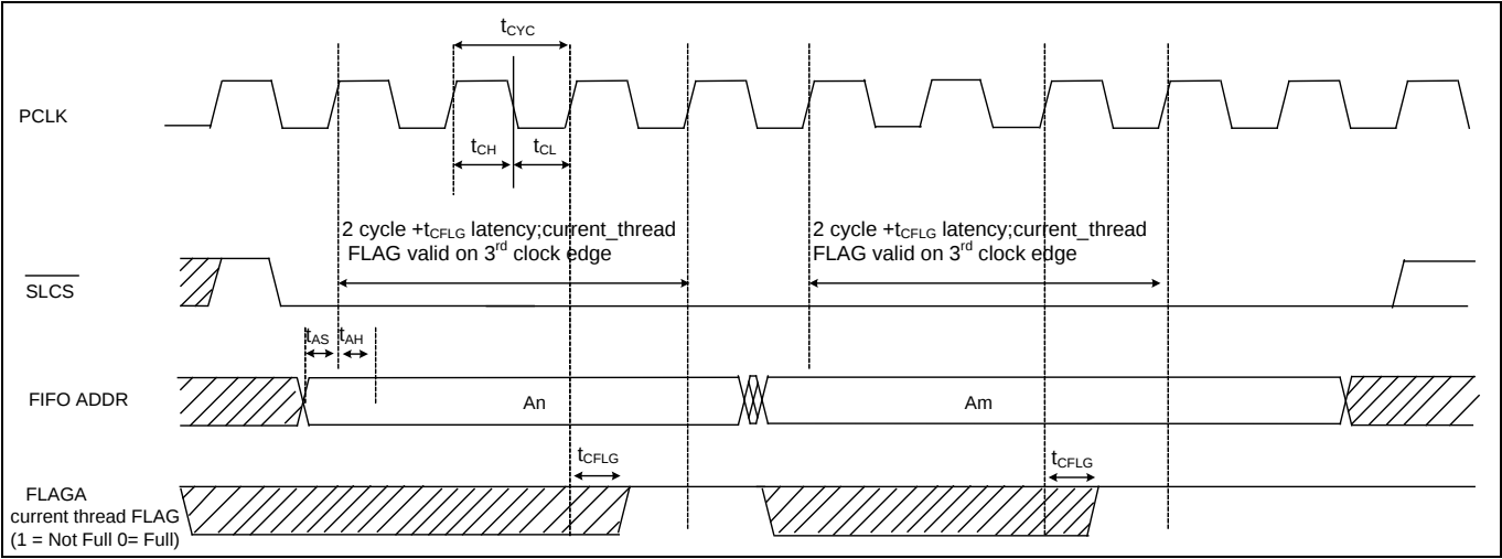
Figure 6 使用当前线程标志情况下开始传输时所发生的额外延迟
