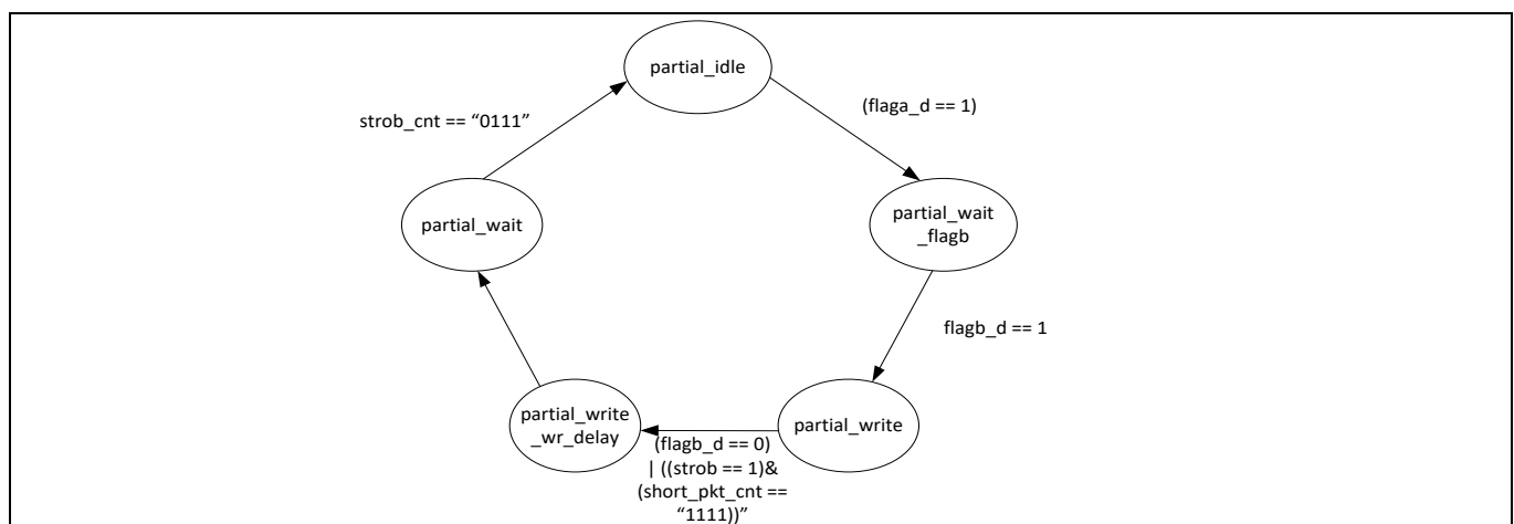
Figure 46 短数据包传输的状态机
