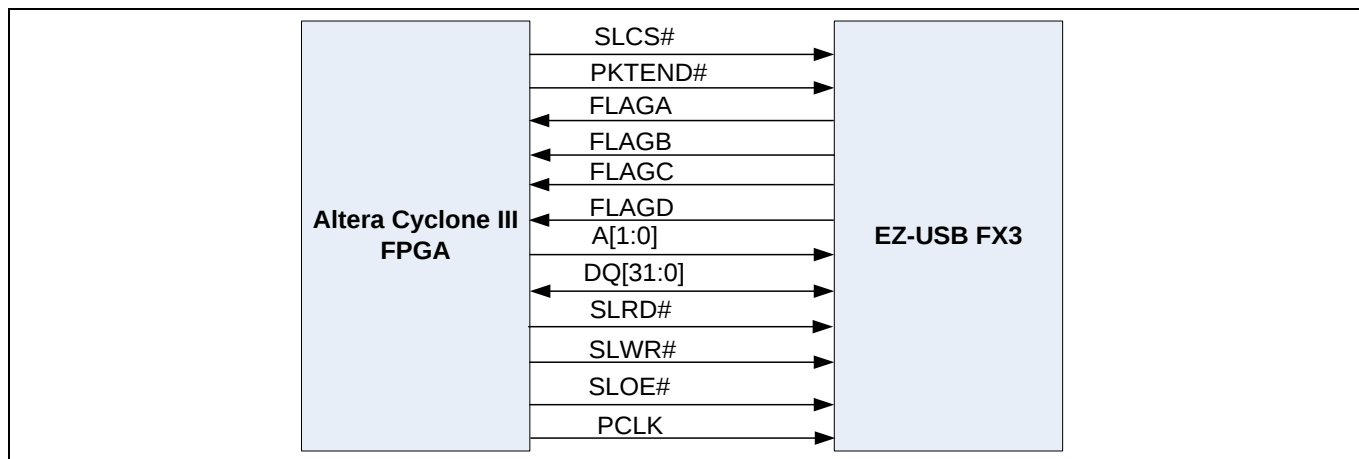
Figure 39 FPGA 和 EZ-USB™ FX3 之间的互连图
