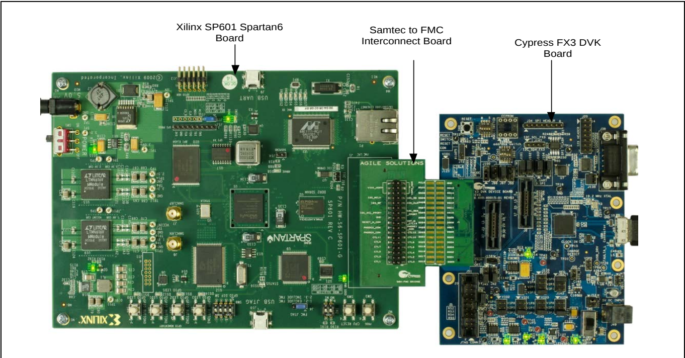
Figure 59 英飞凌 EZ-USB™ FX3 开发套件通过 FMC 互联电路板与 Xilinx SP601 电路板相连
