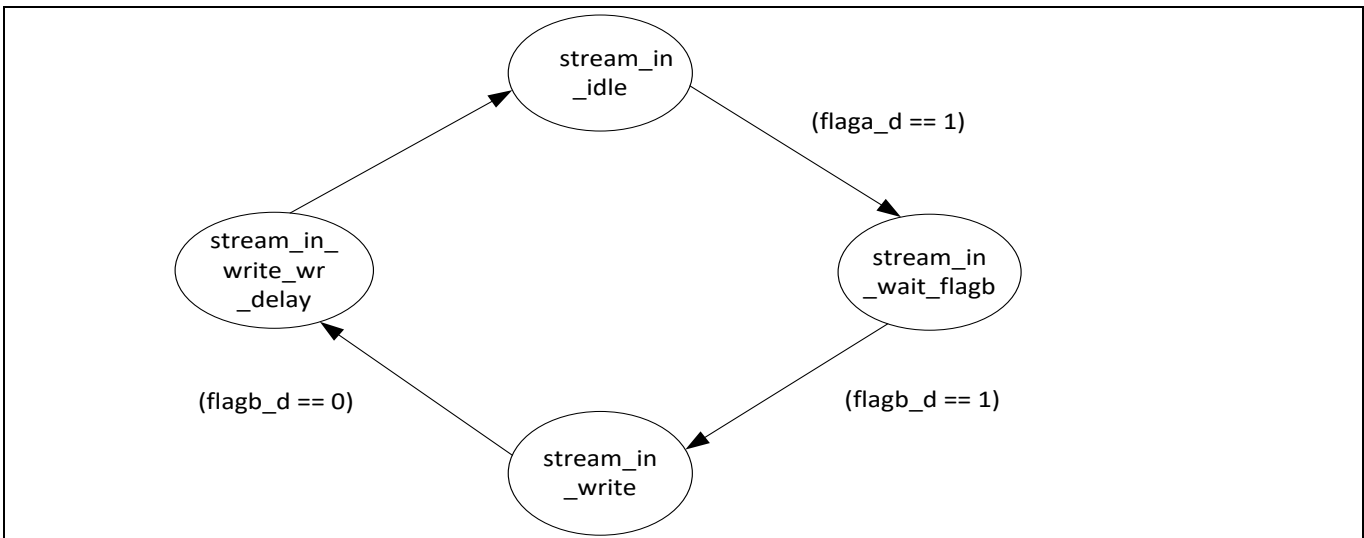
Figure 45 串流 IN 的 FPGA 状态机
