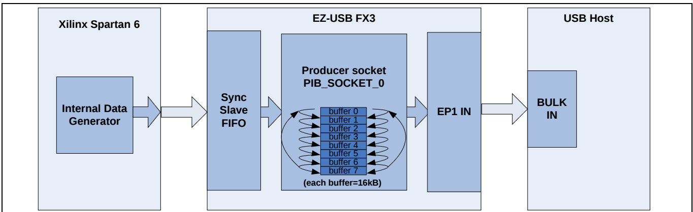
Figure 19 串流 IN 传输设置 – 优化缓冲区数量和大小，以得到更好的性能
