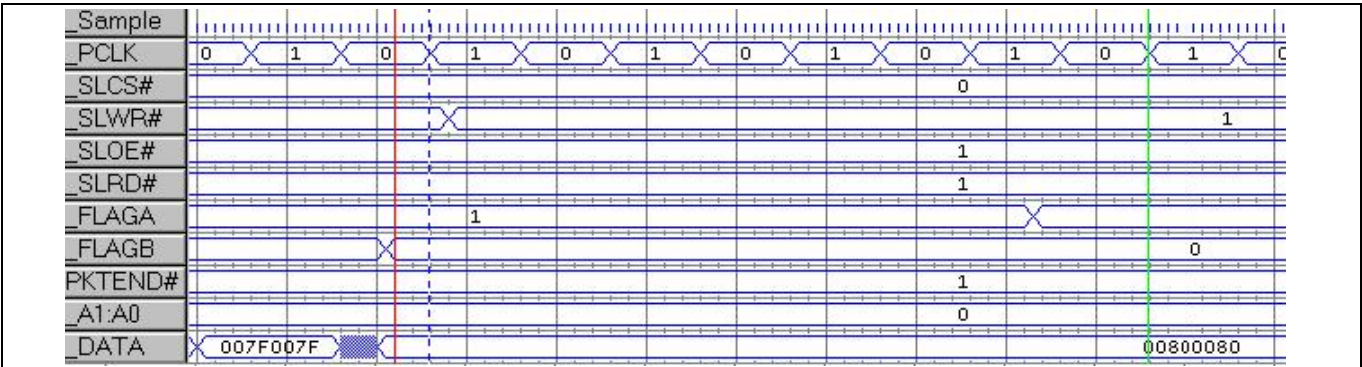
Figure 11 使用 32 位数据总线宽度的突发写入传输 (FLAGA= Current_thread_DMA_RDY, FLAGB= Current_thread_DMA_watermark, watermark = 4)
