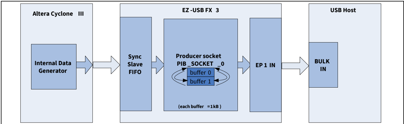
Figure 41 短数据包和 ZLP 传输的设置
