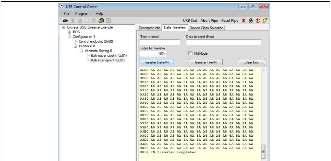
Figure 33 通过使用 Transfer Data-IN 按键启动 BULK IN 传输，以完成回送测试
