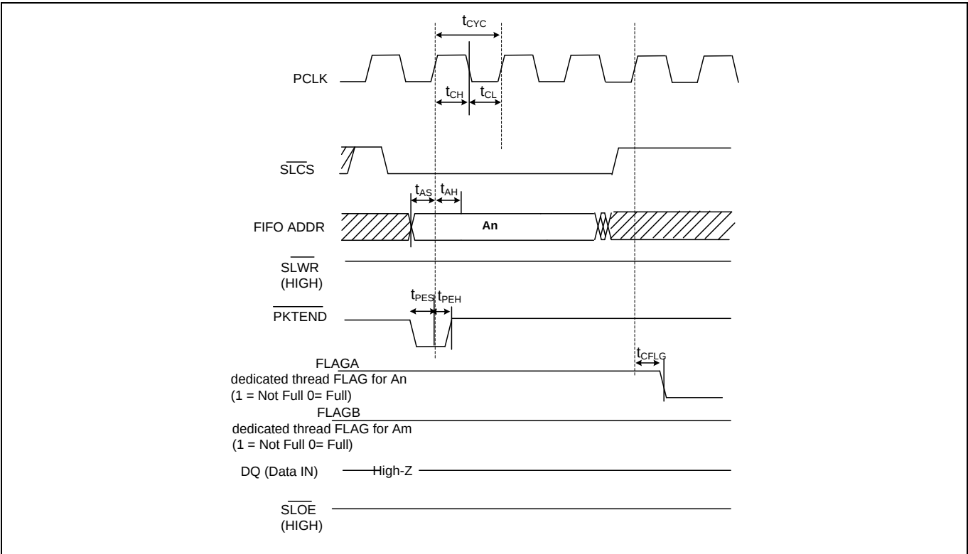
Figure 5 同步 ZLP 写周期时序
