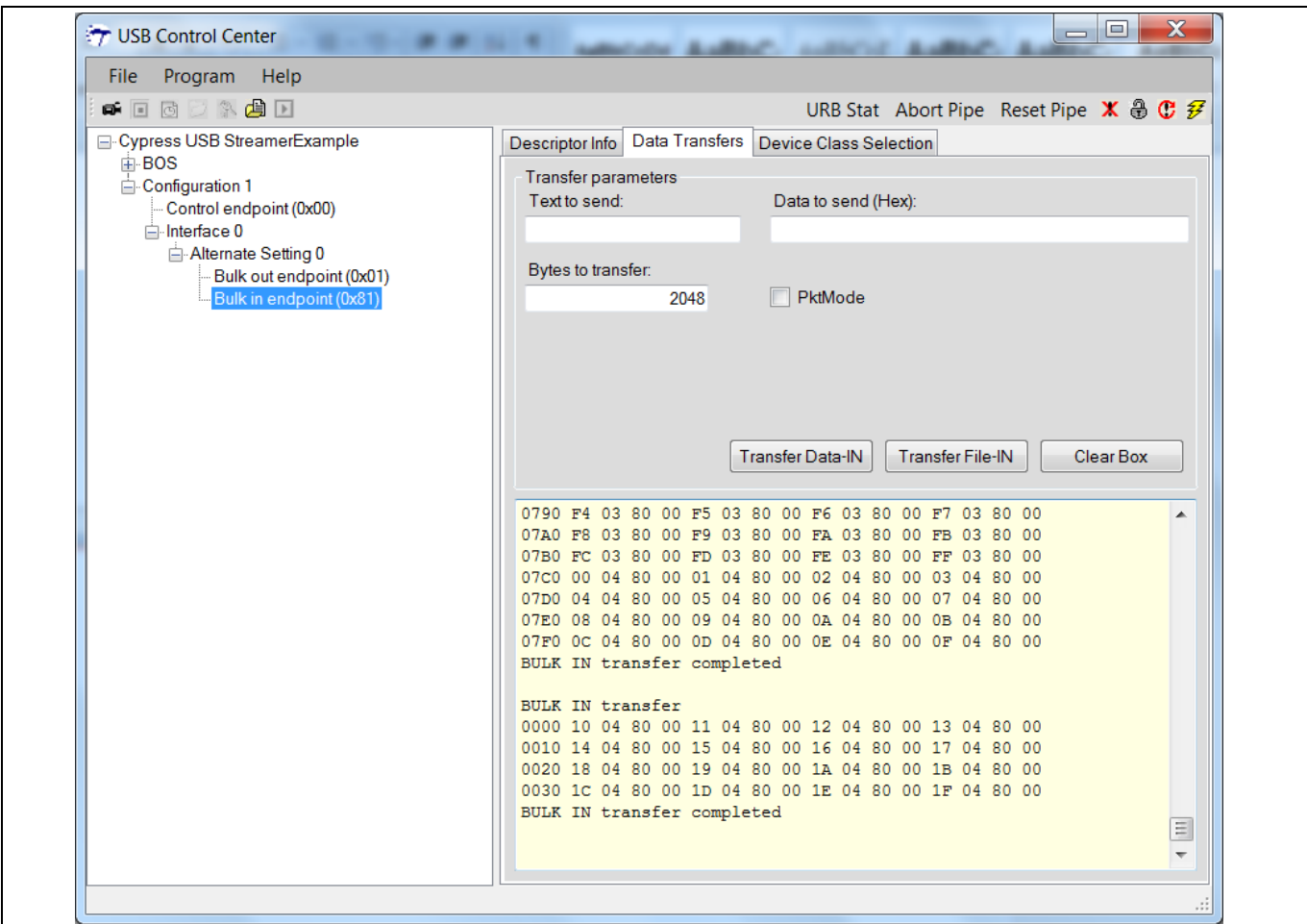
Figure 61 使用 Control Center 读取短数据包
