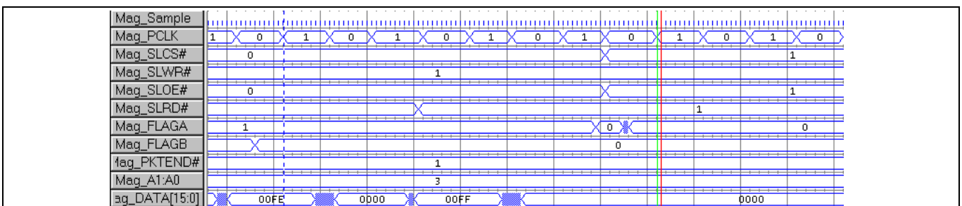
Figure 14 使用 16 位数据总线宽度的突发读取传输 (FLAGA= Current_thread_DMA_RDY, FLAGB= Current_thread_DMA_watermark, watermark = 2)
