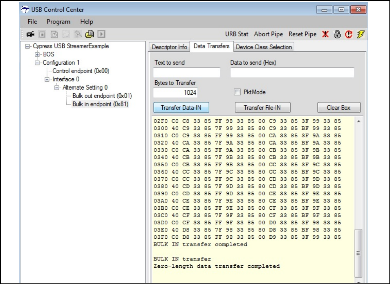
Figure 37 连续执行 Transfer Data-IN 操作分别接收到的完整数据包和零长度数据包
