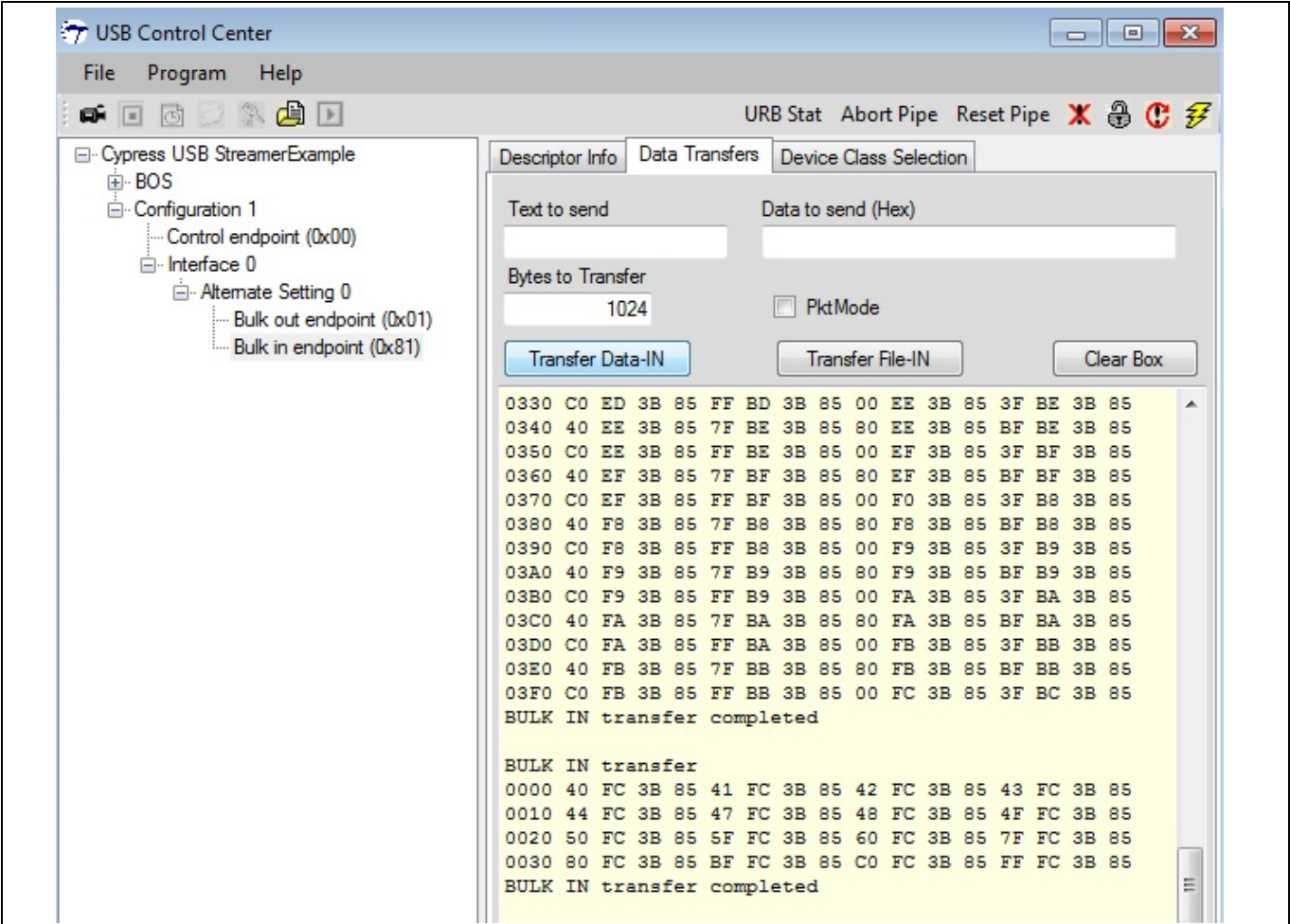
Figure 57 连续执行 Transfer Data-IN 操作分别接收到的完整数据包和短数据包
