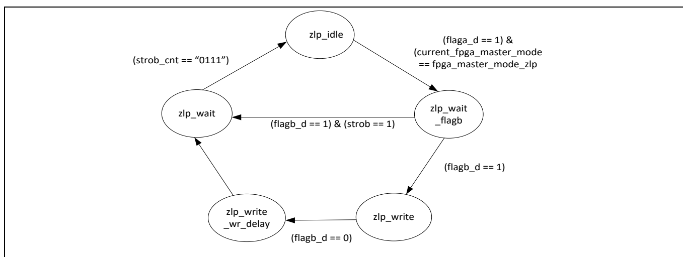
Figure 25 ZLP 传输的状态机
