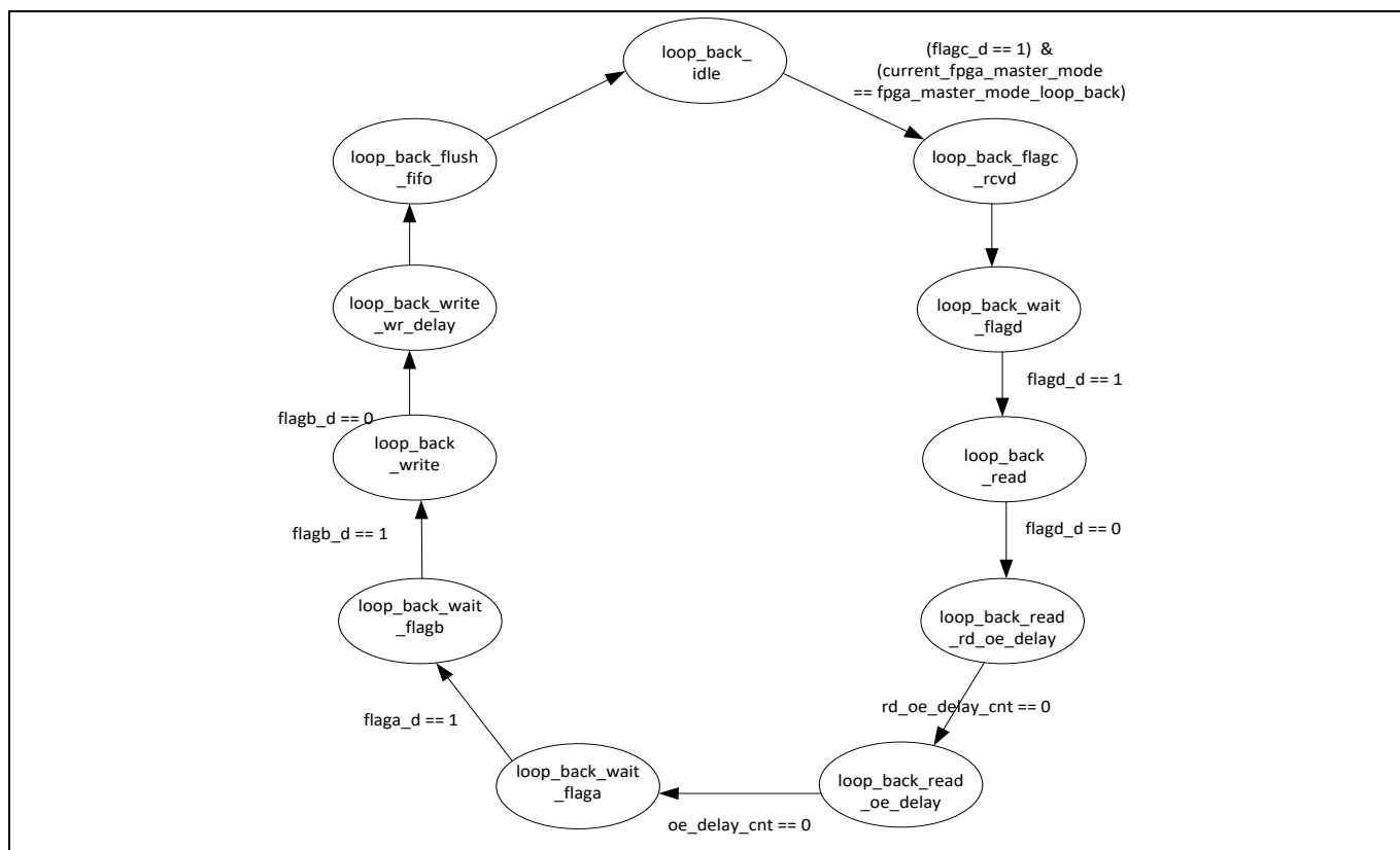
Figure 27 回送传输的状态机
