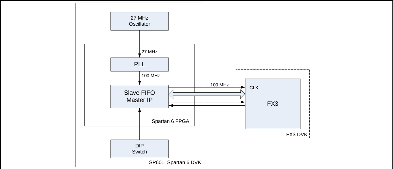
Figure 21 使用 SP601 评估套件实现 Xilinx Spartan 6 (XC6SLX16) FPGA
