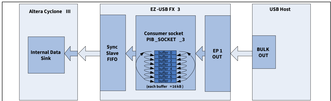
Figure 43 串流 OUT 传输设置 – 优化缓冲区数量和大小，以得到更好的性能
