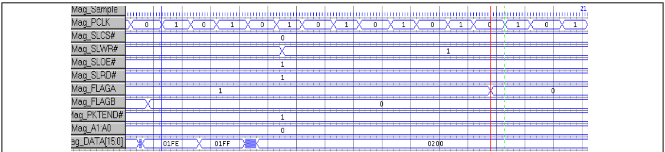
Figure 13 使用 16 位数据总线宽度的突发写入传输 (FLAGA= Current_thread_DMA_RDY, FLAGB= Current_thread_DMA_watermark, watermark = 3)
