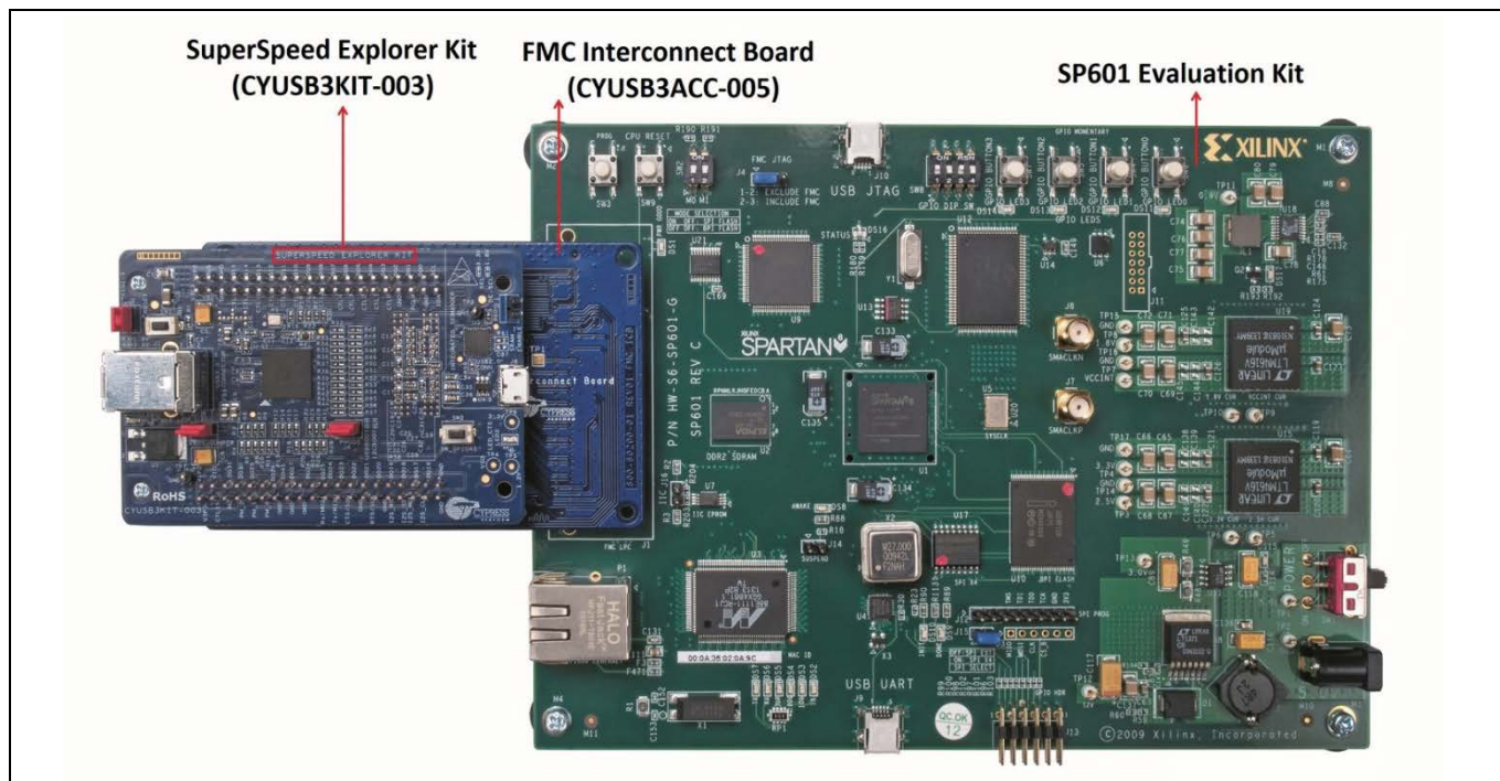
Figure 15 SuperSpeed Explorer 套件通过 FMC 互联电路板与 Xilinx SP601 电路板相连
