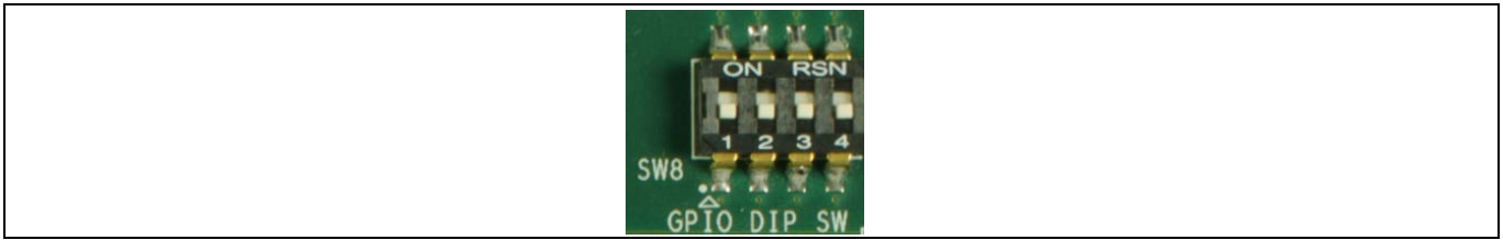
Figure 28 Xilinx SP601 电路板上的 SW8 — 在 FPGA 和 EZ-USB™ FX3 配置前均处于关闭状态
