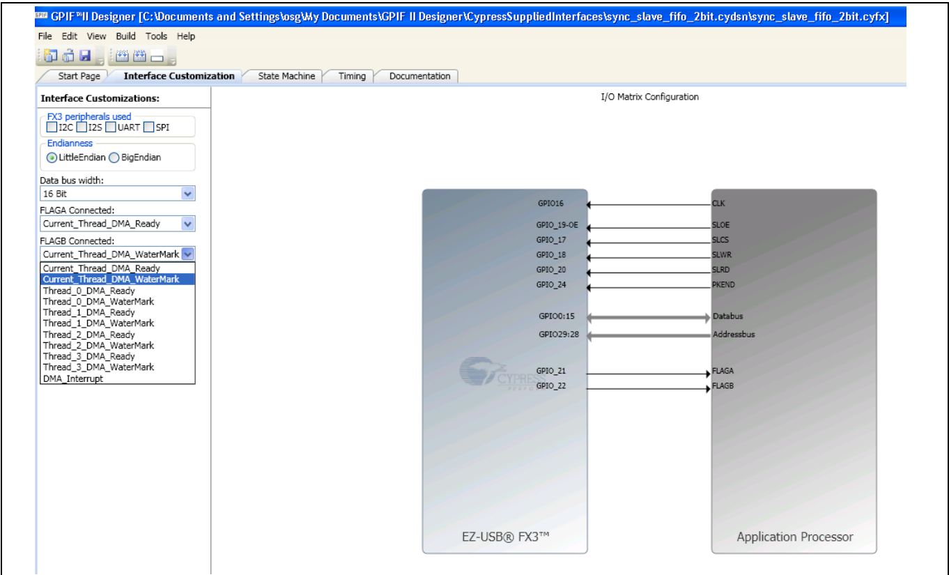
Figure 8 GPIF II Designer 中的标志设置 – Supplied Interfaces 项下的 sync_slave_fifo_2bit
