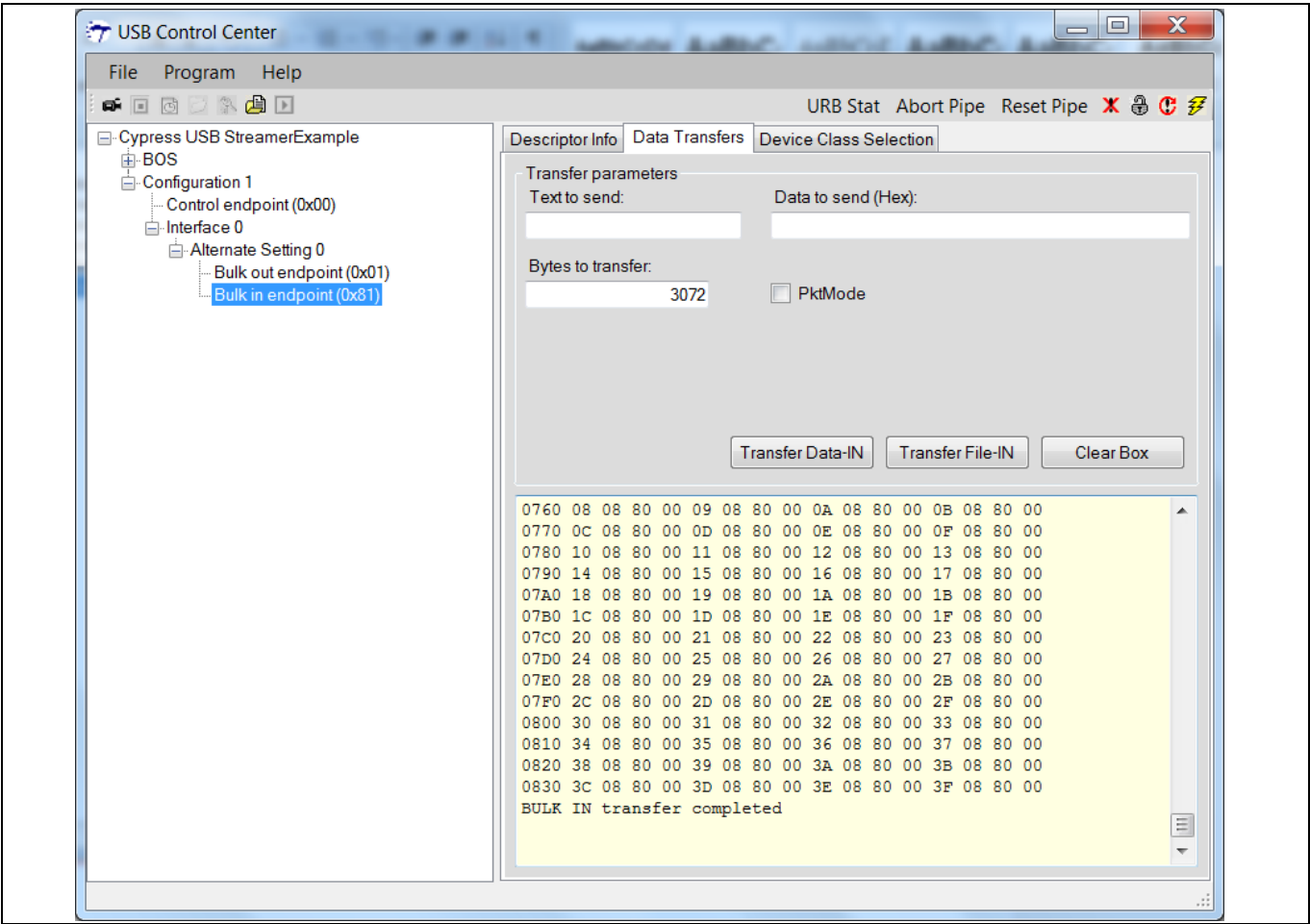
Figure 62 需要的字节多于 DMA 缓冲区大小时的短数据包传输
