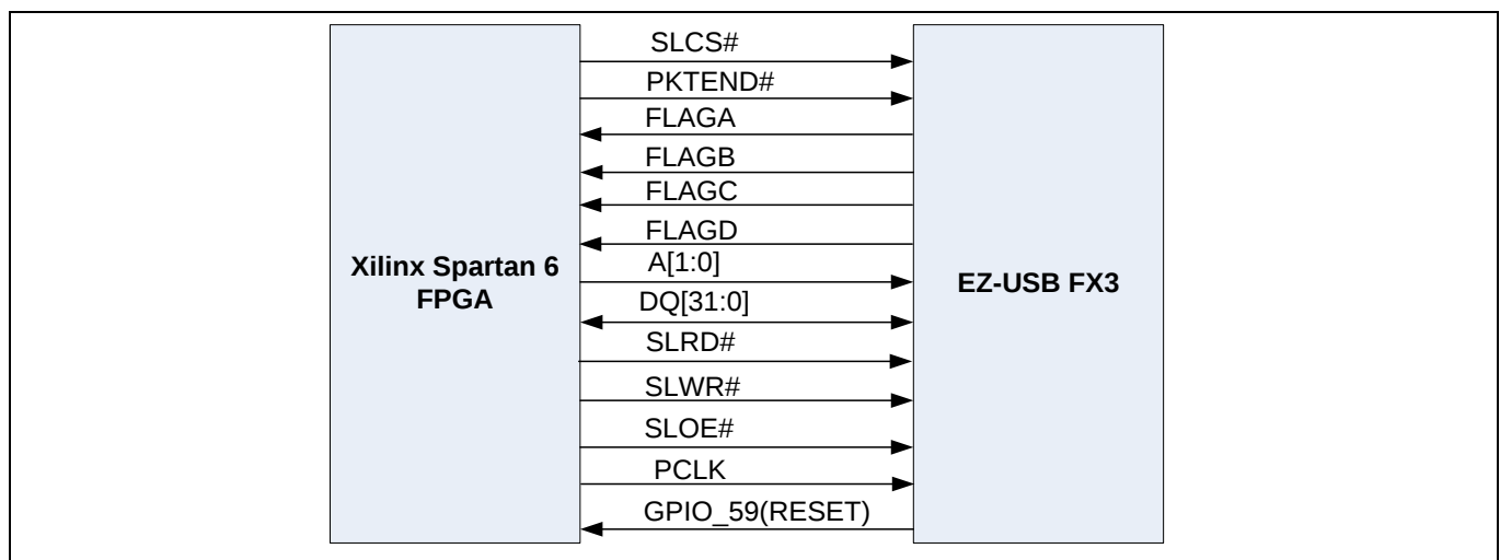
Figure 16 FPGA 和 EZ-USB™ FX3 之间的互连图
