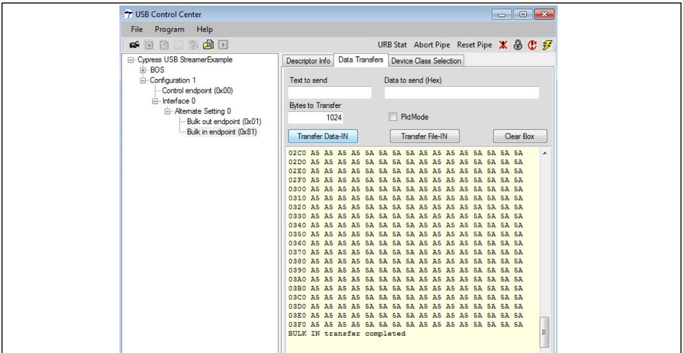
Figure 54 通过使用 Transfer Data-IN 按键启动 BULK IN 传输，以完成回送测试
