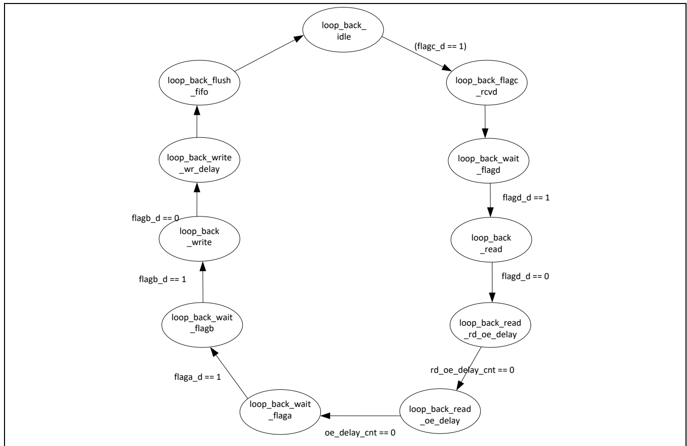
Figure 49 回送传输的状态机
