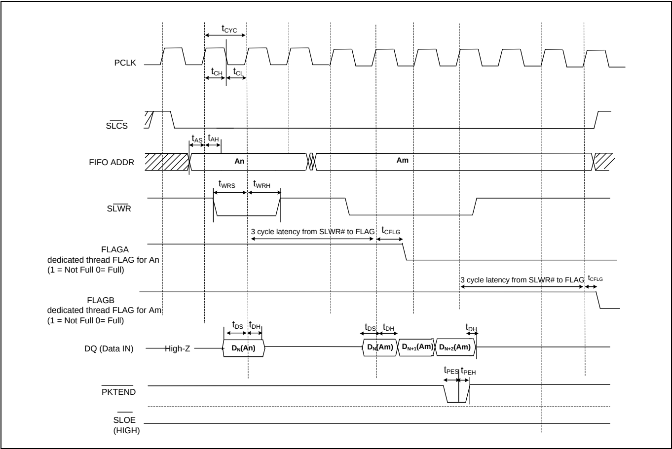
Figure 4 同步从设备 FIFO 写序列
