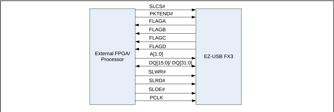
Figure 2 同步从设备 FIFO 接口框图
