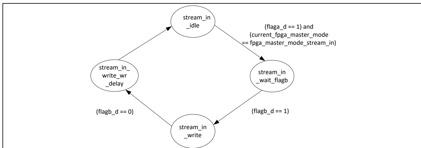
Figure 23 串流 IN 的 FPGA 状态机
