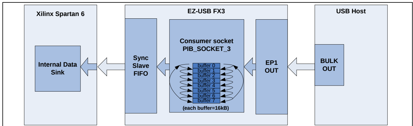
Figure 20 串流 OUT 传输设置 – 优化缓冲区数量和大小，以得到更好的性能
