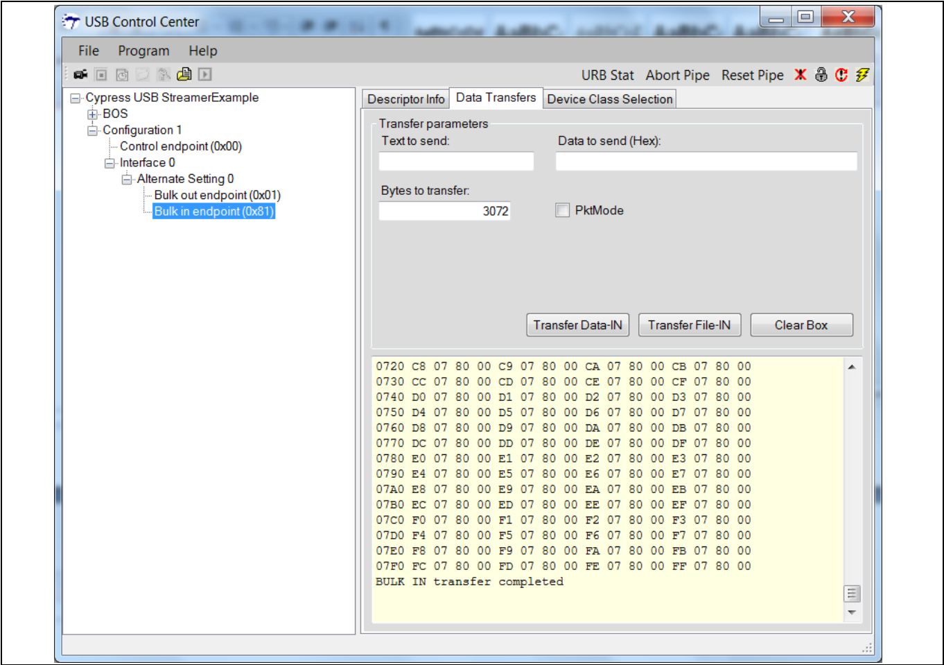
Figure 64 需要的字节多于 DMA 缓冲区大小时的 ZLP 传输
