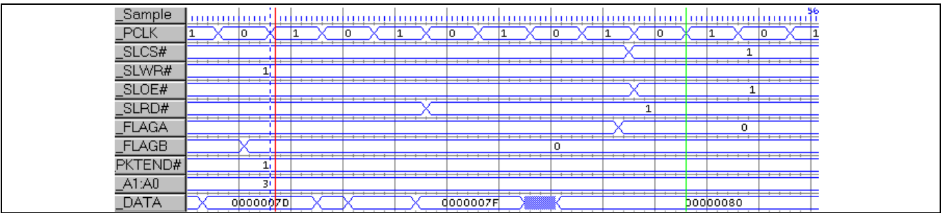
Figure 12 使用 32 位数据总线宽度的突发读取传输 (FLAGA= Current_thread_DMA_RDY, FLAGB= Current_thread_DMA_watermark, watermark = 4)
