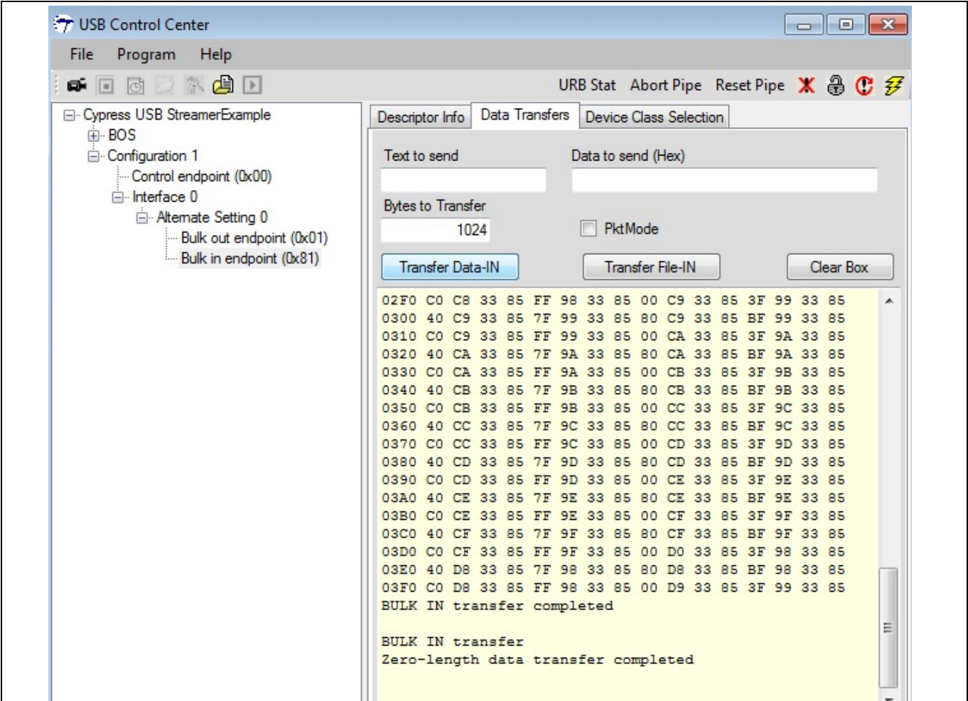
Figure 58 连续执行 Transfer Data-IN 操作分别接收到的完整数据包和零长度数据包
