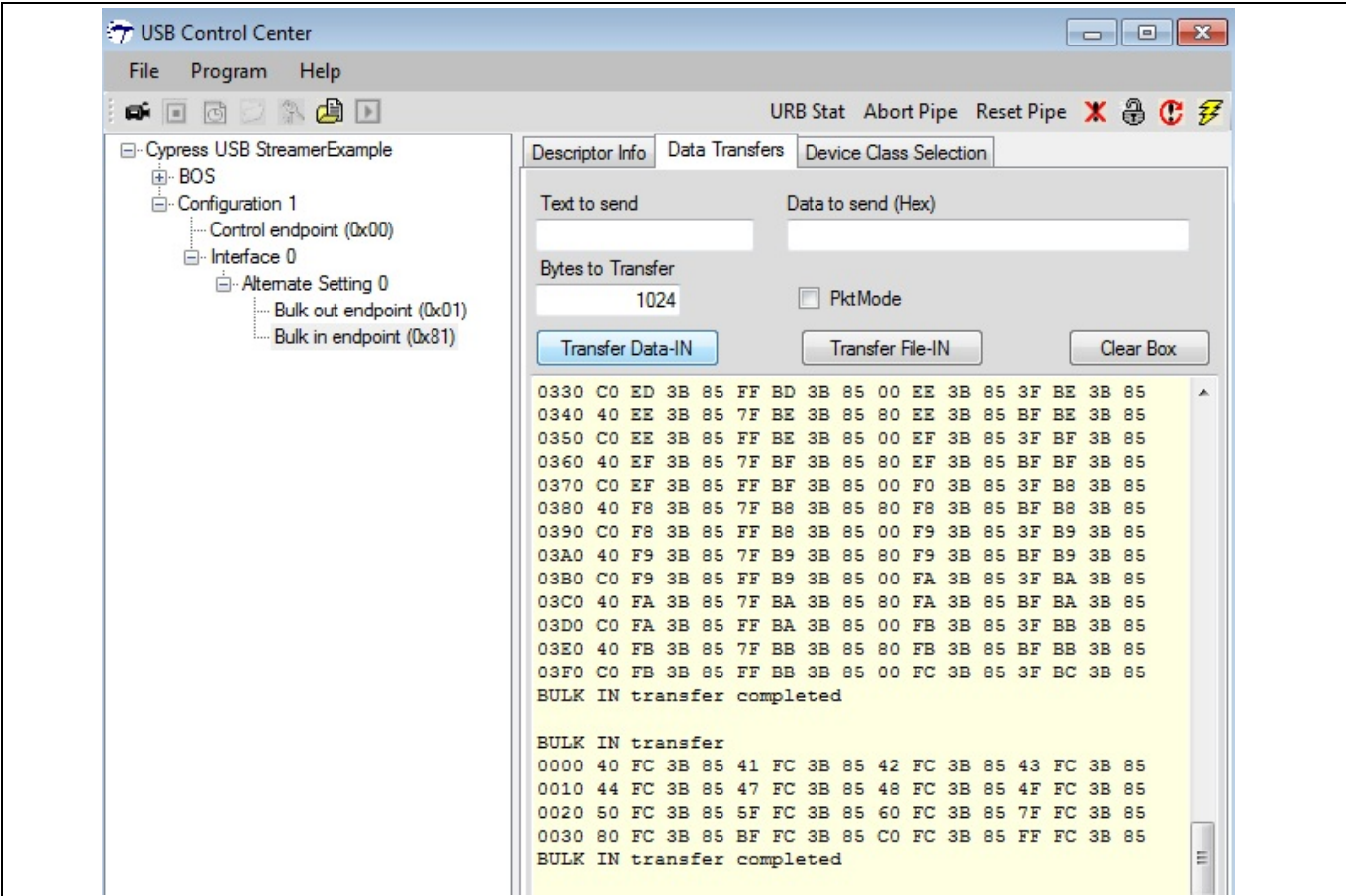
Figure 36 连续执行 Transfer Data-IN 操作分别接收到的完整数据包和短数据包
