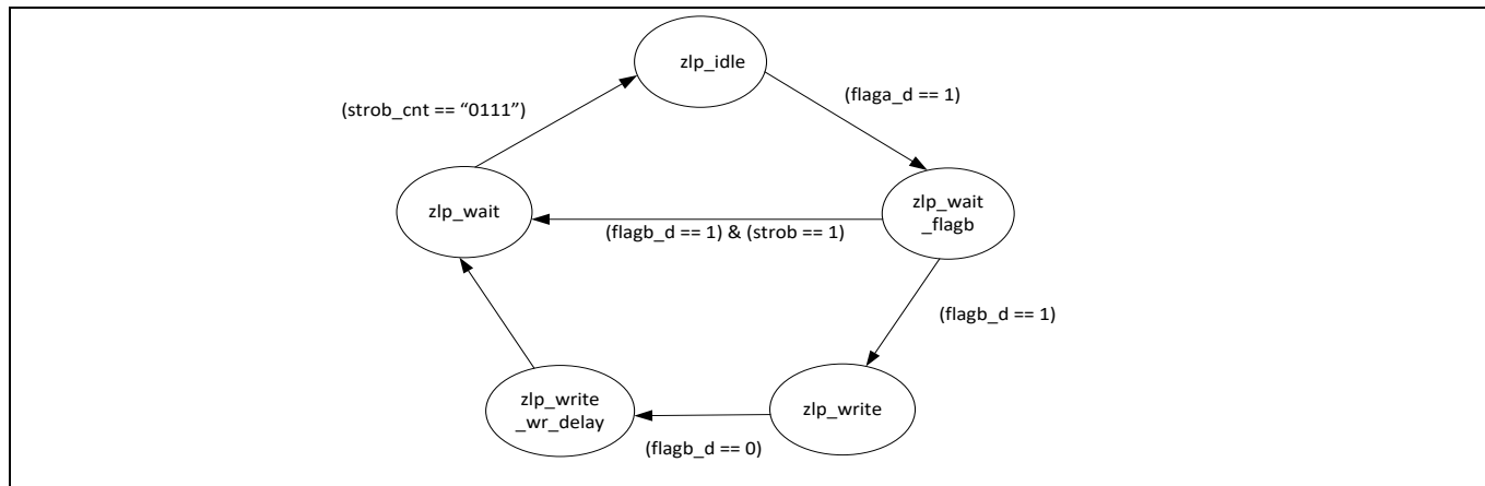
Figure 47 ZLP 传输的状态机
