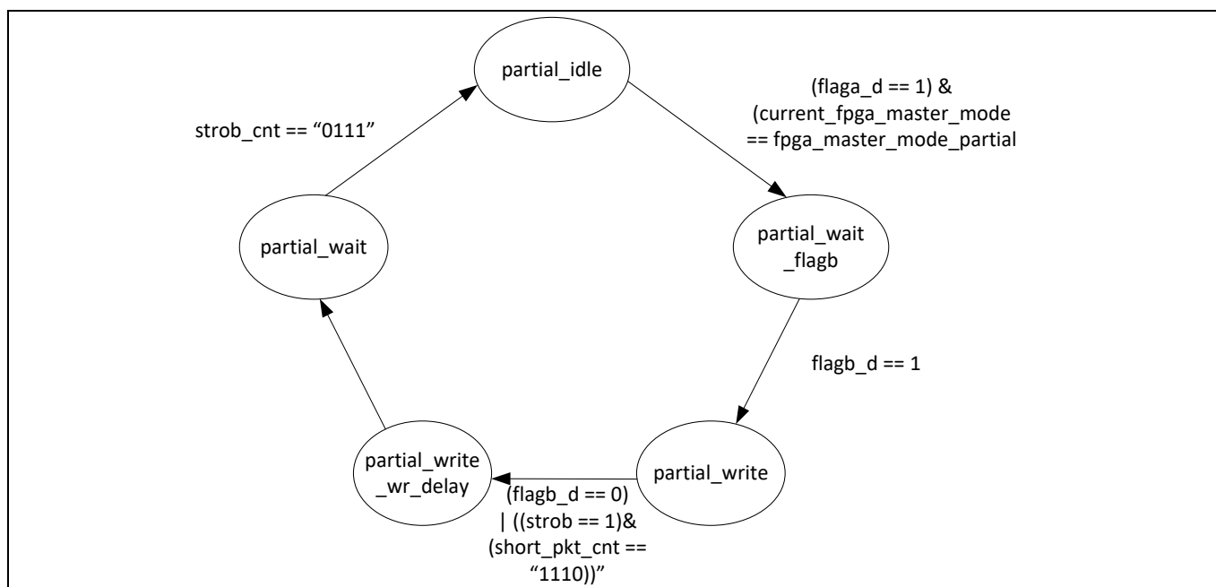
Figure 24 短数据包传输的状态机
