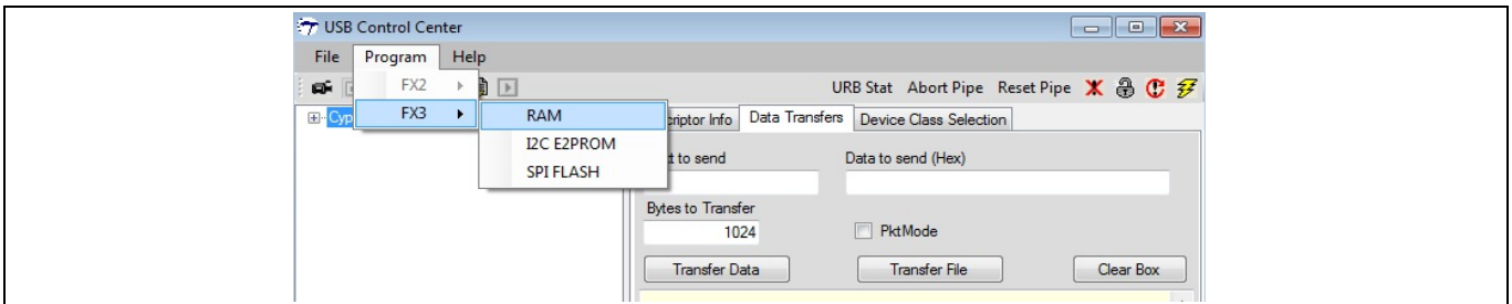
Figure 29 使用 Control Center 编程 EZ-USB™ FX3 固件
