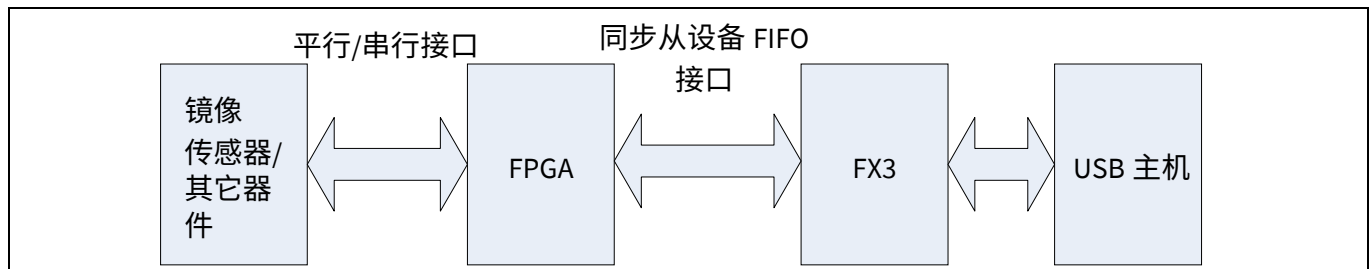
Figure 1 示例应用框图
