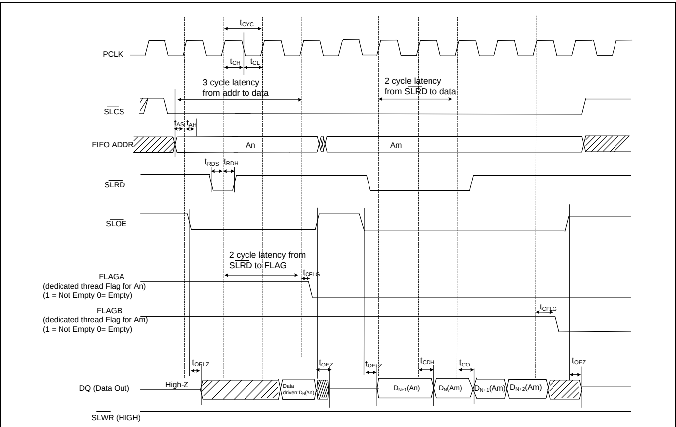
Figure 3 同步从设备 FIFO 读序列
