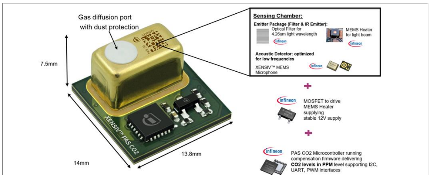
Figure 1 XENSIV™ PAS CO2 gas sensor (PASCO2V0)
