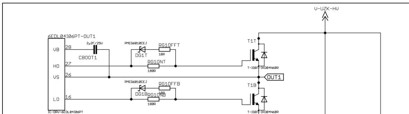
图4 6EDL04I06PT 的栅极驱动器输出。图中仅显示单相输出作为示例
