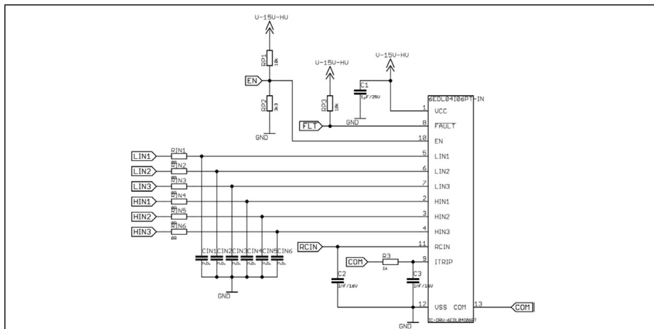
图8 栅极驱动器输入
