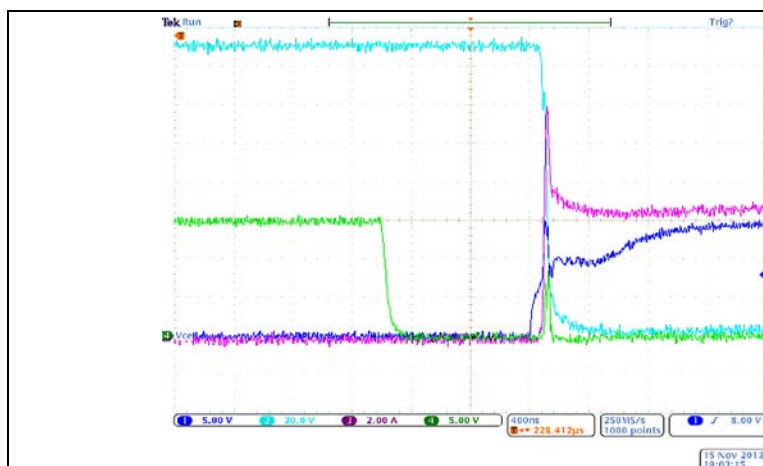
图6 关闭上方 IGBT (1µs 死区时间)
