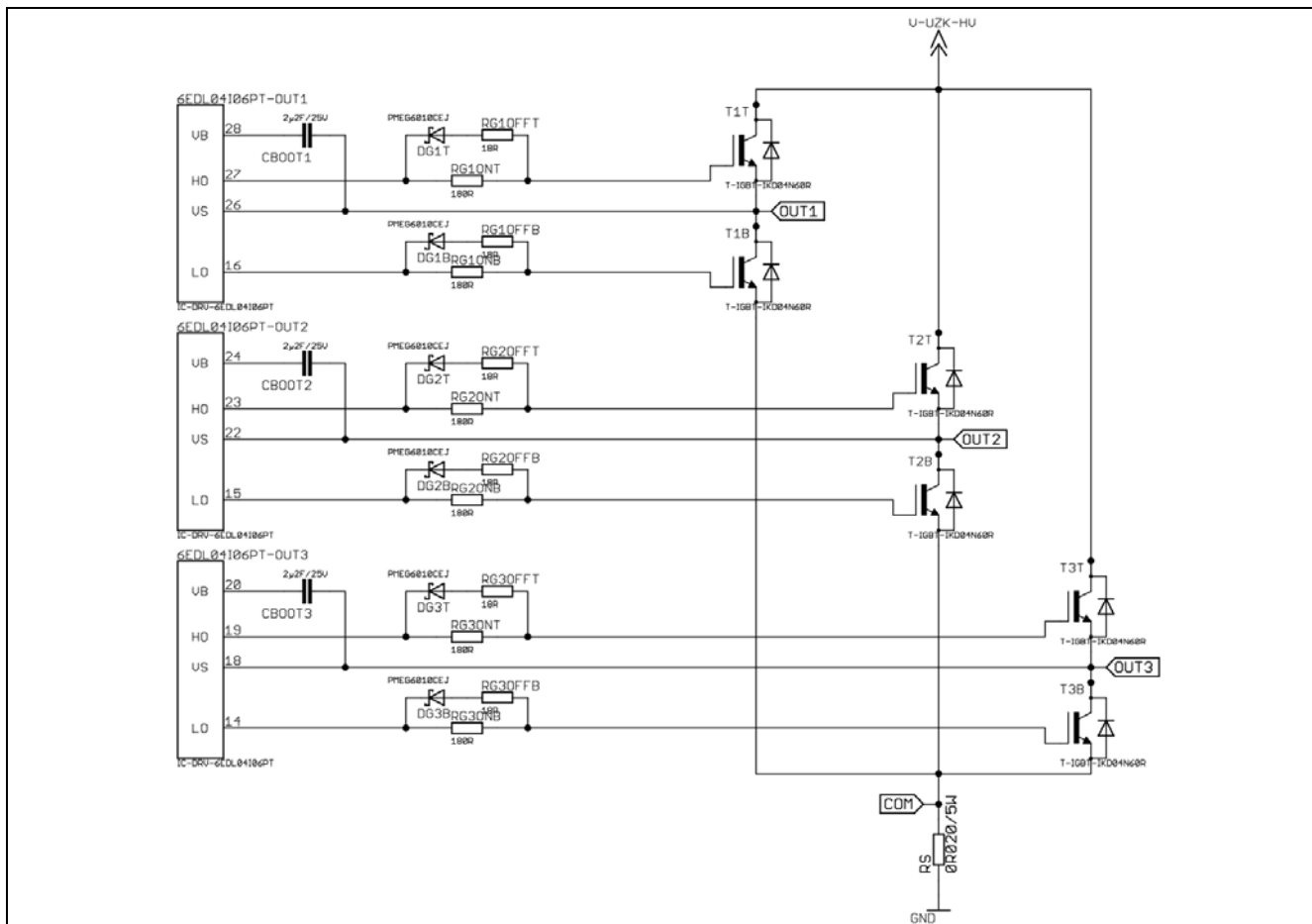
图12 英飞凌驱动器 6EDL04106PT 输出
