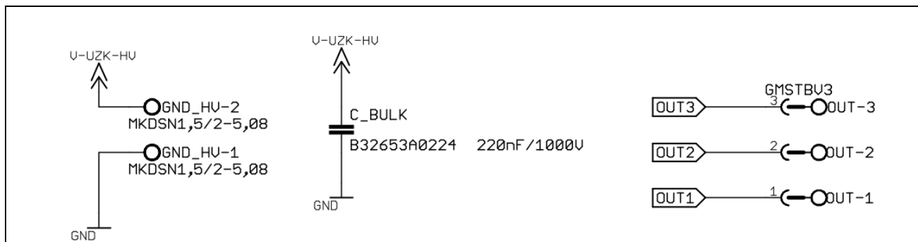
图9 高压电源输入、直流链和负载连接器
