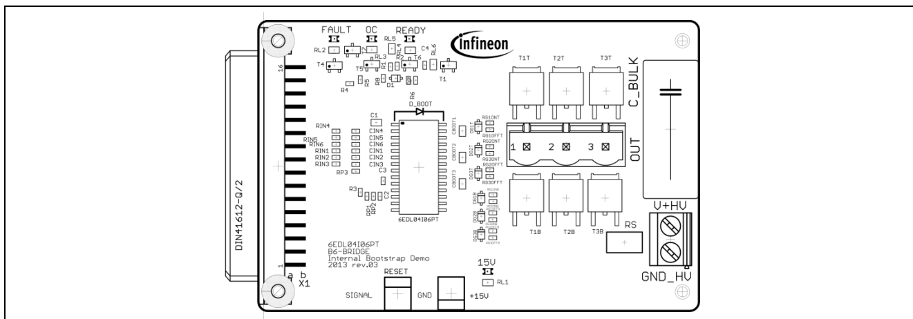
图16 EVAL-6EDL04I06PT 正面贴放视图
