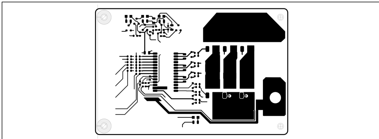
图14 EVAL-6EDL04I06PT 正面布局
