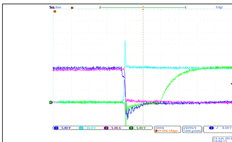
图7 开启上方 IGBT (1µs 死区时间)
