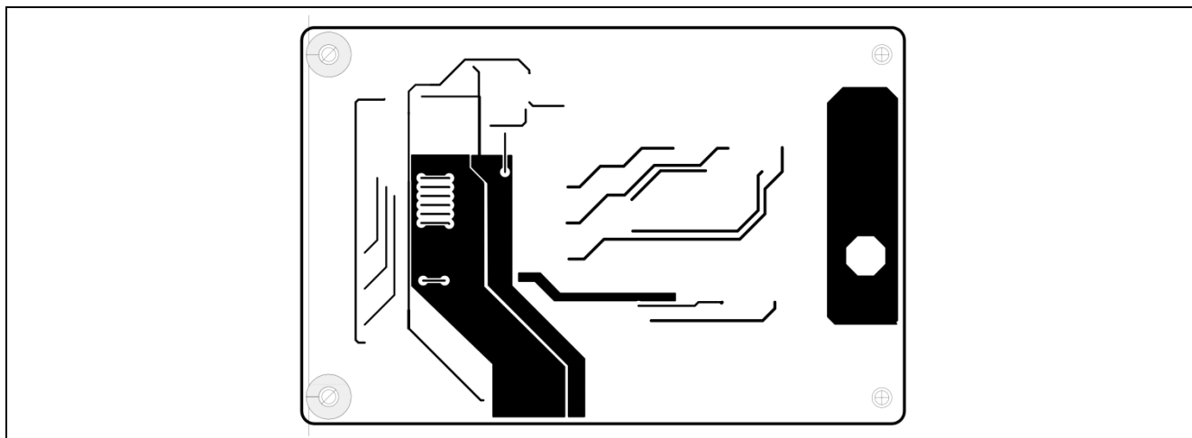
图15 EVAL-6EDL04I06PT 背面布局
