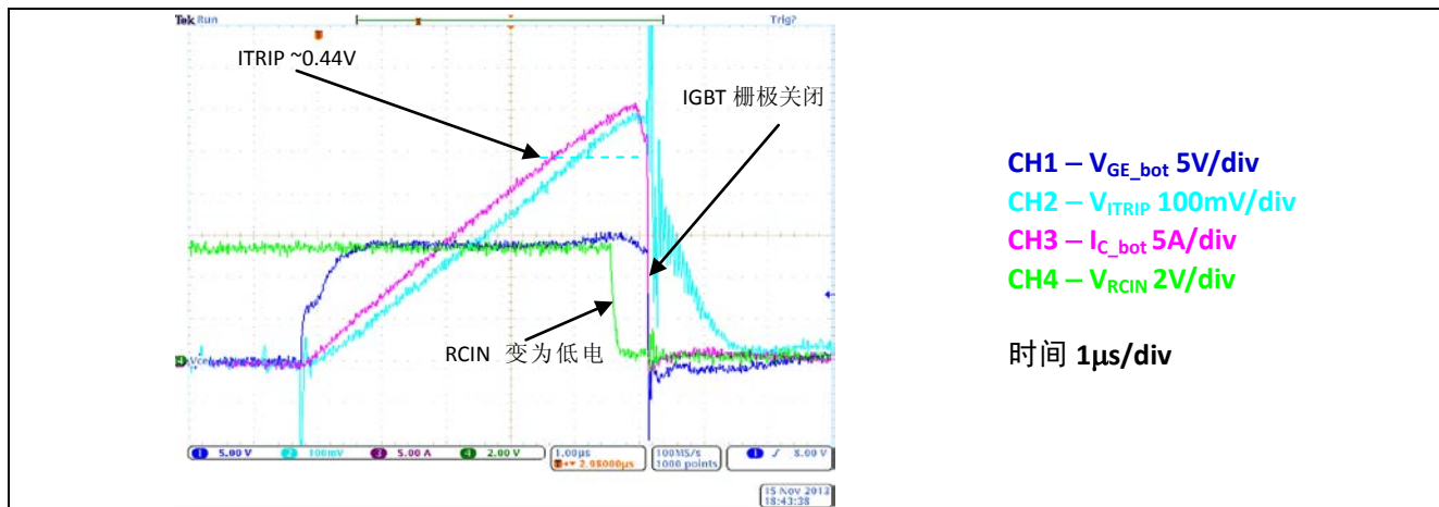
图3 模拟短路期间的过流检测信号
