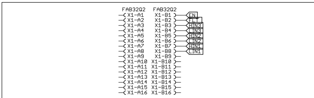
图11 连接器 X1
