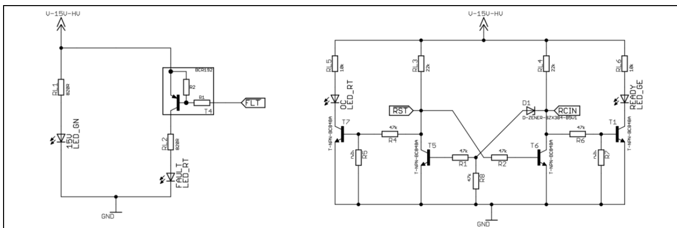
图13 LED、FAULT 和 READY 逻辑
