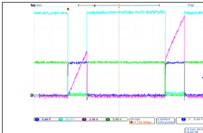
图5 开关序列 (1µs 死区时间)
