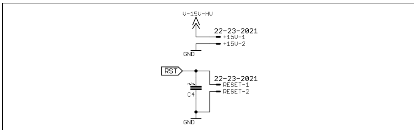
图10 低压电源和复位输入
