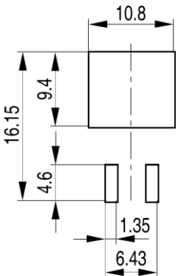
PG-TO263-3-2-FP V03
