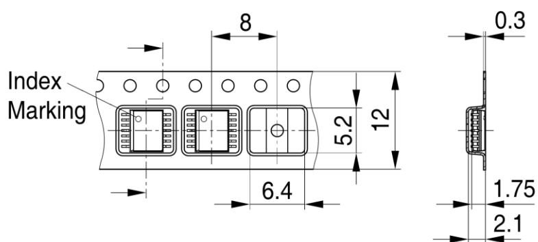
PG-SSOP-14-1,-2,-3,-5-TP V01
