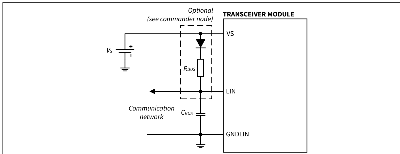
Figure 56 Parameter test circuit
