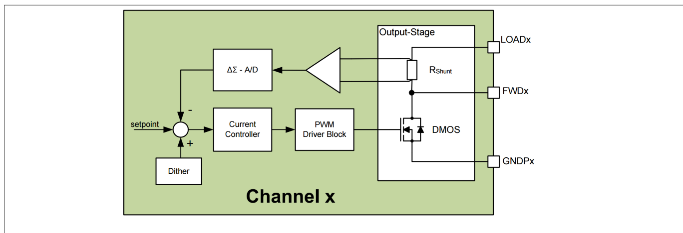
图 5 通道框图
