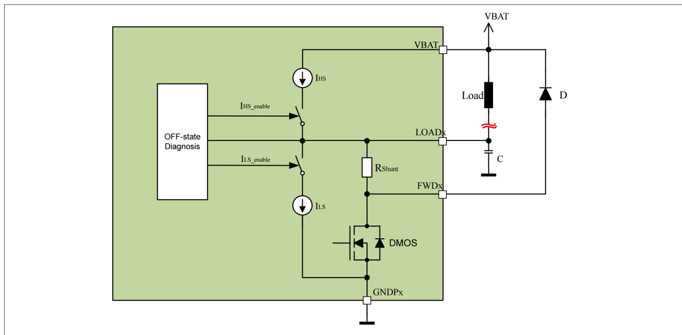
图 18 负载开路
