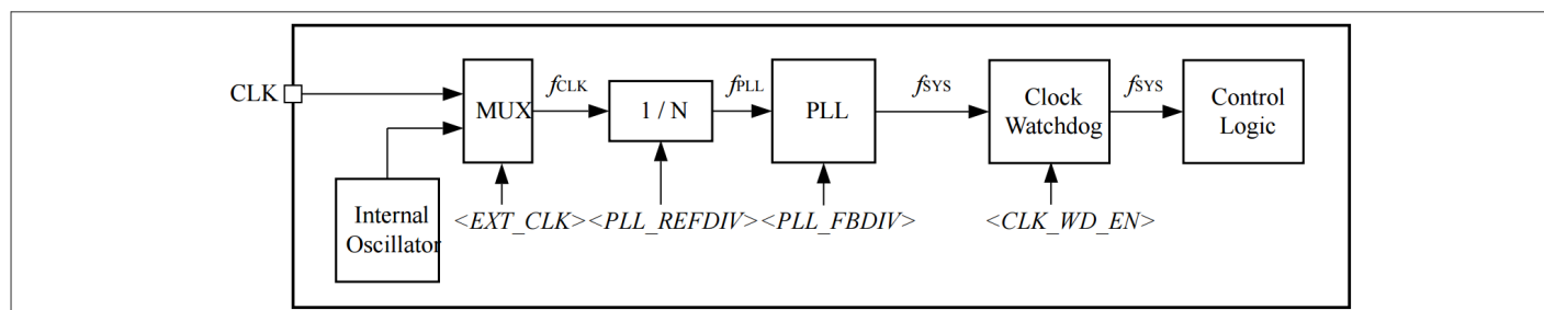
图 3 时钟生成
