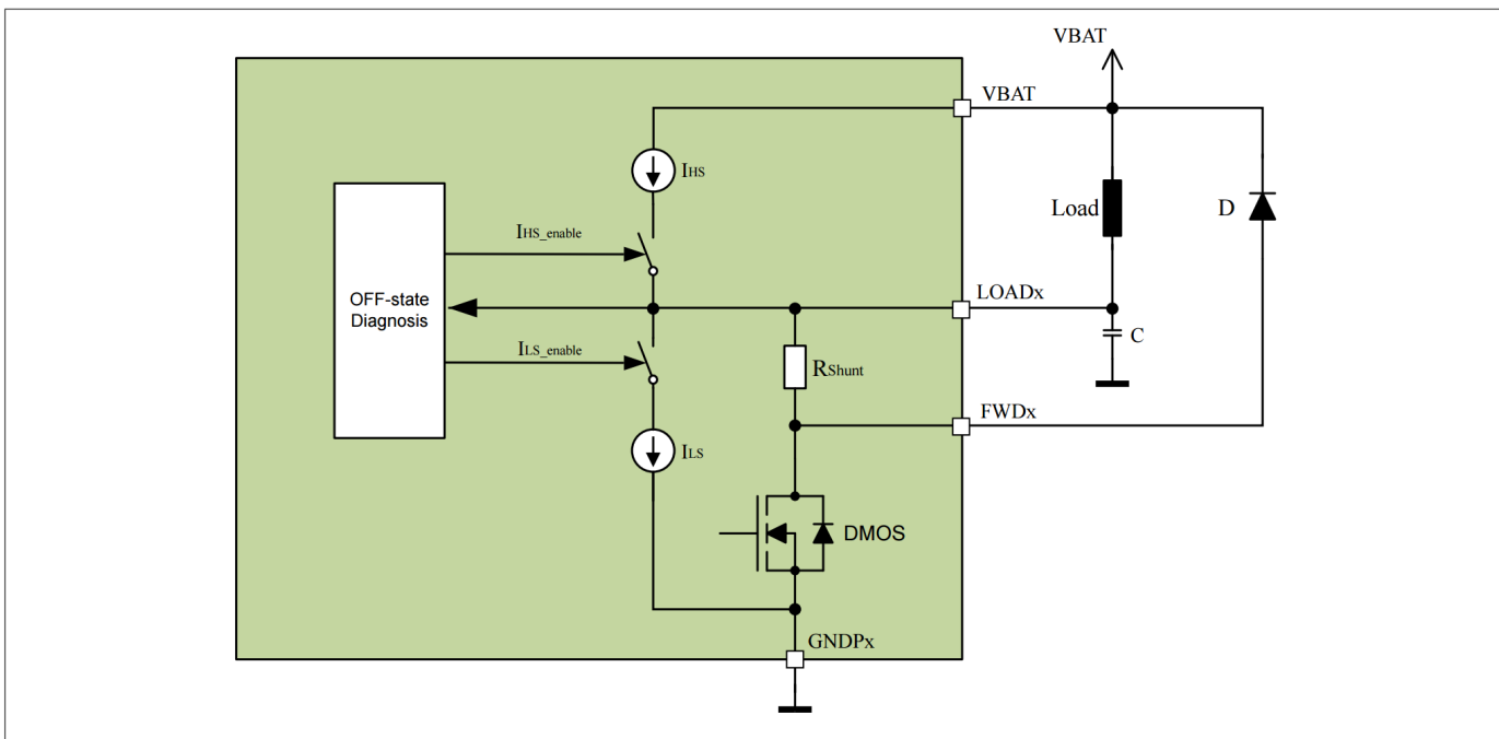
图 14 OFF 状态诊断电路
