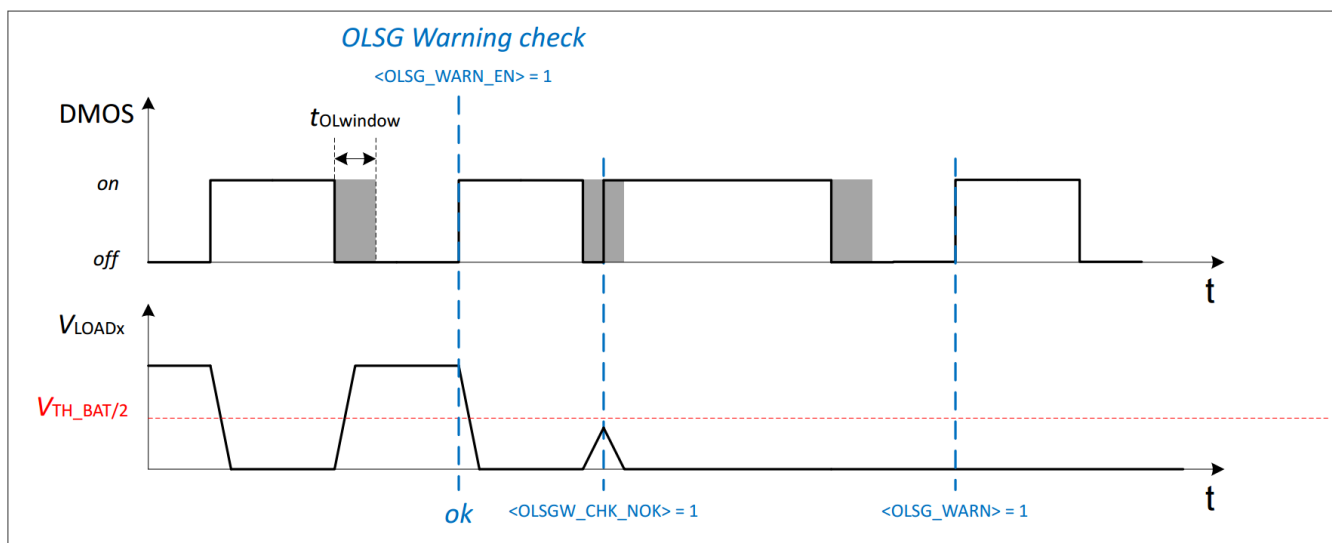
图 17 OLSG-Warning 和 OLSG 警告检查概述
