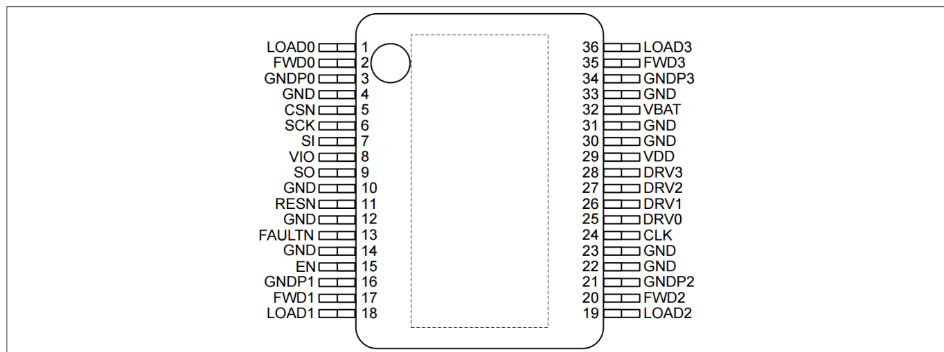
图 2 引脚分配
