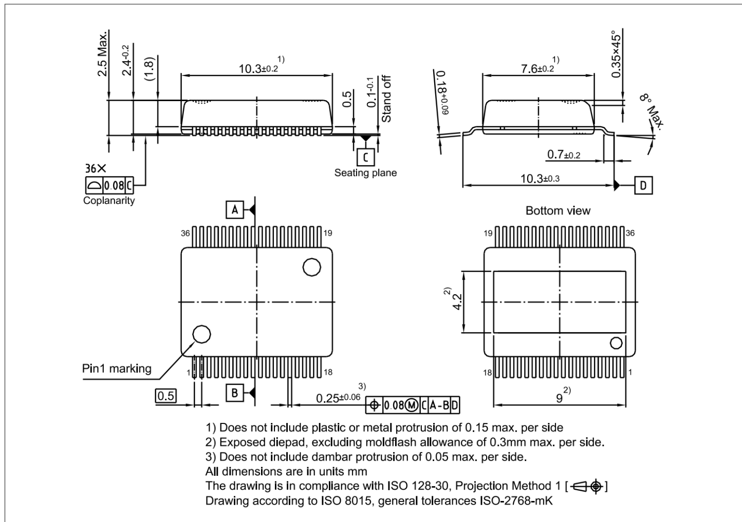
图 27 封装外形
