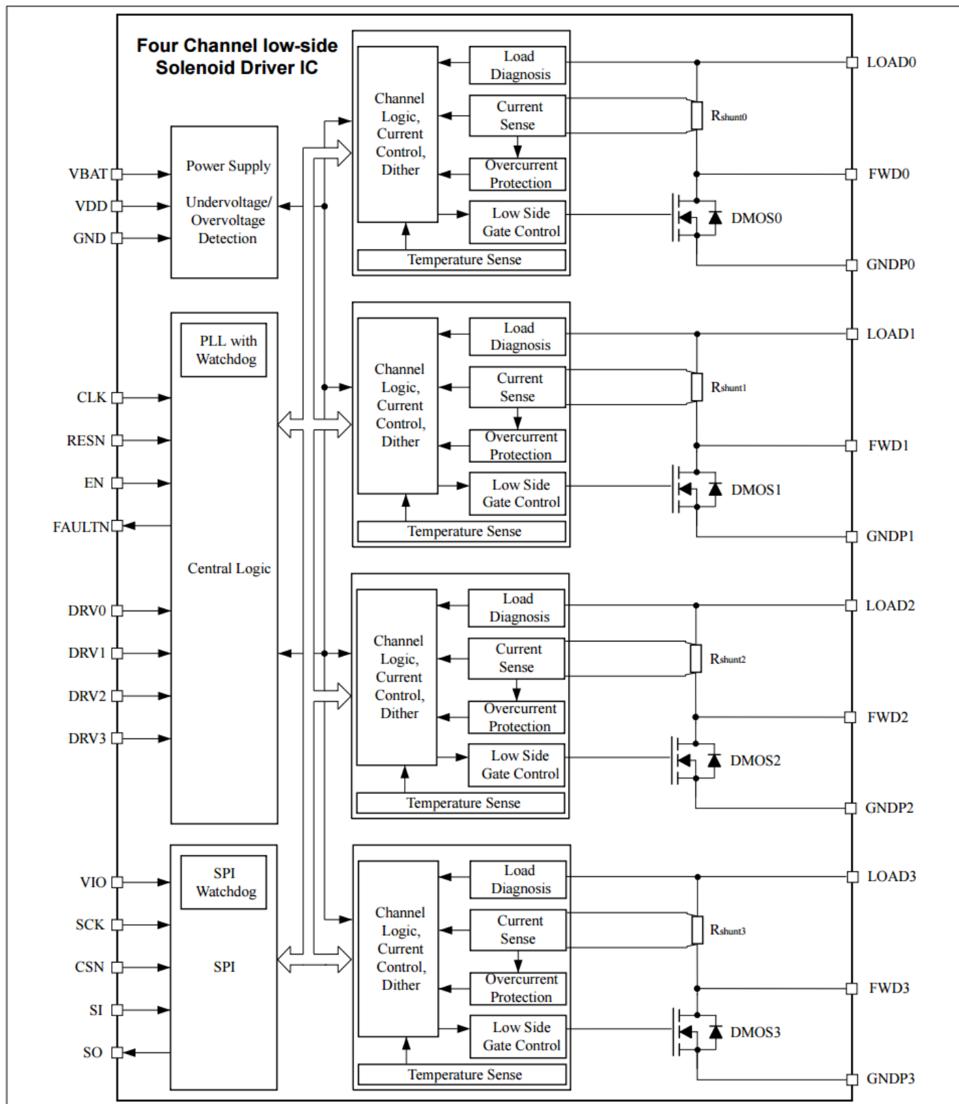
图 1 框图
