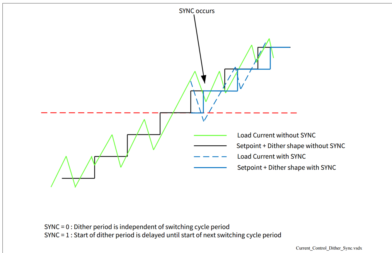
图 13 颤振同步
