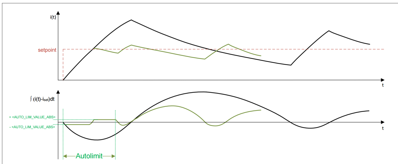
图 9 自动限制值功能
