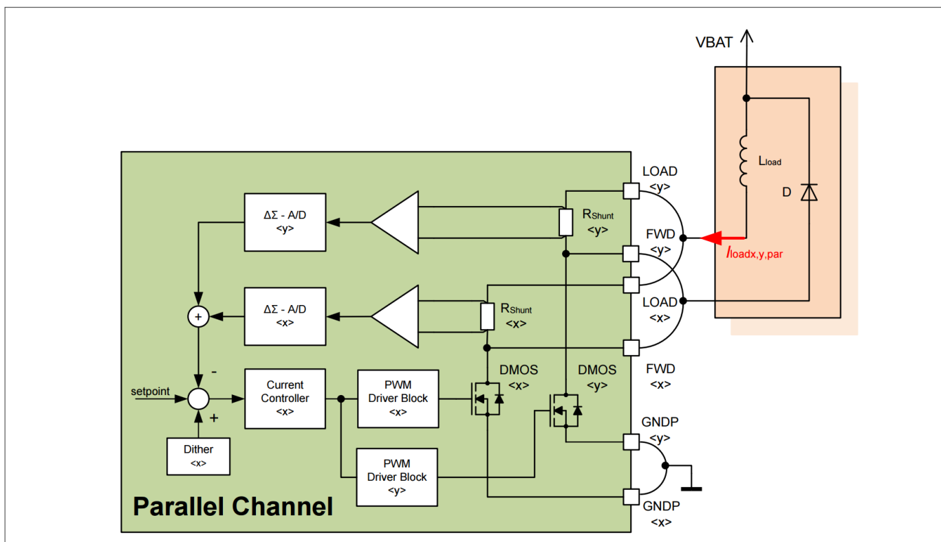
图 6 并联通道配置
