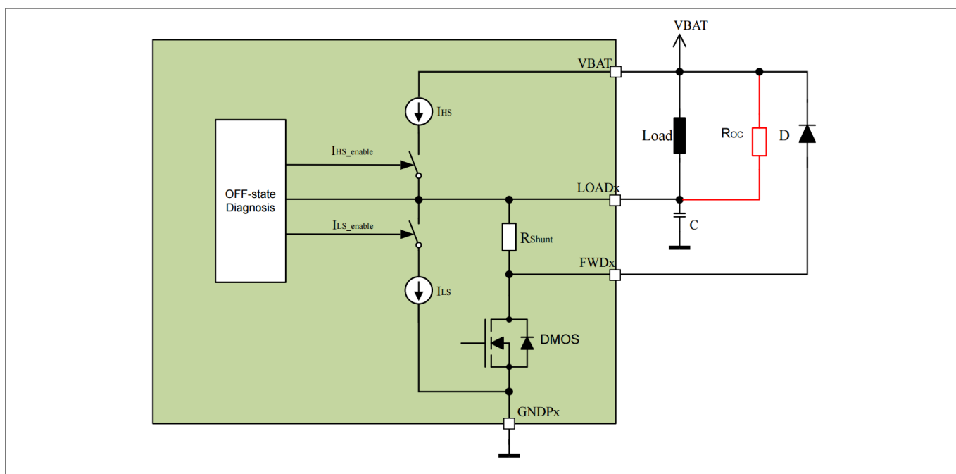
图 20 过流
