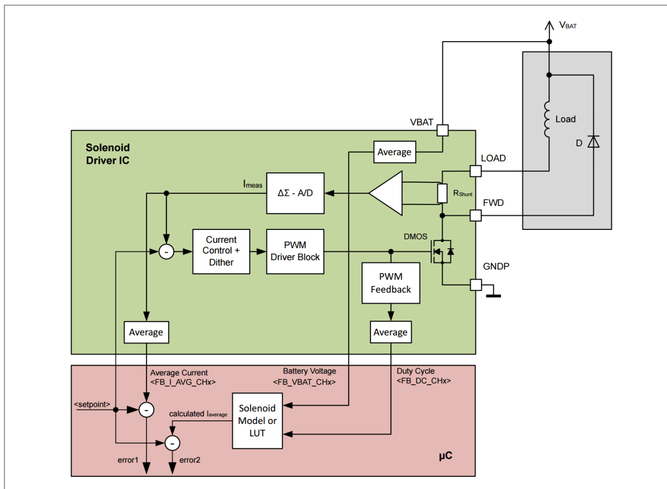
图 21 电流监控
