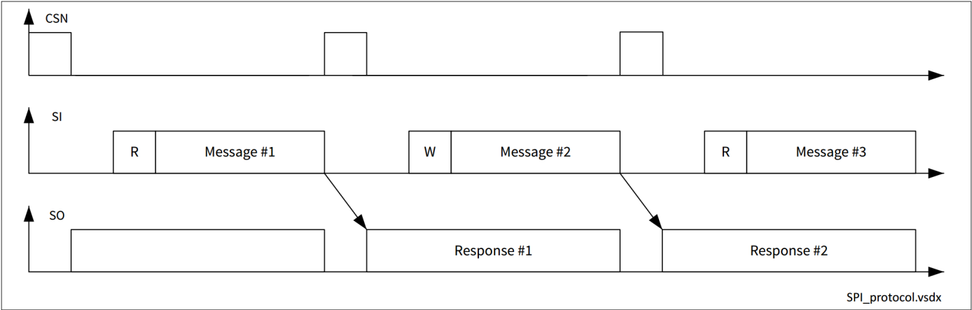
图 25 SPI 协议
