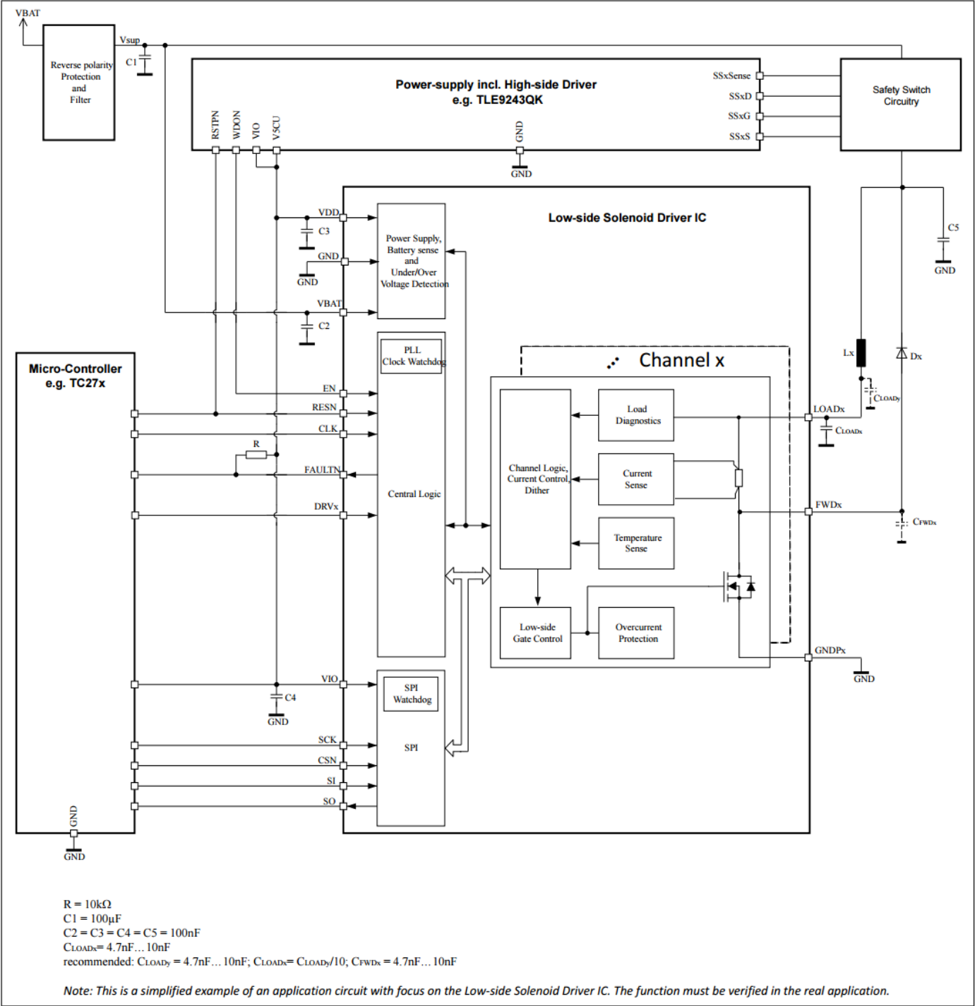
图 26 简化应用电路
