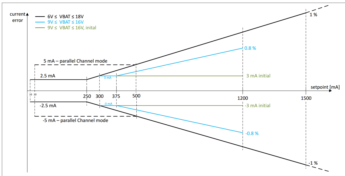
图 7 电流精度规格概述
