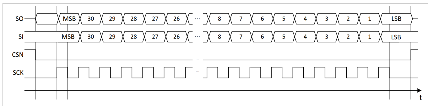
图 23 SPI信号概述
