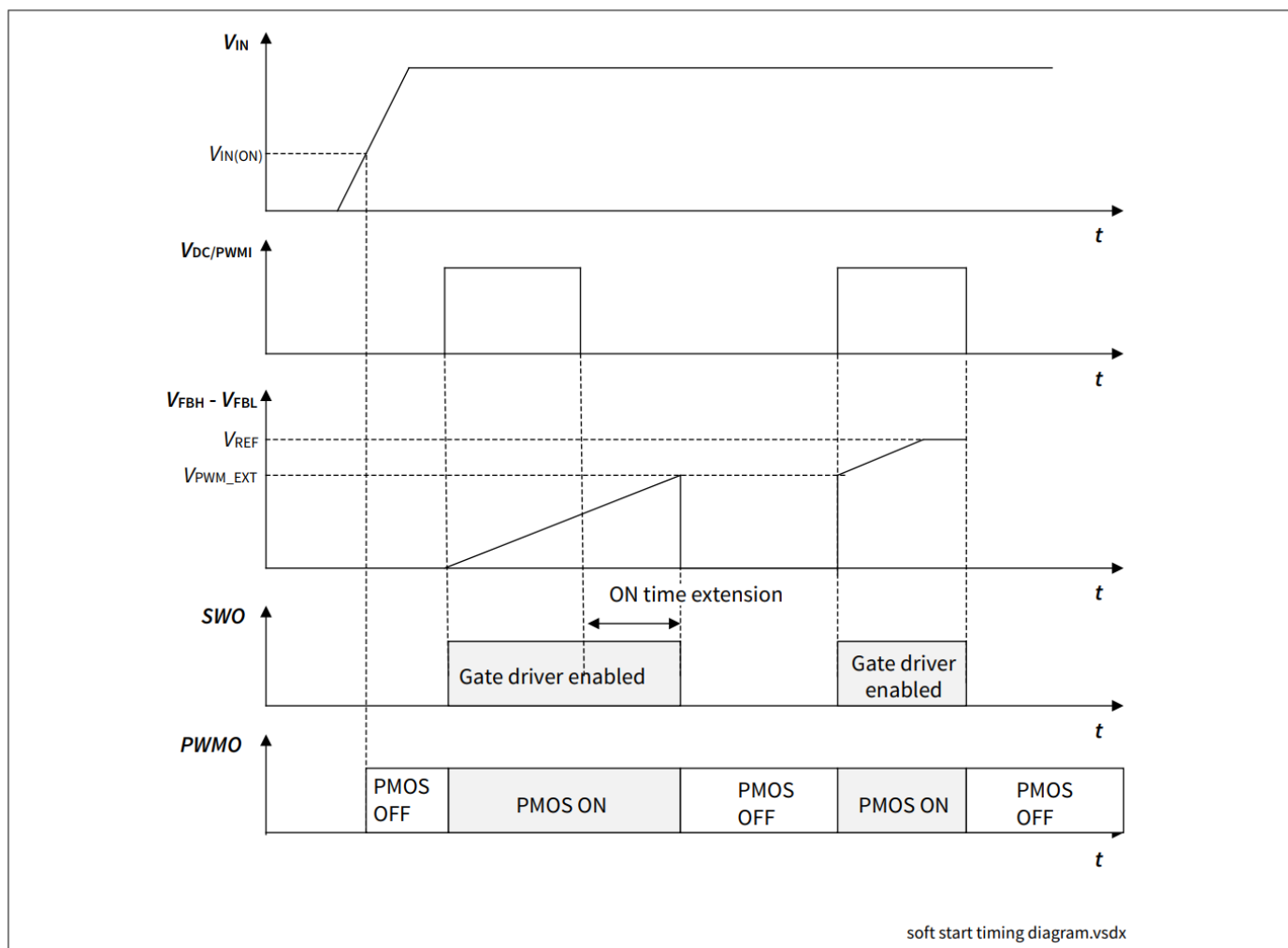
图4 软启动时序图 ( V_{FBH} 、 V_{FBL} 的线性波形是可能的情况的示例)
