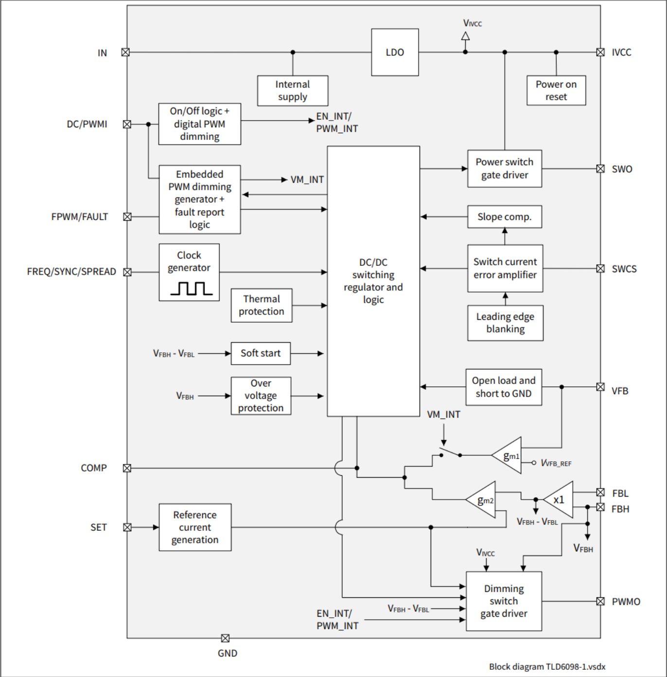
图 2 框图
