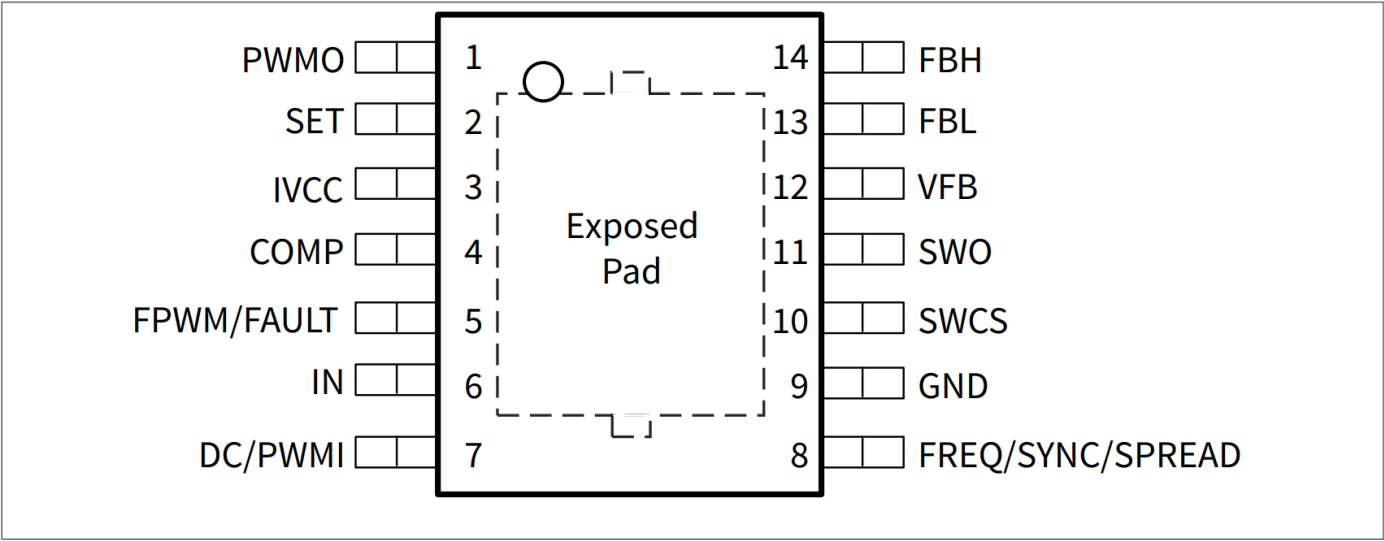
图3 PG-TSDSO-14 引脚配置
