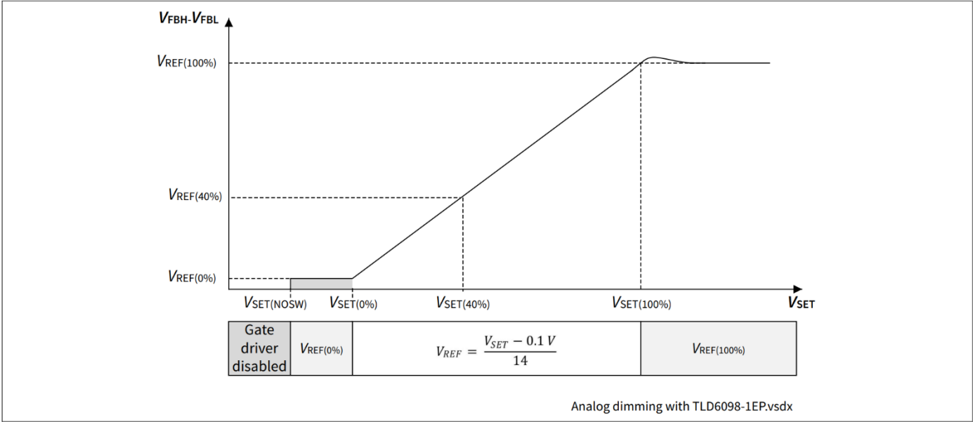
图13 V_{SET} 与基准电压 V_{REF} 的关系
