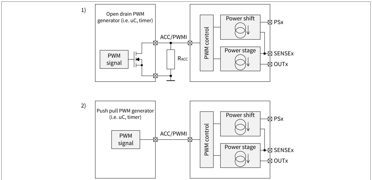
图 5 通过 ACC/PWMI 输入引脚进行 PWM 控制
