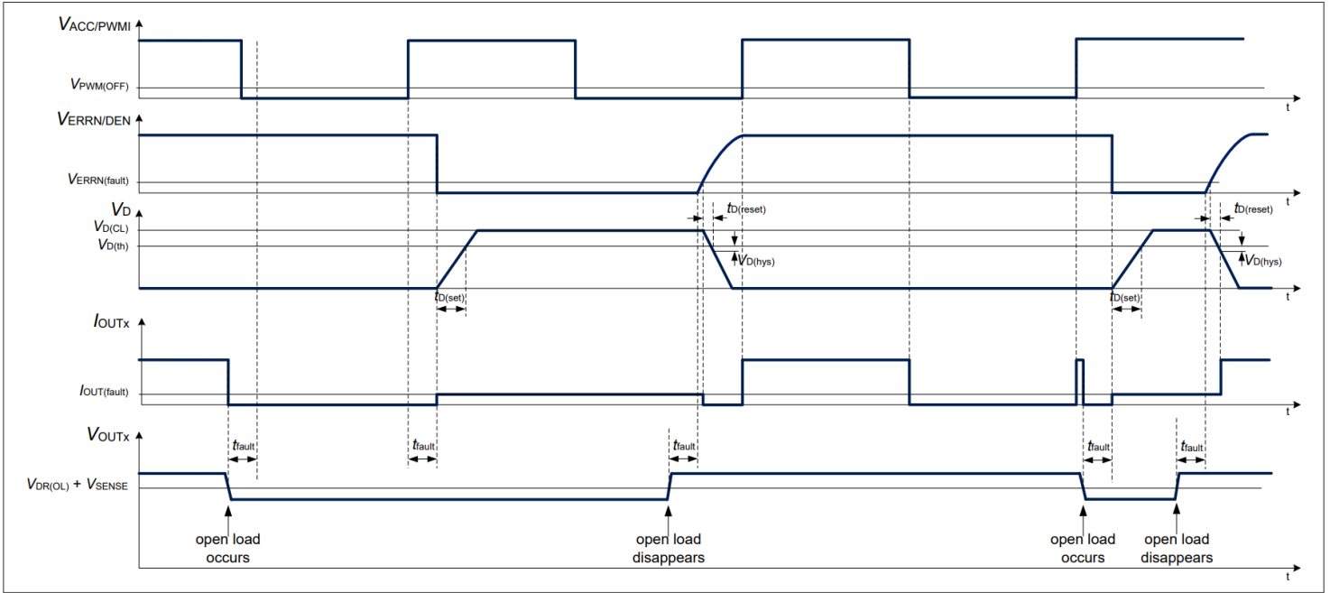
图 15 负载开路条件图示例 1-fail-all-OFF 配置（D 引脚开路或连接到外部电容器）
