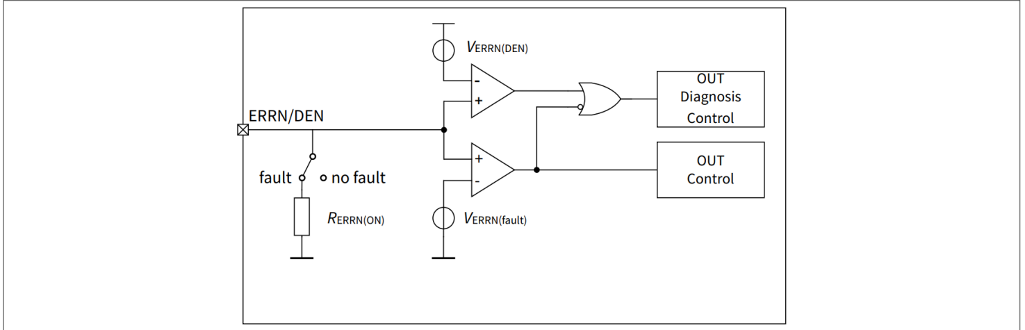
图 12 ERRN/EN 引脚框图
