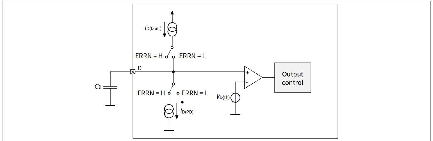
图 14 D 引脚框图
