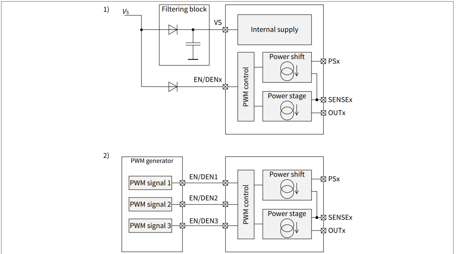
图 6 通过 EN/DENx 输入引脚进行 PWM 控制
