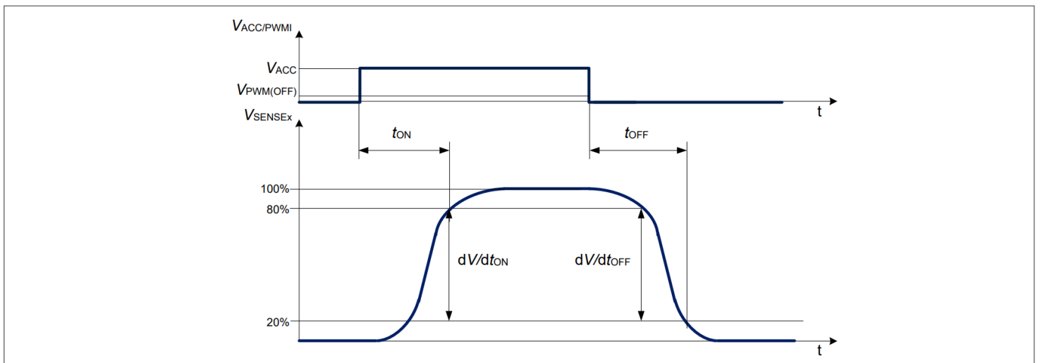
图 7 V_{ACC/PWMI} \geq 2.4 V 时的 PWMI 控制时序图
