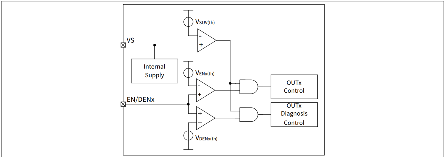
图 11 EN/DEN 框图
