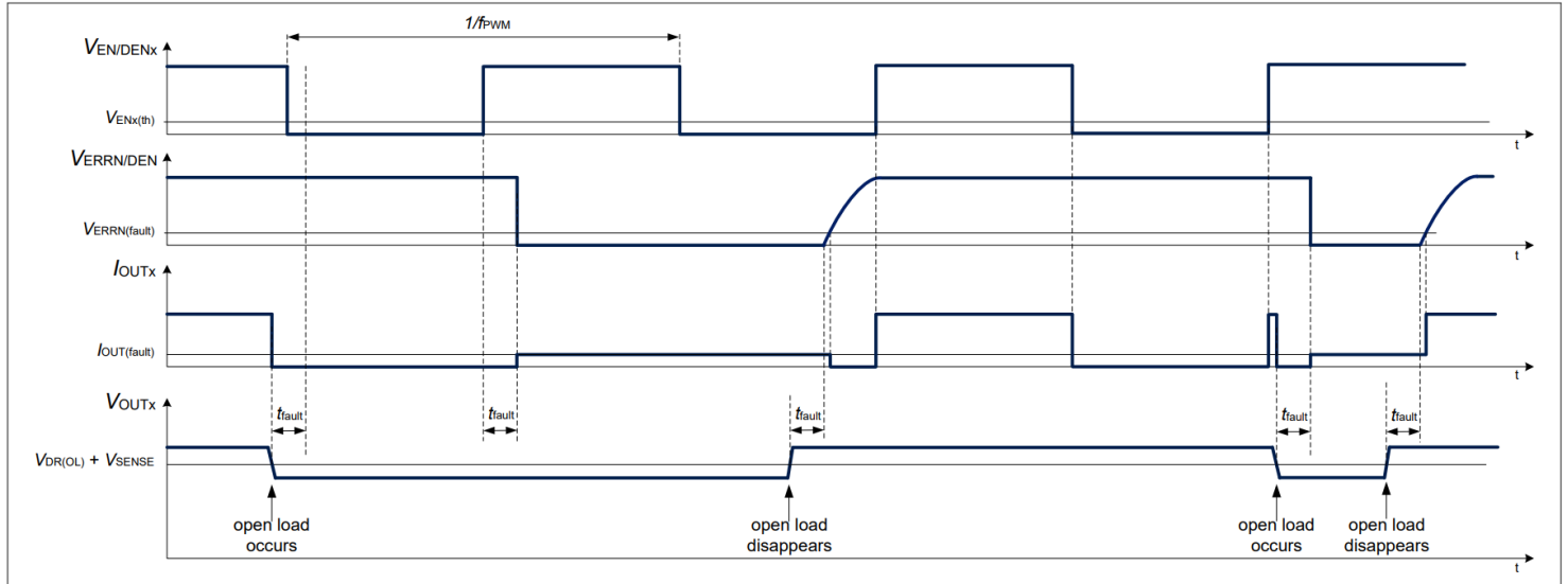
图 20 负载开路条件图示例 1-fail-all-ON 配置 (D 引脚对接地短路)，并在 EN/DENx 引脚上应用数字调光
