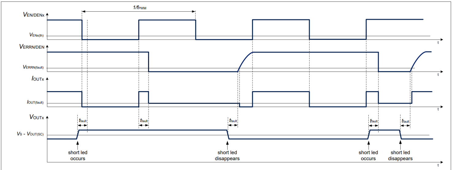
图 22 1-fail-all-ON 配置中的输出短路电源条件图示例 (D 引脚对接地短路), 并在 EN/DENx 引脚上应用数字调光。
