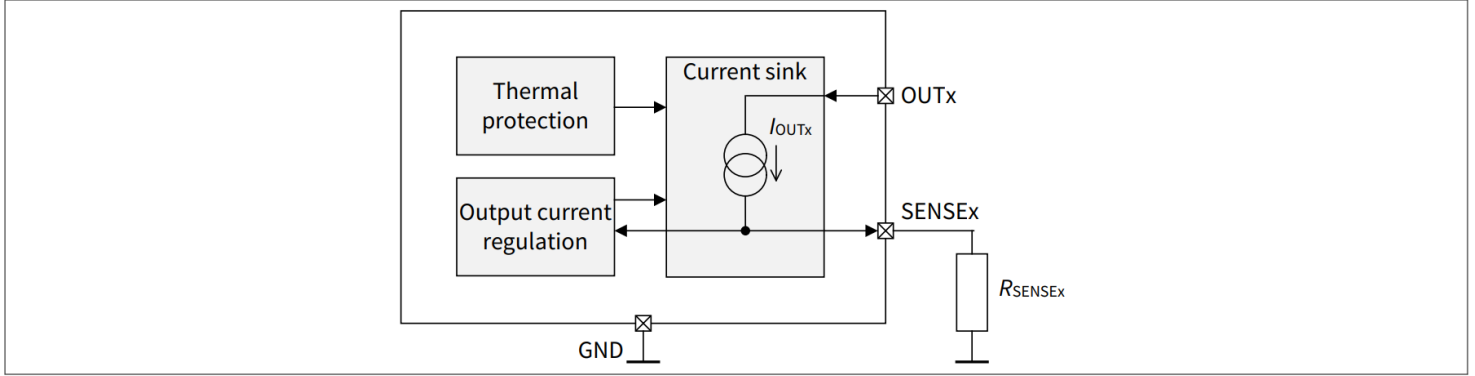
图 4 功率级框图
