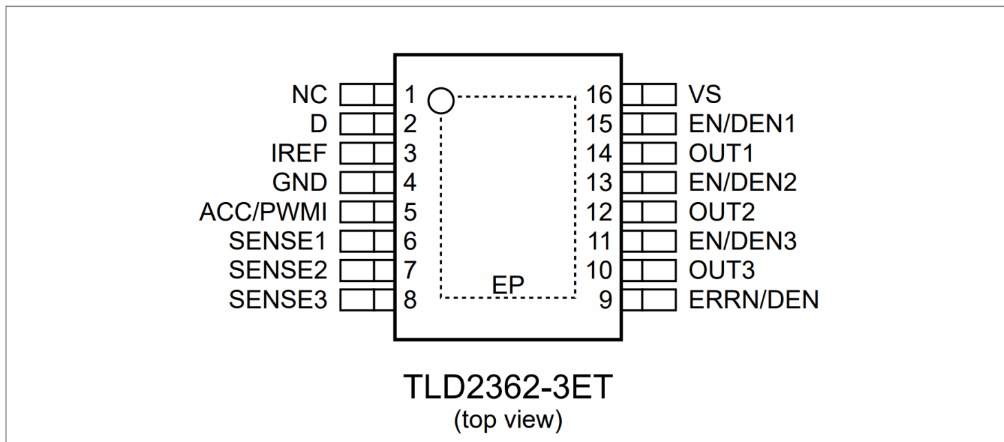
图2 PG-TFDSO-16 引脚配置
