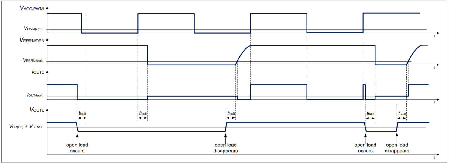
图 19 负载开路条件图示例 1-fail-all-ON 配置 (D 引脚短接到接地)
