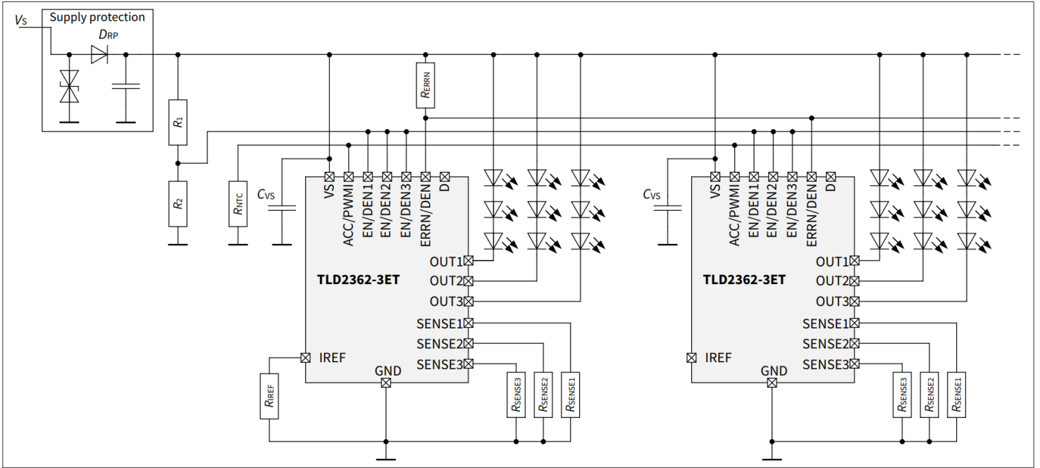
图 23 具有“一错全关”故障管理和中央热降额的共享网络中的应用图示例
