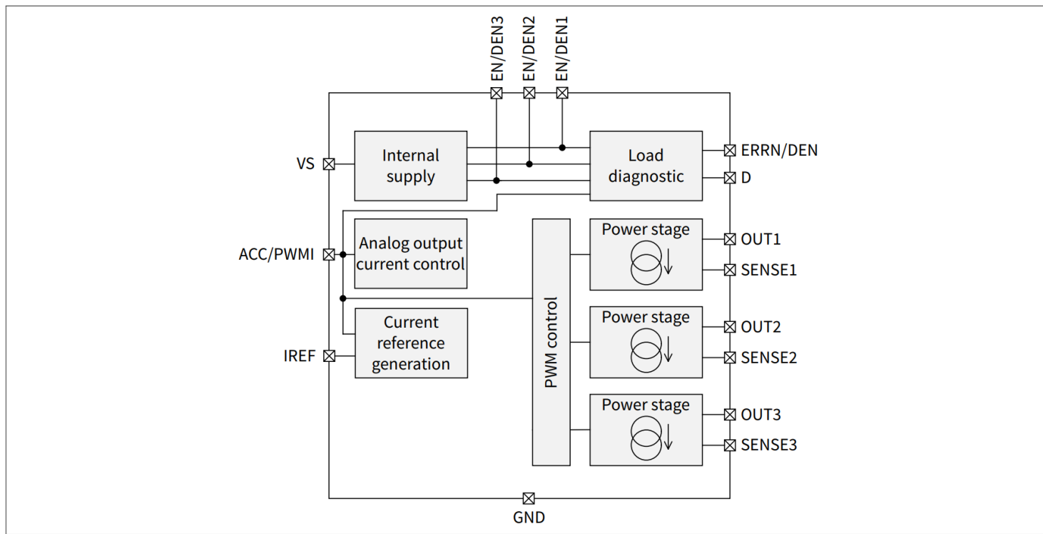
图 1 TLD2362-3ET 框图
