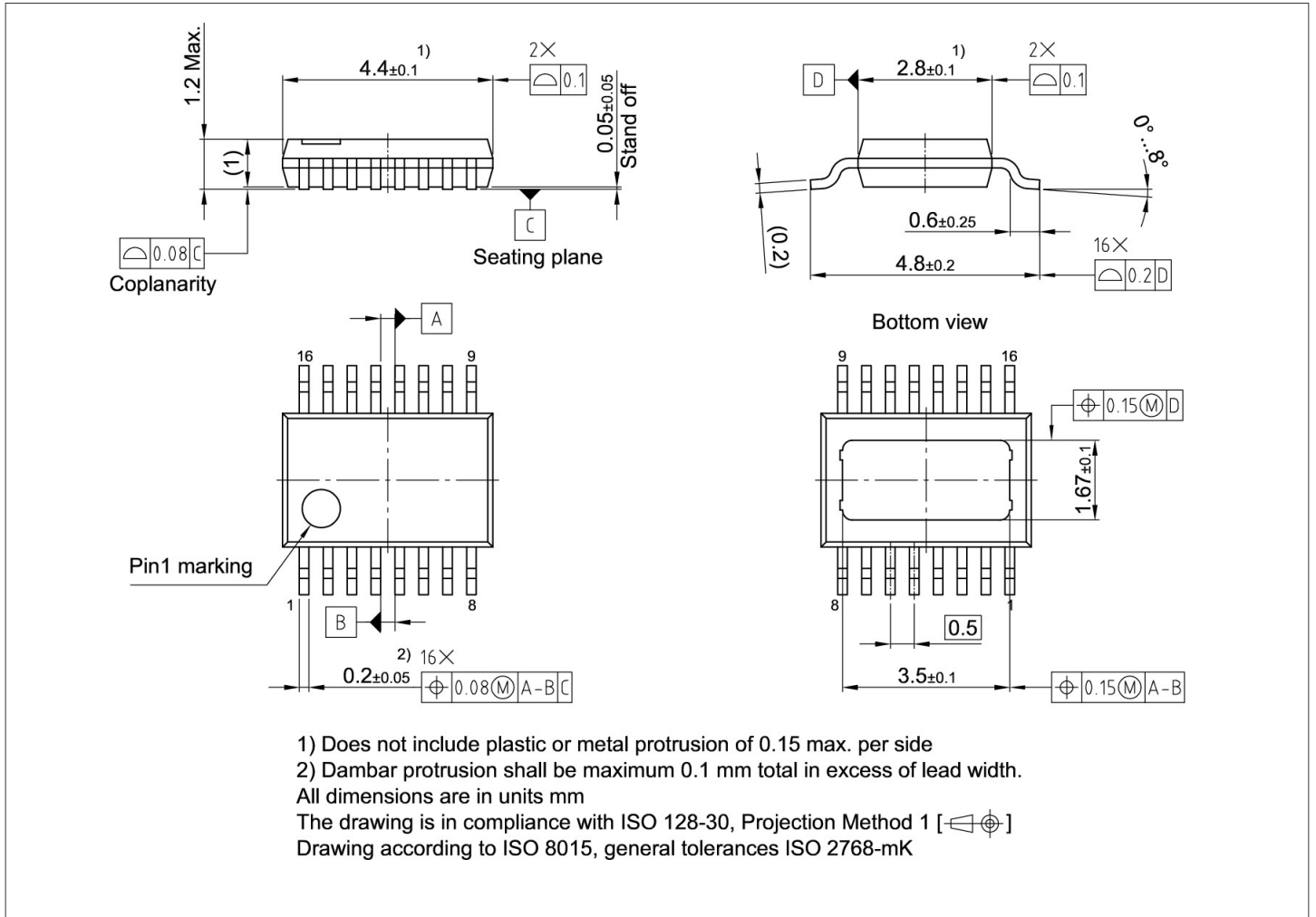
图 25 PG-TFDSO-16 封装外形 png
