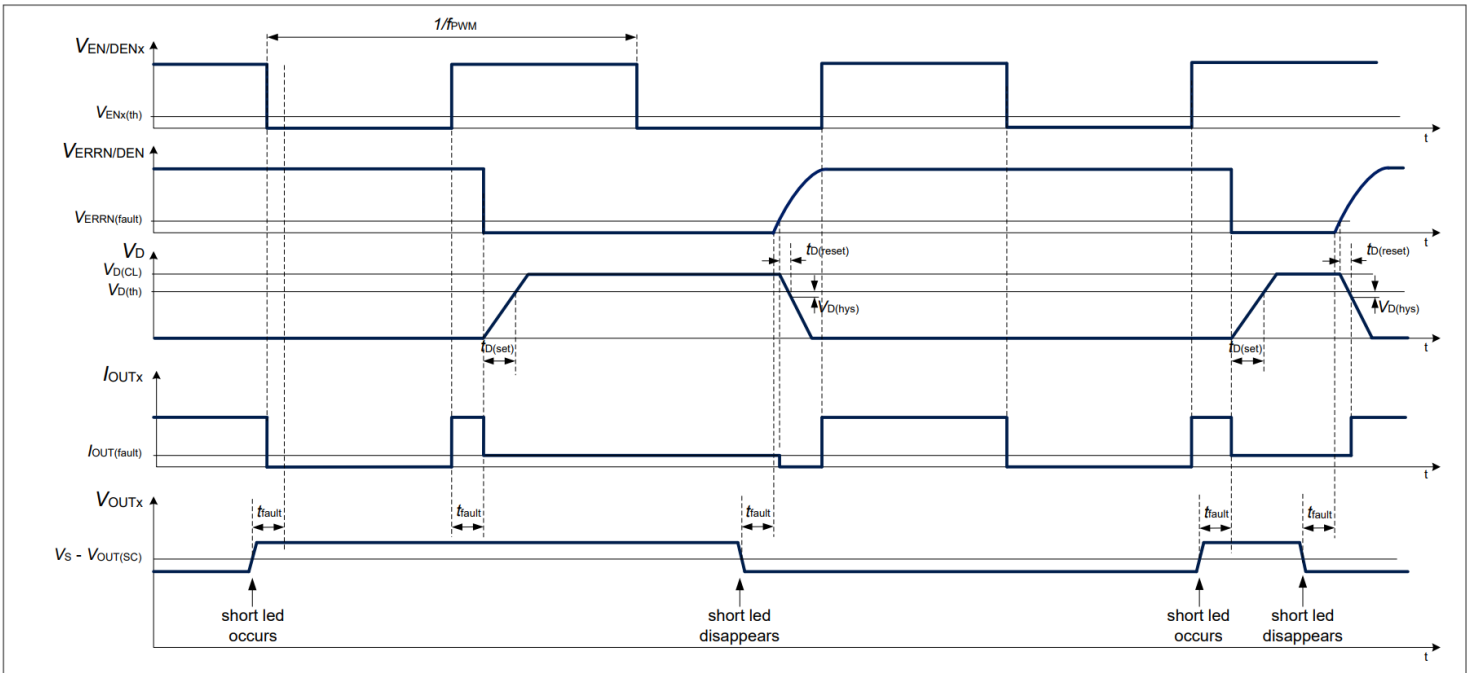
图 18 1-fail-all-OFF 配置中的输出短路电源条件时序图示例（D 引脚开路或连接到外部电容器），并在 EN/DENx 引脚上应用数字调光。
