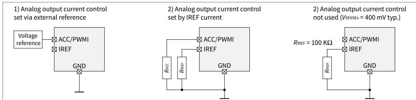
图 10 模拟输出电流控制配置
