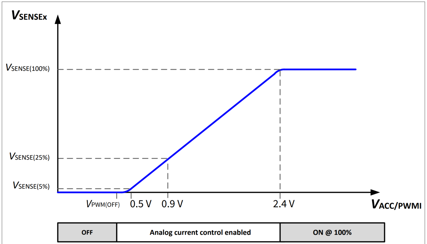
图9 模拟输出电流控制
