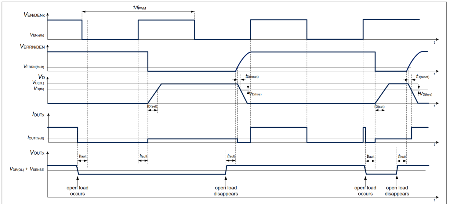
图 16 负载开路条件图示例 1-fail-all-OFF 配置（D 引脚开路或连接到外部电容器），并在 EN/DENx 引脚上应用数字调光
