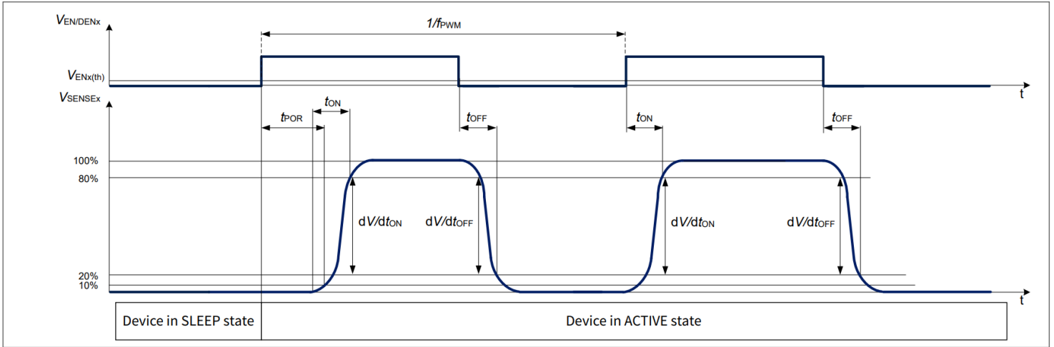
图 8 V_{ACC/PWMI} \geq 2.4V 时 EN/DENx 上的 PWM 控制时序图
