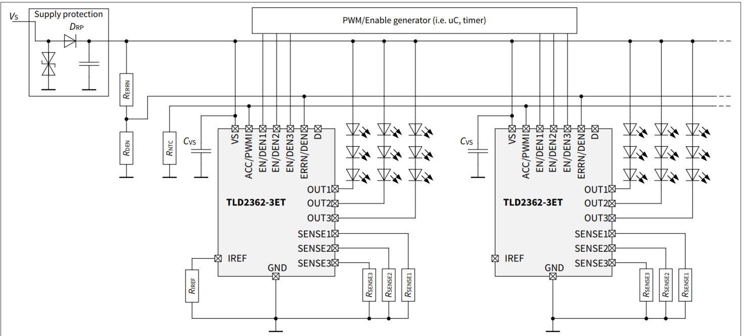
图 24 共享网络中动态照明功能的应用图示例，具有“一错全关”故障管理和中央热降额功能
