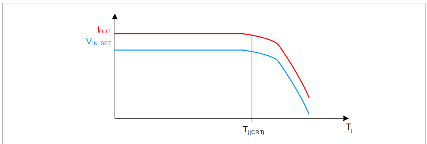
图19 高温下输出电流减少
