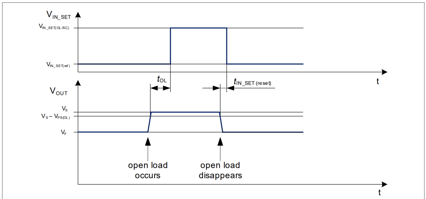
图 14 ST 引脚接地且 V_{DEN} > V_{DEN(akt)} 时负载开路条件下 IN_SET 的行为
