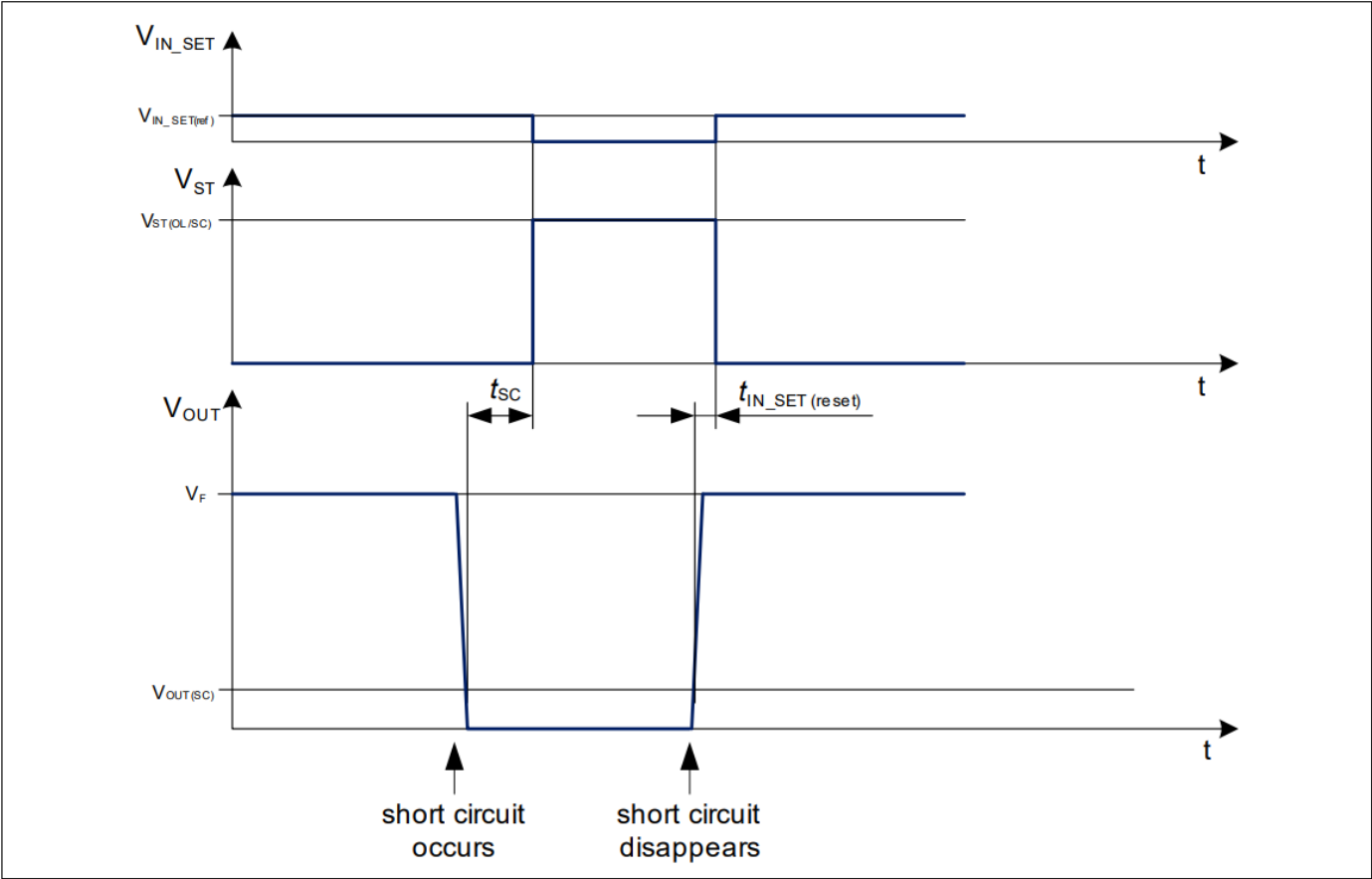
图 17 发生对地短路条件（ST 未连接）且 V_{DEN} > V_{DEN(act)} 期间 IN_SET 和 ST 的行为
