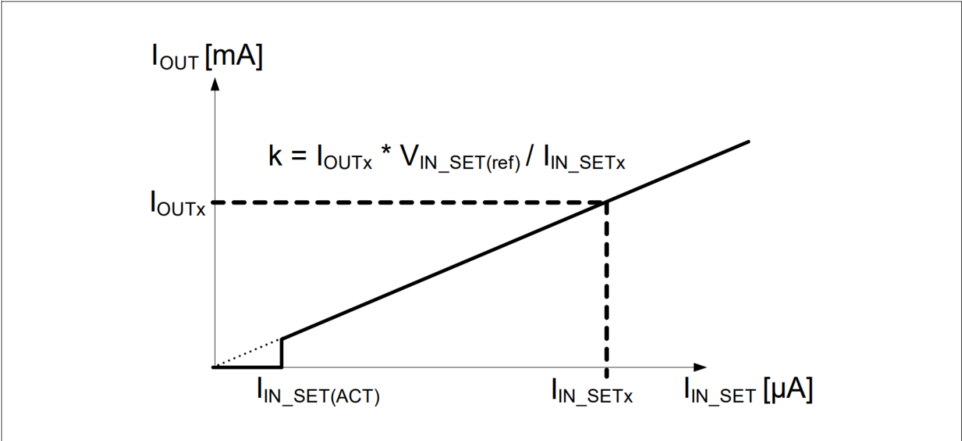
图 10 I_{OUT} 与 I_{INSET}
