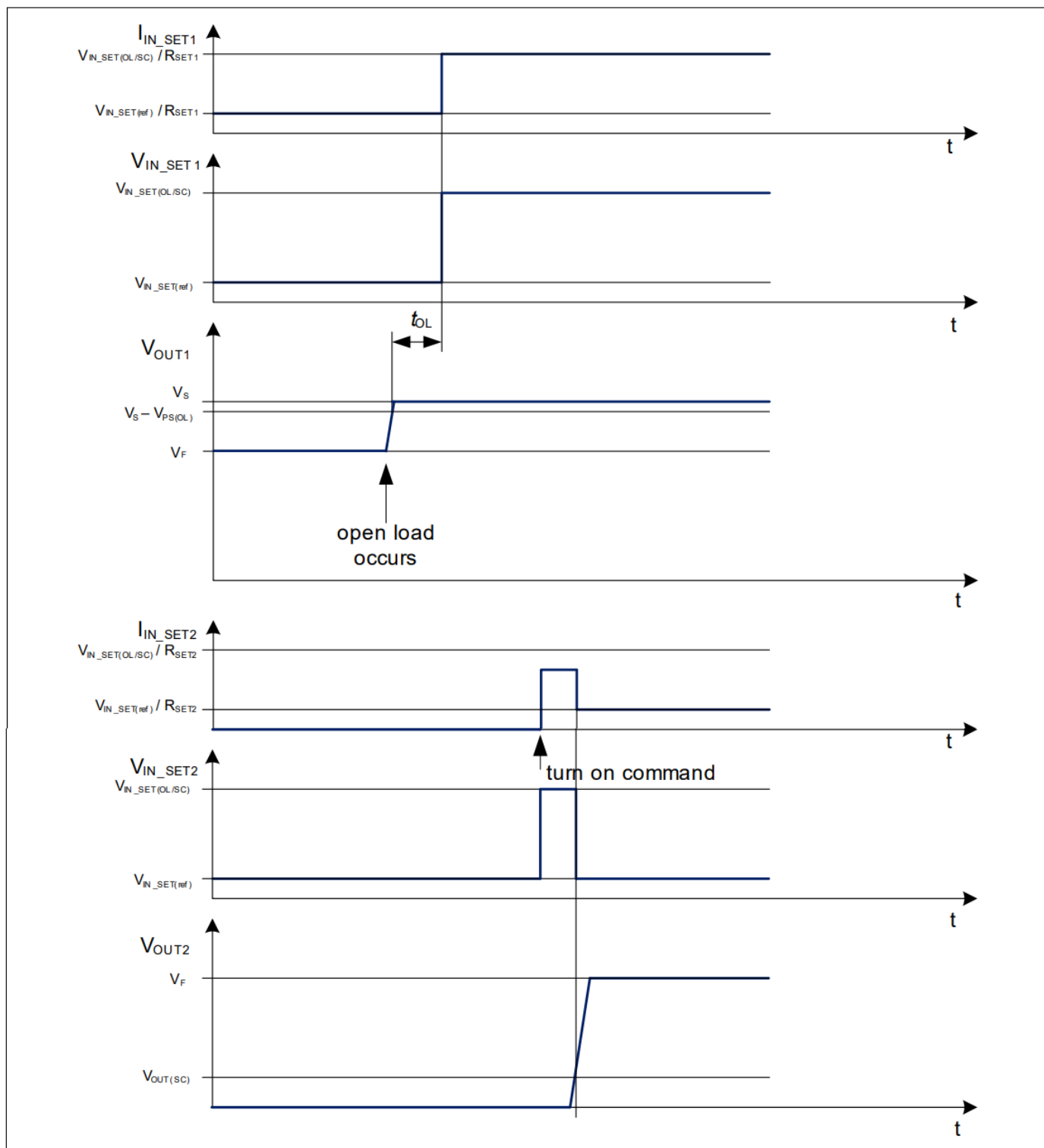
图 18 OUT1 上的单通道故障示例，OUT2 工作在PWM模式，ST 引脚接地且 V_{DEN} > V_{DEN(act)}
