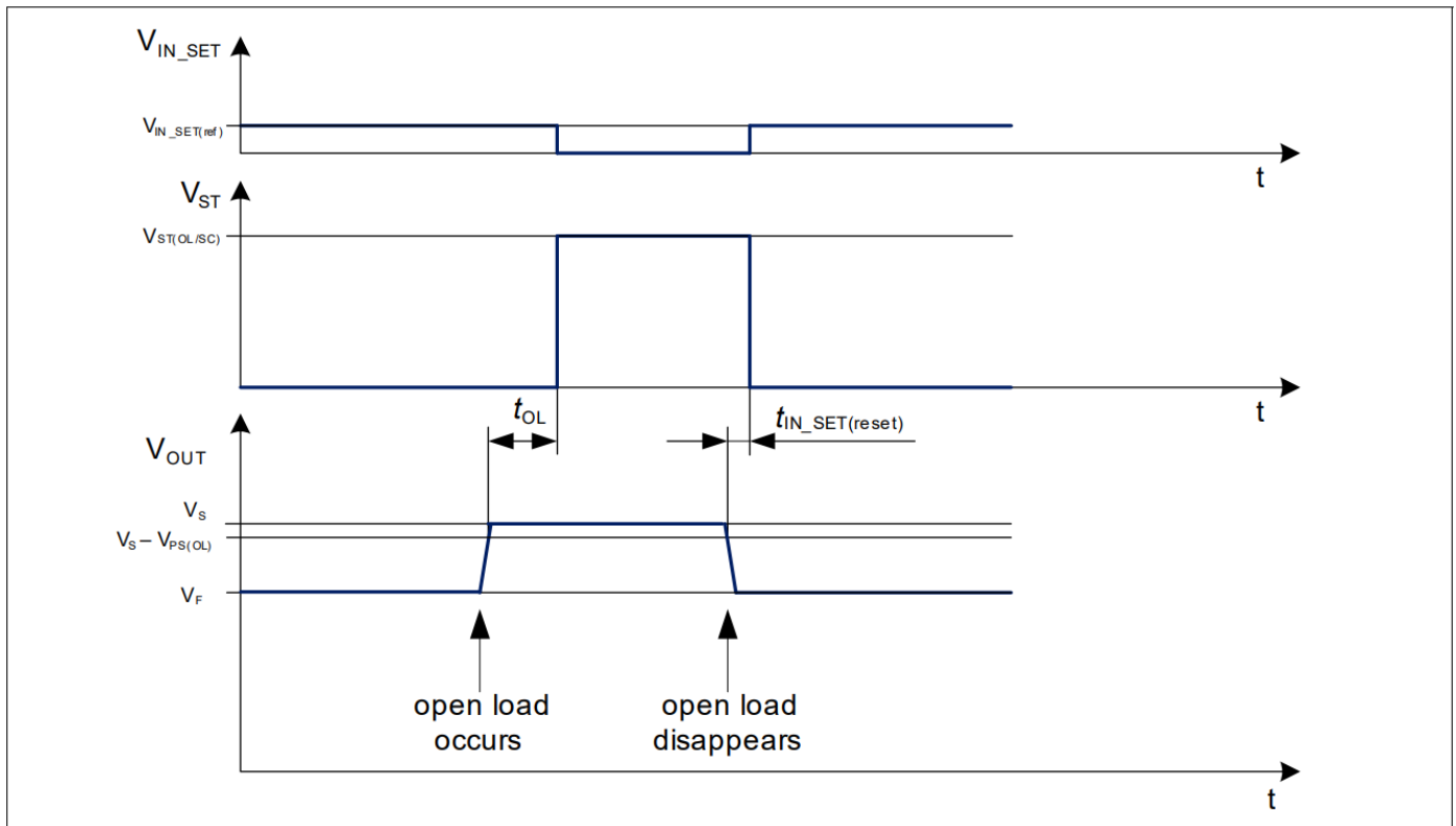
图 15 负载开路条件（ST 未连接）且 V_{DEN} > V_{DEN(akt)} 期间 IN_SET 和 ST 的行为
