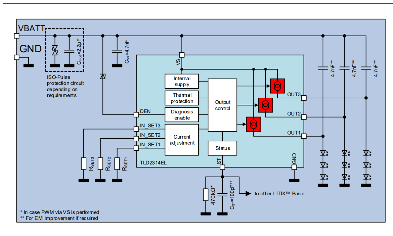
TLD2314EL 应用图
