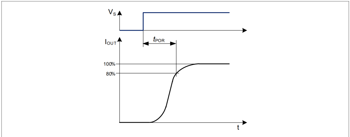
图5 上电复位
