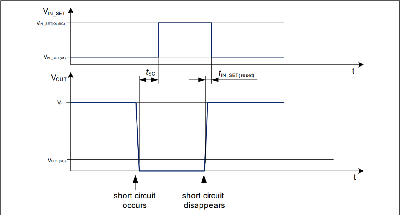
图 16 ST 接地且 V_{DEN} > V_{DEN(act)} 时发生对地短路条件期间的 IN_SET 行为
