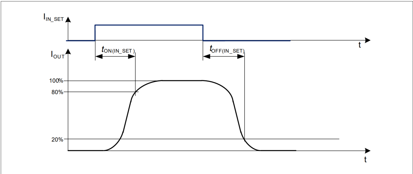
图 9 通过 IN_SET 的开关时间
