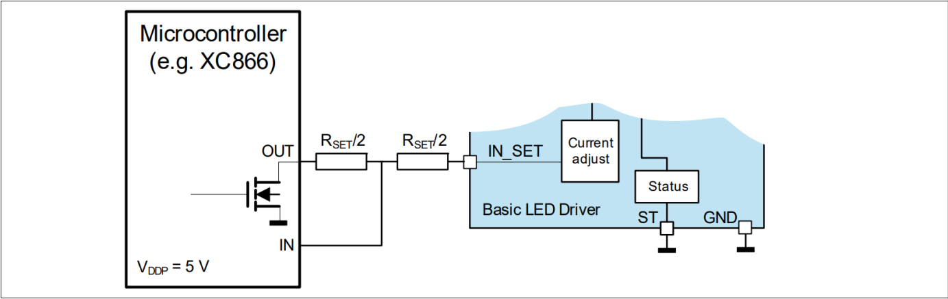
图 7 原理图 IN_SET 接口至 \mu\text{C} ，通过 IN_SET 引脚进行诊断
