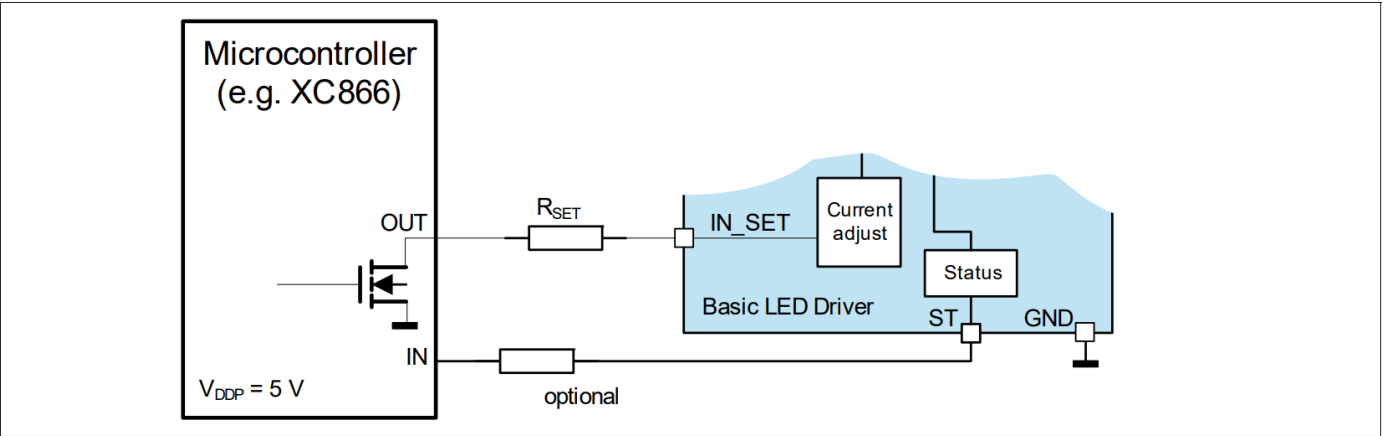
图 8 原理图 IN_SET 接口至 \mu\text{C} ，通过 ST 引脚进行诊断
