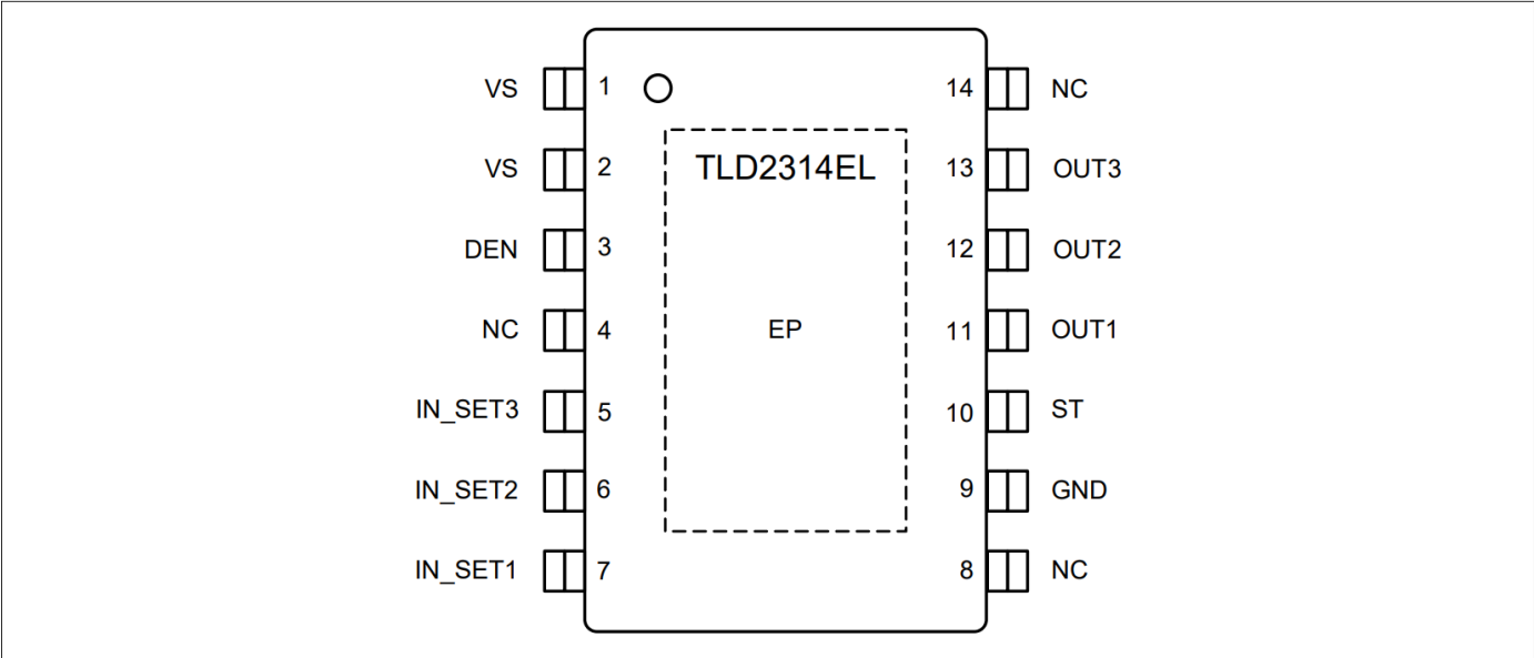
图 2 引脚配置
