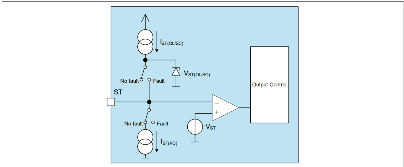
图 12 ST 引脚框图
