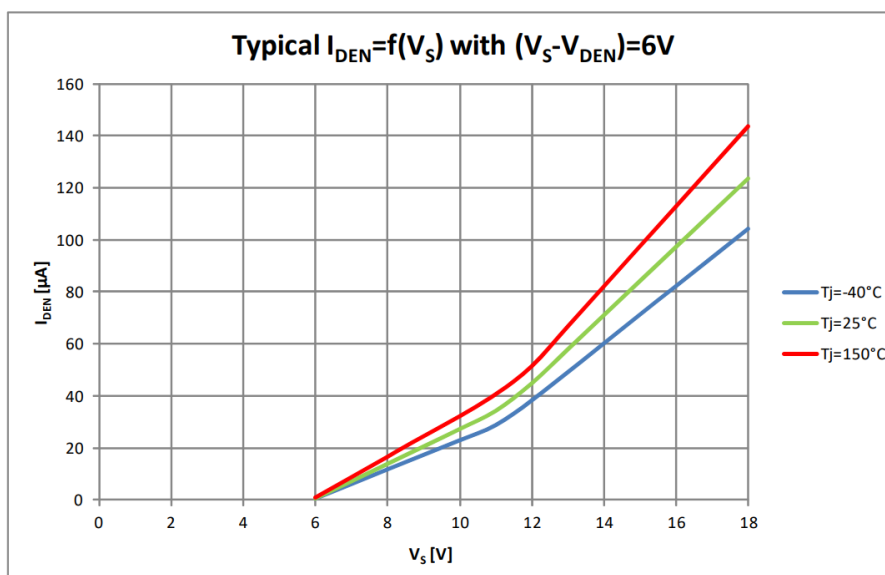
图 4 齐纳二极管电压为 6 V 时的典型 I_{DEN(H)} 电流
