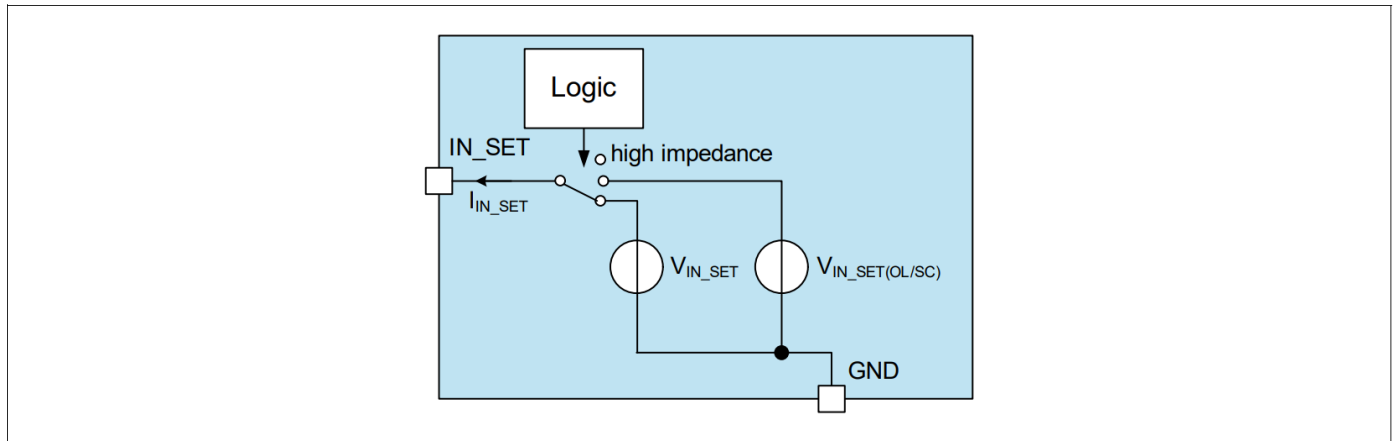
图 6 IN_SET 引脚框图
