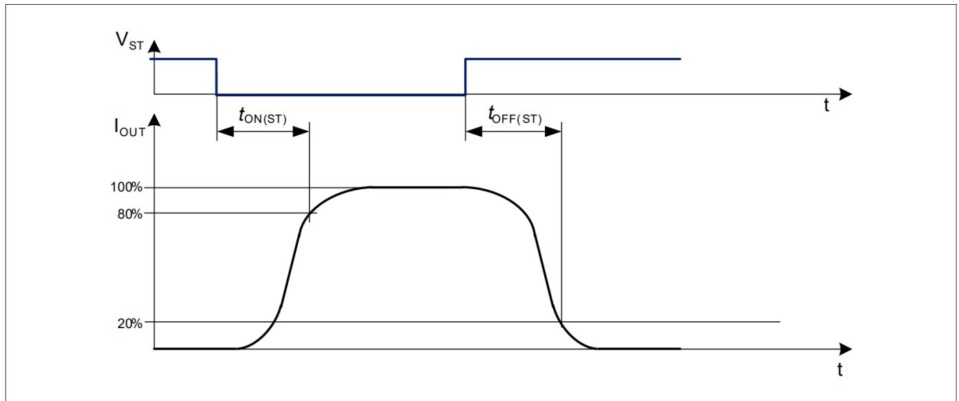
图 13 通过 ST 引脚的开关时间
