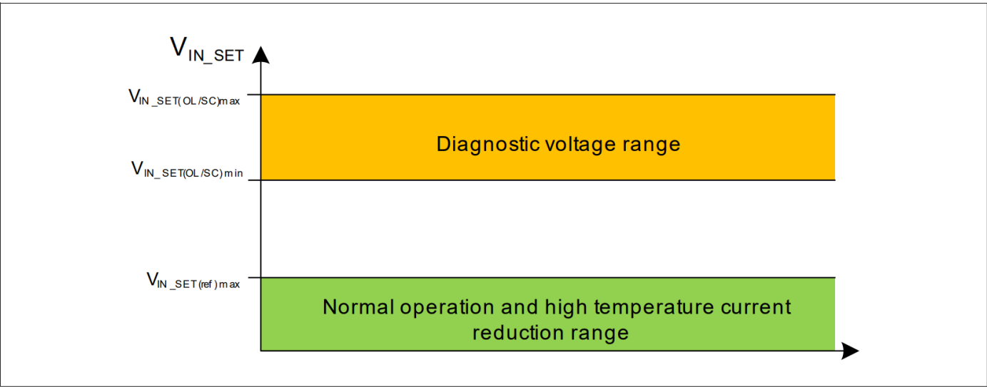
图 11 IN_SET 引脚的电压域（如果 ST 引脚接地）
