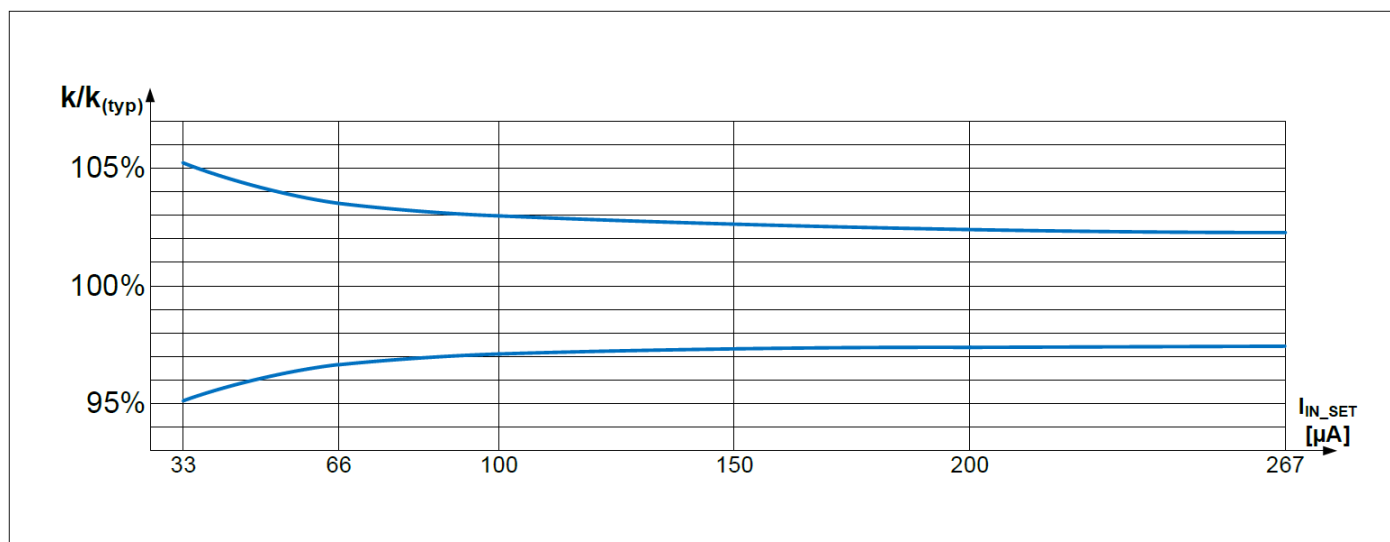
图 8 T_J = 25^\circ C 时的典型输出电流精度 I_{OUT} / I_{IN\_SET}
