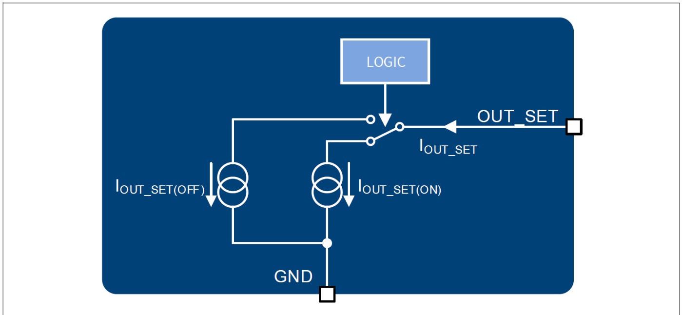
图 10 OUT_SET 引脚框图
