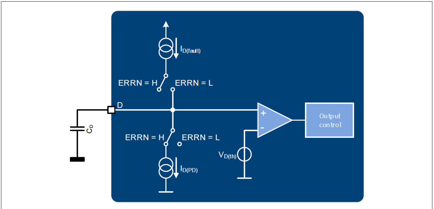
图 17 D 引脚（框图）。
