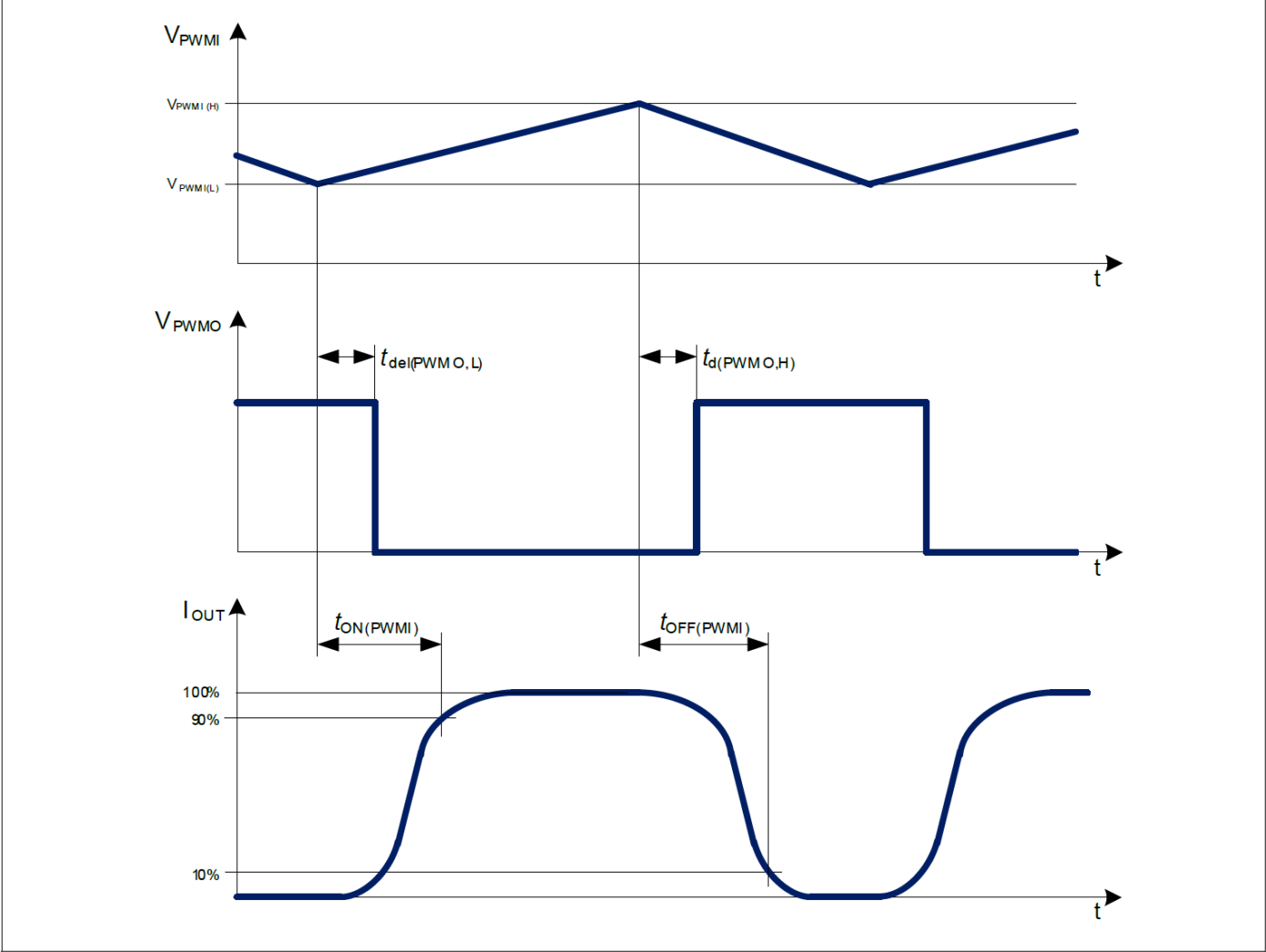
图 24 PWM引擎时序概述
