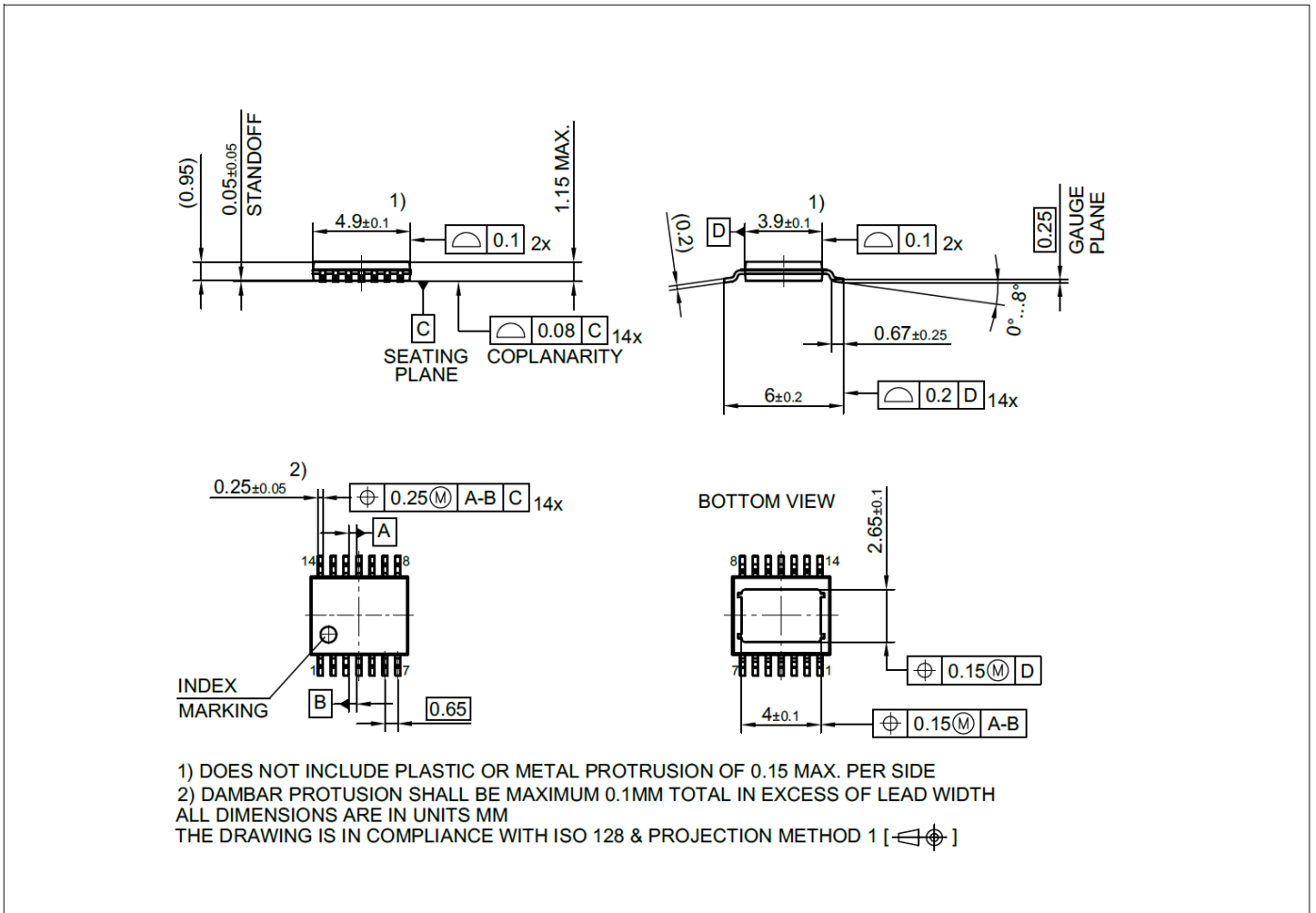
图 28 PG-TSDSO-14
