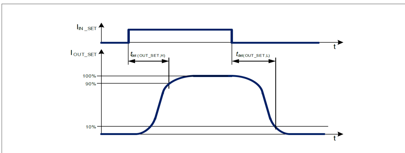
图13 IN_SET至OUT_SET激活和停用延迟时序图
