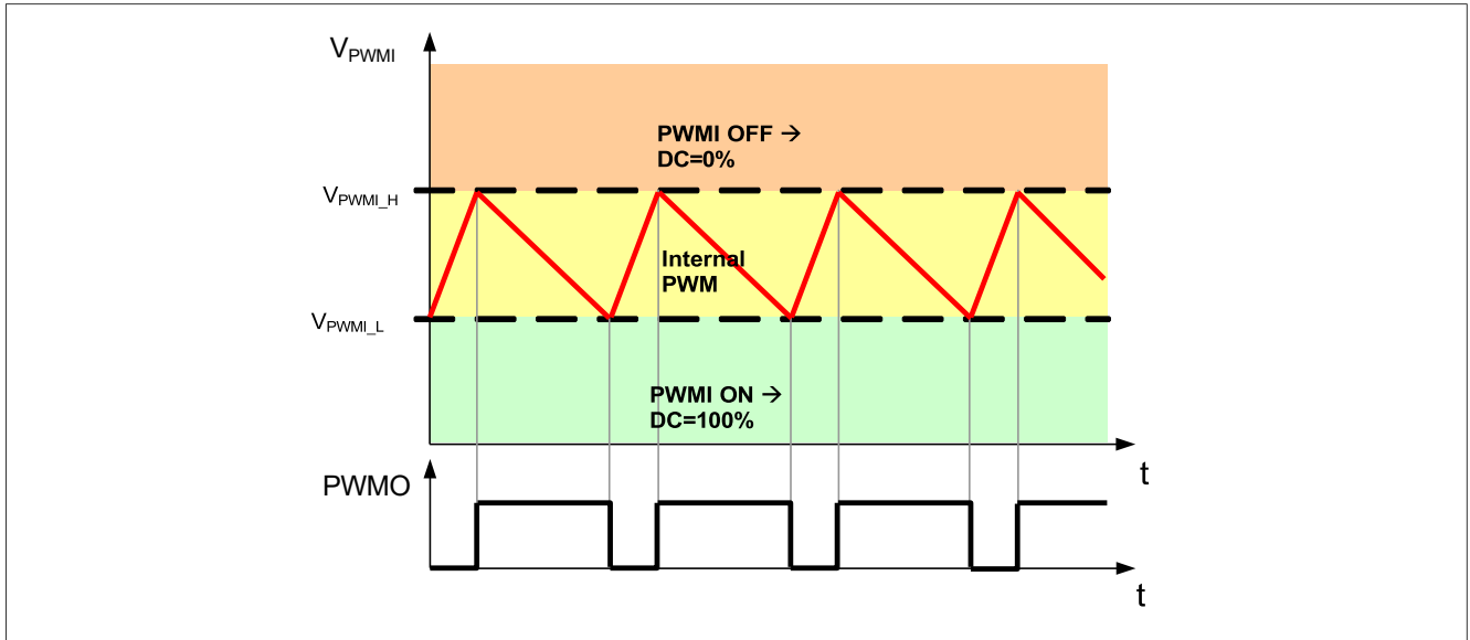
图 23 PWMI 工作电压和时序图示例
