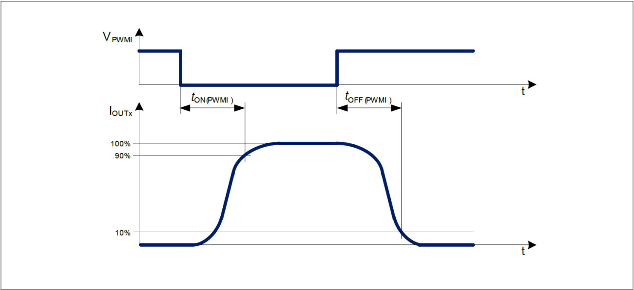
图25 输出激活延迟时序图
