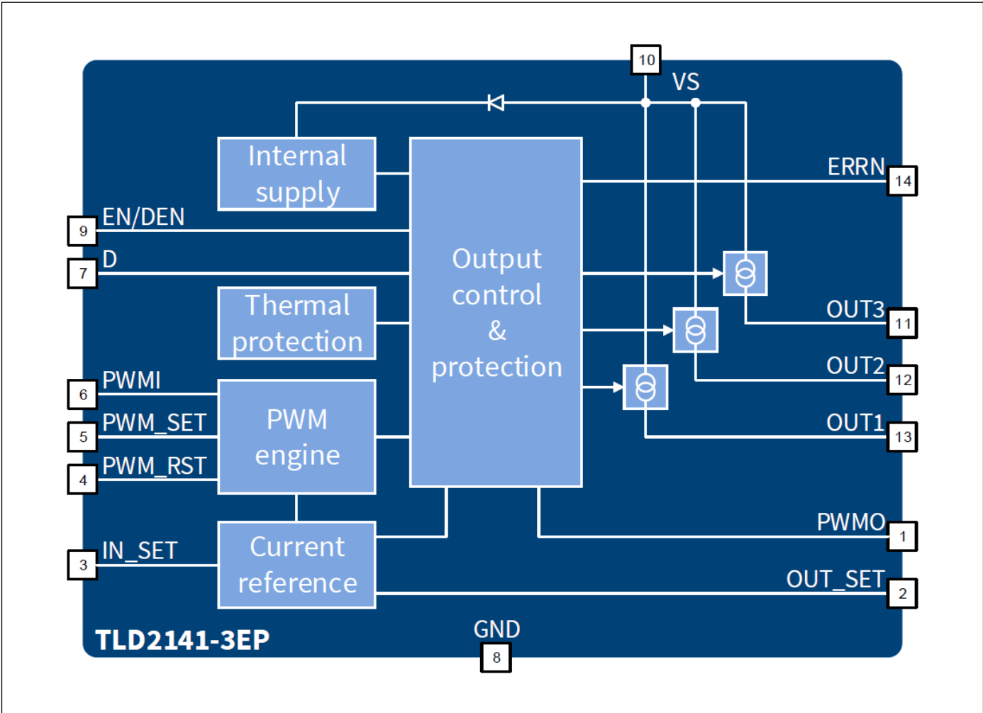
图 1 框图
