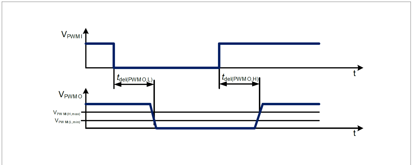
图26 PWMO延迟时序图
