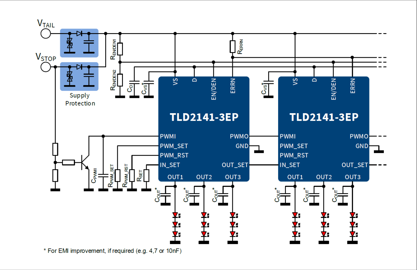
图 27 应用图示例
