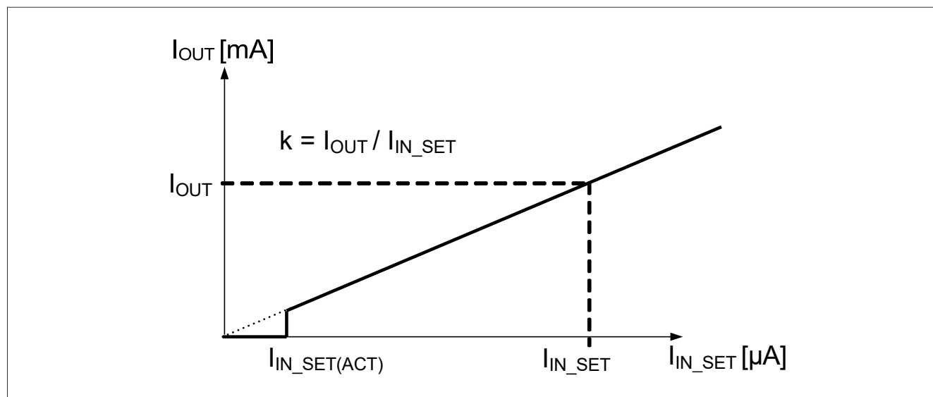
图 7 I_{OUT} 与 I_{IN\_SET}
