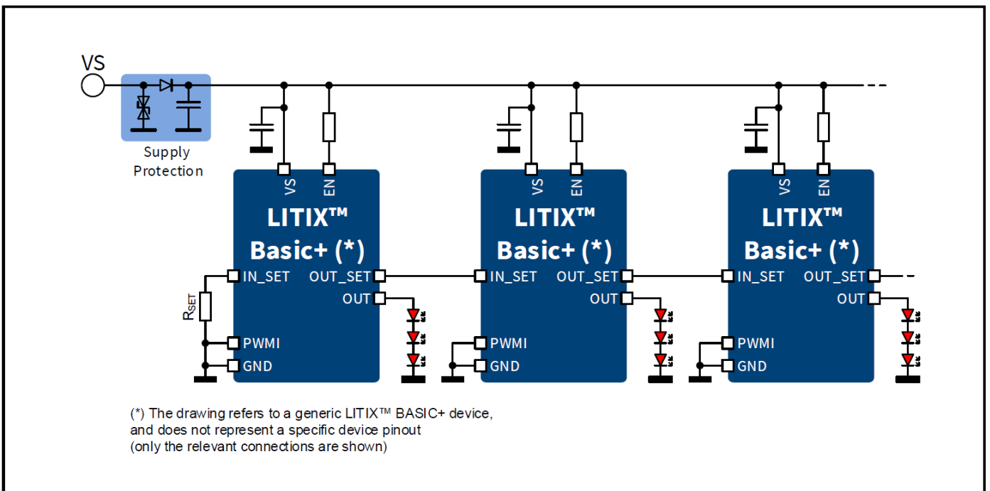
图 11 IN_SET 至 OUT_SET 串行连接示例
