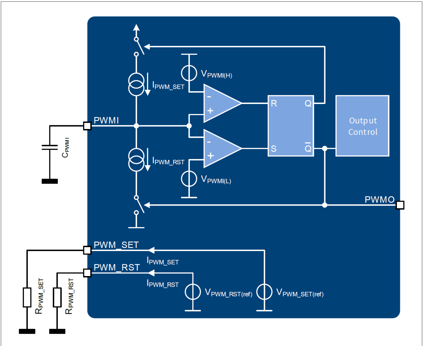
图22 PWM单元概念图（包括PWMO驱动和典型外部电路）
