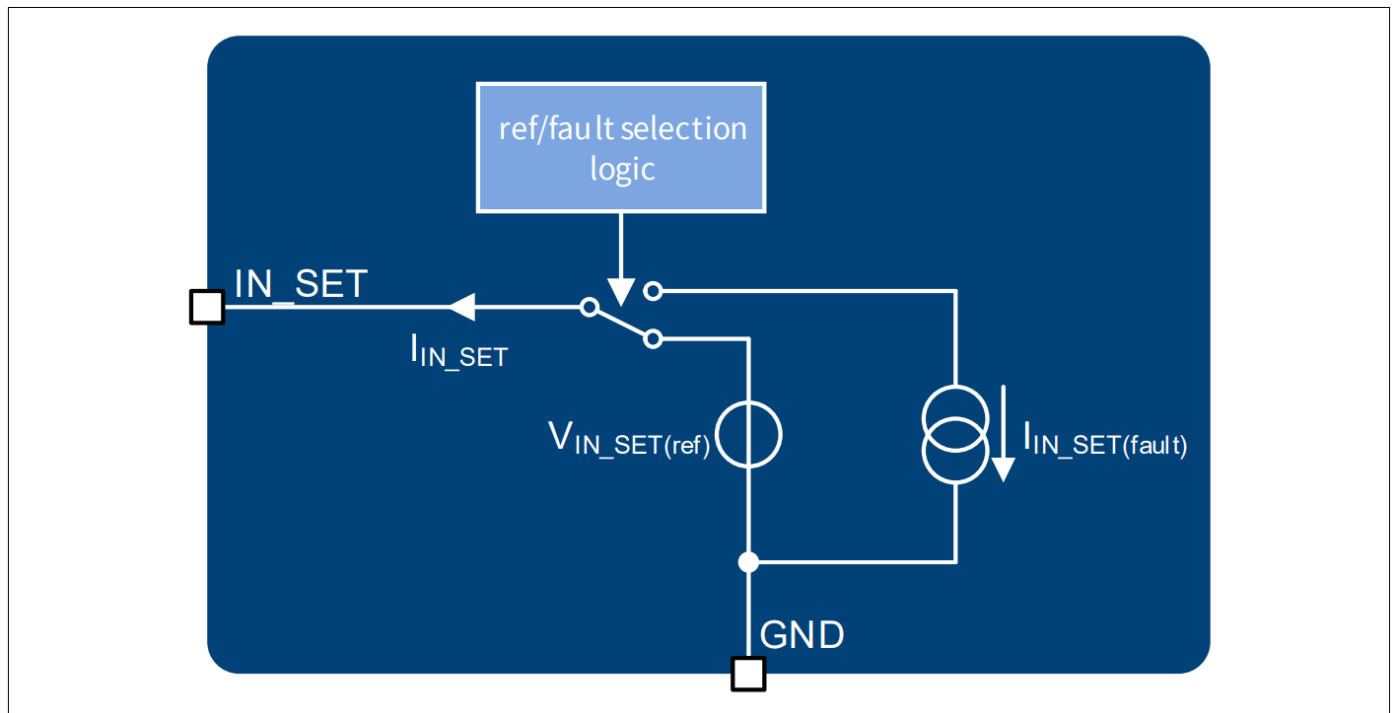
图6 IN_SET 引脚框图
