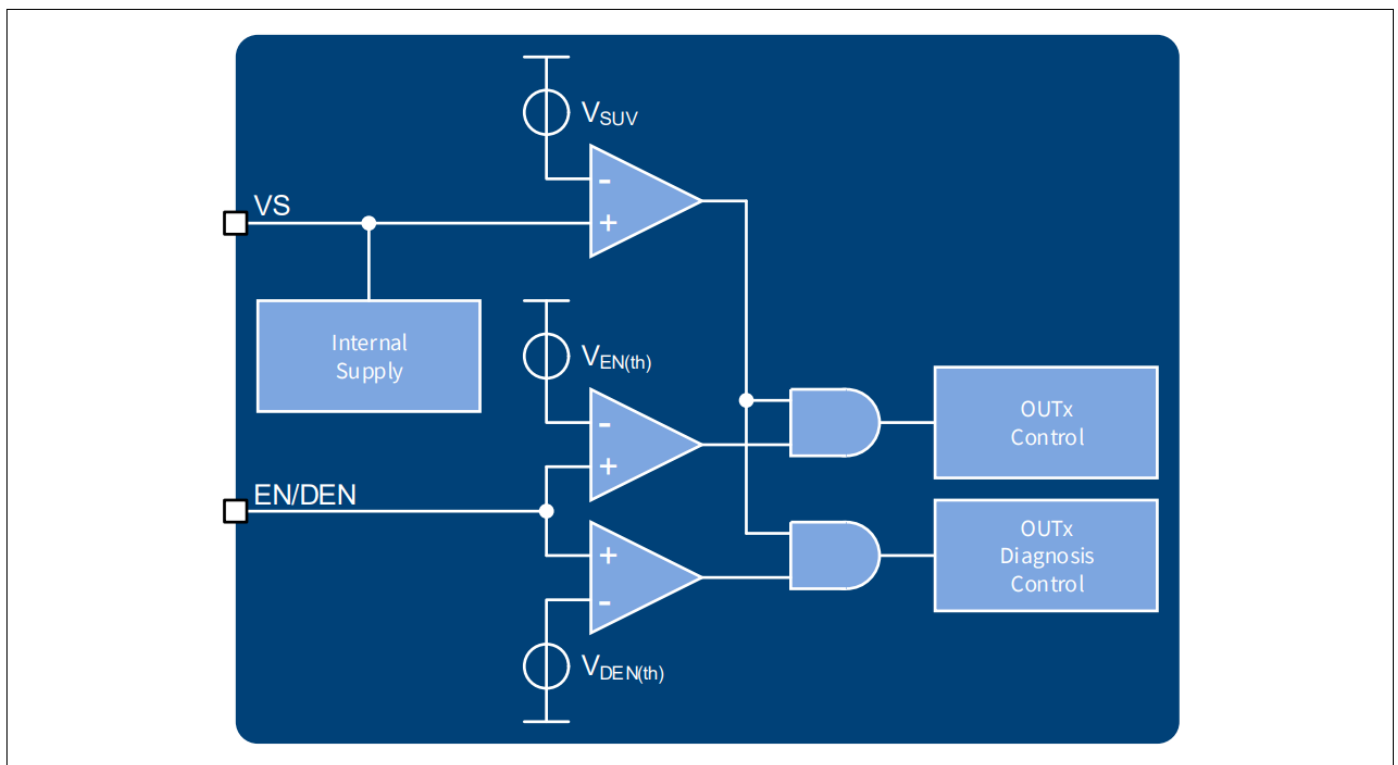
图 3 内部供电
