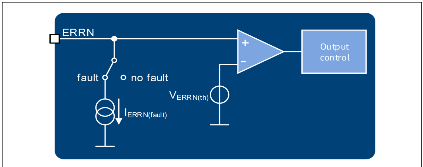
图 15 ERRN 引脚（框图）
