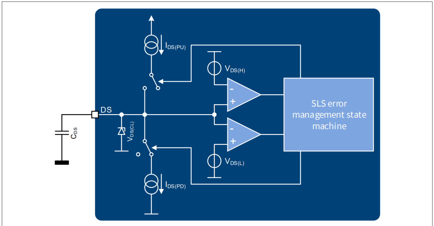
图 23 DS引脚（框图）
