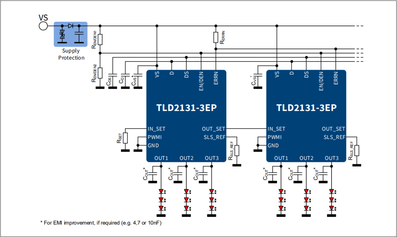
图 26 应用图示例
