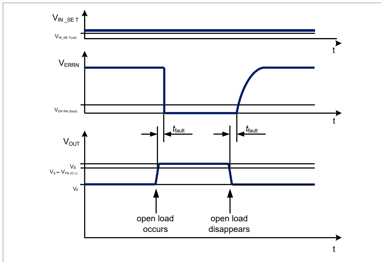
图 20 负载开路条件时序图示例（D引脚接 GND， V_{\text{F}} 代表输出负载的正向电压）
