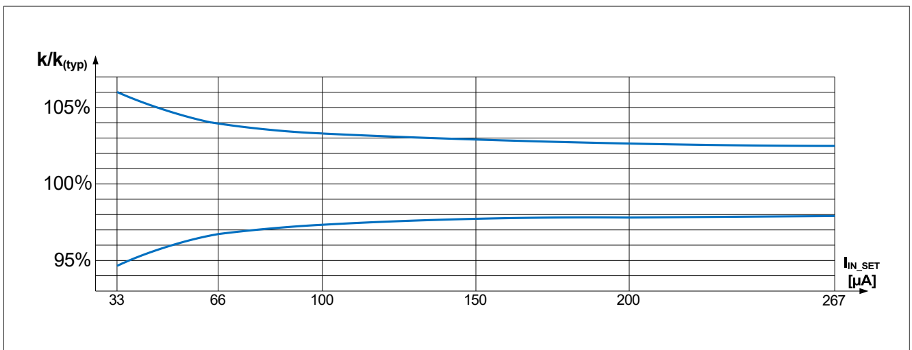
图 8 T_J = 25^{\circ}\text{C} 时的典型输出电流精度 I_{OUT}/I_{IN\_SET}
