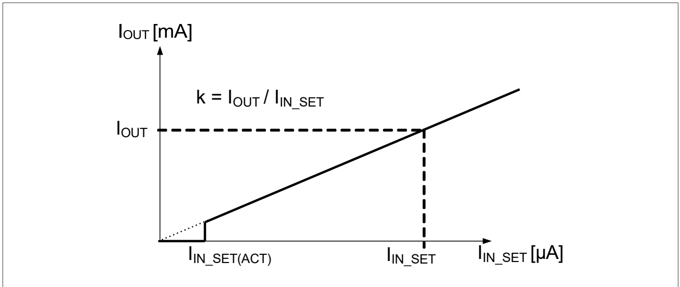
图 7 I_{OUT} 与 I_{IN\_SET}
