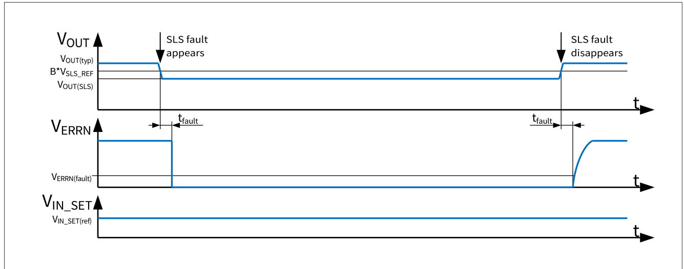
图 25 单LED短路条件图示例 (D 引脚短接到 GND)
