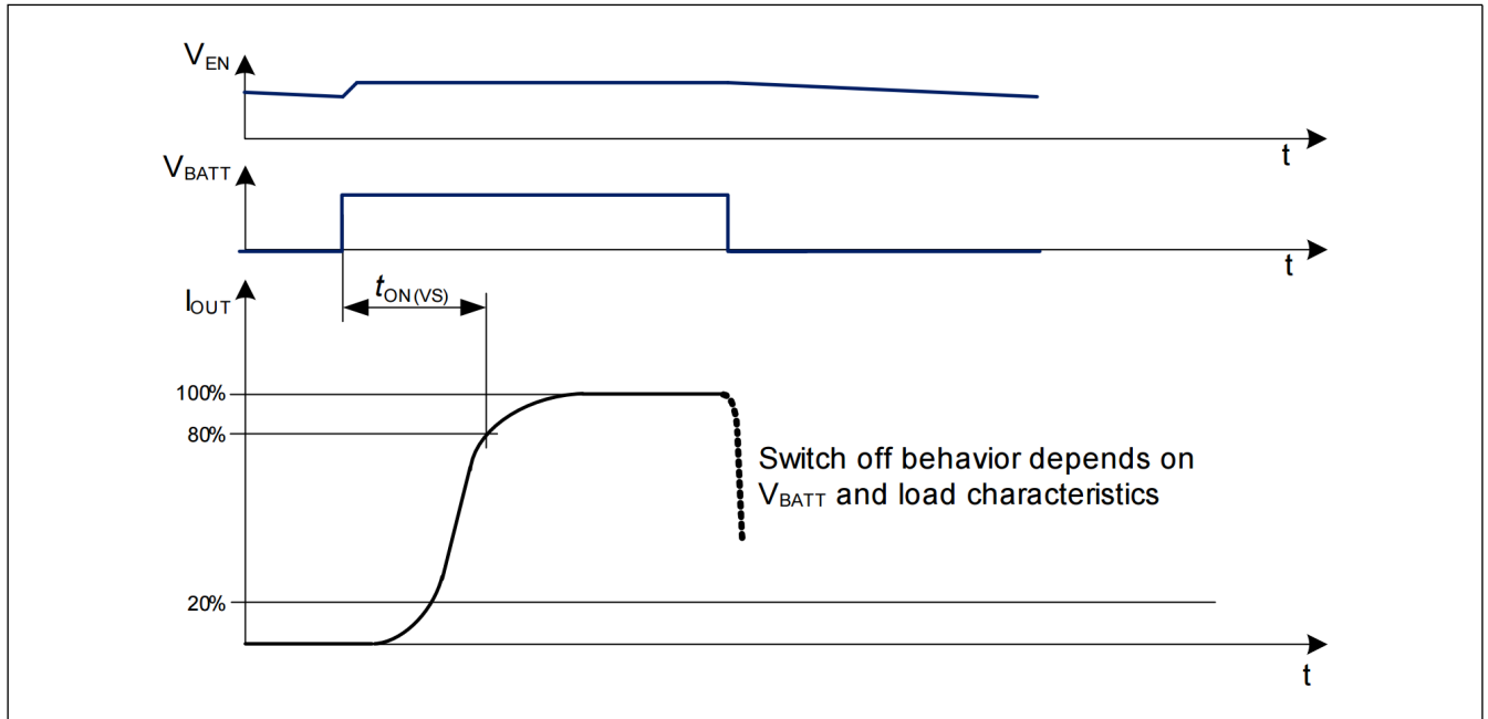
图 6 在 V_{BATT} 上施加快速PWM信号时的典型波形
