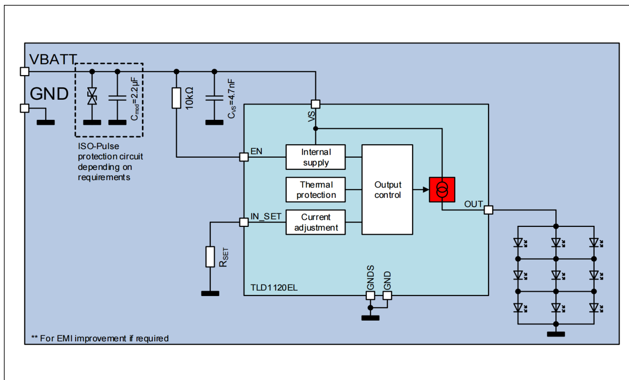
TLD1120EL 应用图
