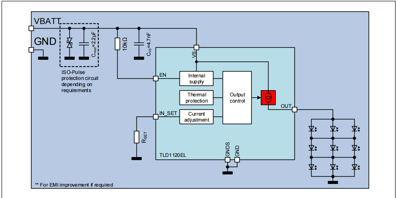
图 12 应用图
