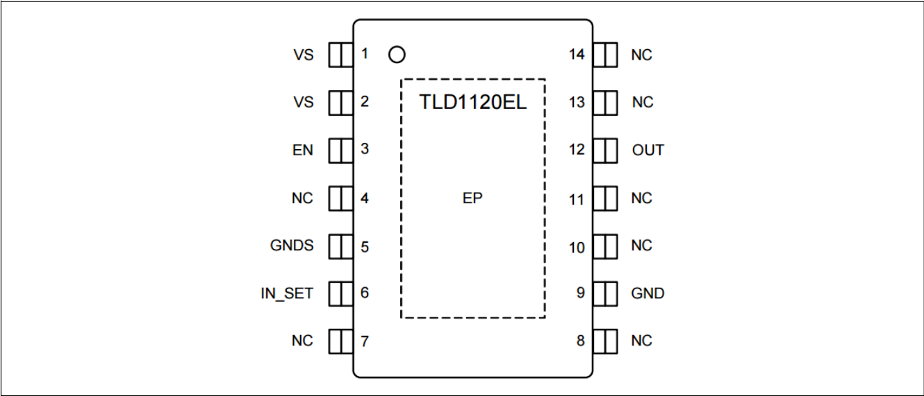
图 2 引脚配置
