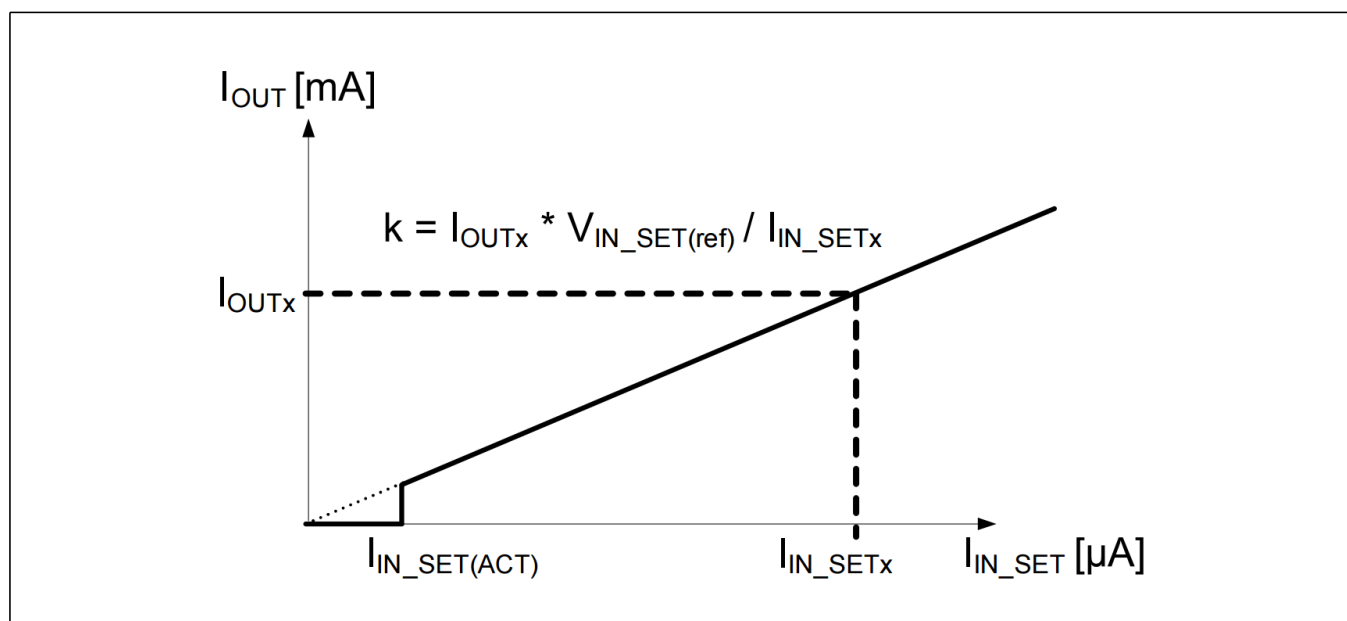
图 10 I_{OUT} 与 I_{INSET}
