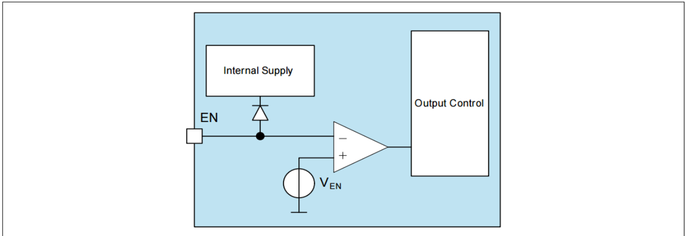
图 3 EN 引脚框图
