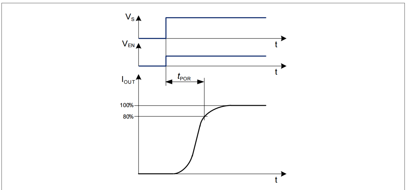
图 4 上电复位
