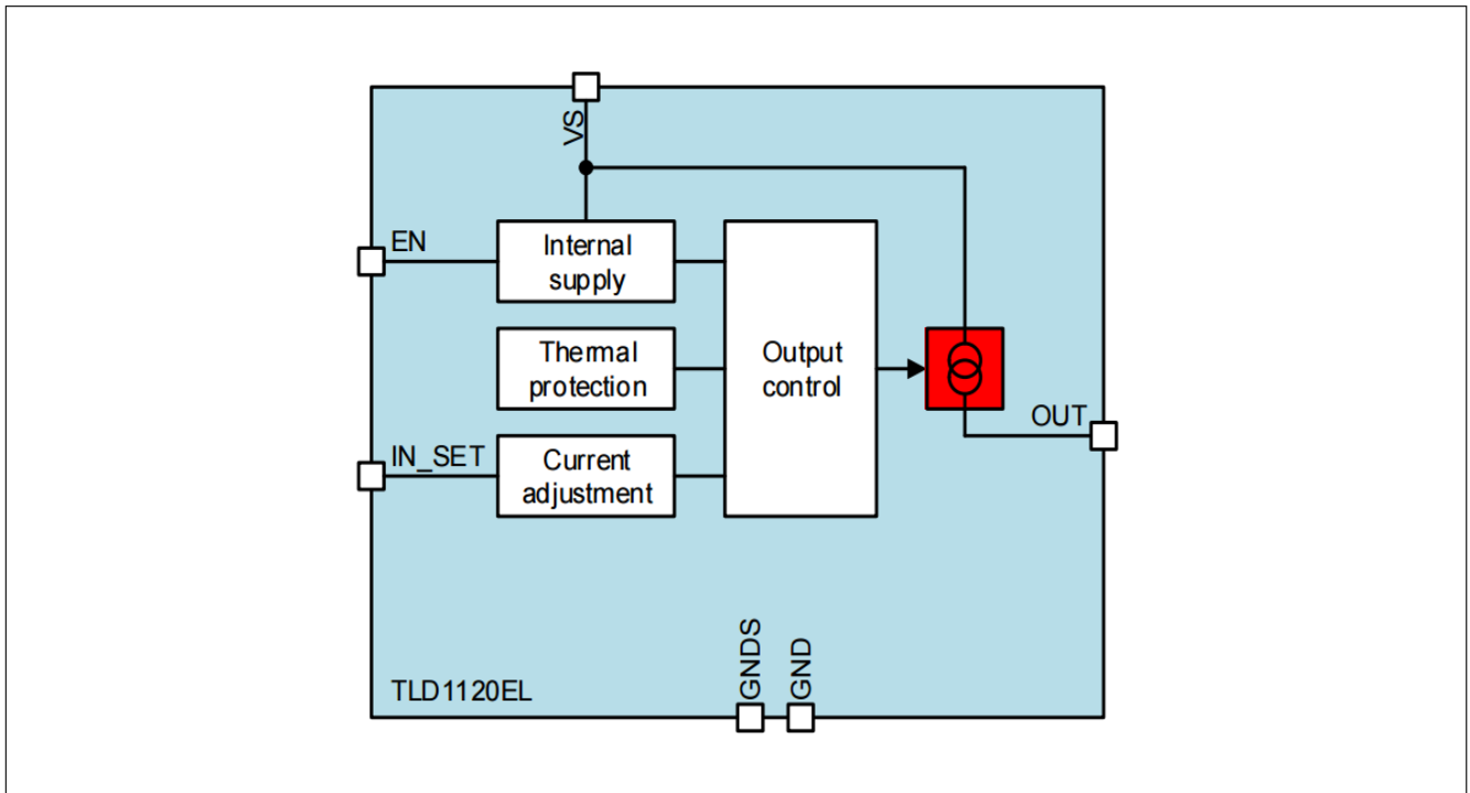
图1 基本框图
