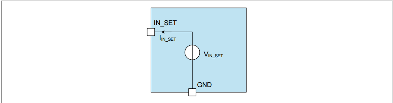
图 7 IN_SET 引脚框图
