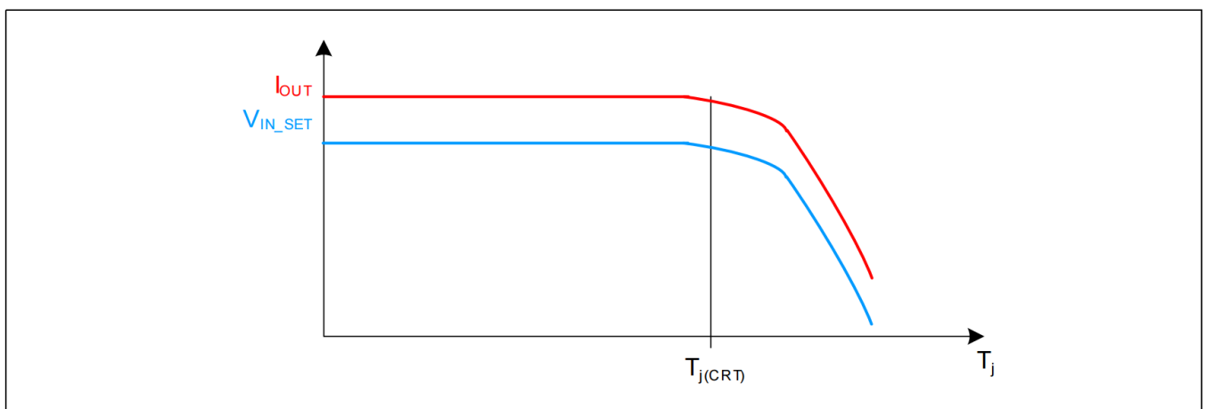
图 11 高温下输出电流减少
