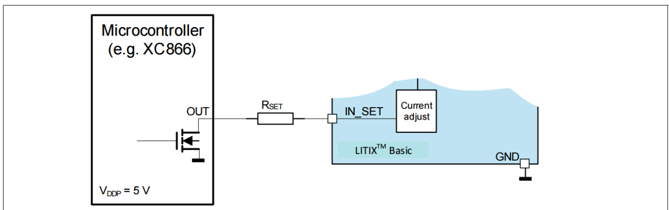
图 8 IN_SET 接口与 \mu C 连接的原理图
