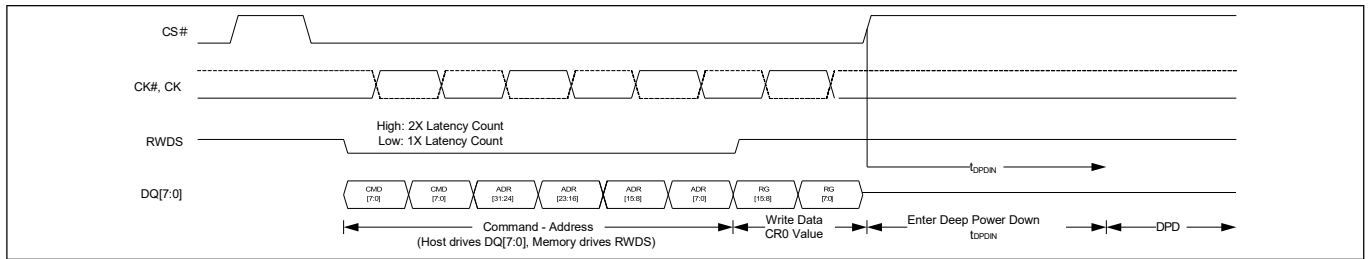
图 17 进入 DPD 传输 [49]
