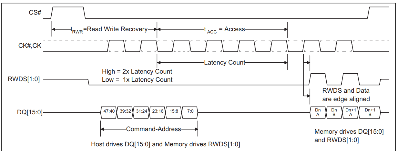
图 1 读取传输，单次初始延迟计数
