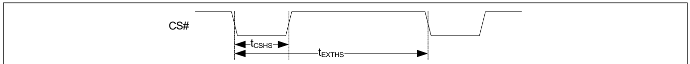
图 16 退出 HS 传输
