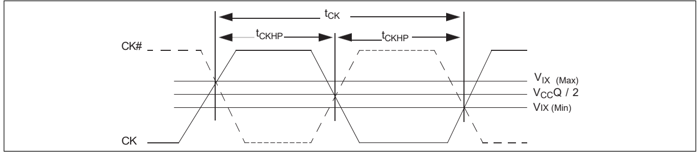
图 28 时钟特性
