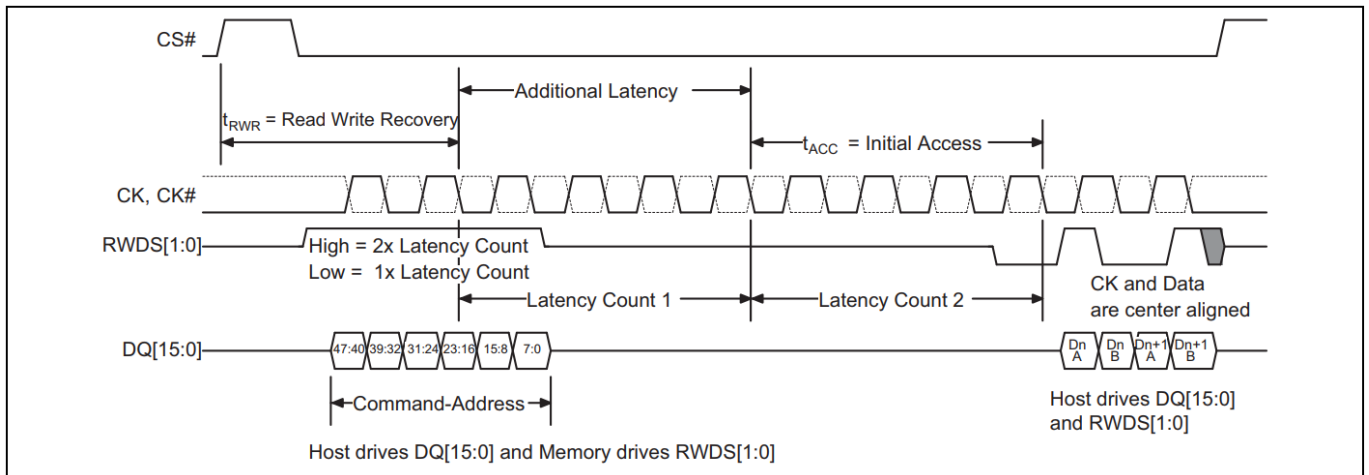
图 11 具有额外初始延迟的写入传输 [33- 36]
