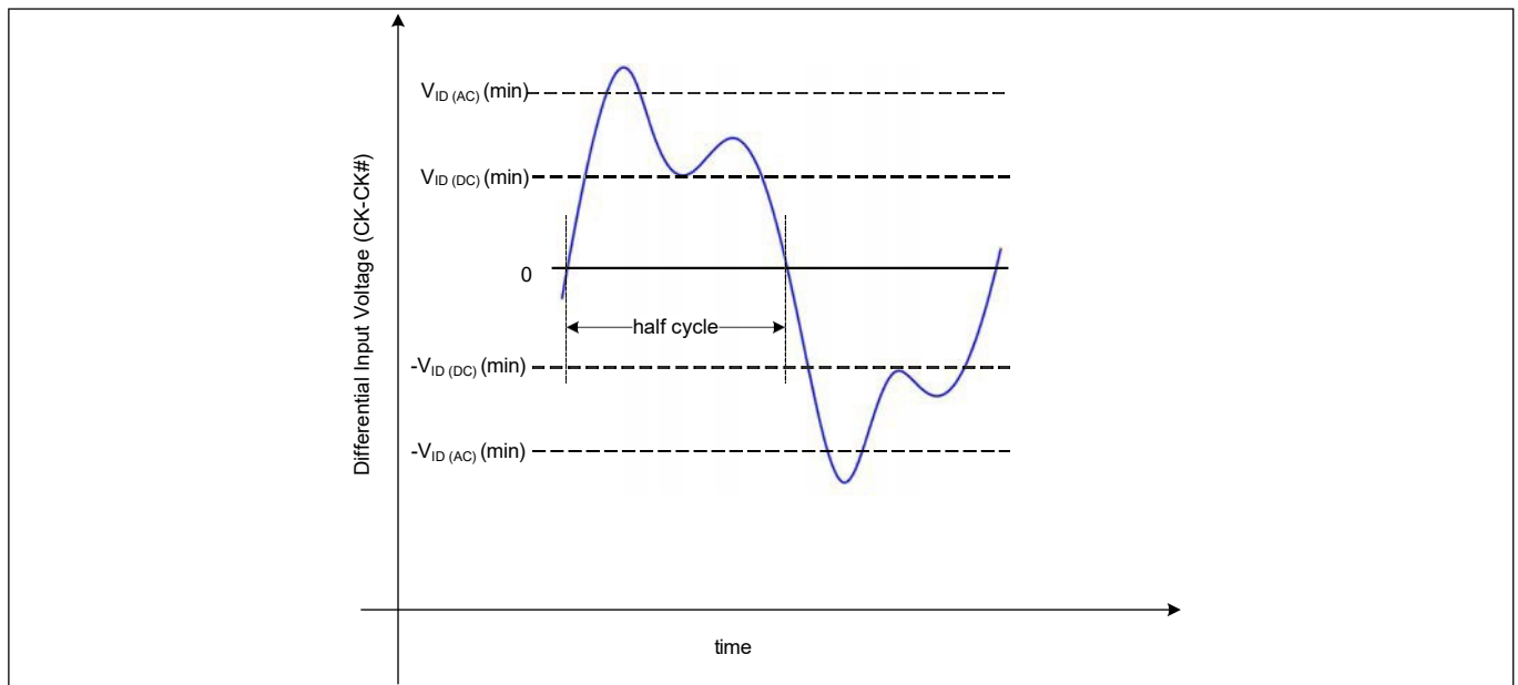
图 29 差分时钟 (CK/CK#) 输入摆幅
