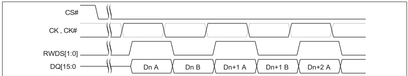
图 7 读取传输期间的数据放置 [12-16]
