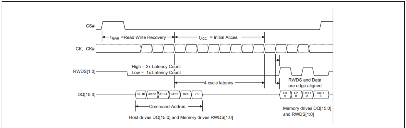
图 10 读取传输, 无需额外的初始延迟 [31 - 32]
