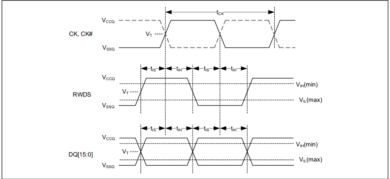
图 34 DDR 输入参考电平
