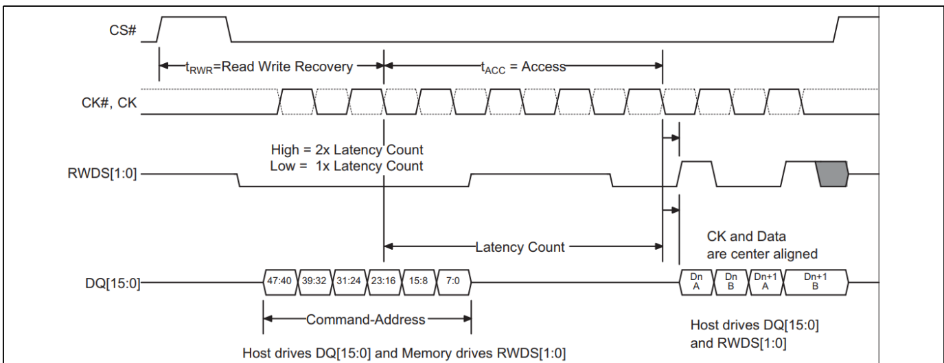
图 12 写入传输, 无额外初始延迟 [37 - 40]
