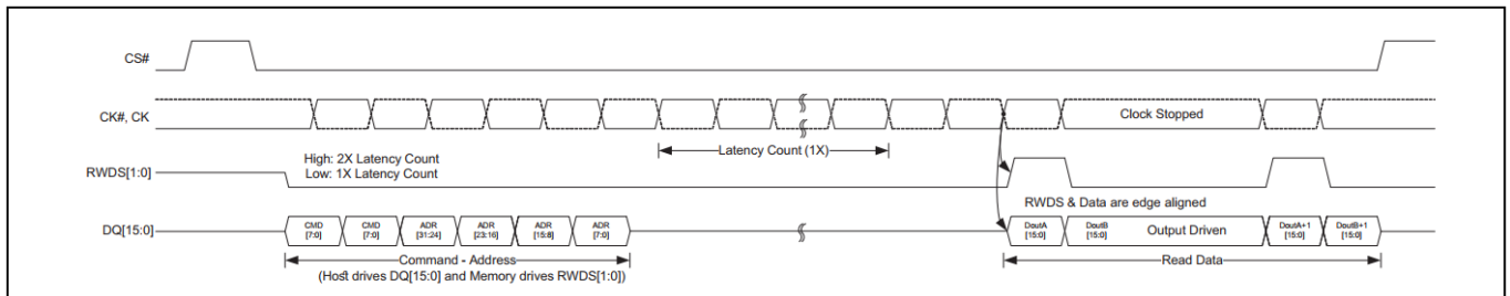
图 14 读取传输期间的有效时钟停止 (DDR) [47,48]
