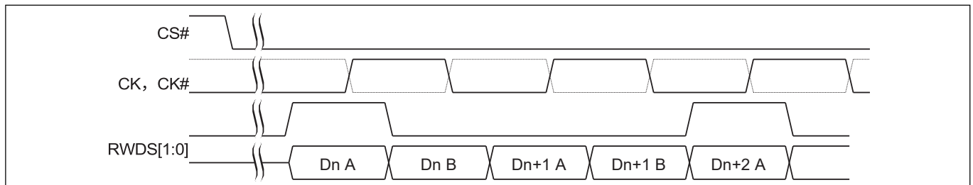
图 8 写入传输期间的数据放置 [12-20]
