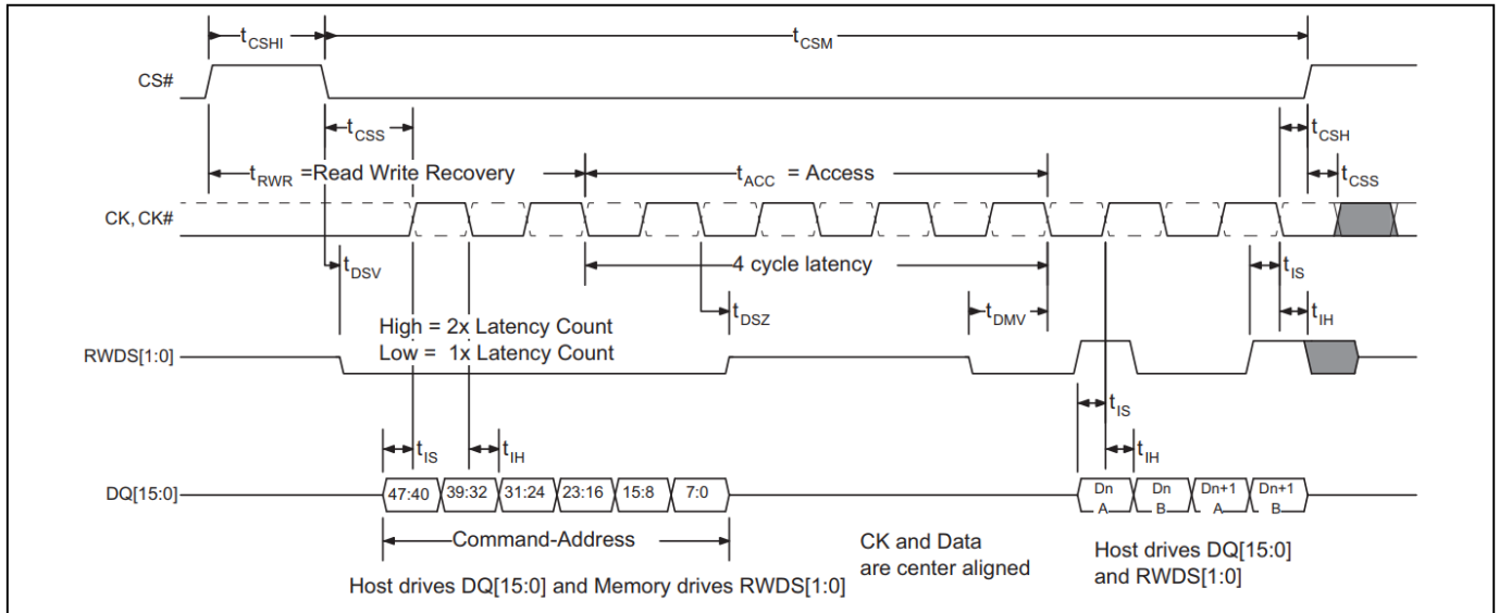
图 33 写入时序图 – 无额外延迟
