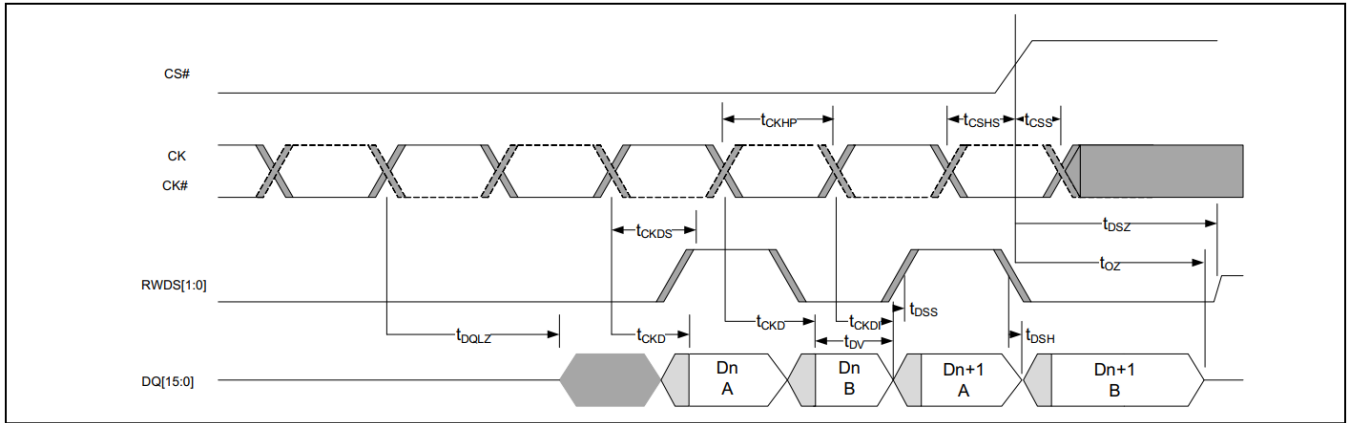
图 32 数据有效时序 [74-76]
