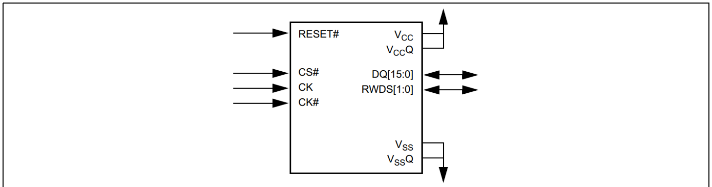
图 5 HYPERRAM™接口 [1]
