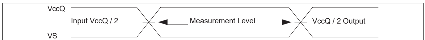
图 27 输入波形和测量电平 [66]
