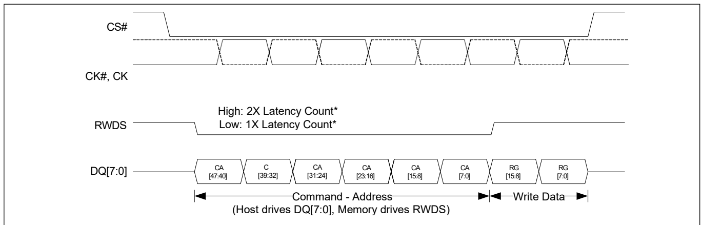
图 13 寄存器写入操作 [41 - 42]
