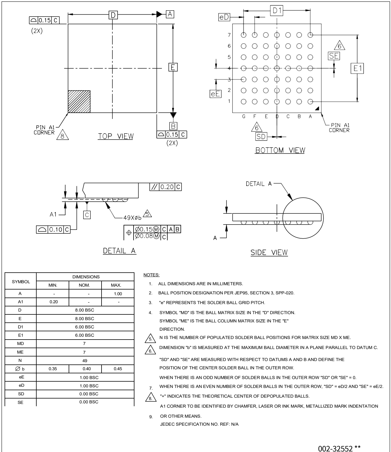
图 37 49 球 FBGA (8.0 × 8.0 × 1.0 mm) 封装外形, 002-32552
