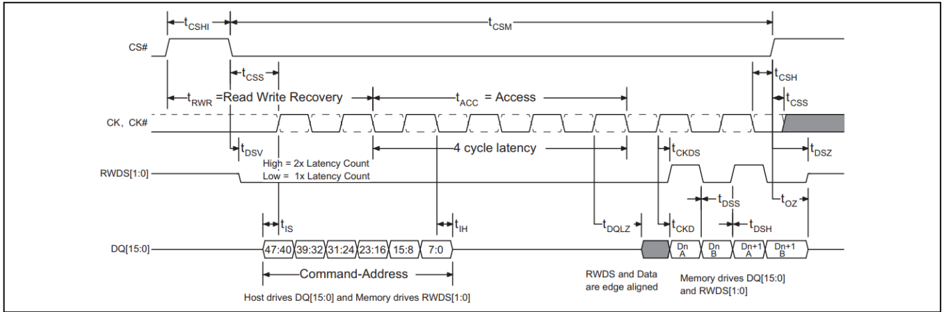
图 30 读取时序图 – 无需额外延迟
