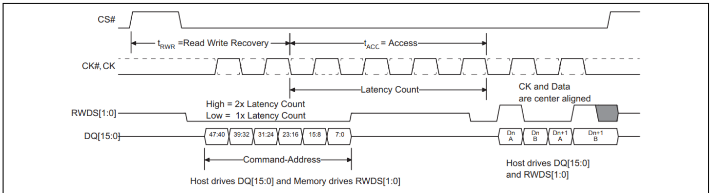
图 3 写入传输，单次初始延迟计数
