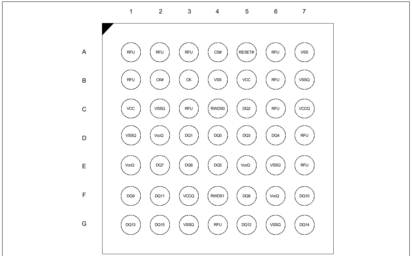
图 36 49 球 FBGA, 8 × 8 mm, 7 × 7 球封装, 俯视图
