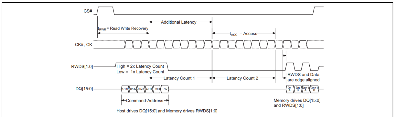
图 9 读取传输具有额外的初始延迟 [21- 30]
