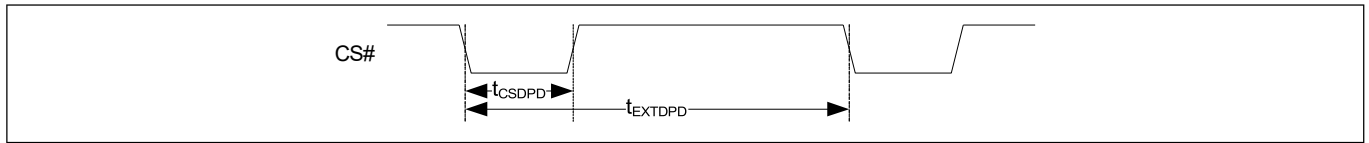
图 18 退出 DPD 传输
