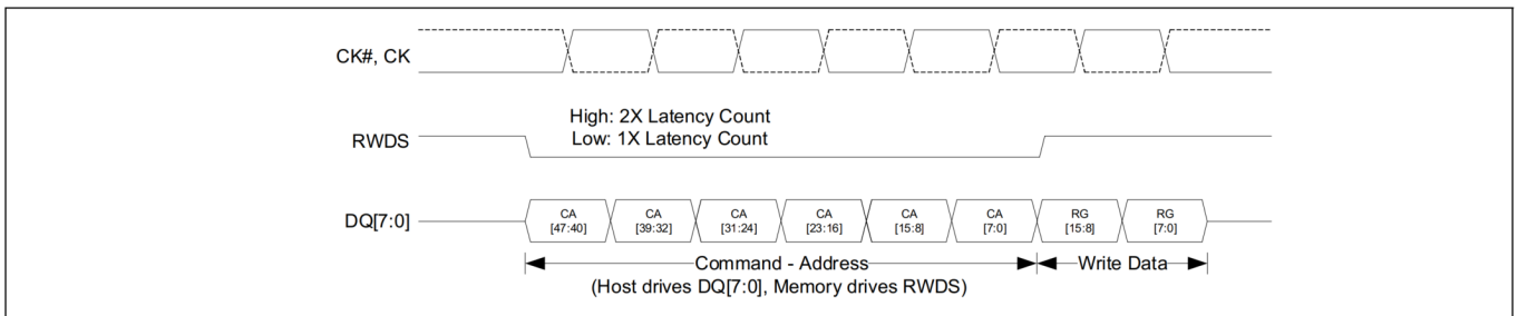
图 13 寄存器写入操作 [38、39]
