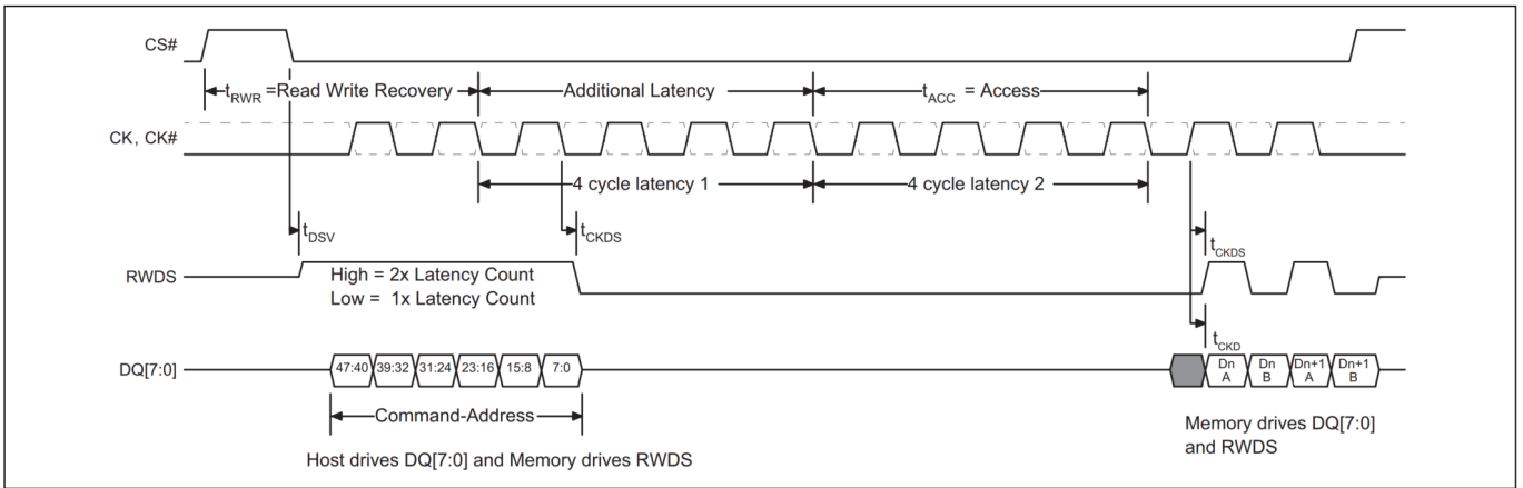
图 31 读取时序图——需要额外的延迟
