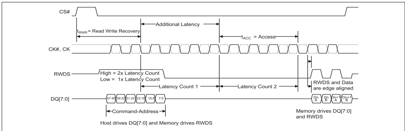
图 9 读取传输具有额外的初始延迟 [20- 28]
