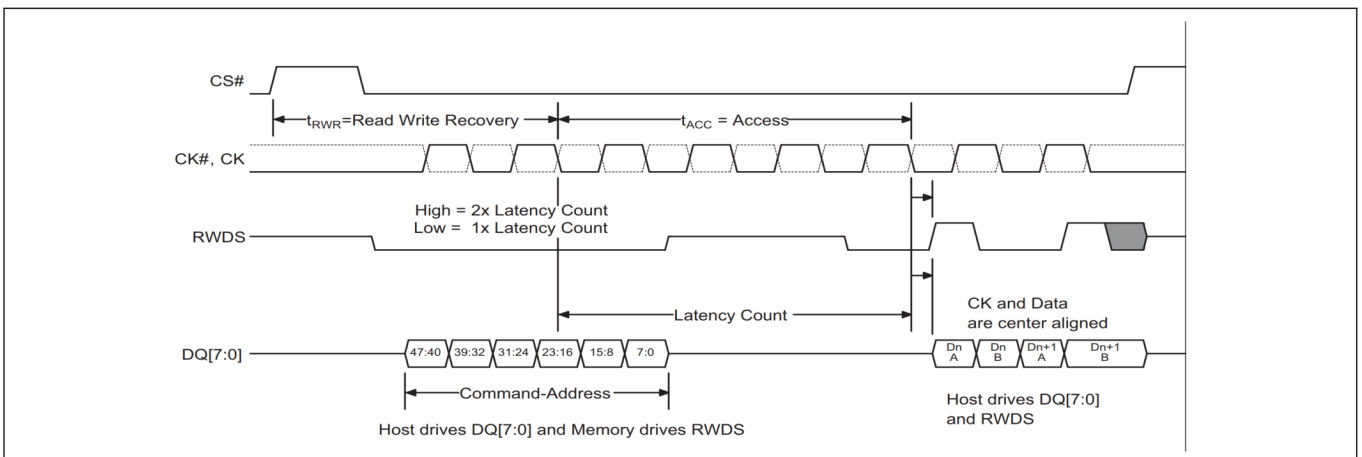
图 12 写入传输，无额外初始延迟 [33-37]
