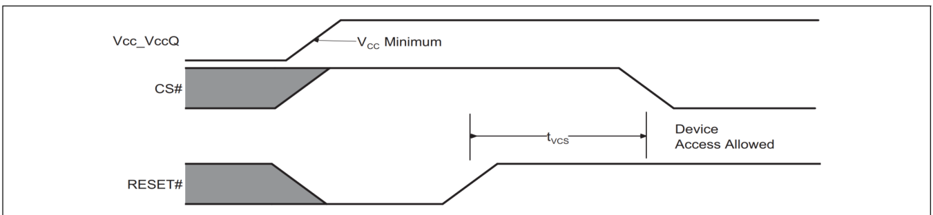
图 22 RESET\# 为低电平时上电
