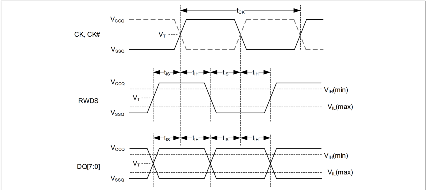
图 34 DDR 输入参考电平
