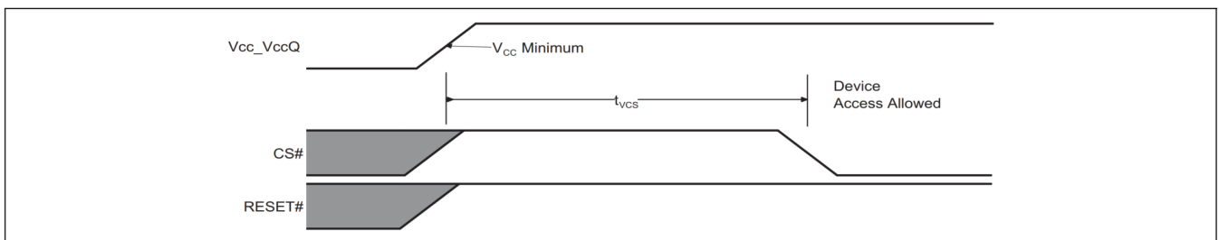
图 21 RESET\# 为高电平时上电
