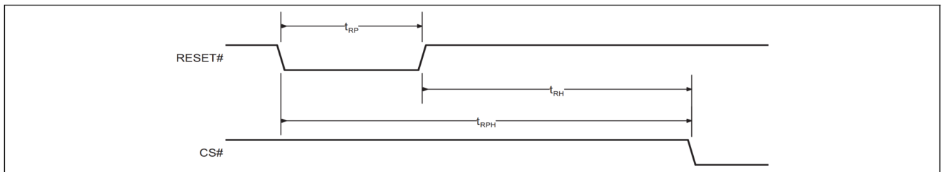
图 24 硬件复位时序图
