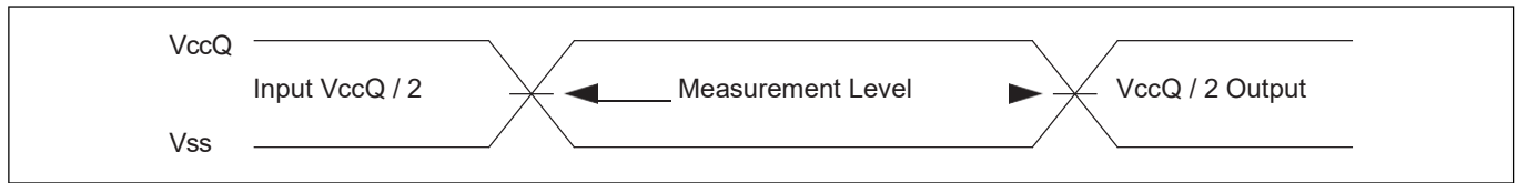
图 27 输入波形和测量电平 [60]
