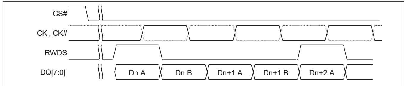
图 8 写入传输期间的数据放置 [16 - 19]
