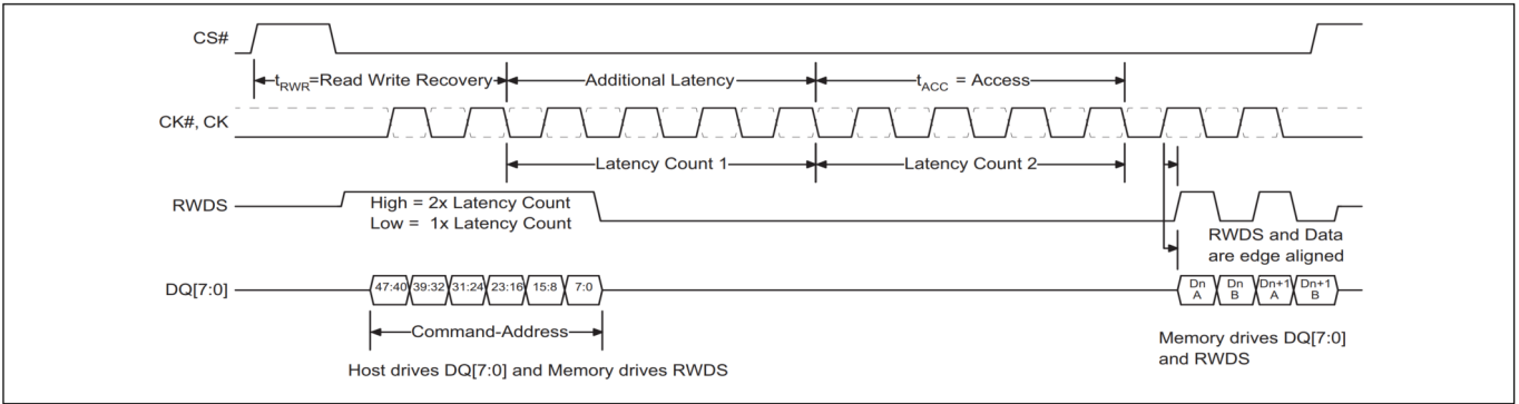
图 2 读取传输，额外延迟计数
