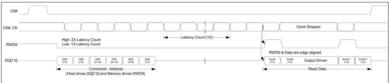
图 14 读取传输期间的有效时钟停止 (DDR) [44]
