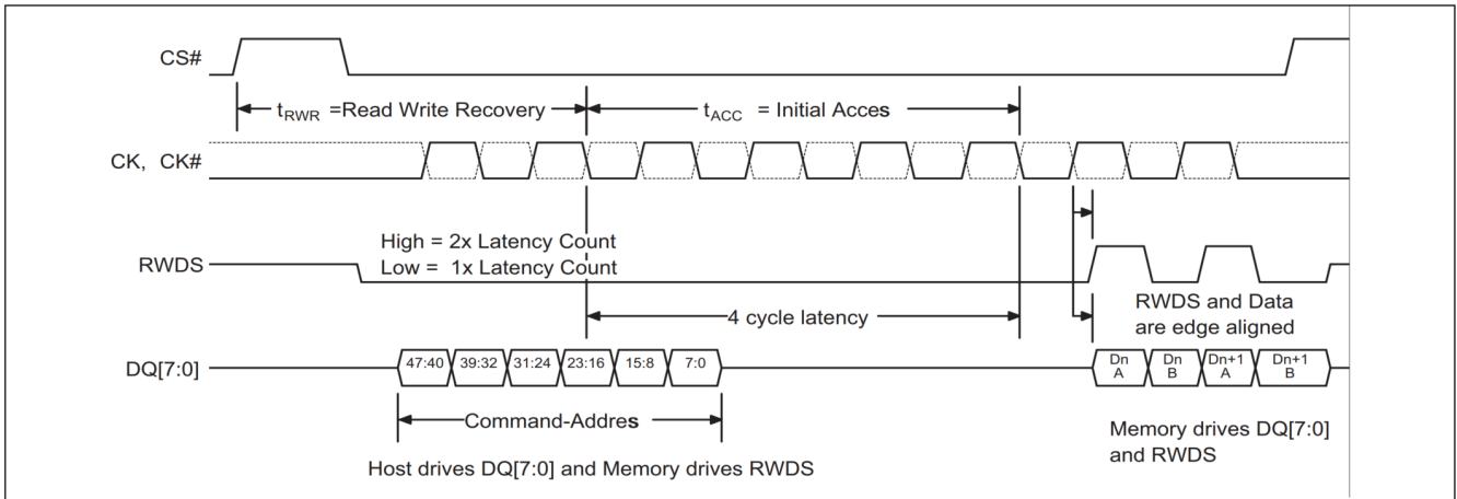
图 10 读取传输，无需额外的初始延迟 [29、30]
