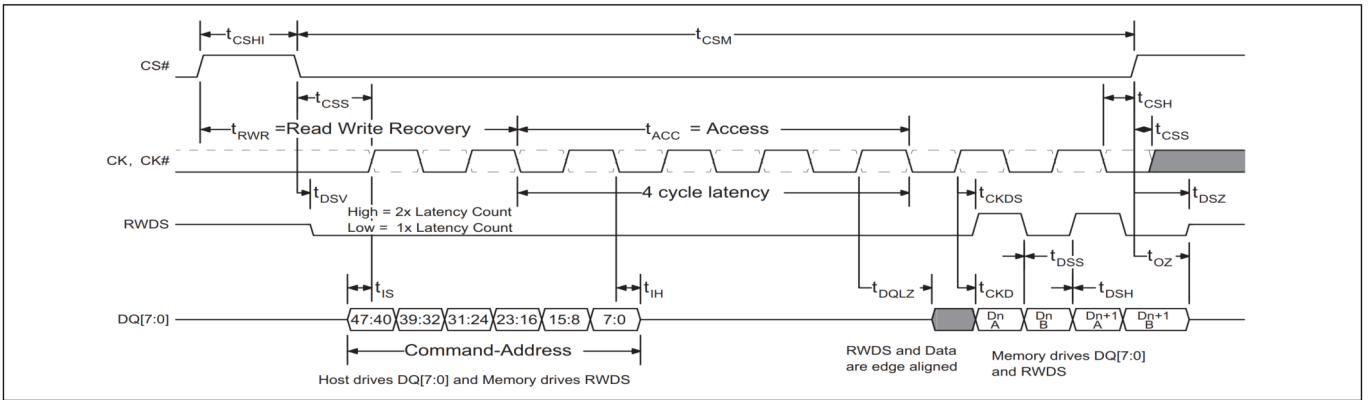
图 30 读取时序图 – 无需额外延迟
