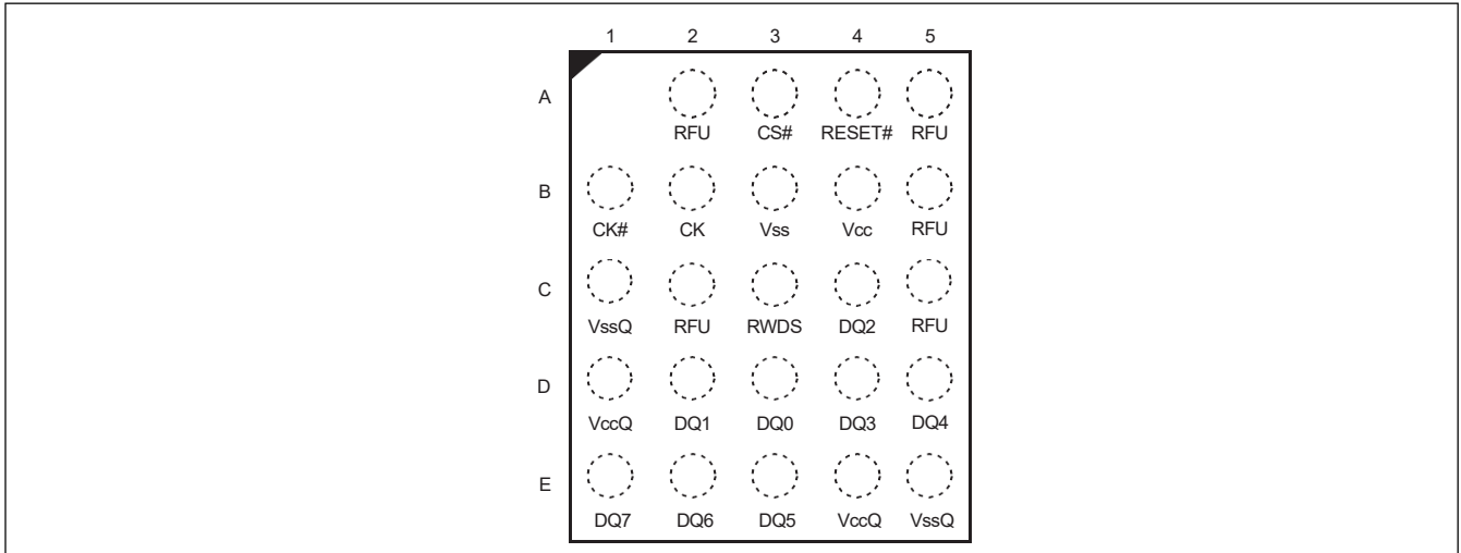
图 36 24 球 FBGA，6 × 8 mm，5 × 5 球封装，俯视图
