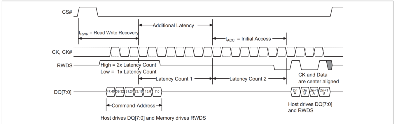
图 11 具有额外初始延迟的写入传输 [31-37]
