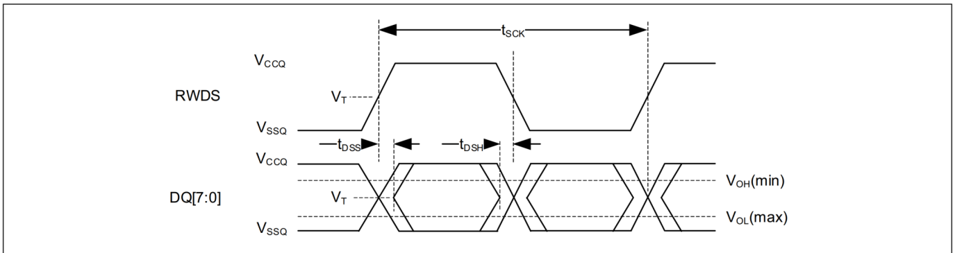
图 35 DDR 输出参考电平
