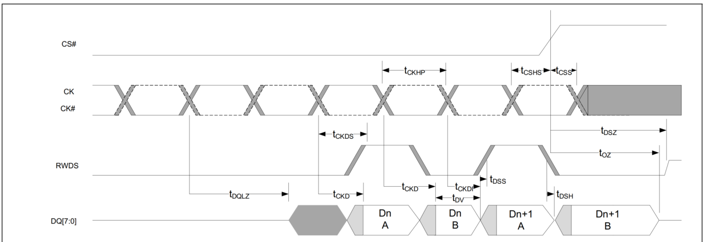
图 32 数据有效过程 [68 - 70]
