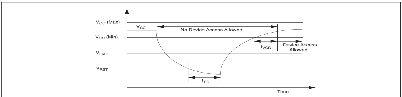
图23 掉电或电压下降
