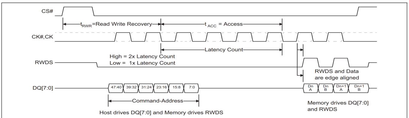
图 1 读取输入，单次初始延迟计数
