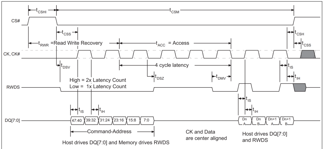
图 33 写入时序图 – 无额外延迟
