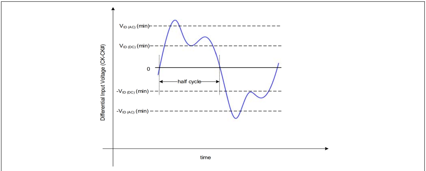
图 29 差分时钟 (CK/CK#) 输入摆幅
