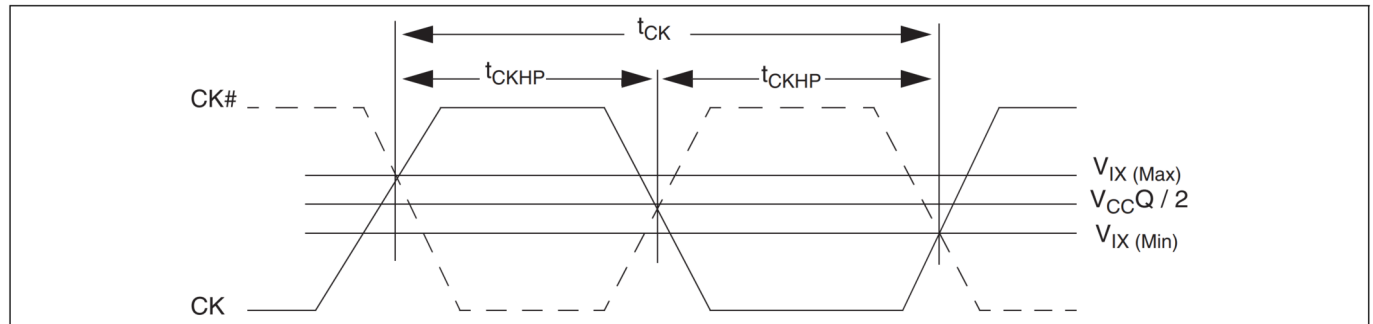
图 28 时钟特性
