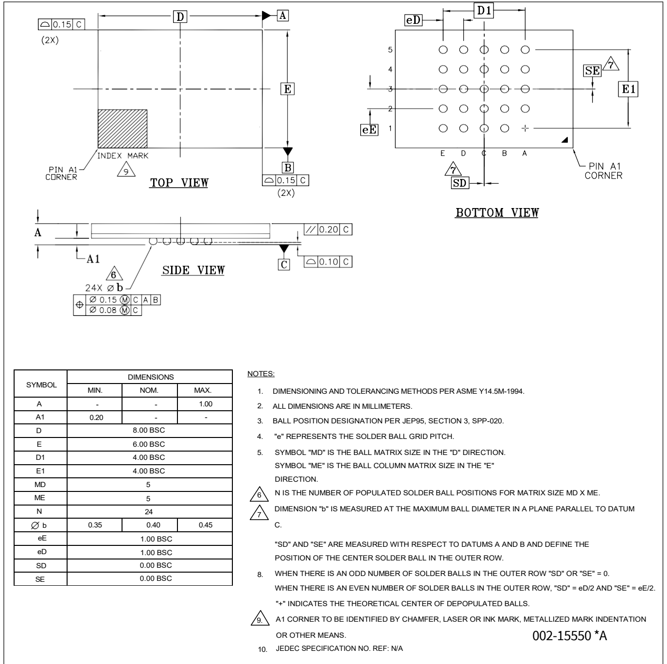
图 37 强化球栅阵列 24 球 6 × 8 × 1.0 mm (VAA024)
