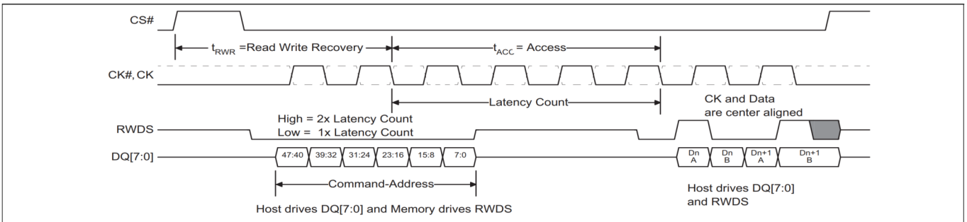
图 3 写入传输，单次初始延迟计数
