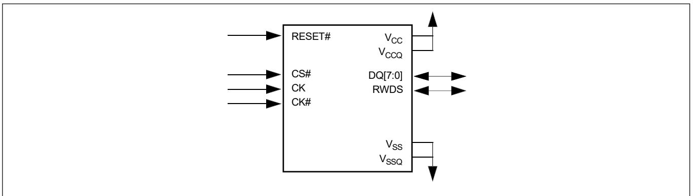
图 5 HYPERRAM™接口 [1]
