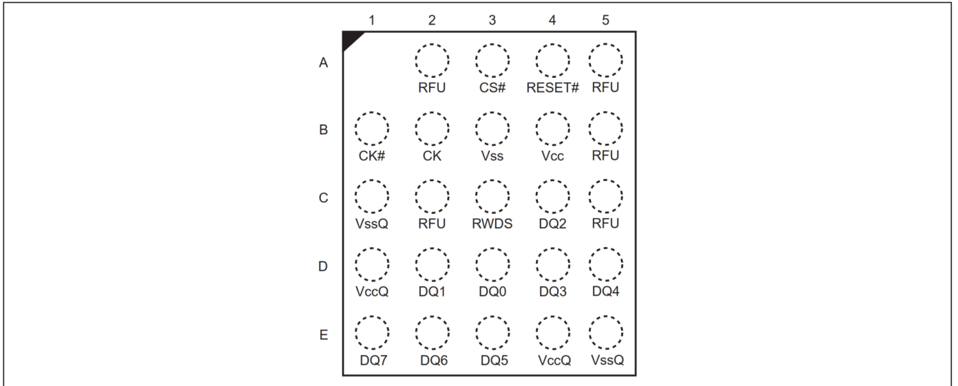
图 40 24 球 FBGA, 6 × 8 mm, 5 × 5 球封装, 俯视图
