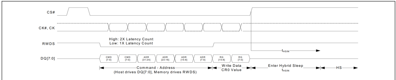
图 23 进入 HS 传输
