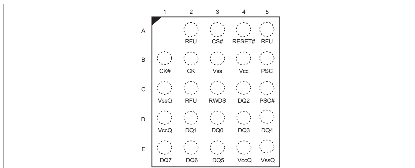
图 43 24 球 FBGA, 5 × 5 球封装, 俯视图
