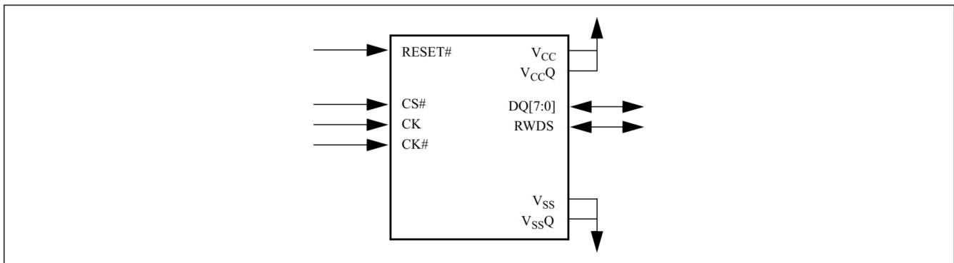
图 7 xSPI (八线) HYPERRAM™接口 [8]
