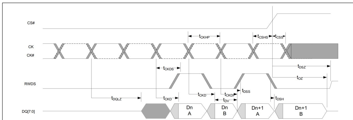
图 38 数据有效时序 [58, 59, 60]
