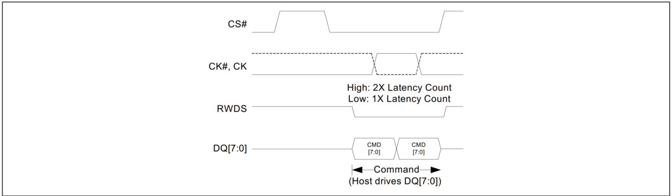
图 1 xSPI (八线) 仅指令传输 (DDR)
