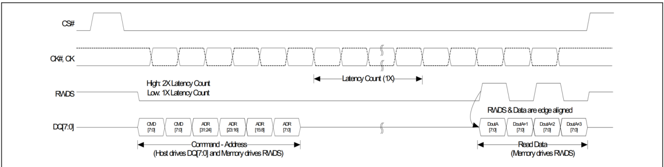
图 5 xSPI (八线) 读取, 1X 延迟传输 (DDR) (所有读取) [6]
