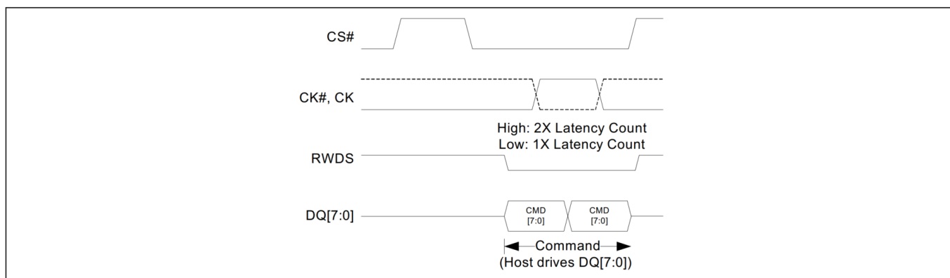
图 8 复位使能传输 (DDR)
