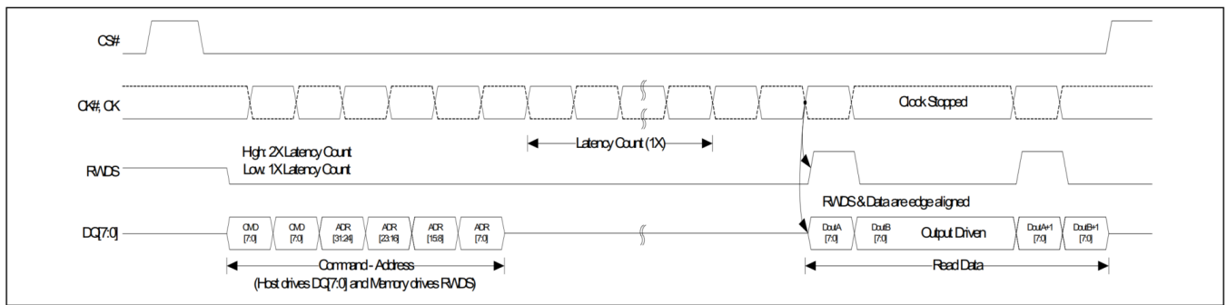
图 22 读取传输期间的有效时钟停止 (DDR) [30]
