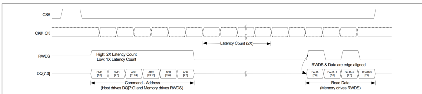
图 14 具有 2X 延迟传输的读取 (DDR) [19]
