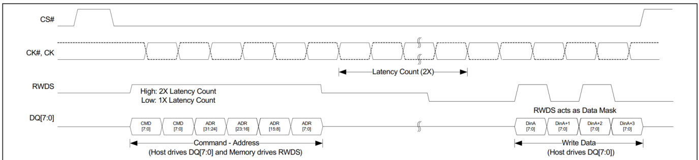
图 16 具有 2X 延迟传输的写入 (DDR) [22, 23]
