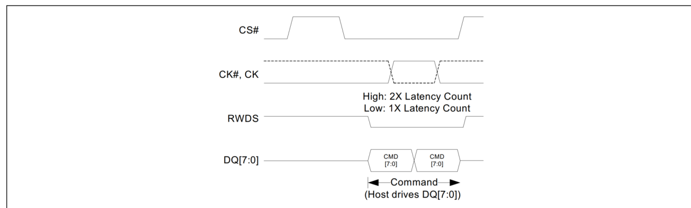
图 12 深度掉电传输 (DDR)
