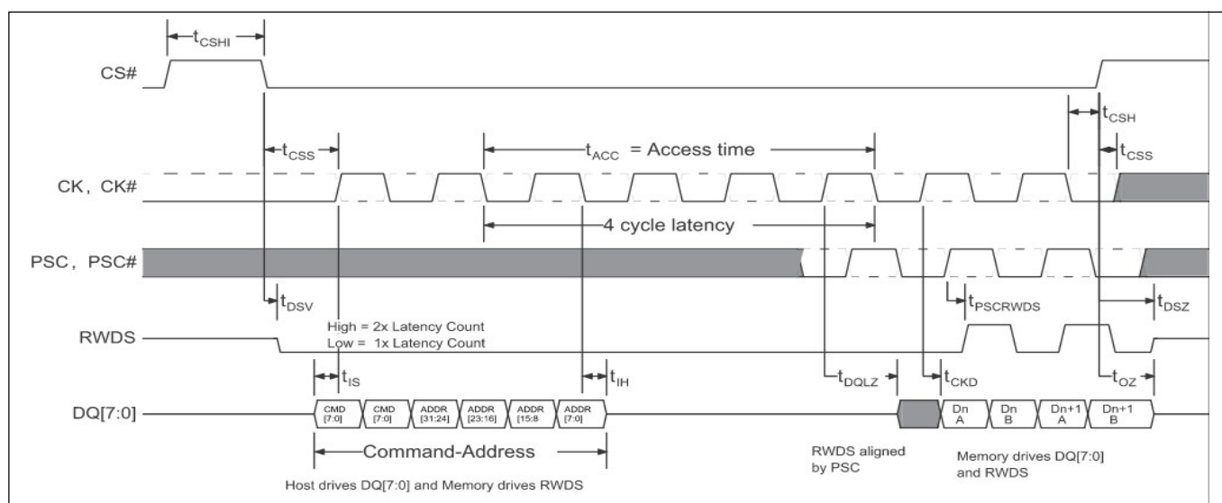
图 44 HYPERRAM™ 存储器 DCARS 时序图 [61, 62, 63]
