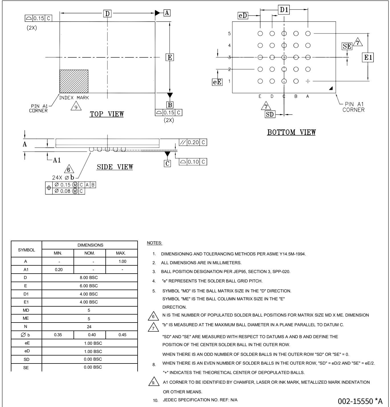
图 41 强化球栅阵列 24 球 6 · 8 · 1.0 mm (VAA024)
