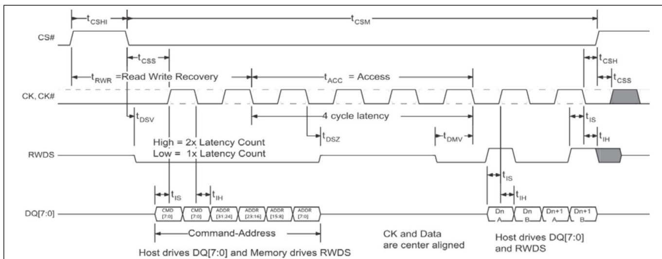
图 39 写入时序图 – 无额外延迟
