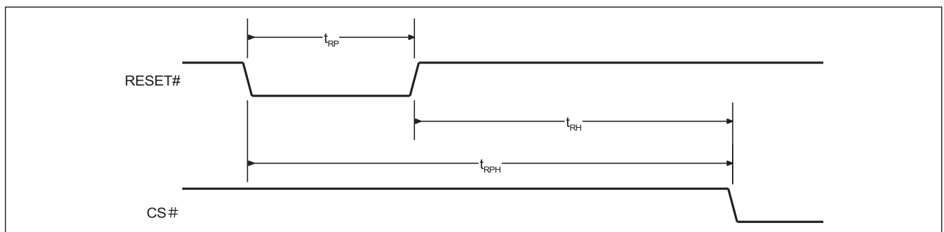
图 32 硬件复位时序图
