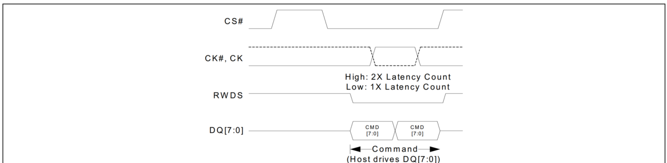
图 17 写入使能传输 (DDR)
