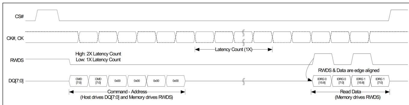
图 10 具有 1X 延迟传输的读取 ID (DDR) [16]
