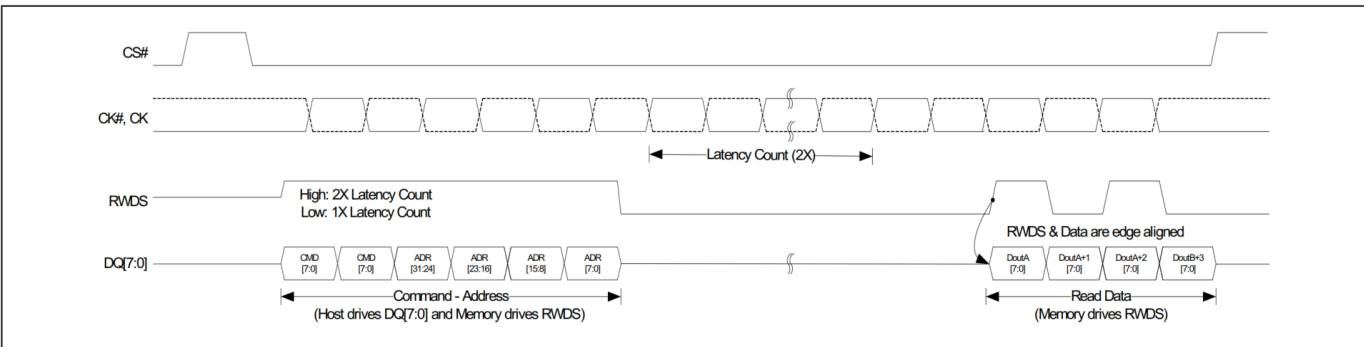
图 6 xSPI (八线) 读取, 2X 延迟传输 (DDR) (所有读取) [7]
