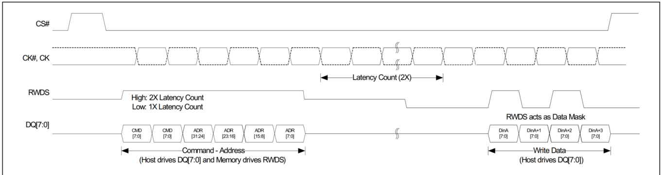
图 4 xSPI (八线) 写入, 具有 2X 延迟传输(DDR) (内存阵列写入) [4,5]
