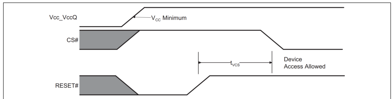
图 30 RESET# 为低电平时上电
