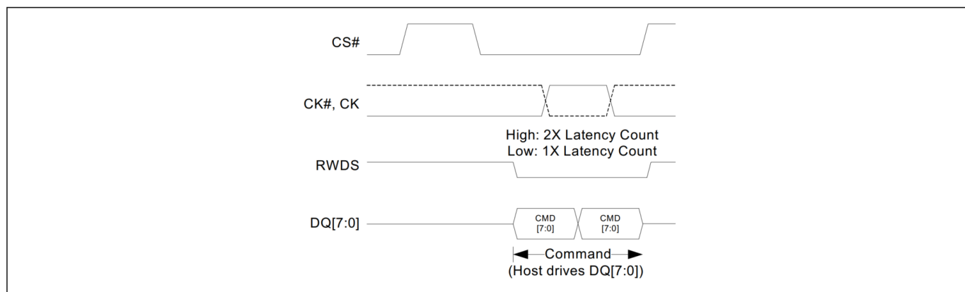
图 9 复位传输 (DDR)
