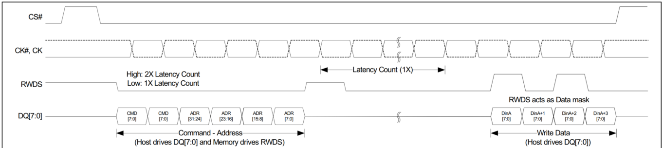
图 15 1X 延迟传输的写入 (DDR) [22, 23]
