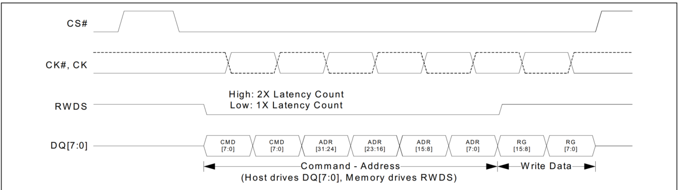
图 2 xSPI (八线) 无延迟写入传输 (DDR) (寄存器写入) [1]
