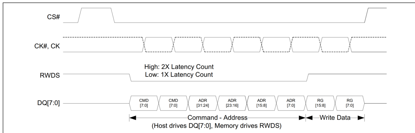
图 21 xSPI (八线) 无延迟写入传输 (DDR) (寄存器写入) [26, 27]
