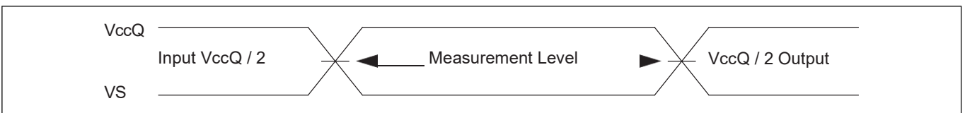
图34 输入波形和测量电平 [48]
