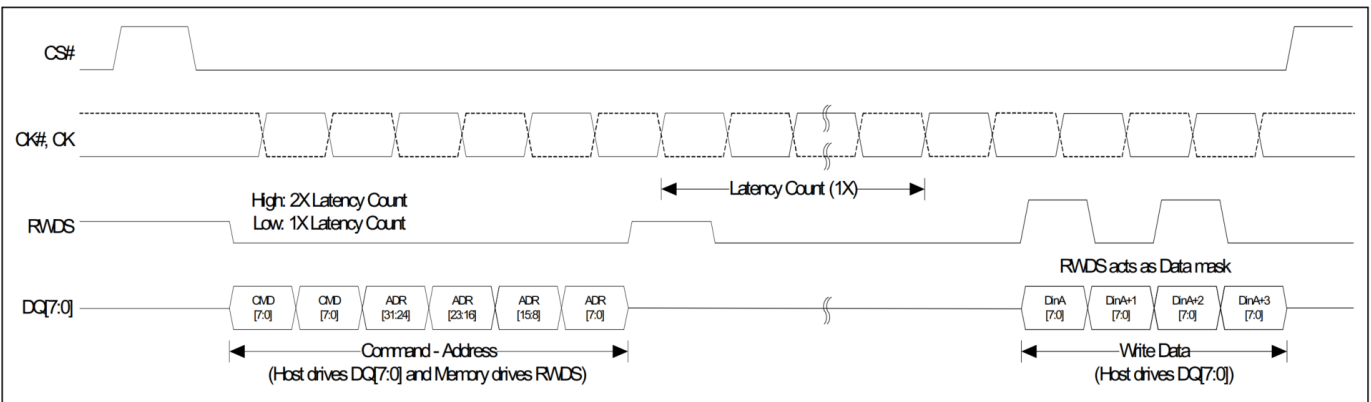
图 3 xSPI (八线) 写入, 具有 1X 延迟传输(DDR) (存储器阵列写入) [2, 3]
