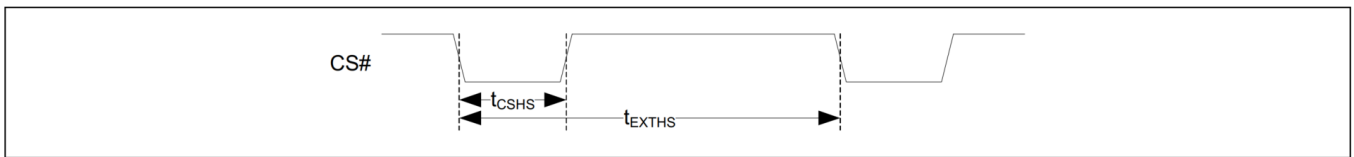
图 24 退出 HS 传输
