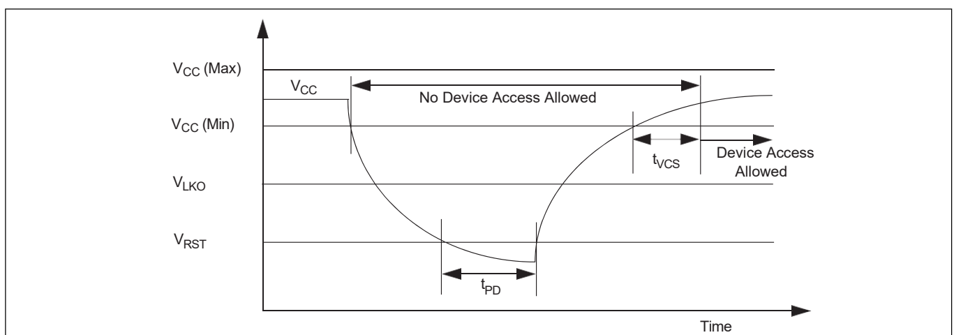
图31 掉电或电压下降
