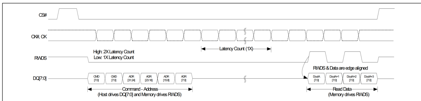
图 13 具有 1X 延迟传输的读取 (DDR) [18]
