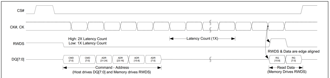
图 19 以 1X 延迟传输读取任意寄存器 (DDR) [24]
