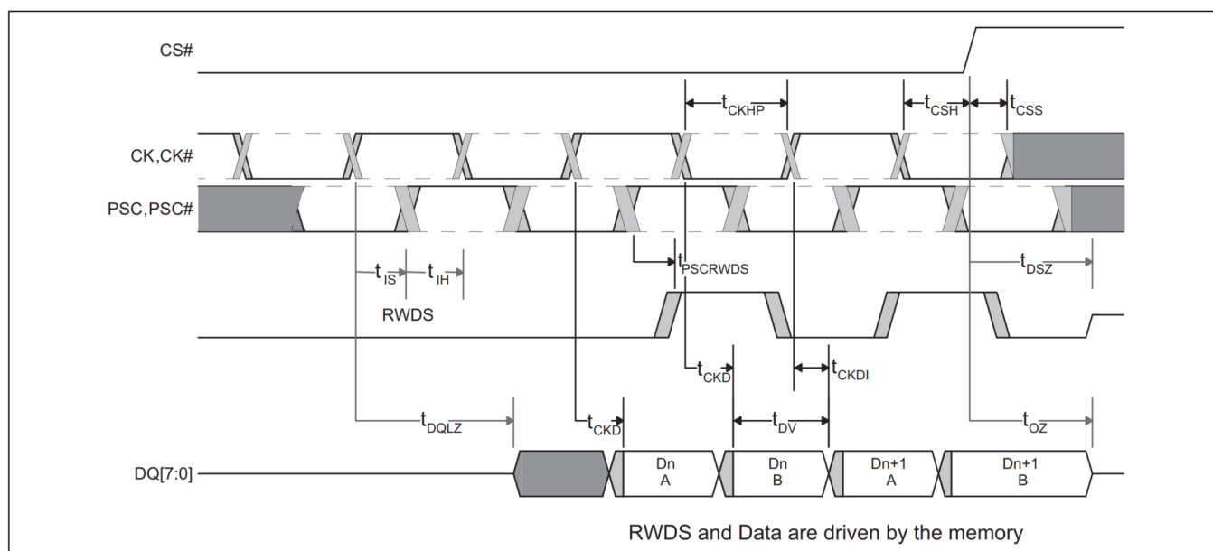
图 45 DCARS 数据有效时序 [64,65,66, 67]
