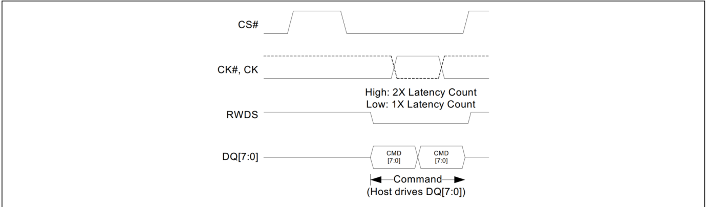
图 18 写入禁止传输 (DDR)
