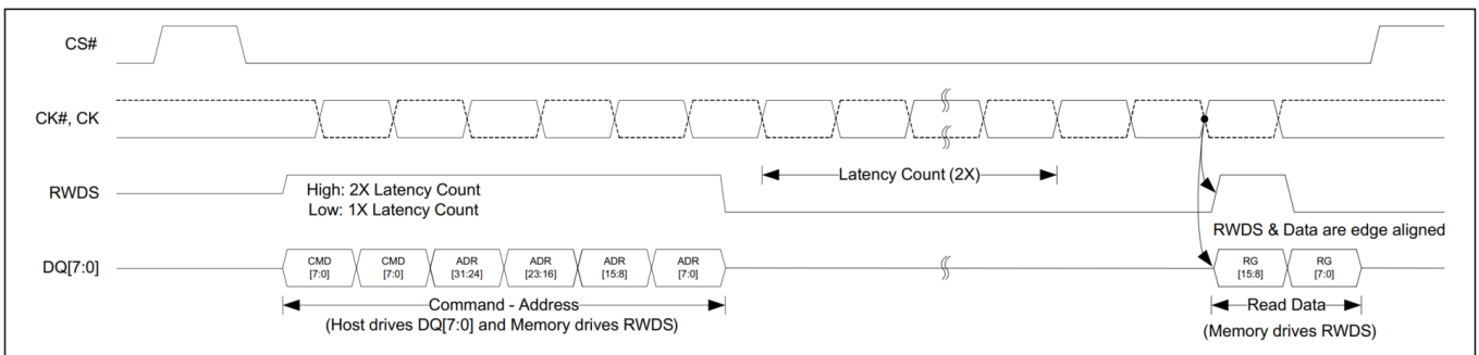
图 20 以 2X 延迟传输读取任意寄存器 (DDR) [25]
