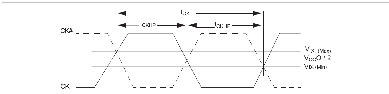
图 35 时钟特性
