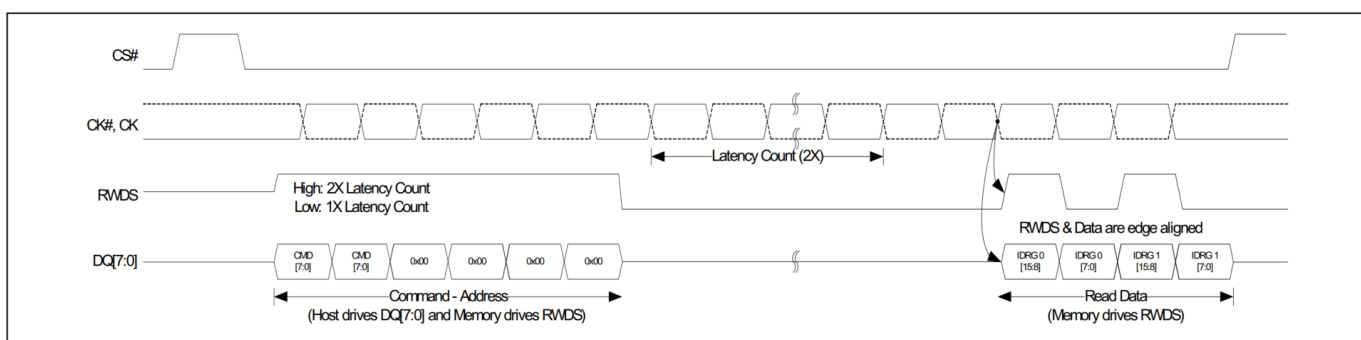
图 11 具有 2X 延迟传输的读取 ID (DDR) [17]
