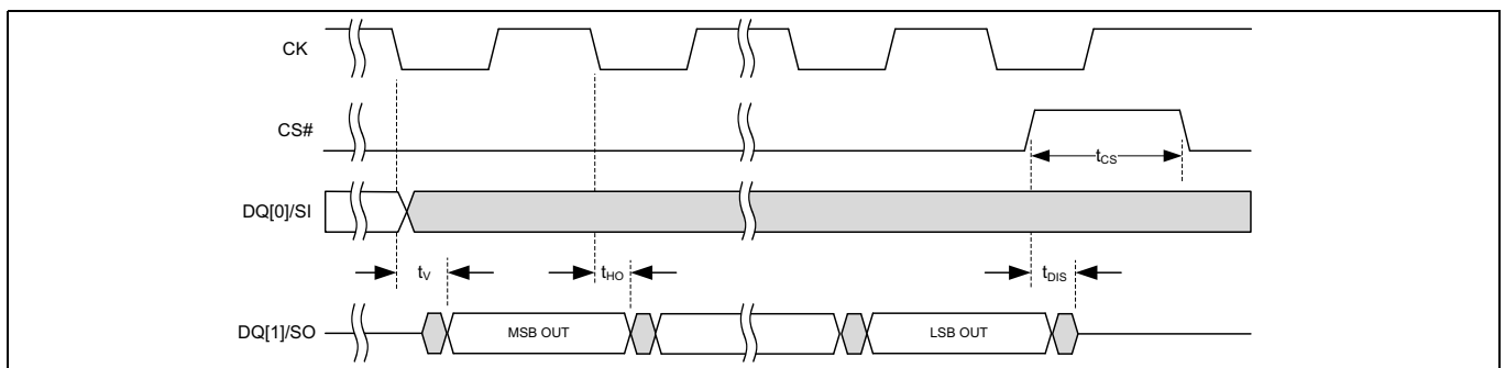
Figure 62 SPI 出力タイミング
