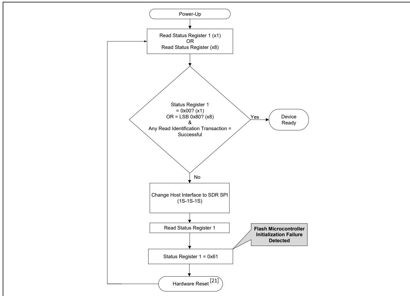
Figure 32 マイクロコントローラー初期化失敗検出用のホスト ポーリング シーケンス
