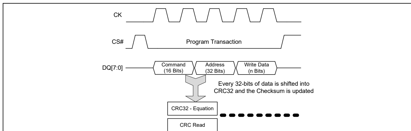
Figure 24 CRC によるプログラム保護
