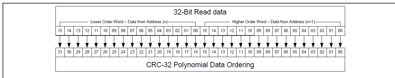
Figure 25 CRC-32 データ順序
