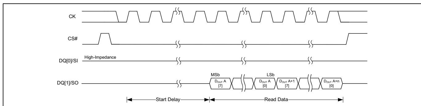
Figure 13 出力データ シーケンスのある SPI トランザクション (オートブート)
