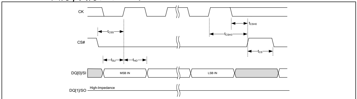
Figure 61 SPI 入力タイミング
