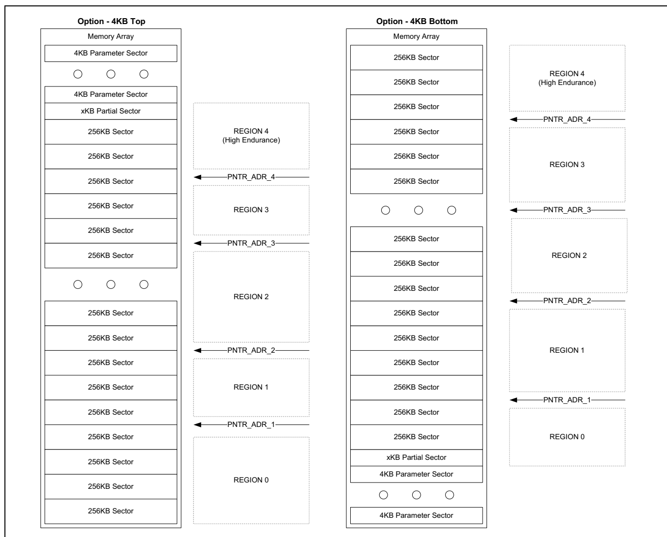
Figure 20 インフィニオン Endurance Flex アーキテクチャ概要
