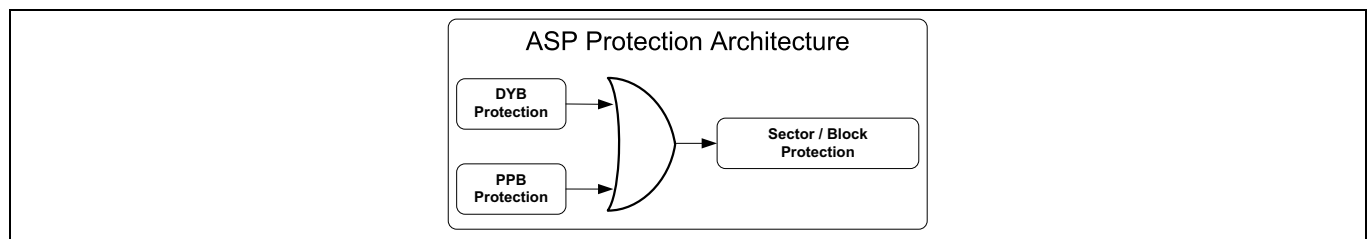
Figure 28 DVB と PPB の保護制御
