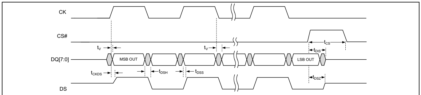
Figure 64 HYPERBUS™ DDR 出力タイミング
