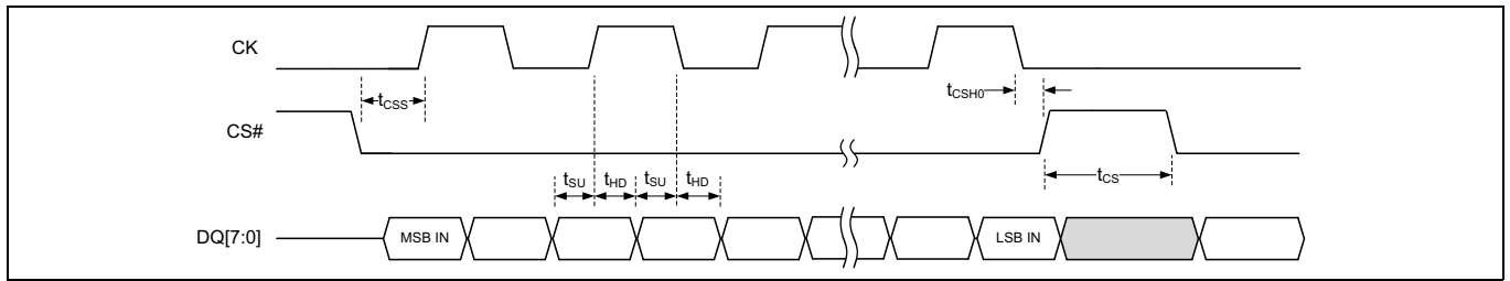
Figure 63 HYPERBUS™ DDR 入力タイミング
