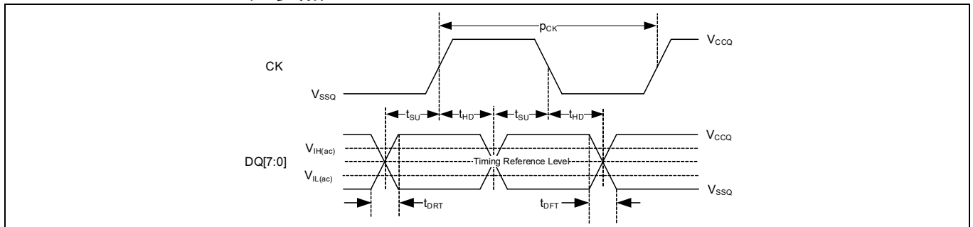
Figure 56 入力タイミング参照レベル
