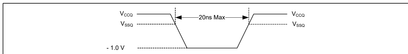
Figure 52 最大負オーバーシュート波形
