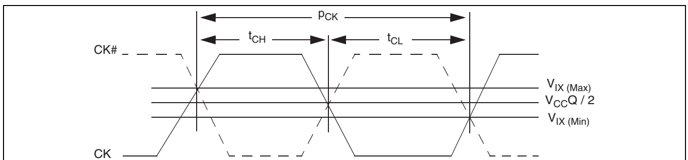
Figure 60 差動クロック タイミング
