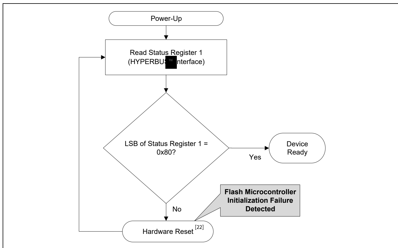
Figure 33 マイクロコントローラー初期化失敗検出用のホスト ポーリング シーケンス (x8 ブート オプション)
