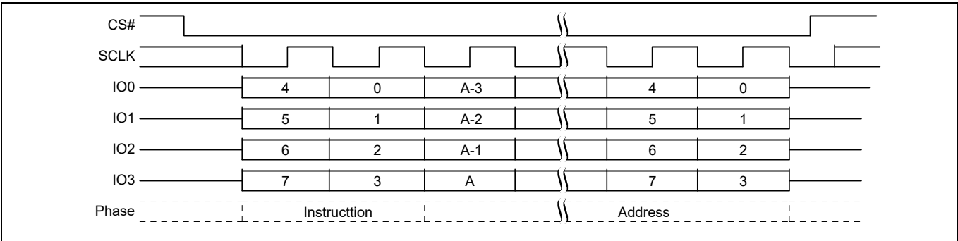
图 98 QPI 模式下的 IBL 命令序列 [50、51]
