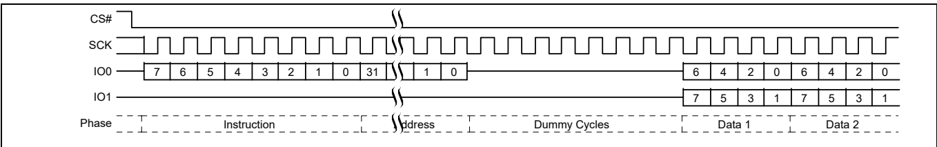
图 17 双线输出读命令
