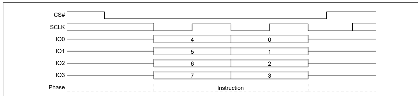
图 122 QPI 模式下的软件复位 / 模式位命令序列
