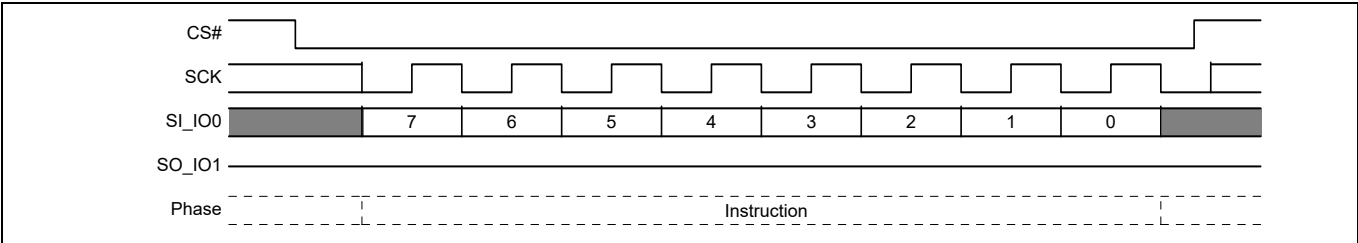
图 57 退出 4 字节地址模式 (4BEX E9h) 命令序列
