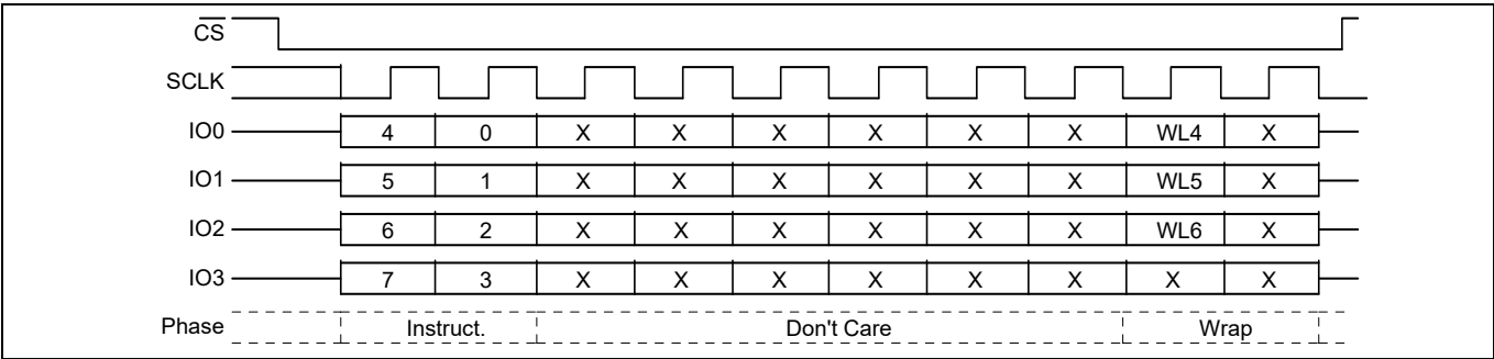
图 62 QPI 模式下的设置突发长度命令序列
