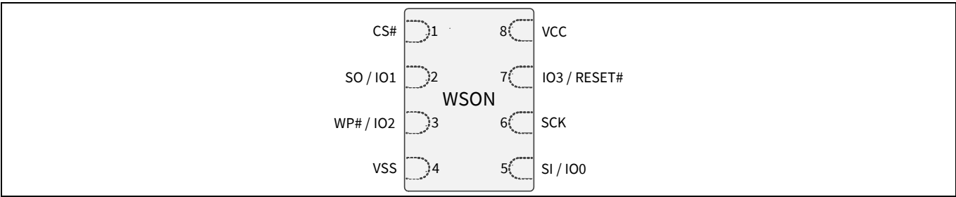
图 4 8 引脚封装 (WSON 6 x 8) (WSON 5 x 6), 俯视图 [2]
