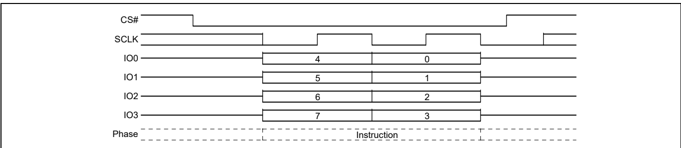
图 102 QPI 模式下的全局 IBL 锁定 (GBL) 命令序列
