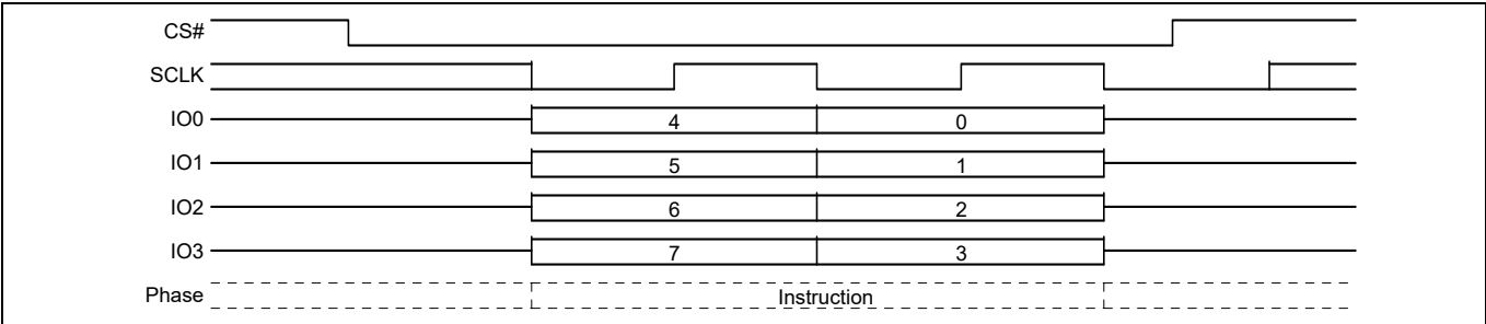
图 114 保护寄存器锁定 (PRL) 命令序列 — QPI 模式
