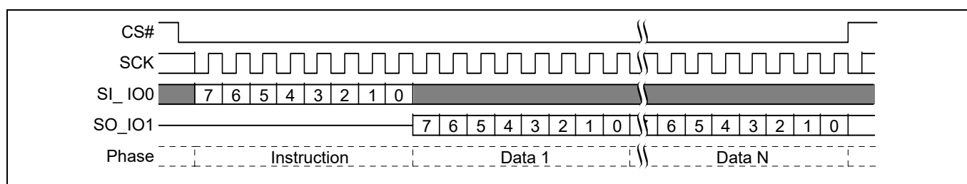
图 27 读取标识（RDID）命令序列
