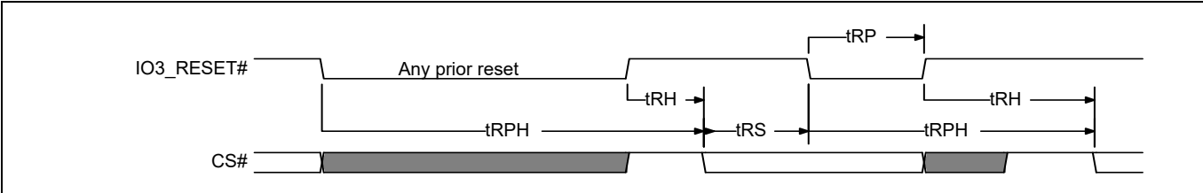
图 140 未启用四线模式或 QPI 模式，并且启用了 IO3 / RESET# 时的硬件复位
