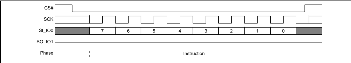
图 91 擦除或编程恢复的命令序列
