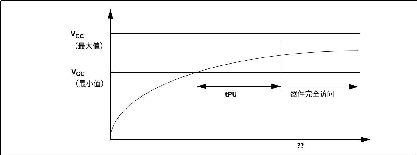
图 131 上电 [63、64]
