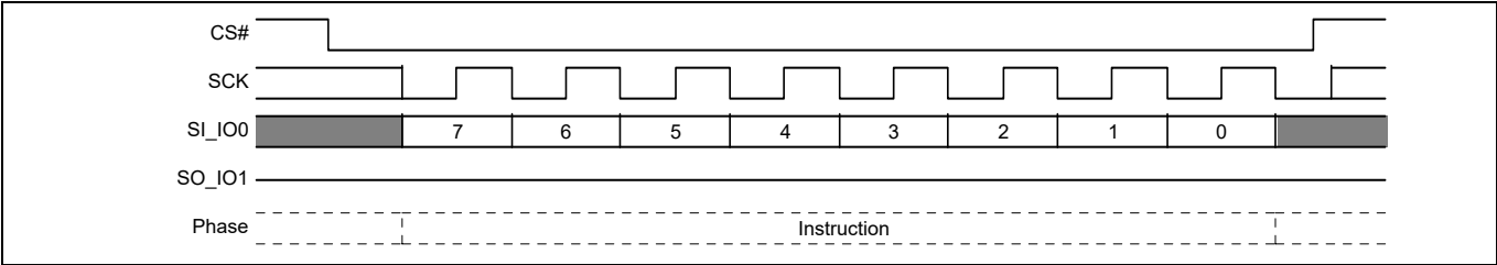
图 45 易失性寄存器的写入启用 (WRENV) 命令序列
