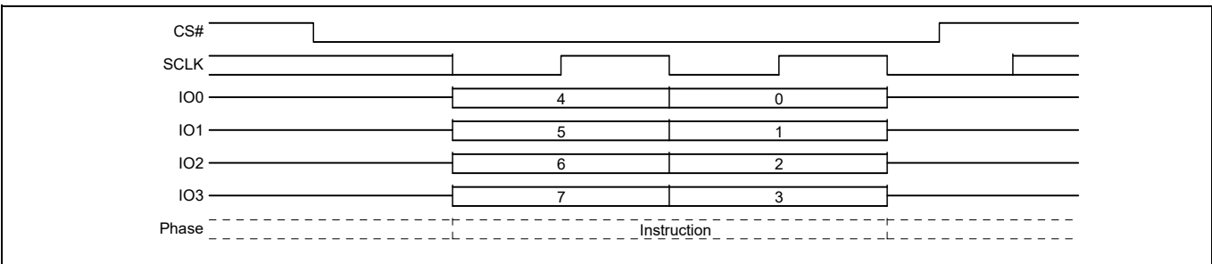
图 104 QPI 模式下的全局 IBL 解锁 (GBUL) 命令序列
