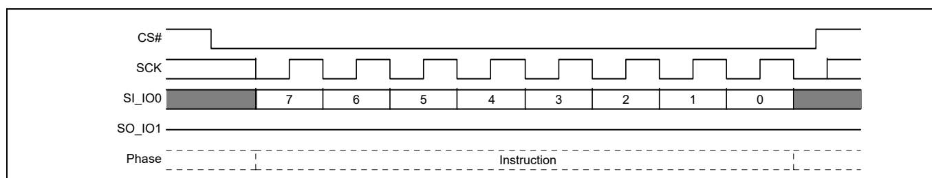
图 41 写入启用 (WREN) 命令序列
