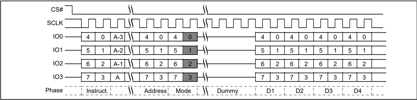
图 72 在 QPI 模式下初始访问的四线 I/O 读取命令序列 [34]
