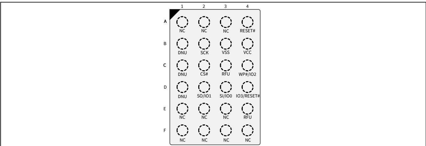
图 6 24 球形焊盘 BGA, 4x6 球型焊盘封装 (FAC024), 俯视图 [4]
