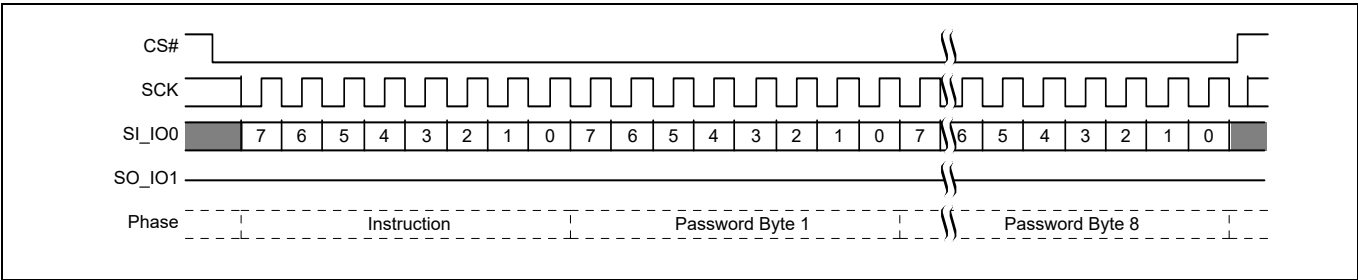
图 117 密码编程 (PASSP) 命令序列
