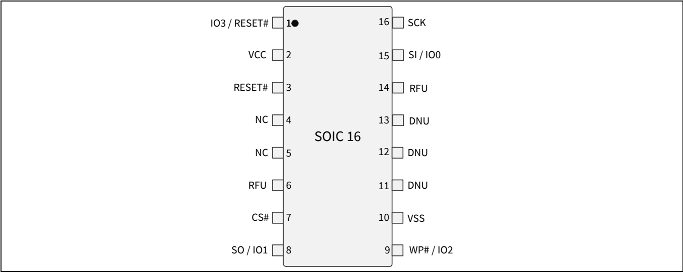
图 1 16 引脚 SOIC 封装 (S03016), 俯视图
