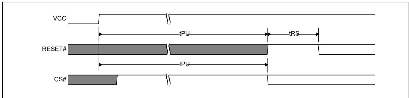
图 138 由硬件复位随后的 POR
