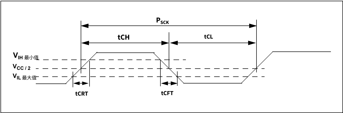
图 142 时钟时序
