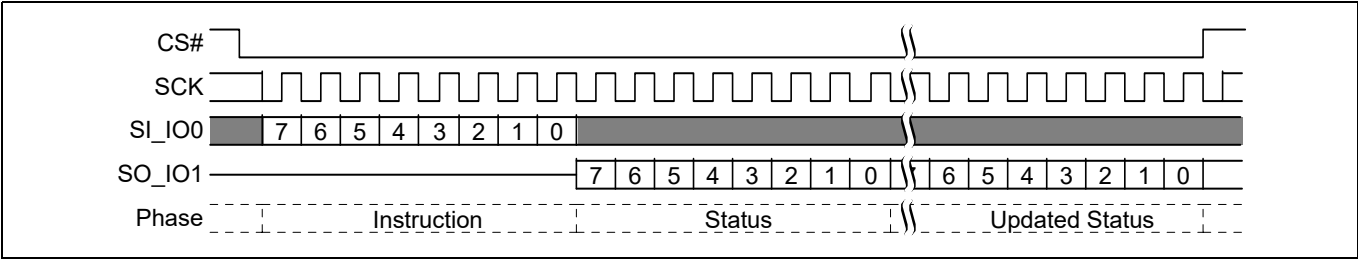
图 35 读取状态寄存器 1 (RDSR1) 命令序列
