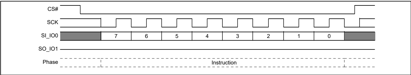
图 88 编程或擦除挂起命令序列
