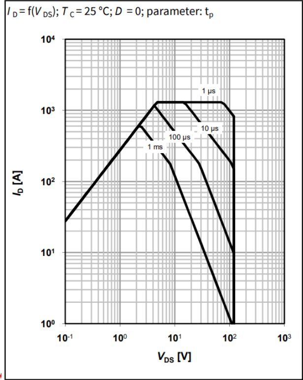
3 安全工作区
