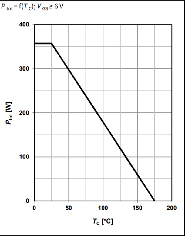
1 功率耗散
