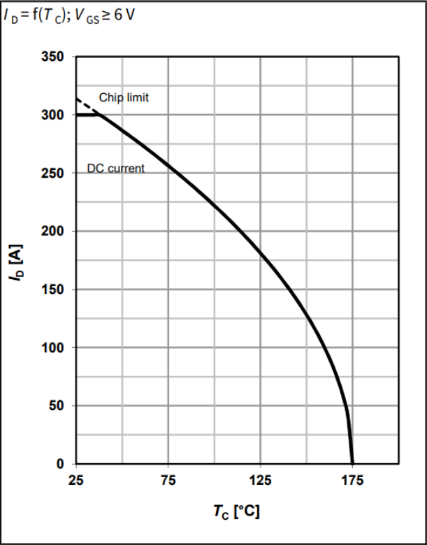
2 漏极电流
