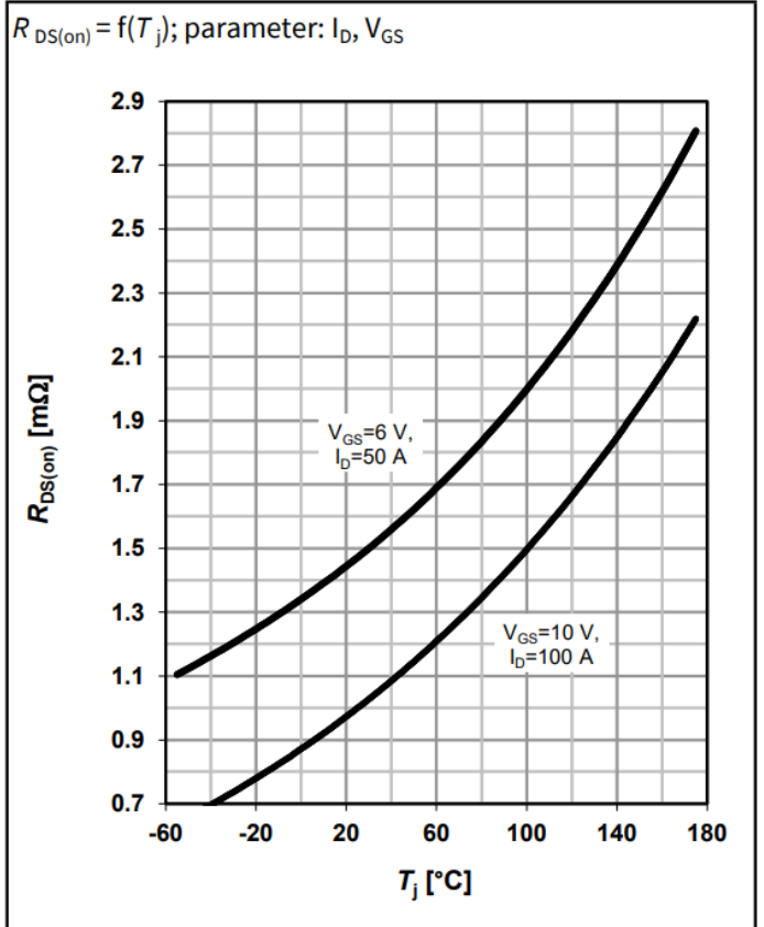
8 典型漏源导通电阻
