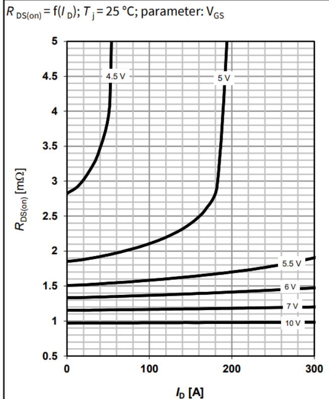
6 典型漏源导通电阻
