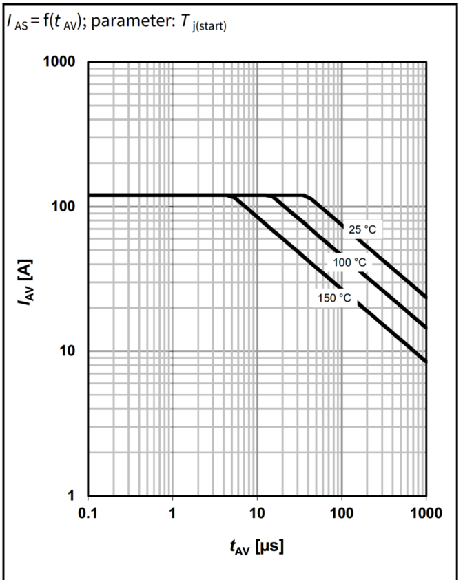
12 典型雪崩特性
