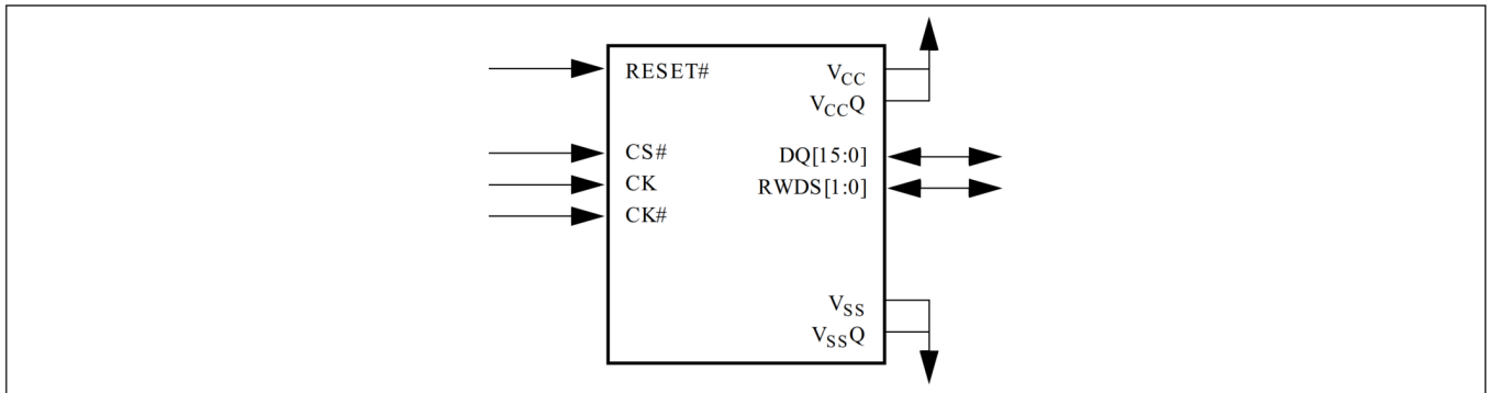
图 5 HYPERRAM™接口 [1]
