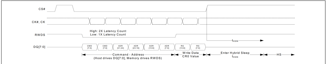
图 15 进入 HS 传输
