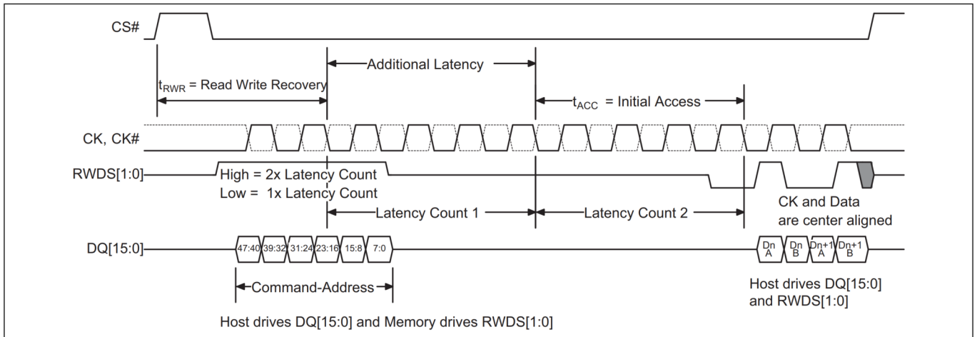
图 11 具有额外初始延迟的写入传输 [33-36]
