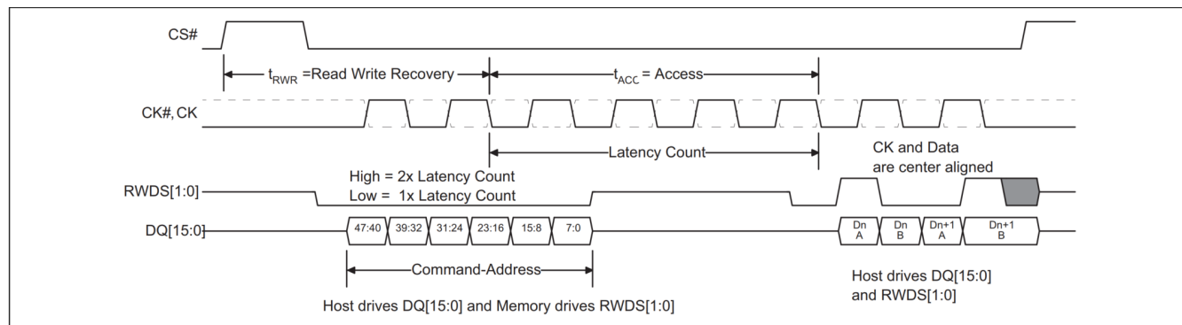
图 3 写入传输，单次初始延迟计数
