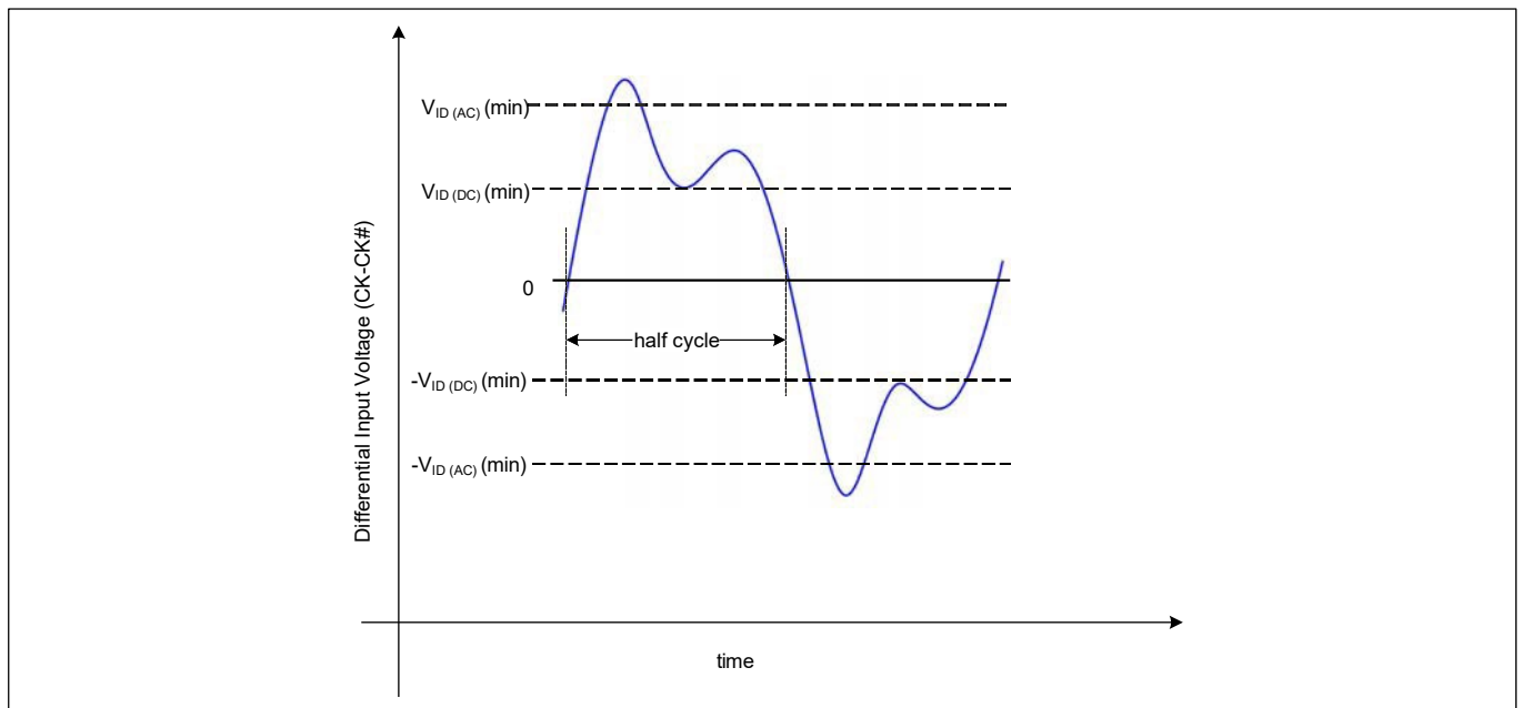
图 29 差分时钟 (CK/CK#) 输入摆幅
