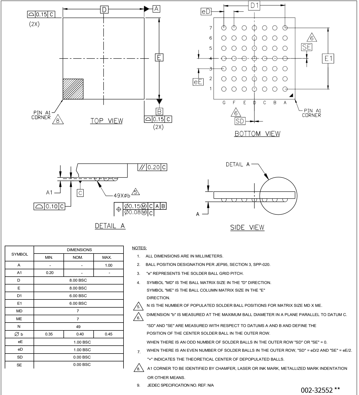
图 37 封装外形, 49 球 BGA 8.0 mm · 8.0 mm · 1.0 mm VAD049
