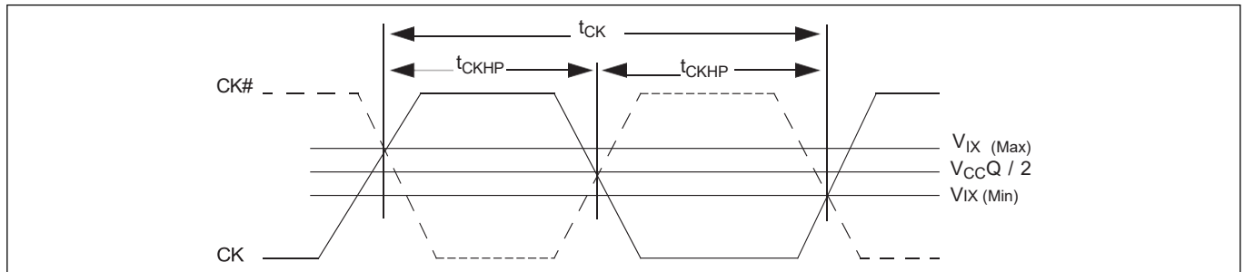
图 28 时钟特性
