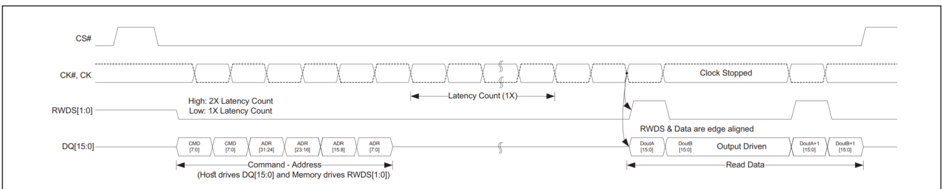
图 14 读取传输期间的有效时钟停止 (DDR) [47, 48]
