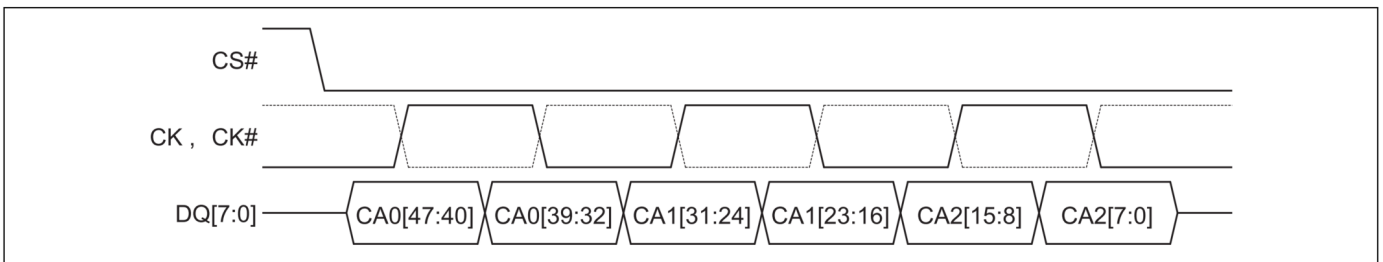
图 6 指令-地址 (CA) 序列 [3-7]
