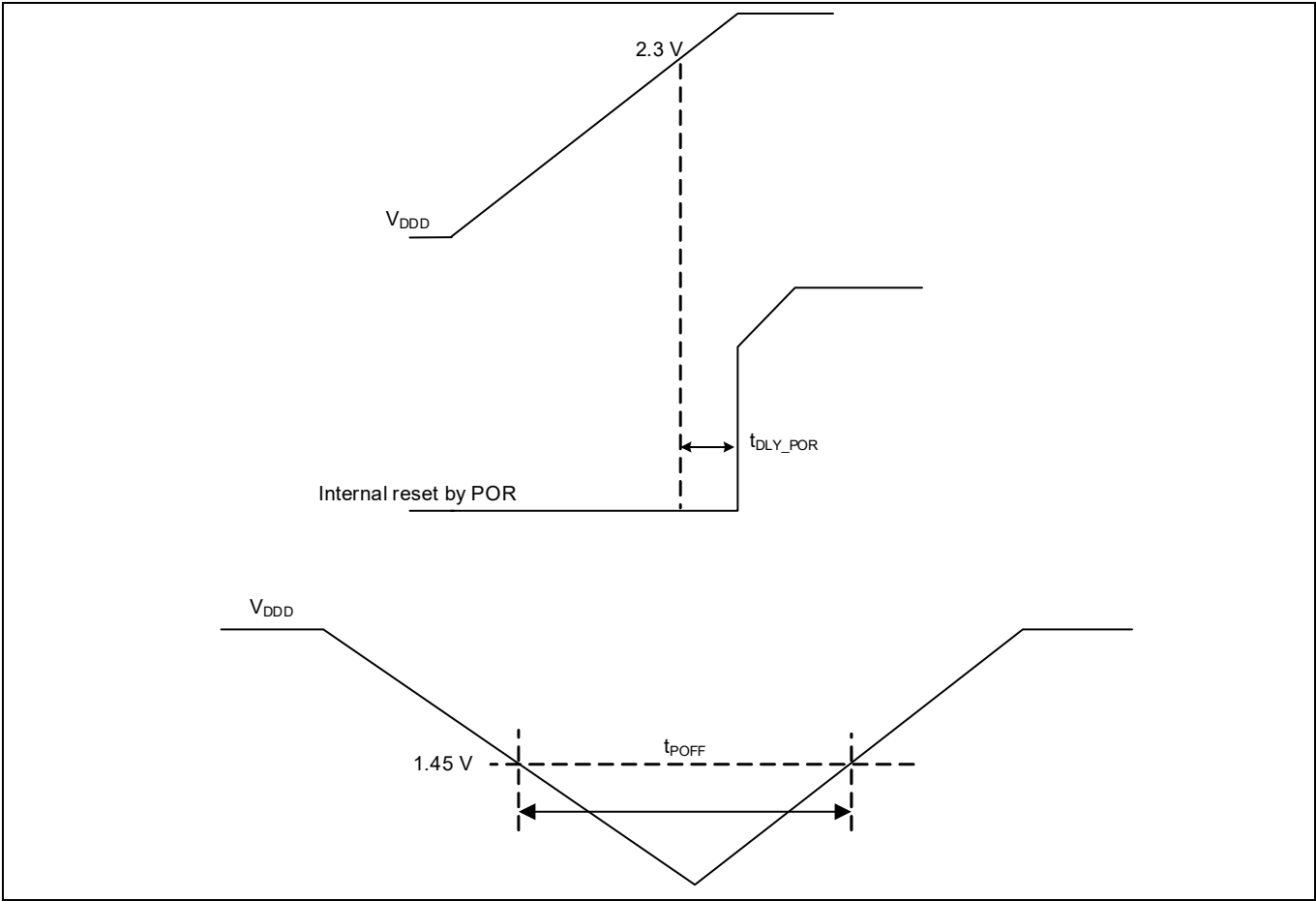
Figure 28 POR specifications
