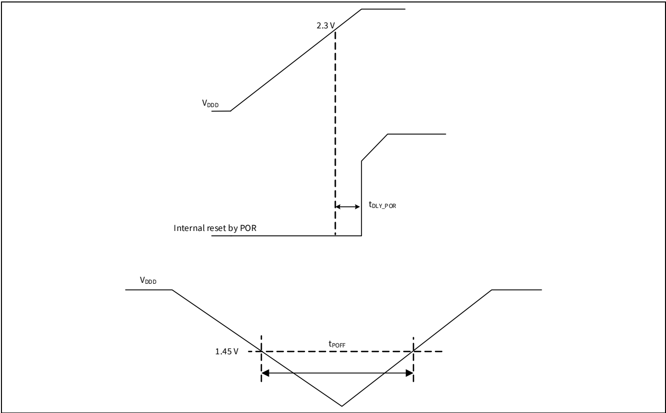
Figure 29 POR specifications
