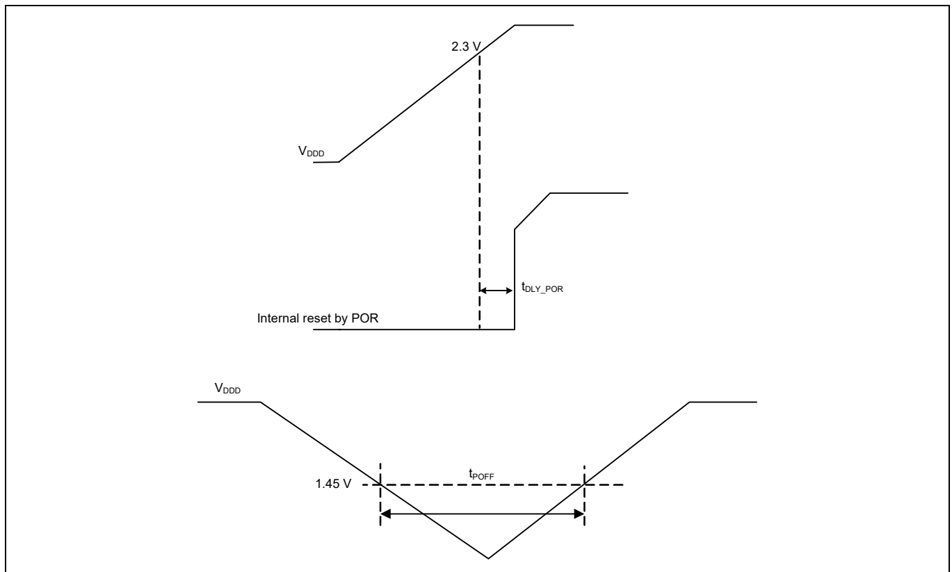
Figure 29 POR specifications
