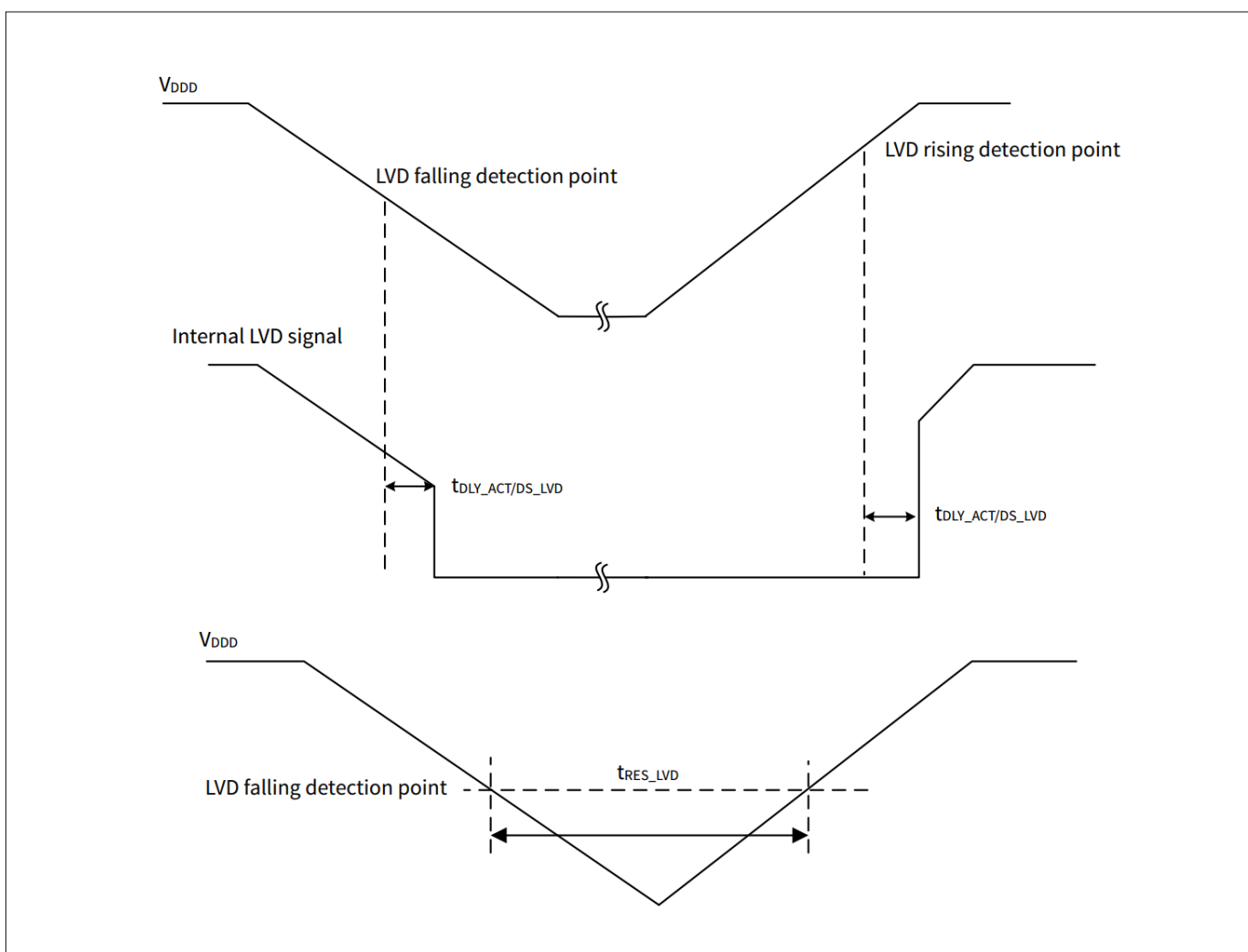
图 34 LVD规格
