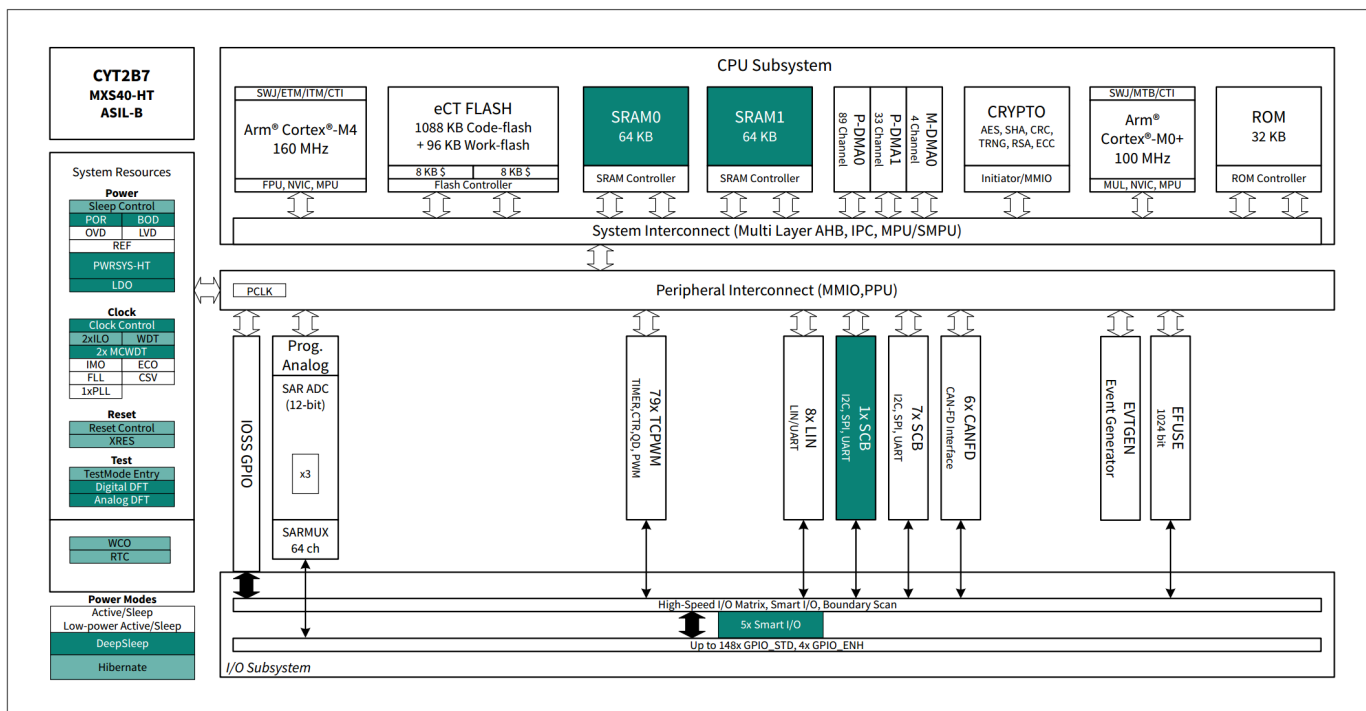
图 1 框图
