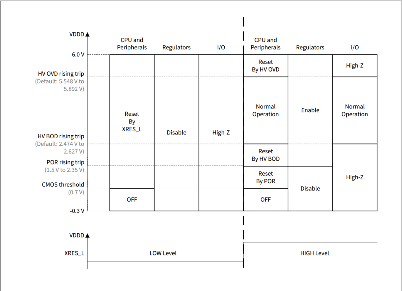
图 28 器件操作电源范围
