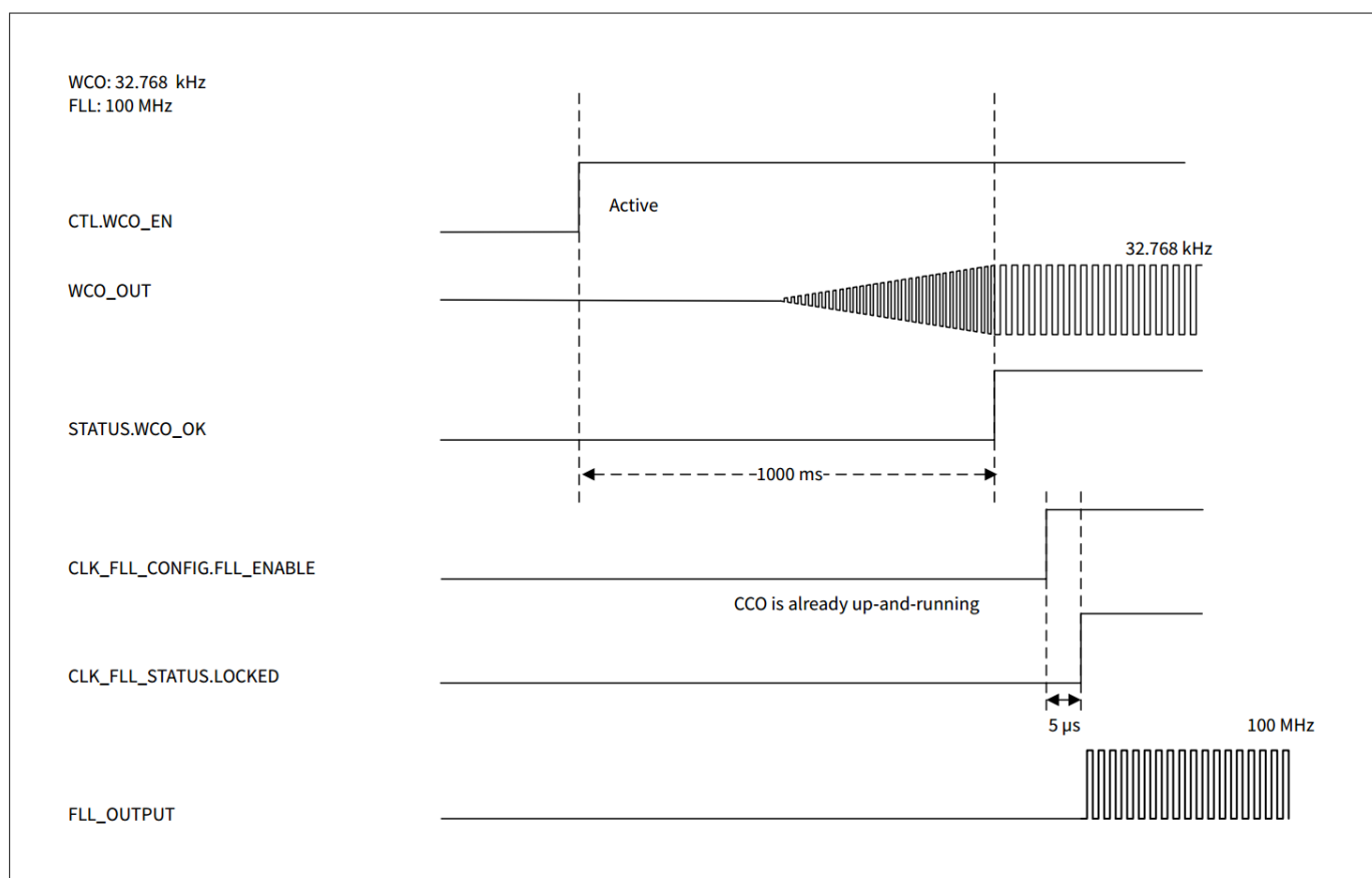
图 39 WCO 至 FLL 图
