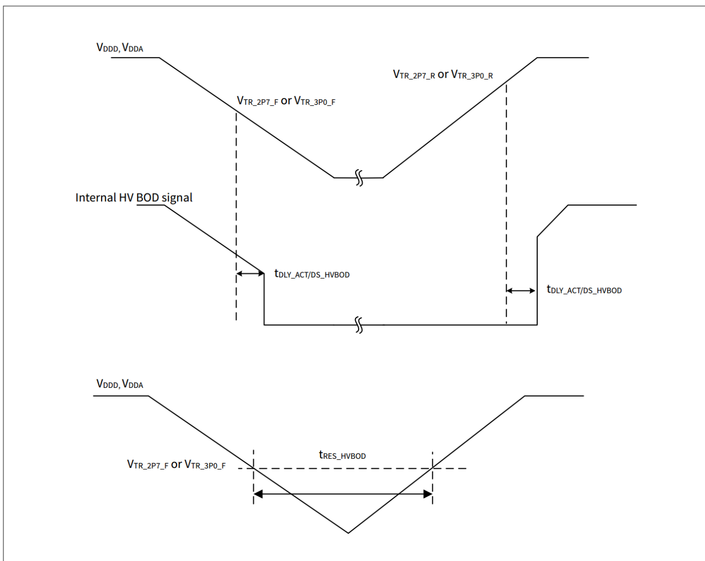
图 30 高压 BOD 规格
