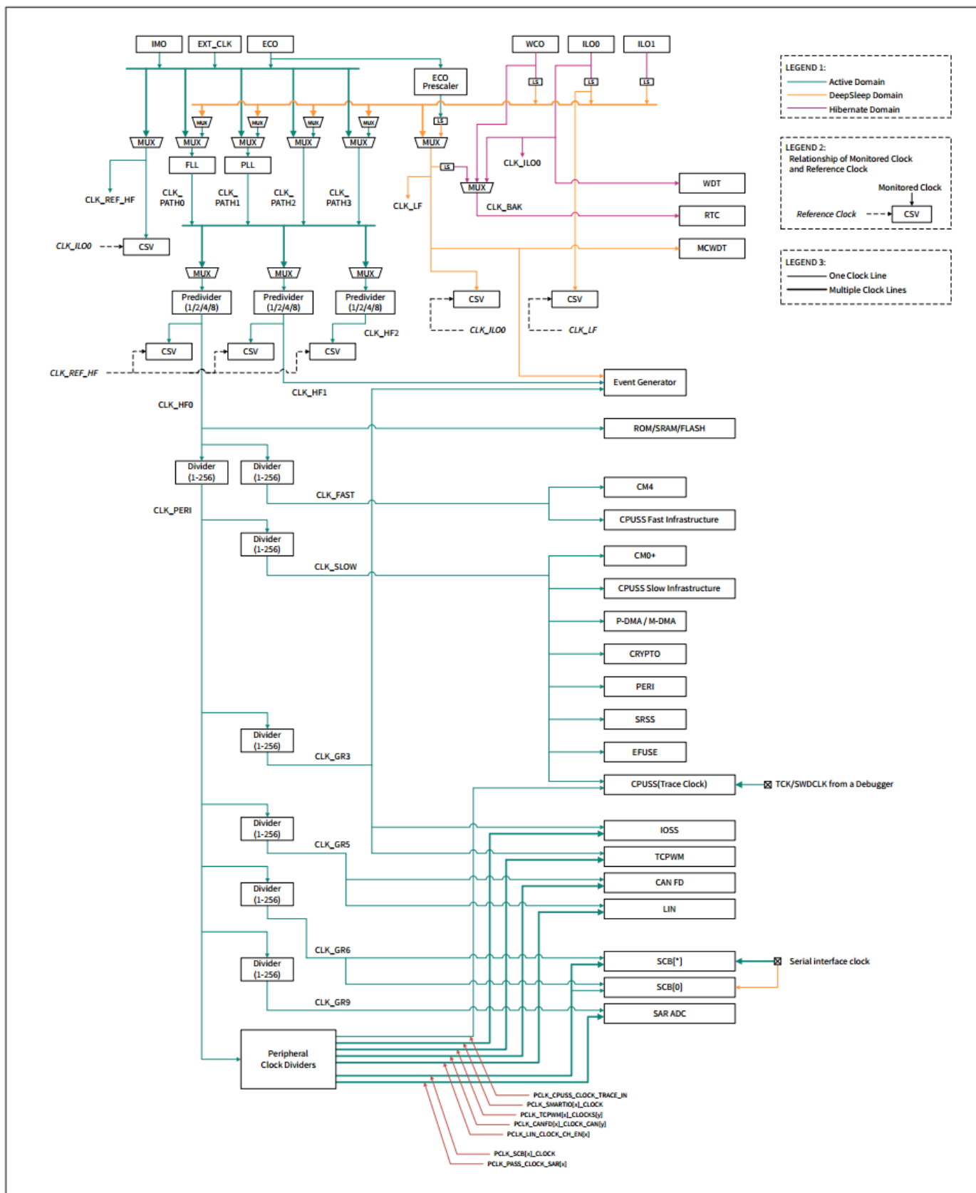
图 3 CYT2B7 时钟图
