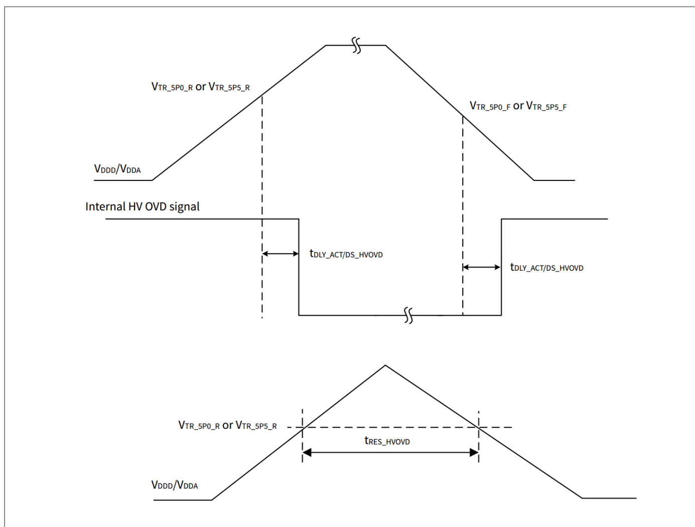
图 32 高压 OVD 规格
