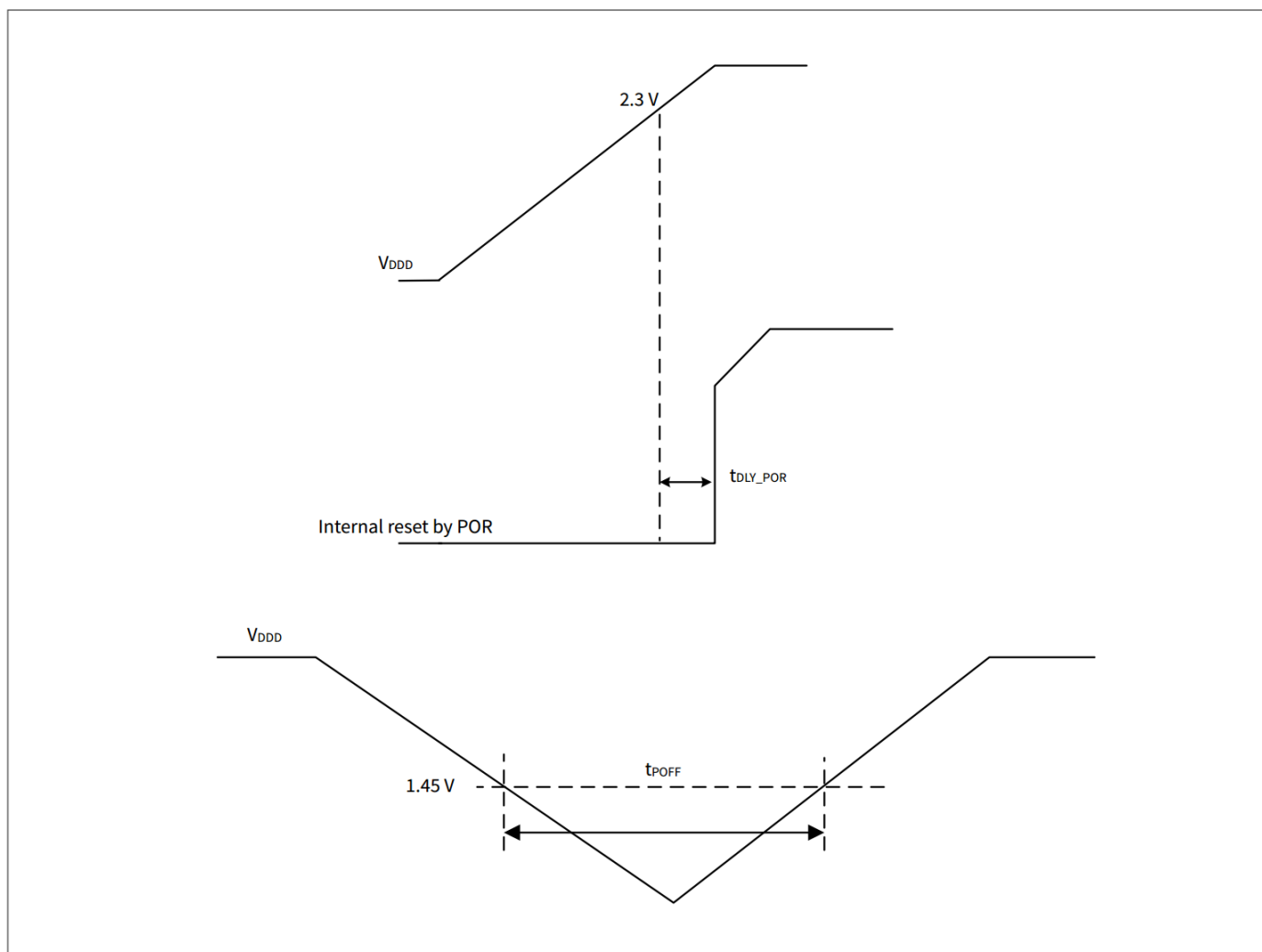
图 29 POR 规格
