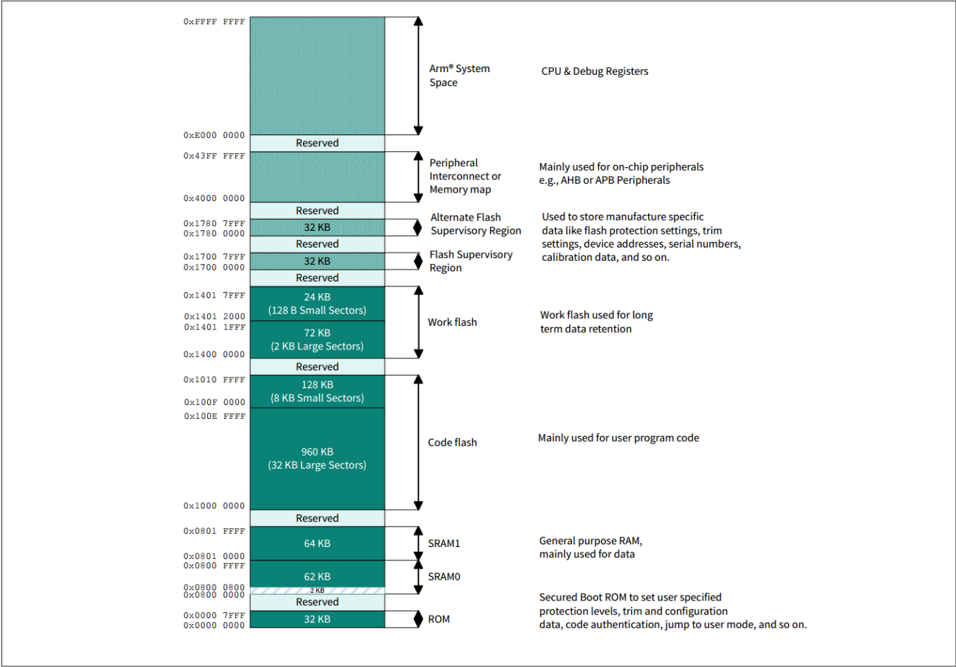
图 2 CYT2B7 地址映射 12) , 13)
