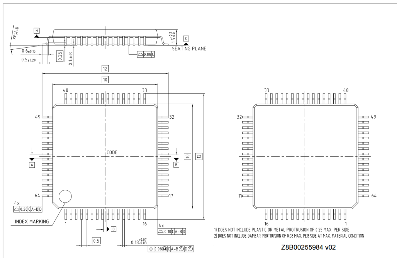
图 41 144-LQFP 封装外形 (PG-LQFP-144)
