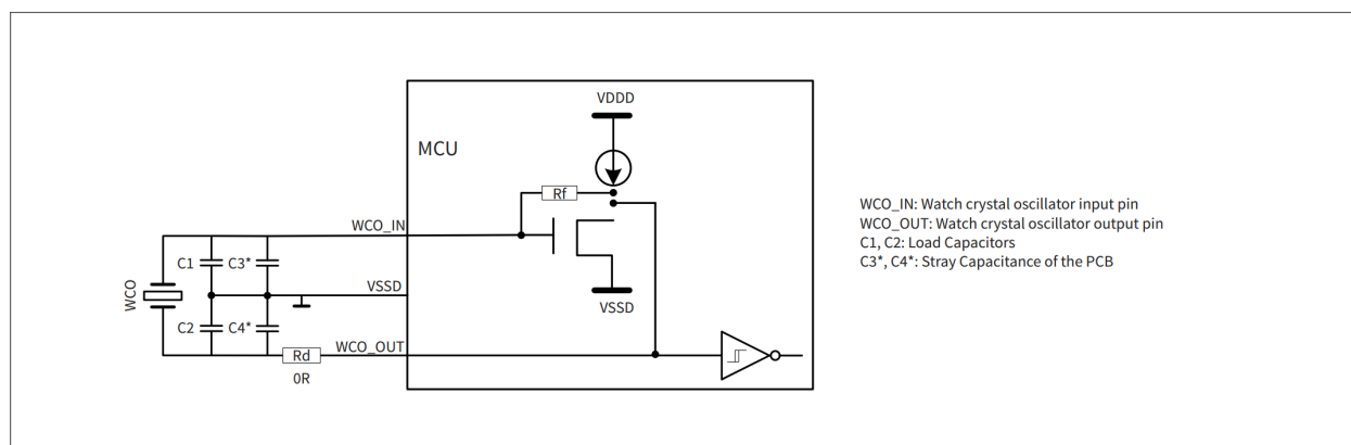
图 37 WCO 连接方案 18)
