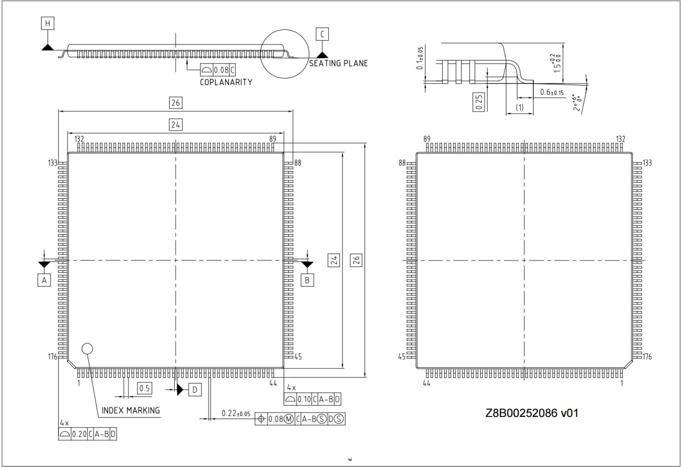
图 40 176-LQFP 封装外形 (PG-LQFP-176)
