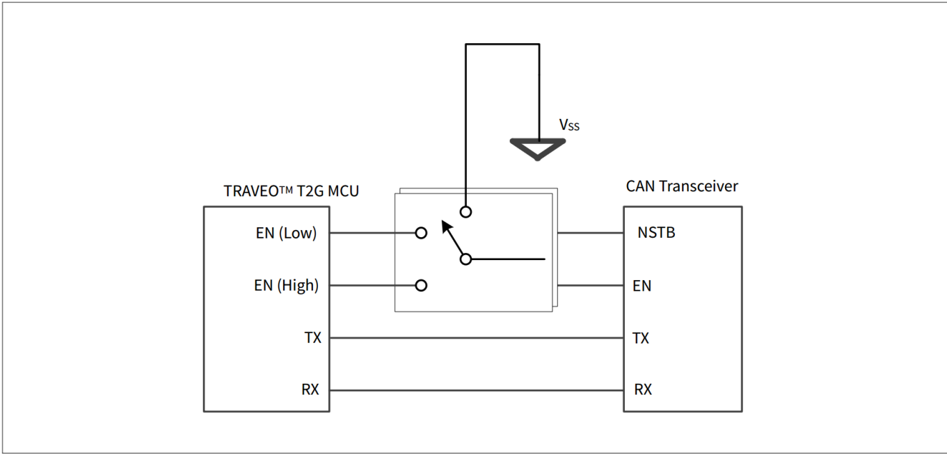
图 46 MCU 至 CAN 收发器连接
