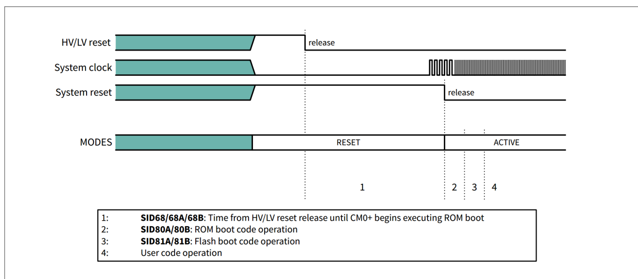
图 17 复位序列
