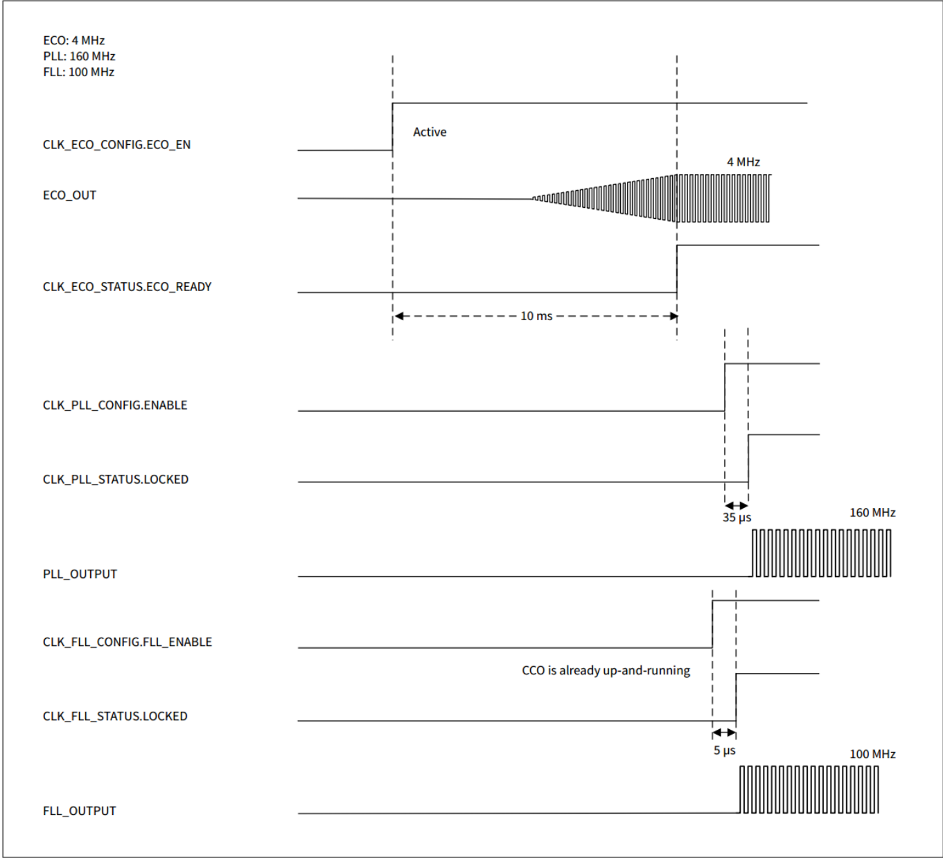
图 38 ECO 至 PLL 或 FLL 图
