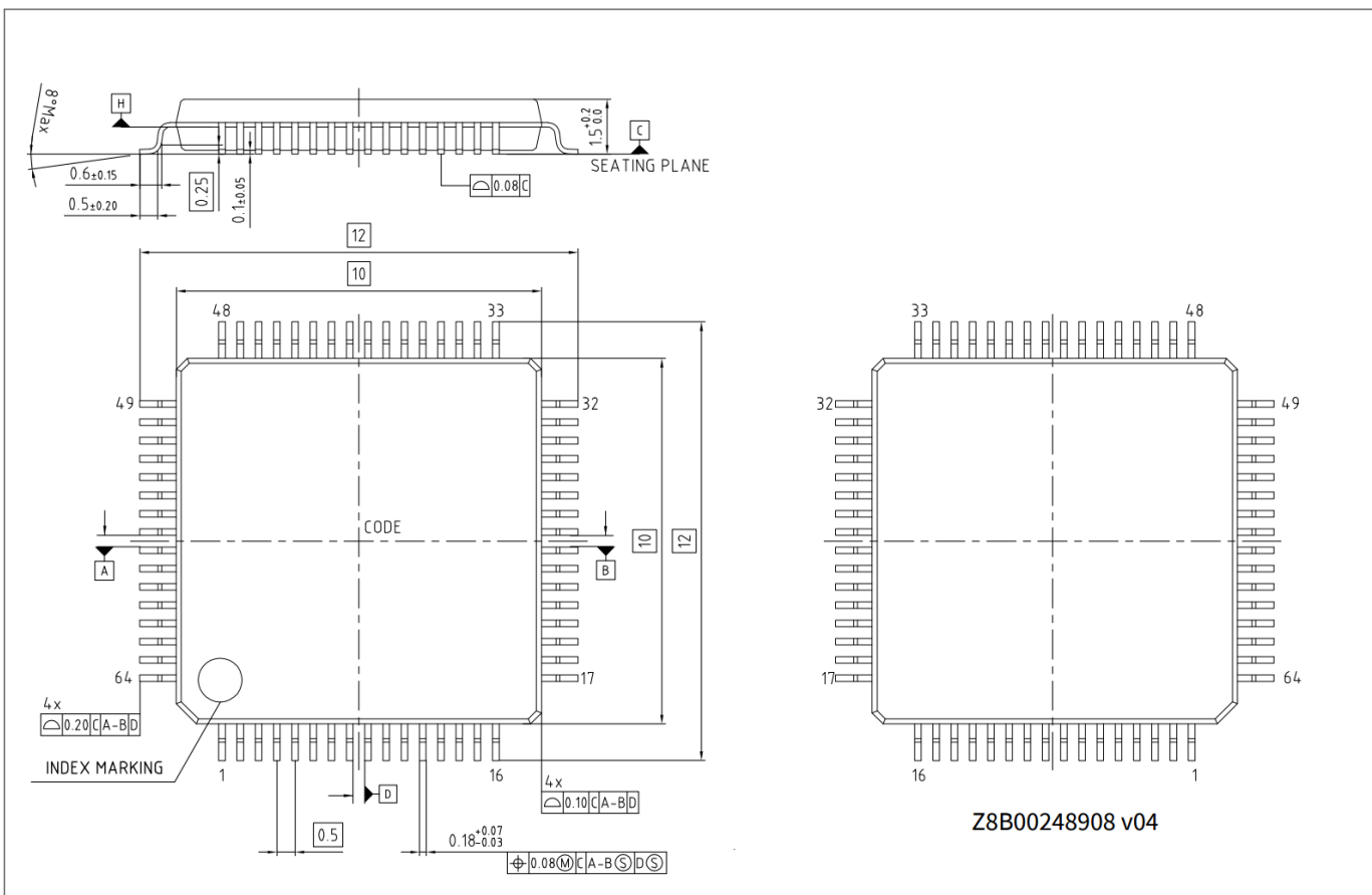
图 44 64-LQFP 封装外形 (PG-LQFP-64)
