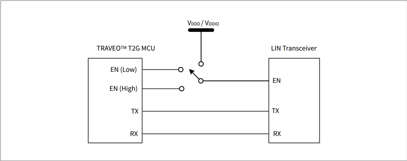
图 47 MCU 至 LIN 收发器连接
