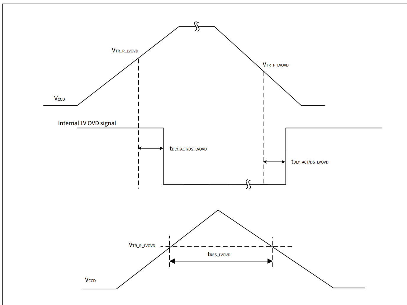
图 33 低压 OVD 规格
