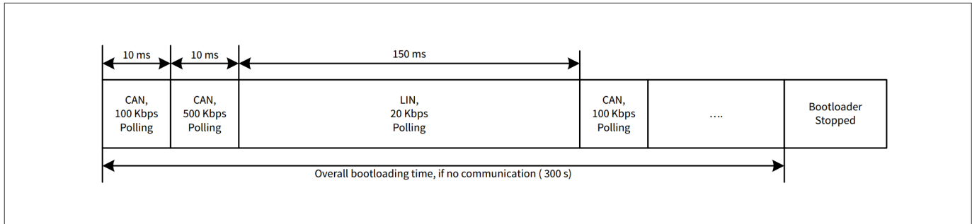
图 45 引导加载序列
