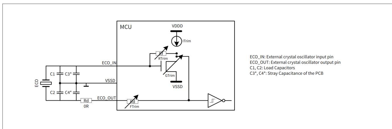
图 36 ECO 连接方案 17)
