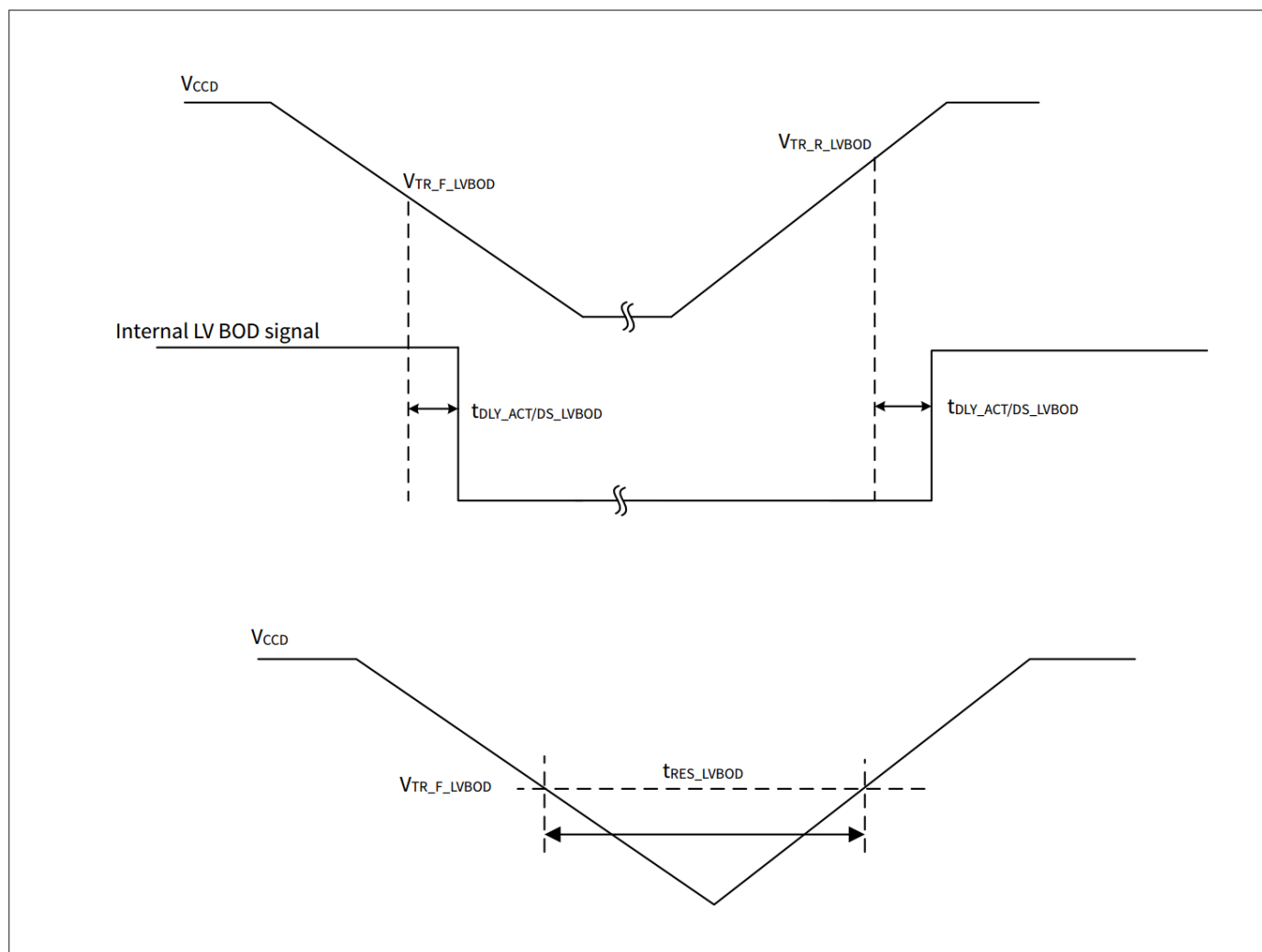
图 31 低压 BOD 规格
