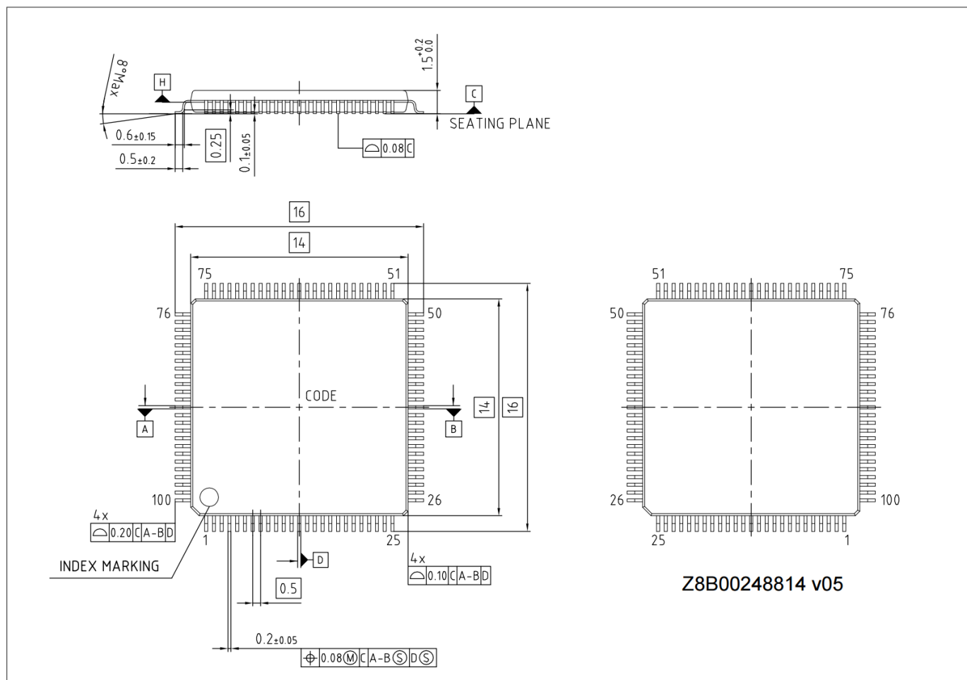
图 42 100-LQFP 封装外形 (PG-LQFP-100)
