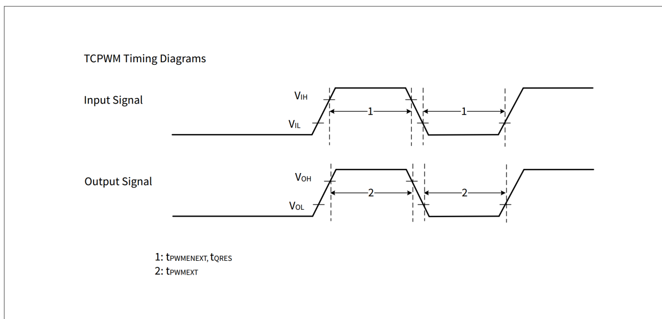
图 22 TCPWM 时序图
