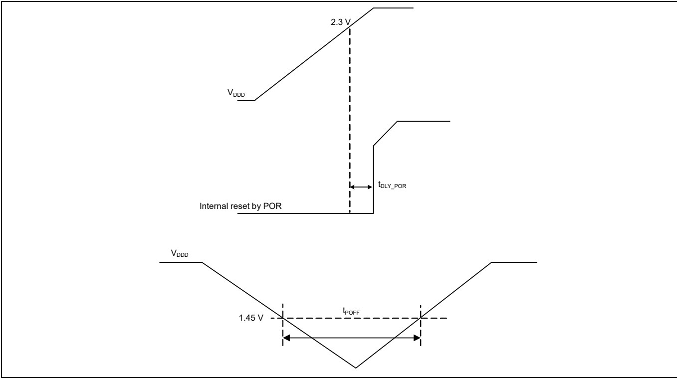
Figure 24 POR specifications
