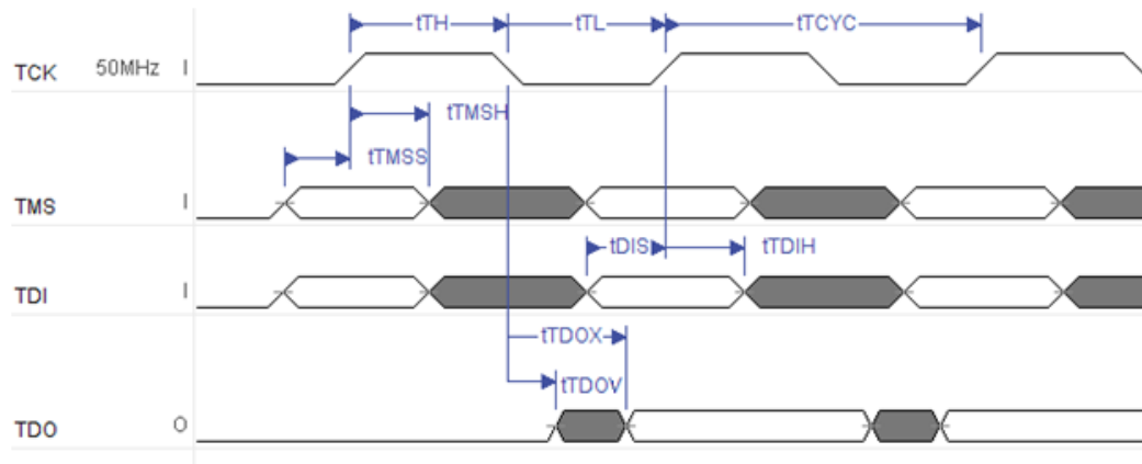
图 6. TAP 时序图
