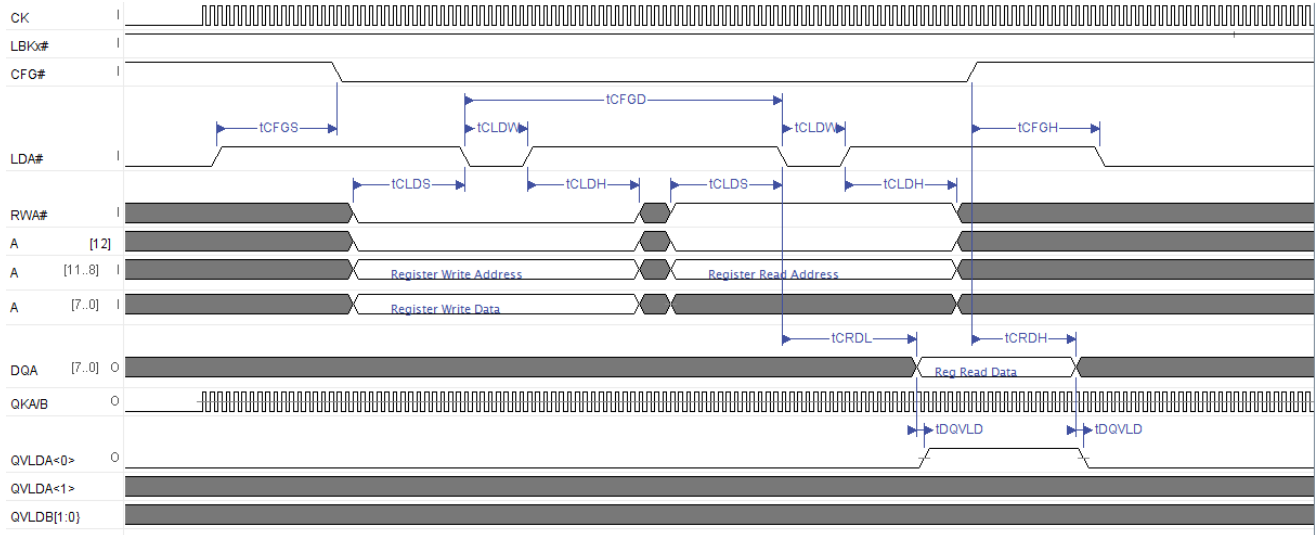
图 14. 配置写入和读取操作的时序波形
