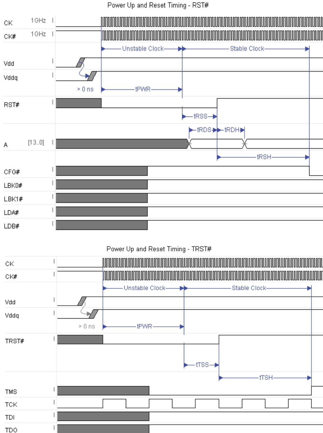
图 16. 复位时序波形
