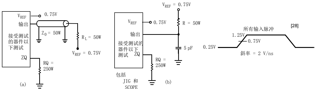
图 4. 交流测试负载和波形
