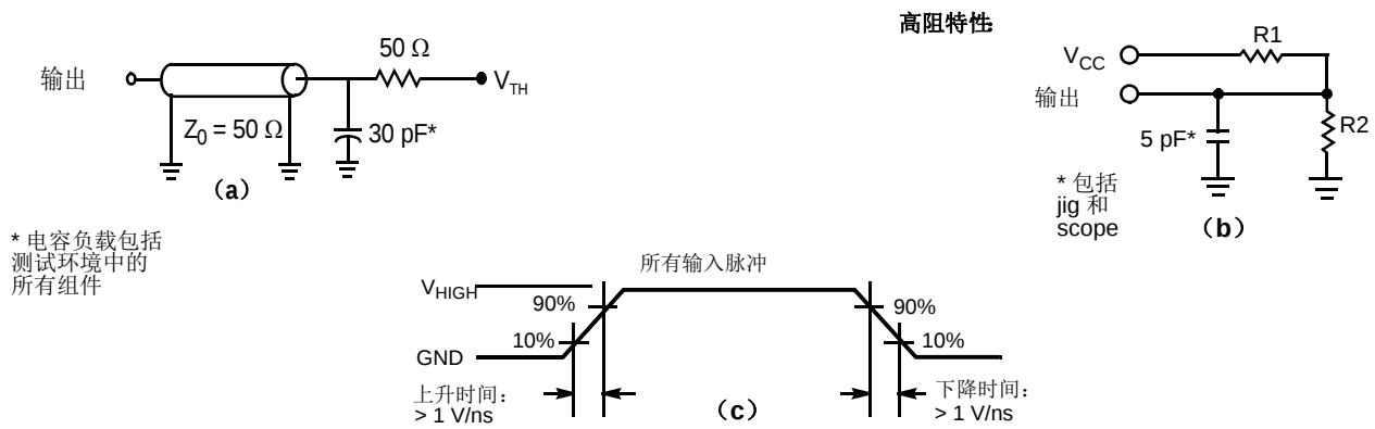
图 3. 交流测试负载和波形 [8]
