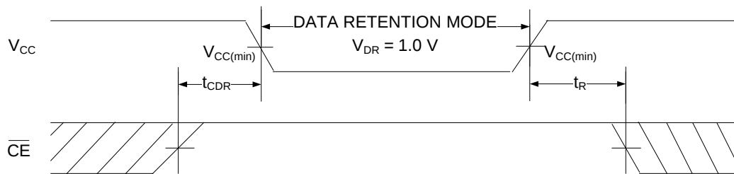
图 4. 数据保持波形 [9]
