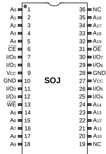
图 1. 36-SOJ 引脚分布 [2]
