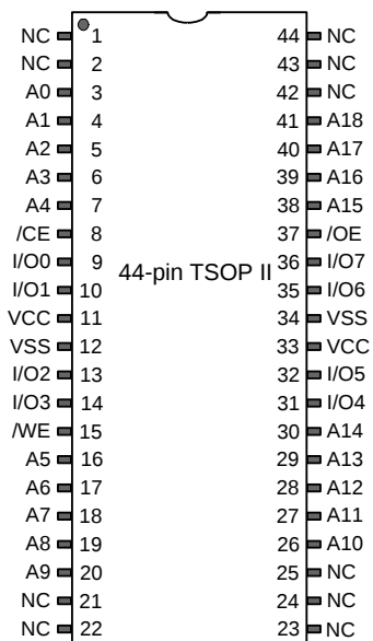
图 2. 44-TSOP II 引脚分布，单芯片使能 [3]
