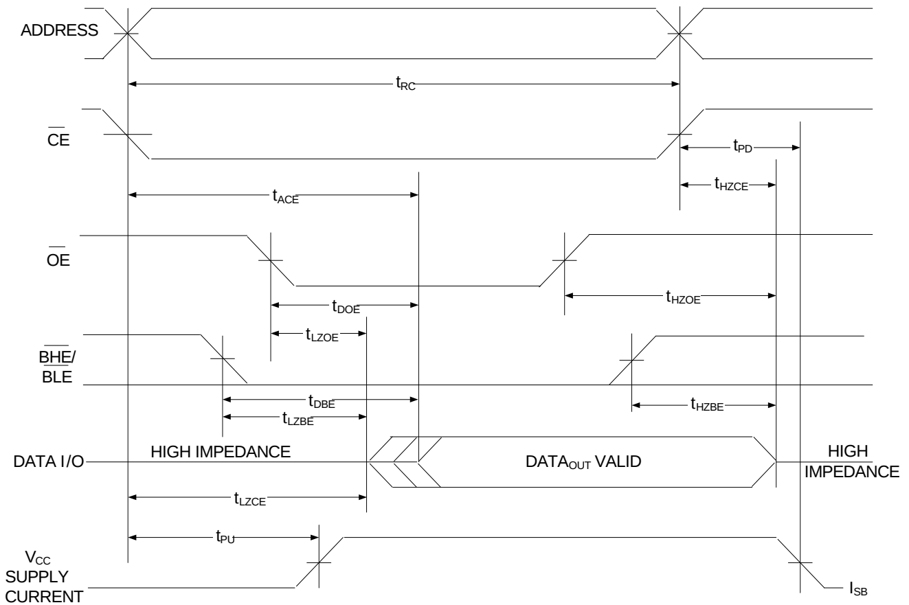
图 6. 第二个读周期（由 \overline{OE} 控制） [16、17]
