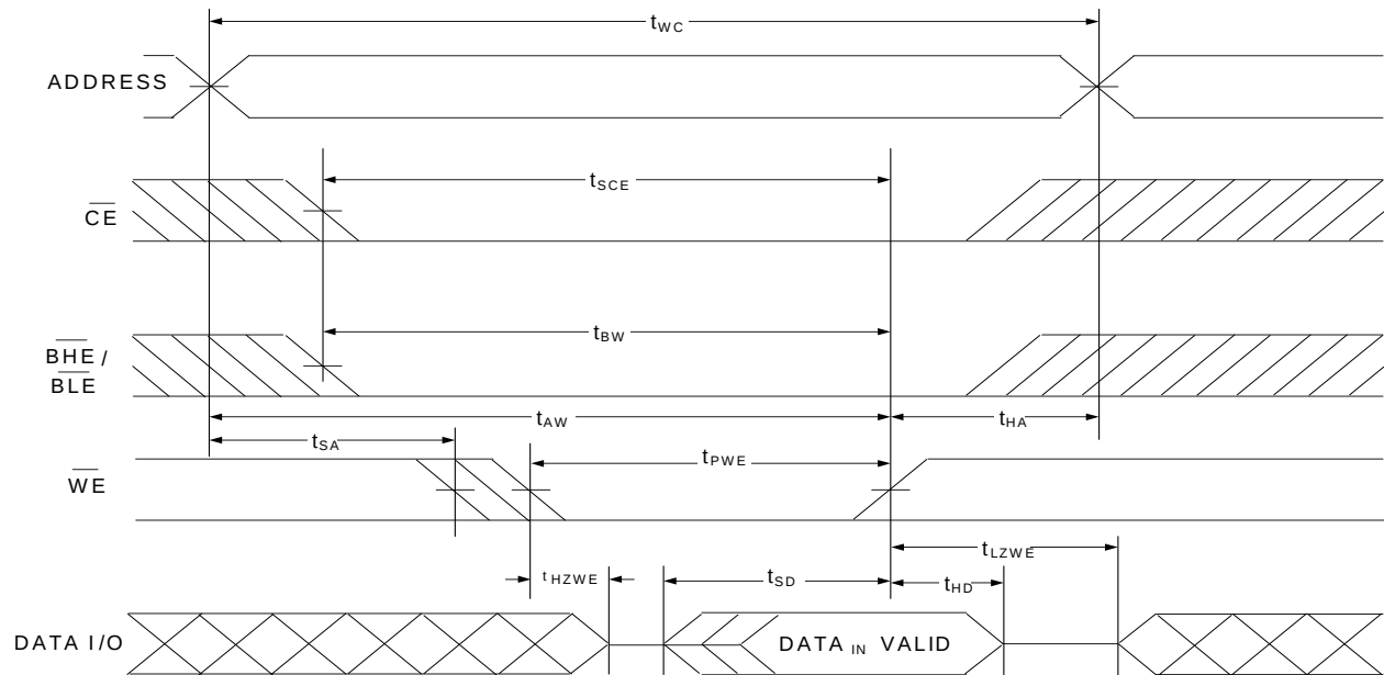
图 8. 第二个写周期（由 \overline{WE} 控制， \overline{OE} 为低电平） [18、19、20]
