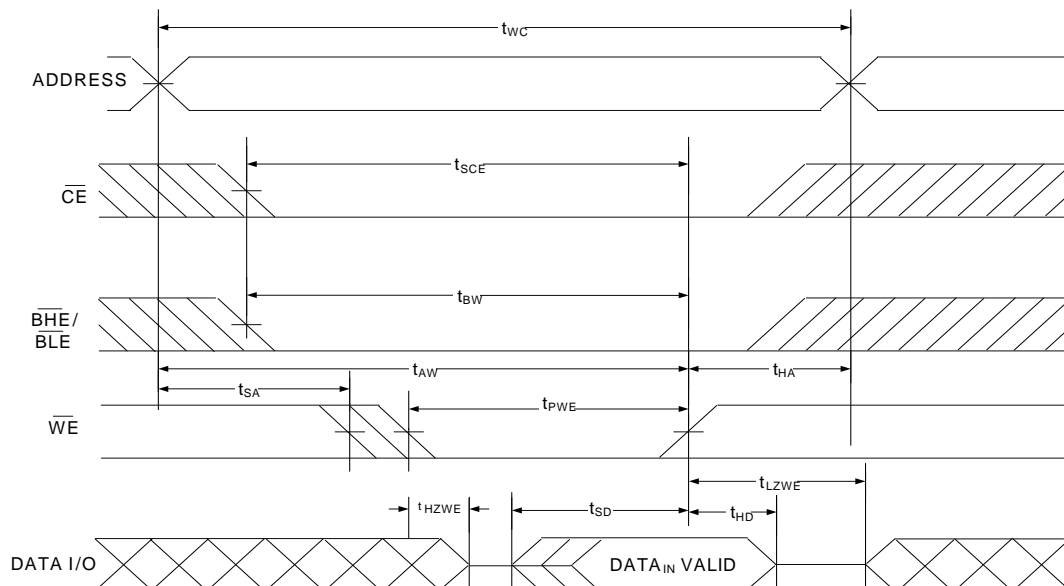
図 15. 書き込みサイクル 3 ( \overline{\text{WE}} 制御、 \overline{\text{OE}} LOW) [32、33、34、35]
