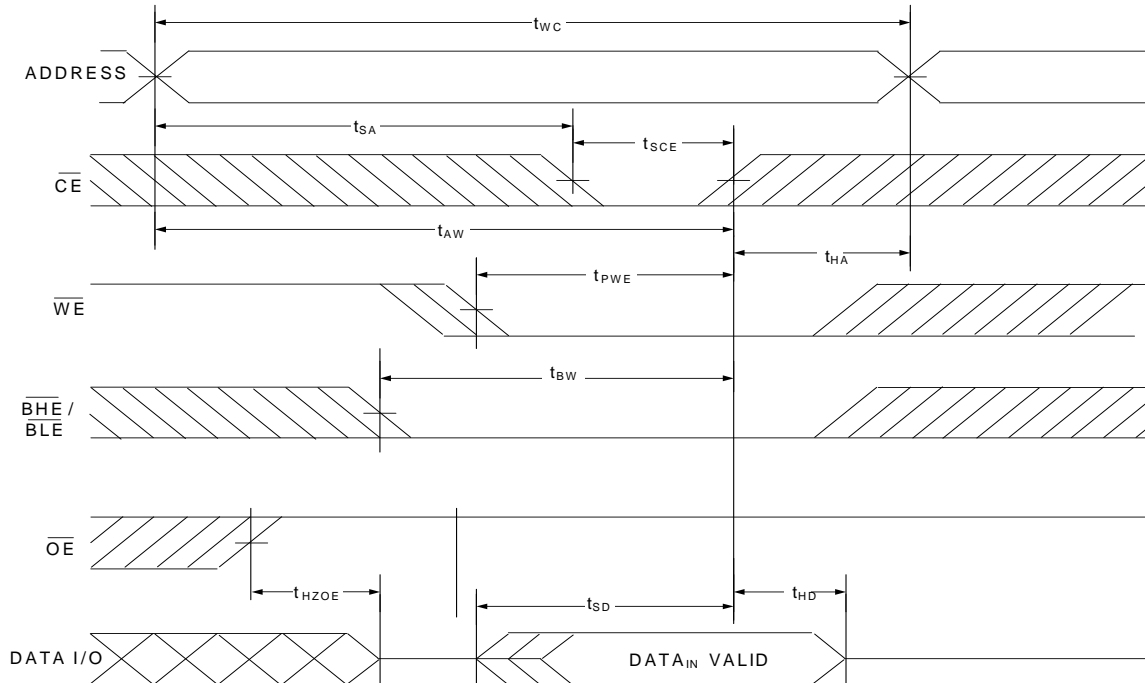
図 15. 書き込みサイクル 3 ( \overline{\text{WE}} 制御、 \overline{\text{OE}} LOW) [32、33、34、35]
