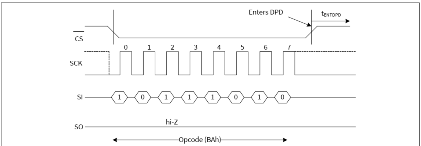
图 19 DPD 进入时序
