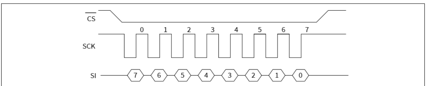
图5 SPI模式3
