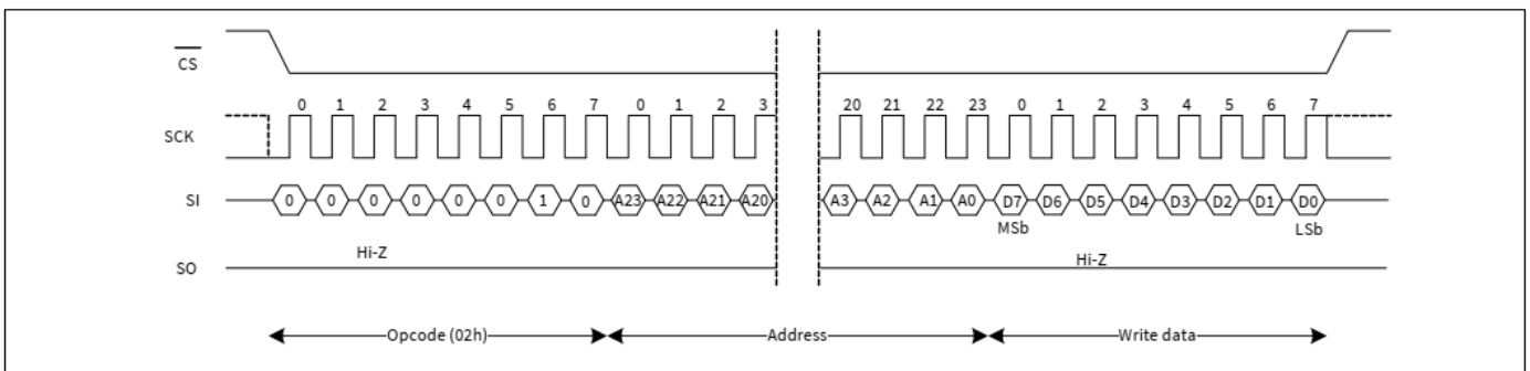
图 10 存储器写入（未显示 WREN）操作
