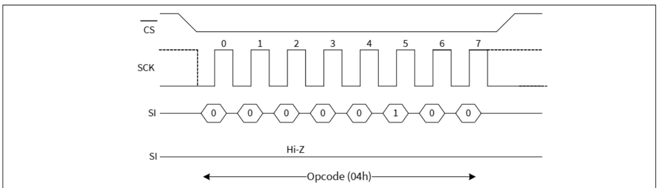
图 7 WRDI 总线配置
