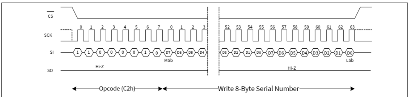
图 17 写入序列号 (未显示 WREN) 操作
