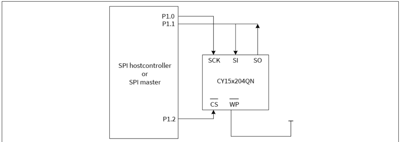
图 3 无SPI端口的系统配置
