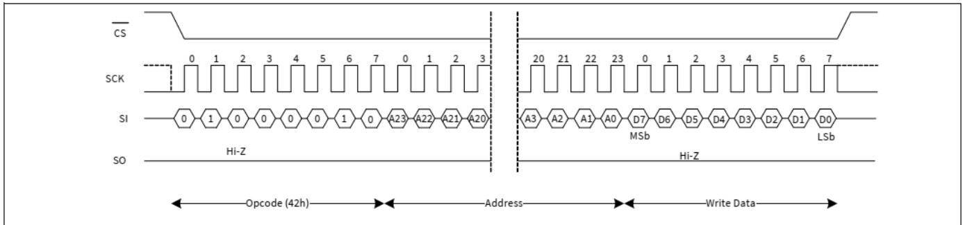
图 13 特殊扇区写 (未显示 WREN) 操作
