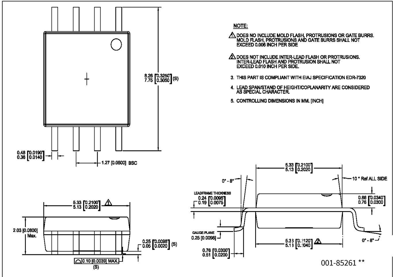
图 25 8 引脚SOIC (208 Mils) 封装外形, 001-85261
