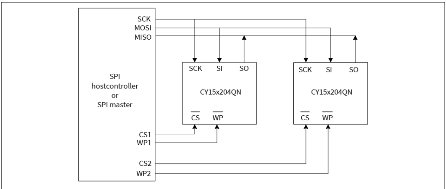
图2 使用SPI端口的系统配置
