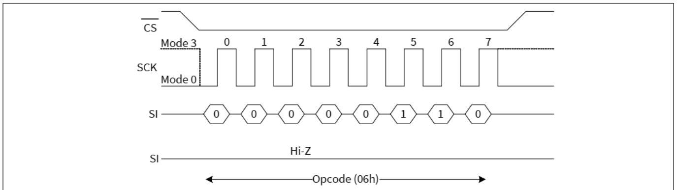
图 6 WREN 总线配置
