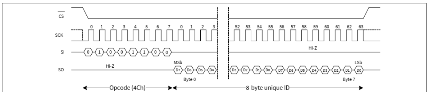
图 16 读取唯一 ID
