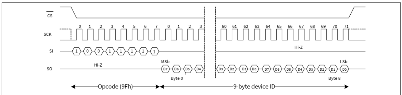
图 15 读取设备 ID
