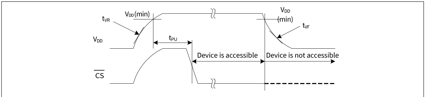
图 24 上电时序
