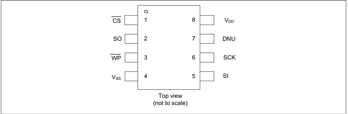
图 1 8 引脚 SOIC 引脚排列
