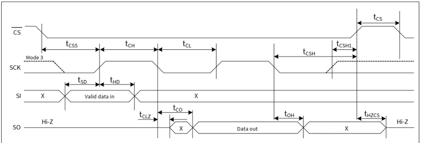
图 22 同步数据时序（模式 0 和模式 3）
