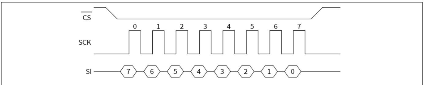
图4 SPI模式0
