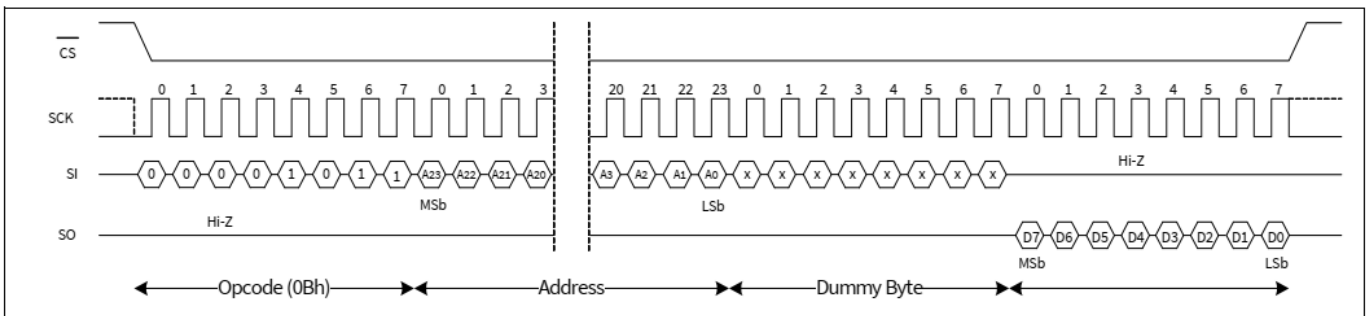
图 12 快速读操作
