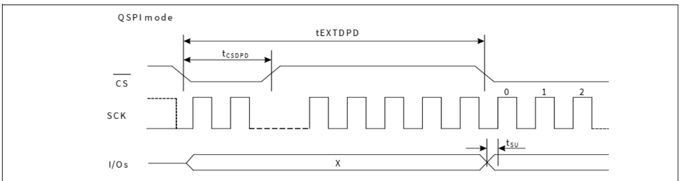
图 20 DPD 退出时序
