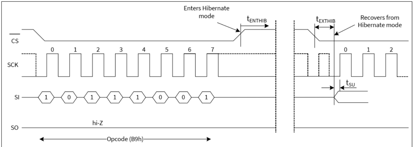
图 21 休眠模式操作
