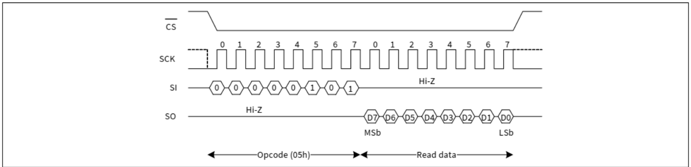
图 8 RDSR 总线配置
