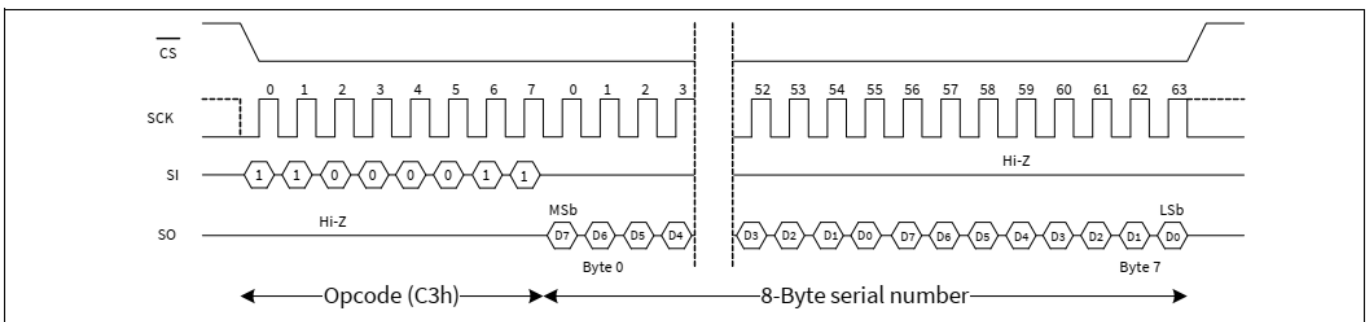
图18 读取序列号操作
