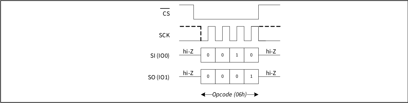
Figure 7 DPI 模式下的 WREN 总线配置
