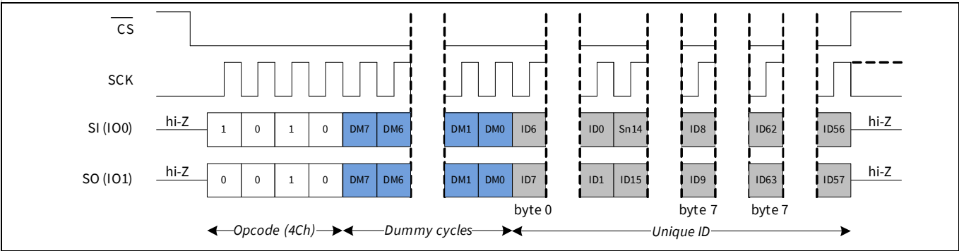
Figure 91 DPI 模式下的读取唯一 ID
