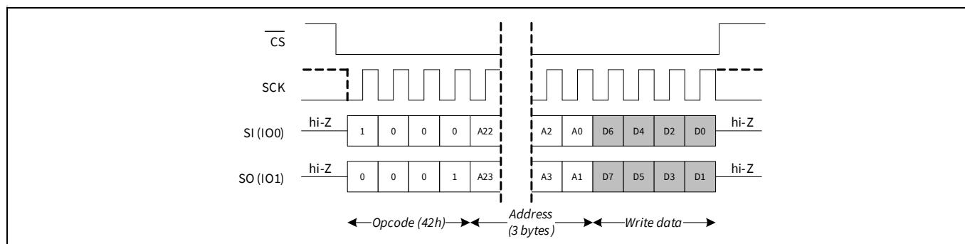
Figure 67 DPI 模式下的特殊扇区写入 (SSWR) (WREN 未显示)
