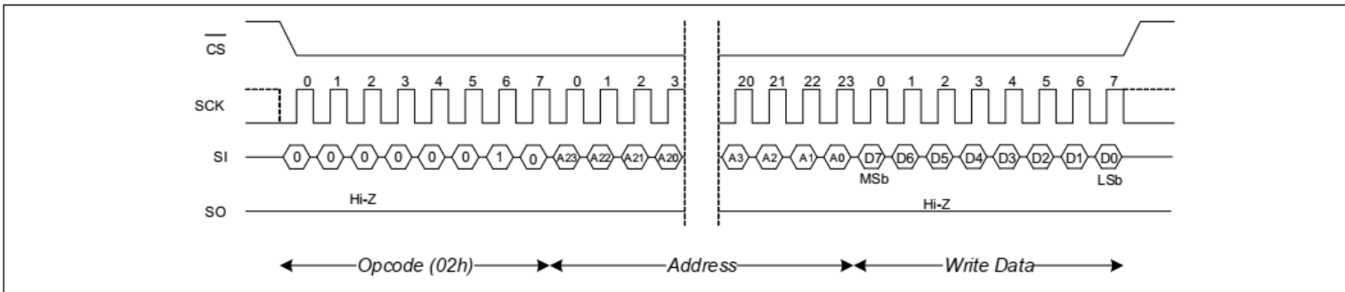
图8 存储器写入操作
