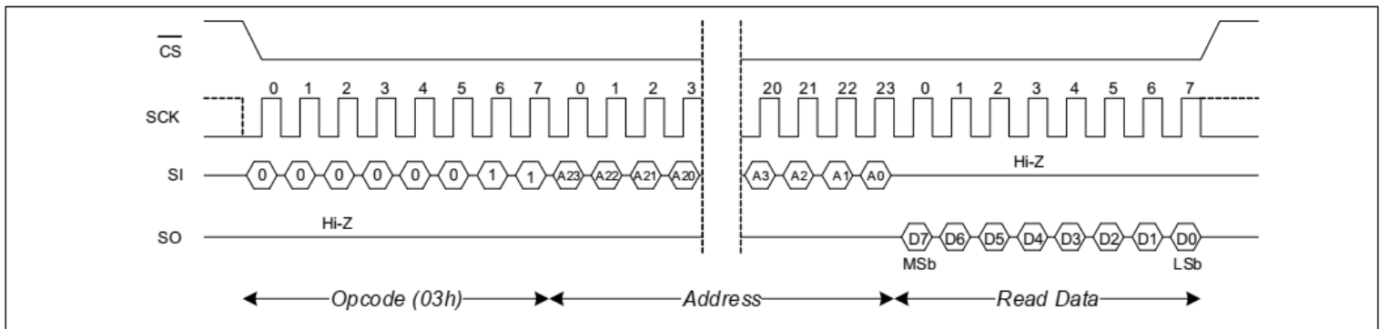
图 9 存储器读操作
