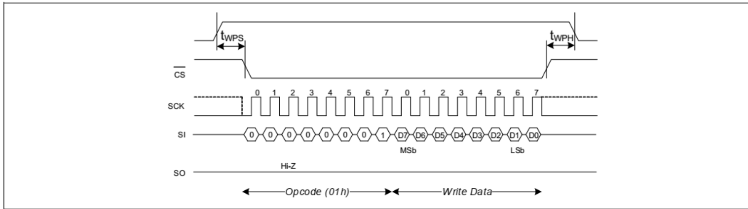
图 21 写状态寄存器 (WRSR) 操作期间的写保护时序
