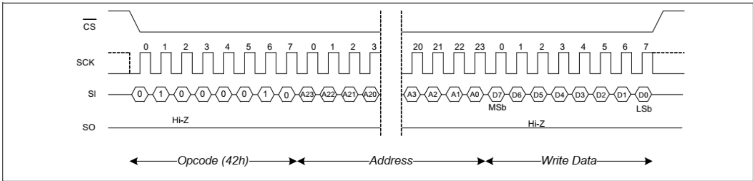
图 11 特殊扇区写入操作
