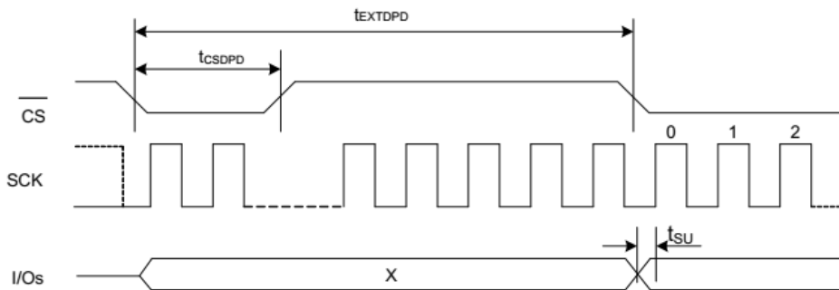
图 18 DPD 退出时序
