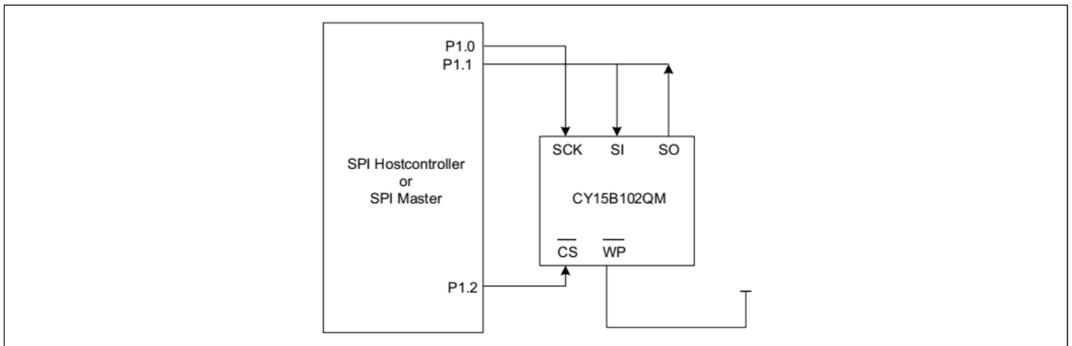
图 3 无SPI端口的系统配置
