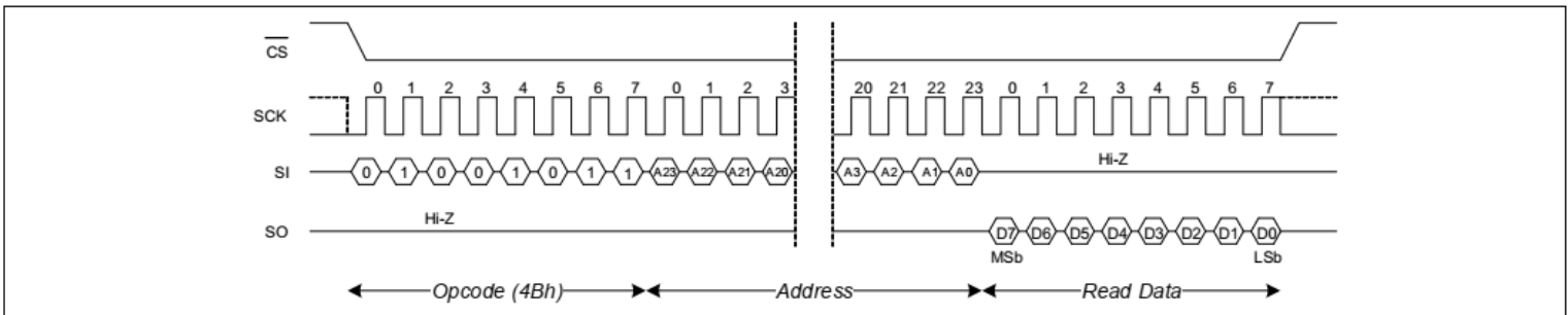
图 12 特殊扇区读操作
