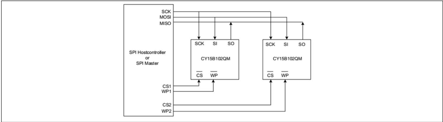
图 2 使用SPI端口的系统配置
