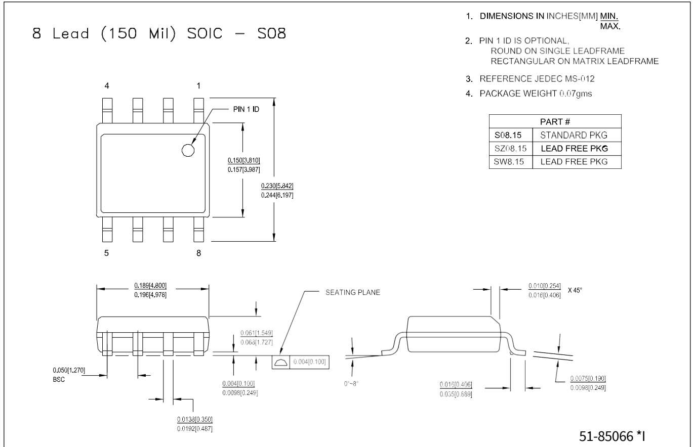
图 23 8 引脚SOIC (150 Mils) 封装外形图， 51-85066
