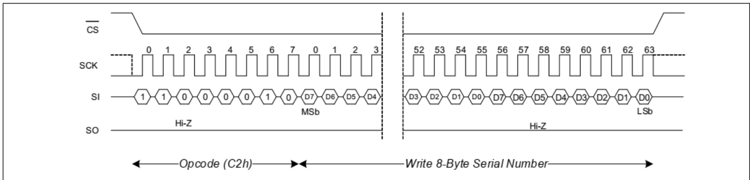
图 15 写入序列号操作
