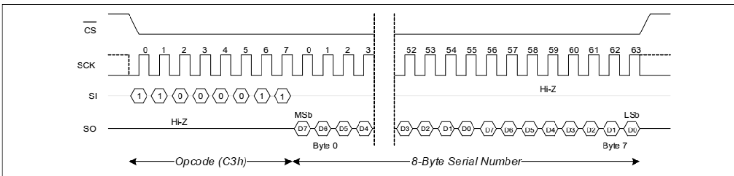
图16 读取序列号操作
