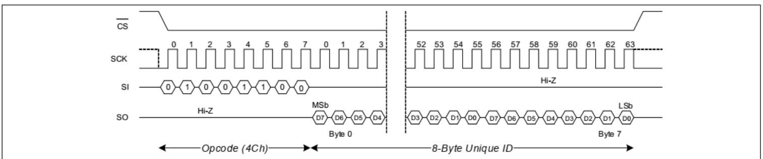
图 14 读取唯一 ID
