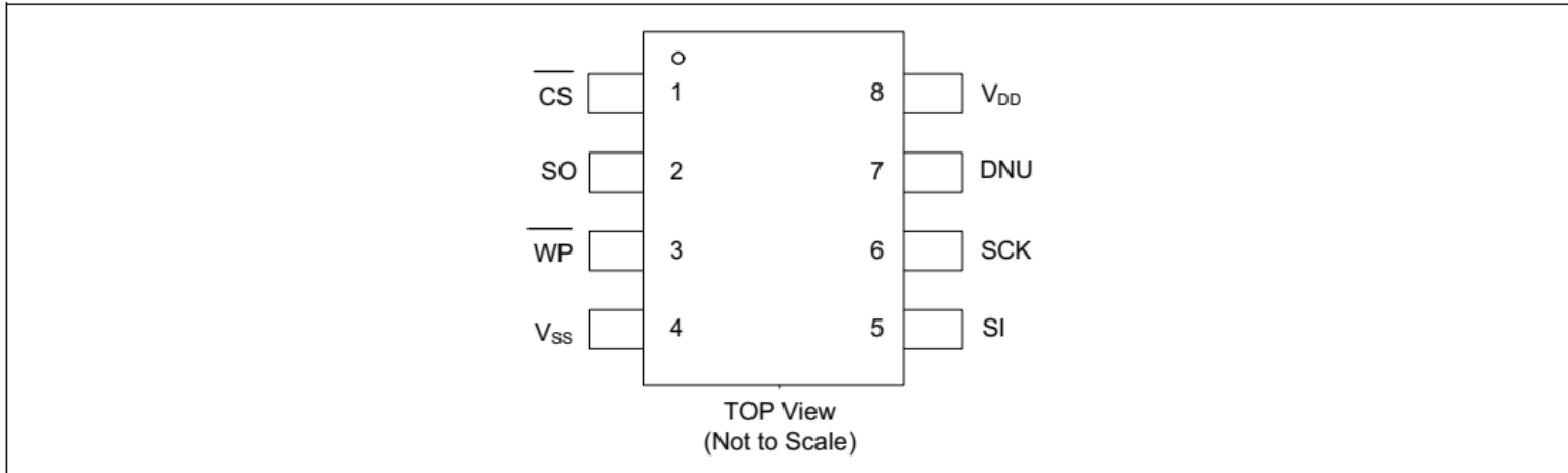
图 1 8 引脚 SOIC 引脚排列
