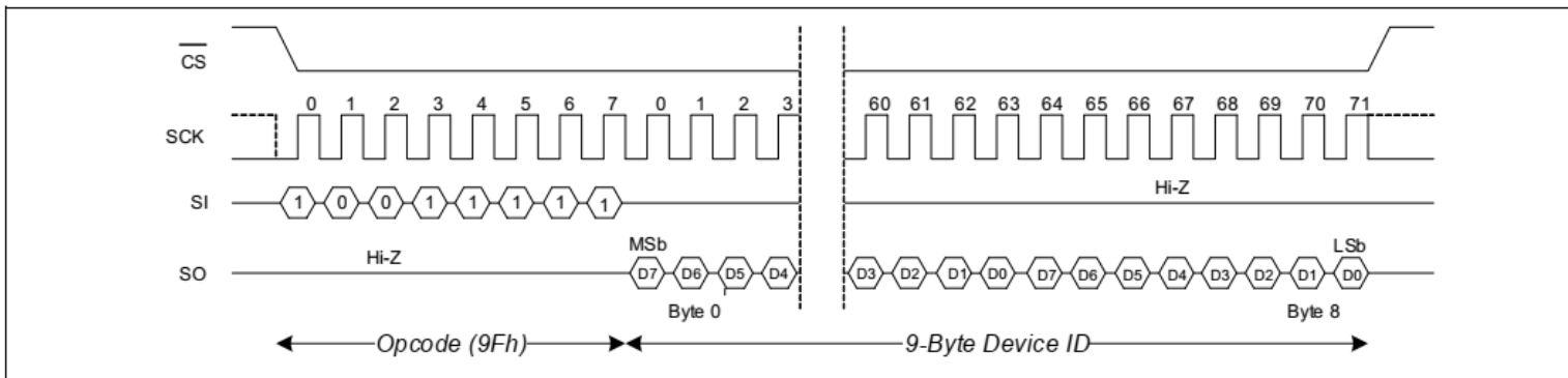
图 13 读取器件 ID
