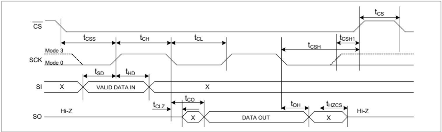
图 20 同步数据时序 (模式 0 和模式 3)
