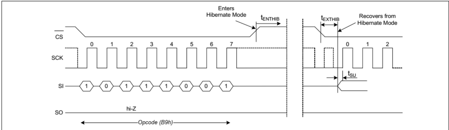
图 19 休眠模式操作
