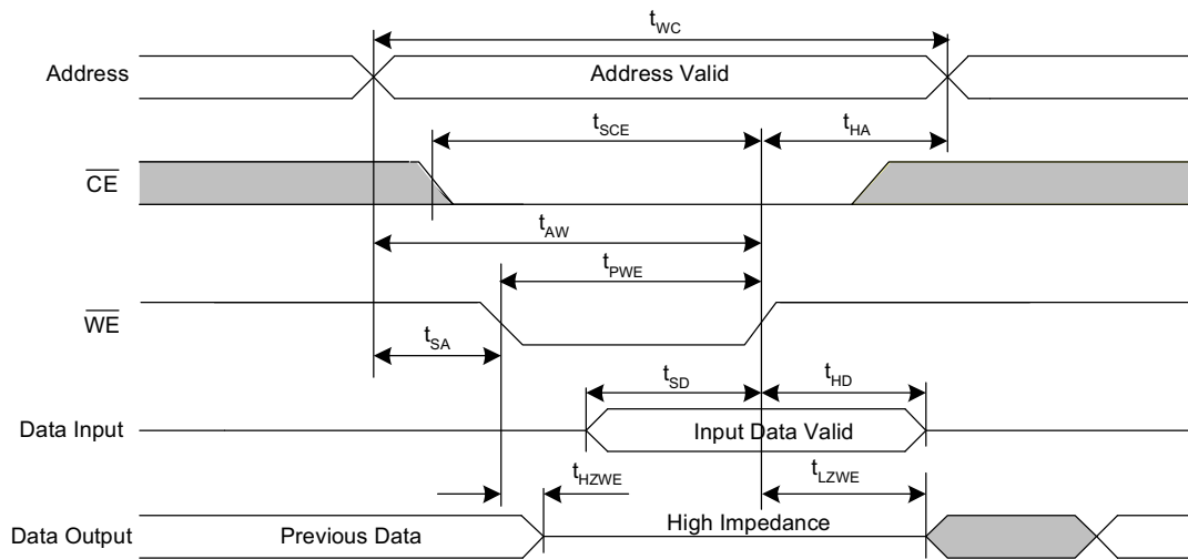
图 7. SRAM 写周期 #2 ( \overline{\text{CE}} 控制) [22, 23, 24]
