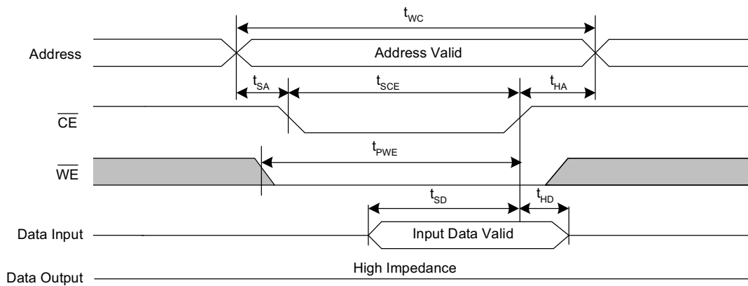
图 7. SRAM 写周期 #2 ( \overline{\text{CE}} 控制) [22, 23, 24]
