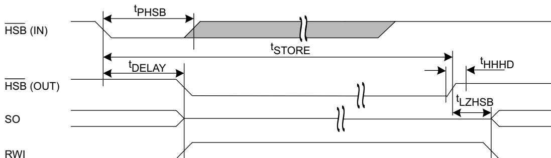
图 11. 硬件存储周期 [36]
