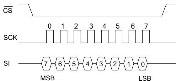
図 4. SPI モード 0
