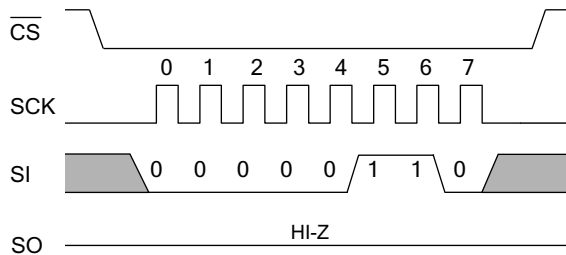
図 9. WREN 命令
