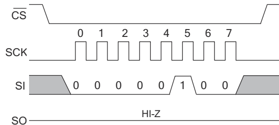
図 10. WRDI 命令
