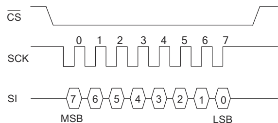
図 5. SPI モード 3
