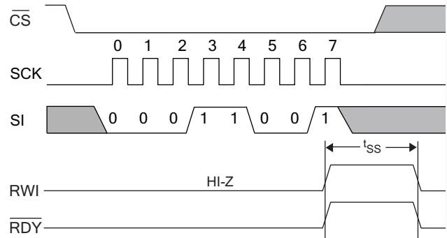
図 40. AutoStore ディスエーブルサイクル
