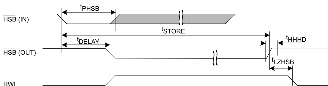
図 41. ハードウェア STORE サイクル [28]
