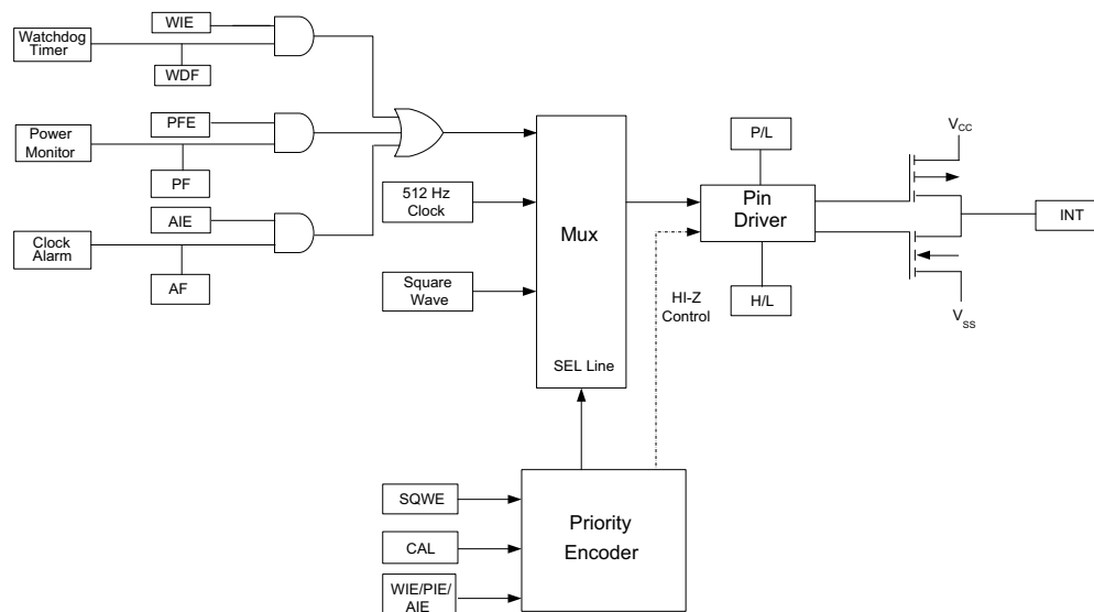
図 32. 割り込みブロック ダイアグラム
