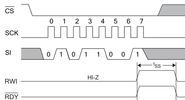
図 39. AutoStore イネーブルサイクル
