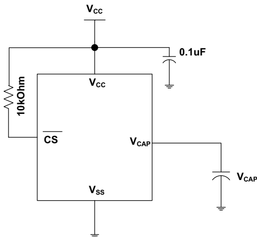
図 2. AutoStore モード
