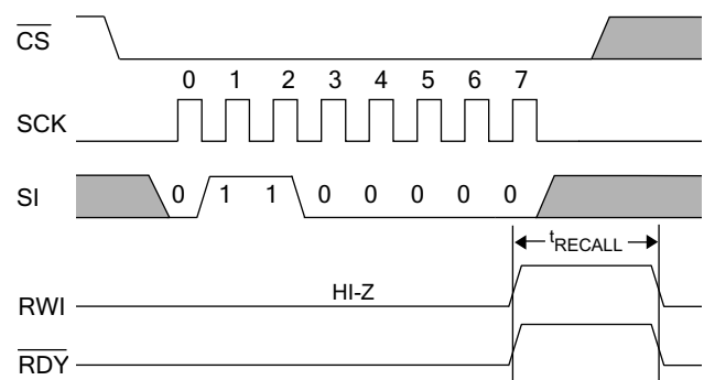
図 38. ソフトウェア RECALL サイクル [27]
