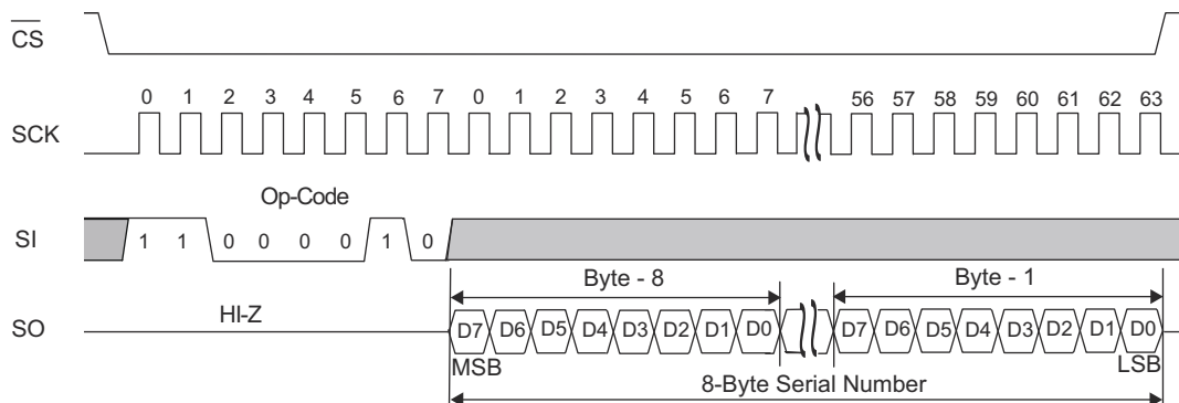
図 25. RDSN 命令
