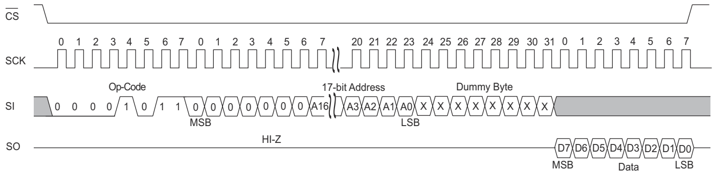
図 13. 高速読み取り命令タイミング
