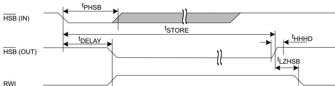
Figure 32. Hardware STORE Cycle [28]
